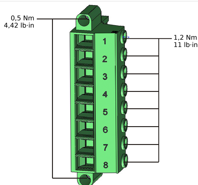
Fig. 146: Bornes de mesure de tension de la carte de mesure « TU » (↳ « 2.6.1 TU - Entrées de mesure de tension »).
