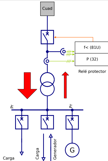
Fig. 103: Reducción de carga centralizada por subfrecuencia en redes eléctricas con alimentación temporal
