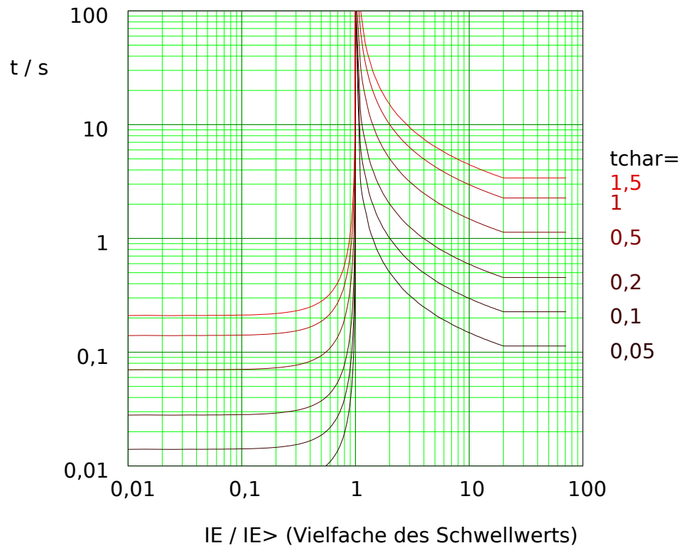
Abb. 82: NINV: Rückfallverzögerung (linke Hälfte, IE < IE> ) und Auslöseverzögerung (rechte Hälfte, IE > IE> ), Beispieldiagramm für I_{E,max} = 20 \cdot IE> .
