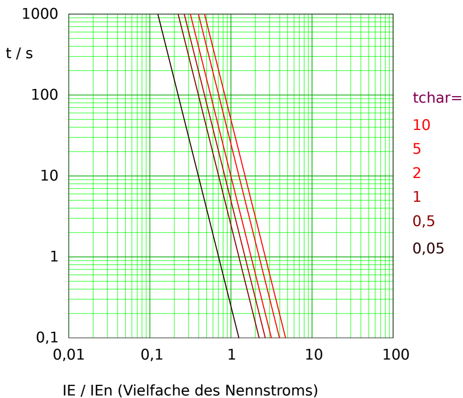
Abb. 94: Auslösekurve „I4T“, wobei nur der Bereich IE > IE_{n>} jeweils anwendbar ist. Beispieldiagramm für gemessenen (nicht empfindlichen) Erdstrom.
