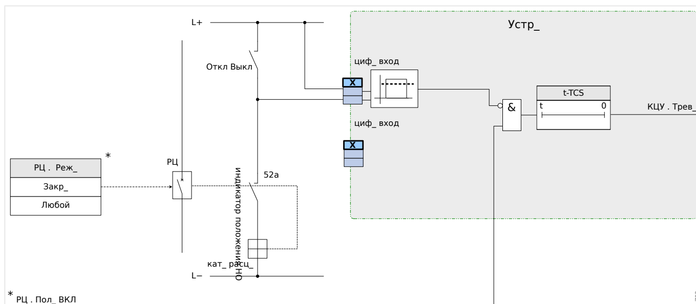
Рис. 116: Пример соединения: контроль цепи отключения только с одним вспомогательным контактом выключателя «Всп Вкл» (52а).
