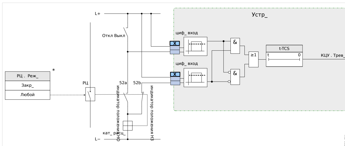
Рис. 115: Пример соединения: контроль цепи отключения с двумя вспомогательными контактами выключателя «Всп Вкл» (52а) и «Всп Выкл» (52b).
