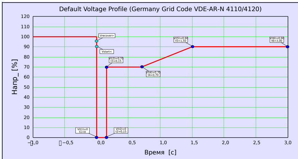
Рис. 80: Профиль LVRT по умолчанию (тип I).
