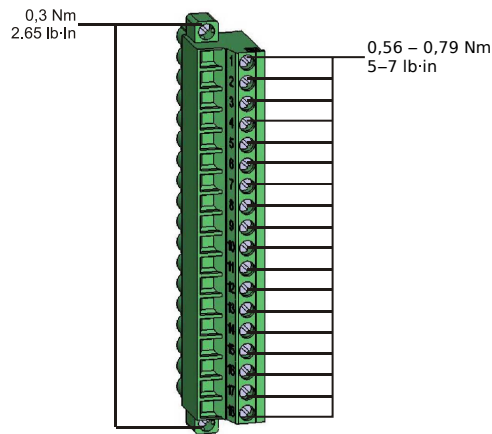
Рис. 139: Измерительные контакты плат измерения напряжения «TU-OR5» и «TU-DI8».
