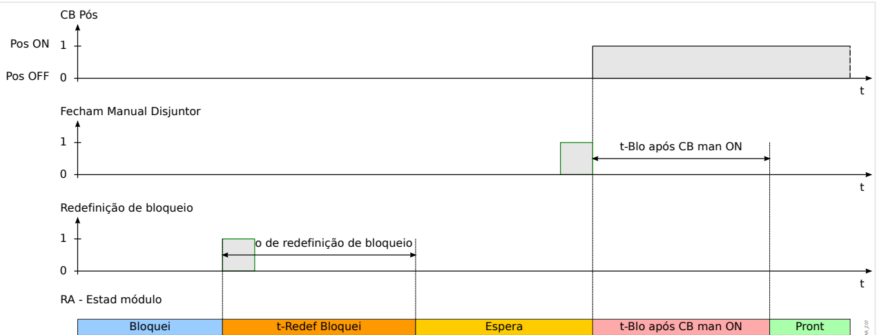
Fig. 107: A lógica de reinicialização de travamento no caso do reinício do travamento vir antes do fechamento manual do disjuntor
