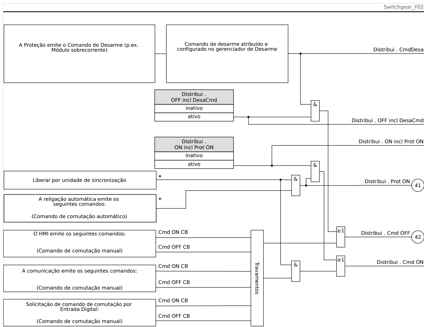
Fig. 122: Travamentos (Peças rotuladas com “*”: a disponibilidade depende do tipo de dispositivo solicitado.)
