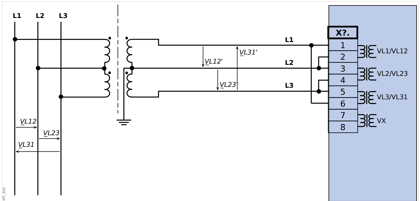
Fig. 34: Medição de voltagem bifásica - fiação das entradas de medição: "Delta Aber"
