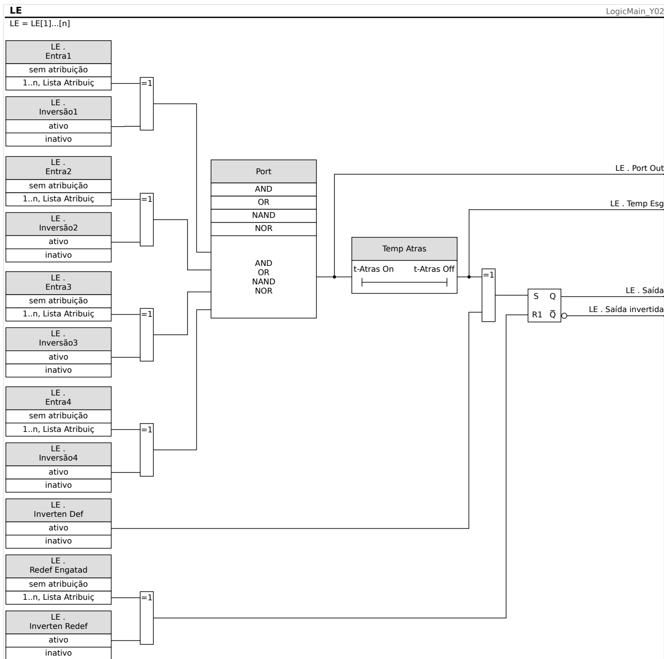
Fig. 131: Visão Geral Detalhada - Diagrama Lógico Geral.
