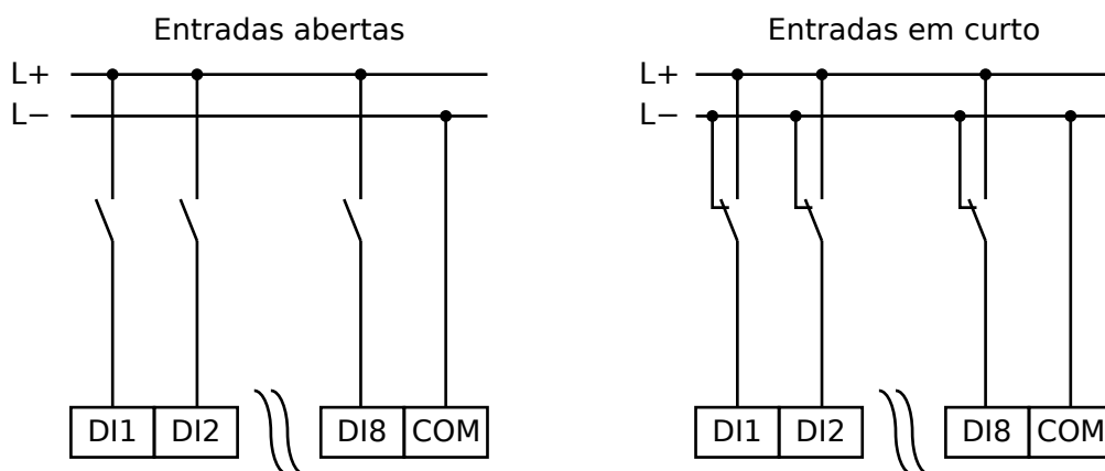
Fig. 140: Estado seguro das entradas digitais
