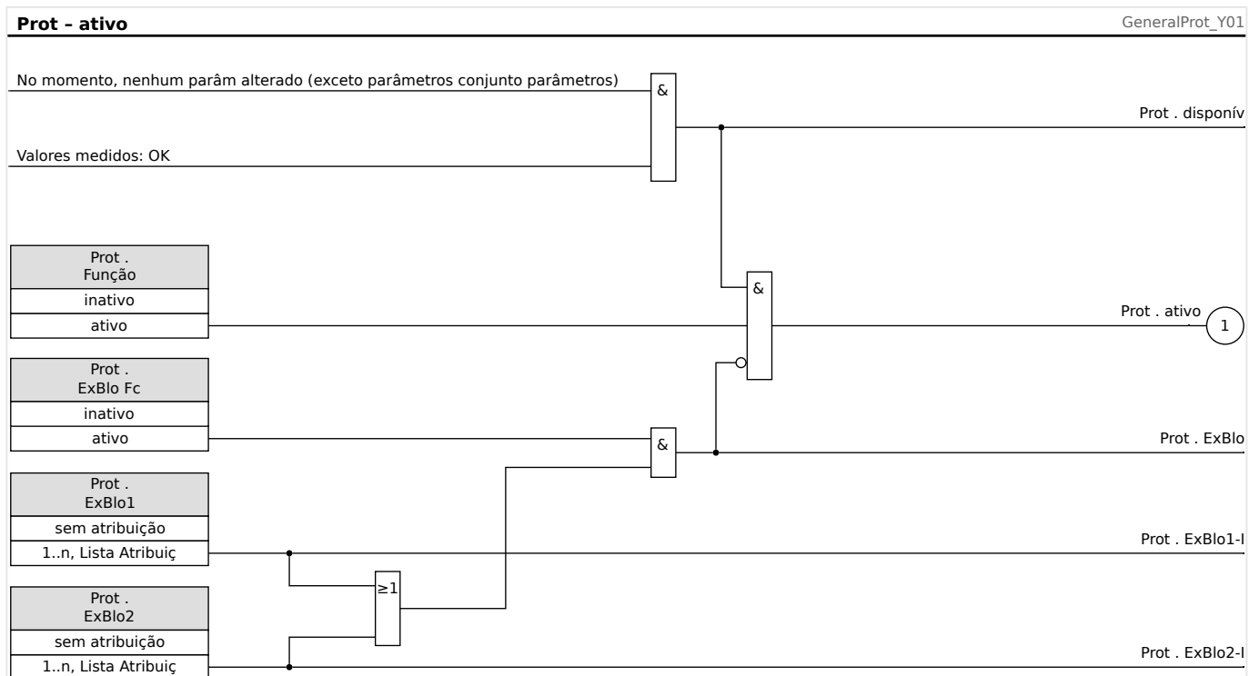
Fig. 60: Disponibilidade do módulo de proteção geral.
