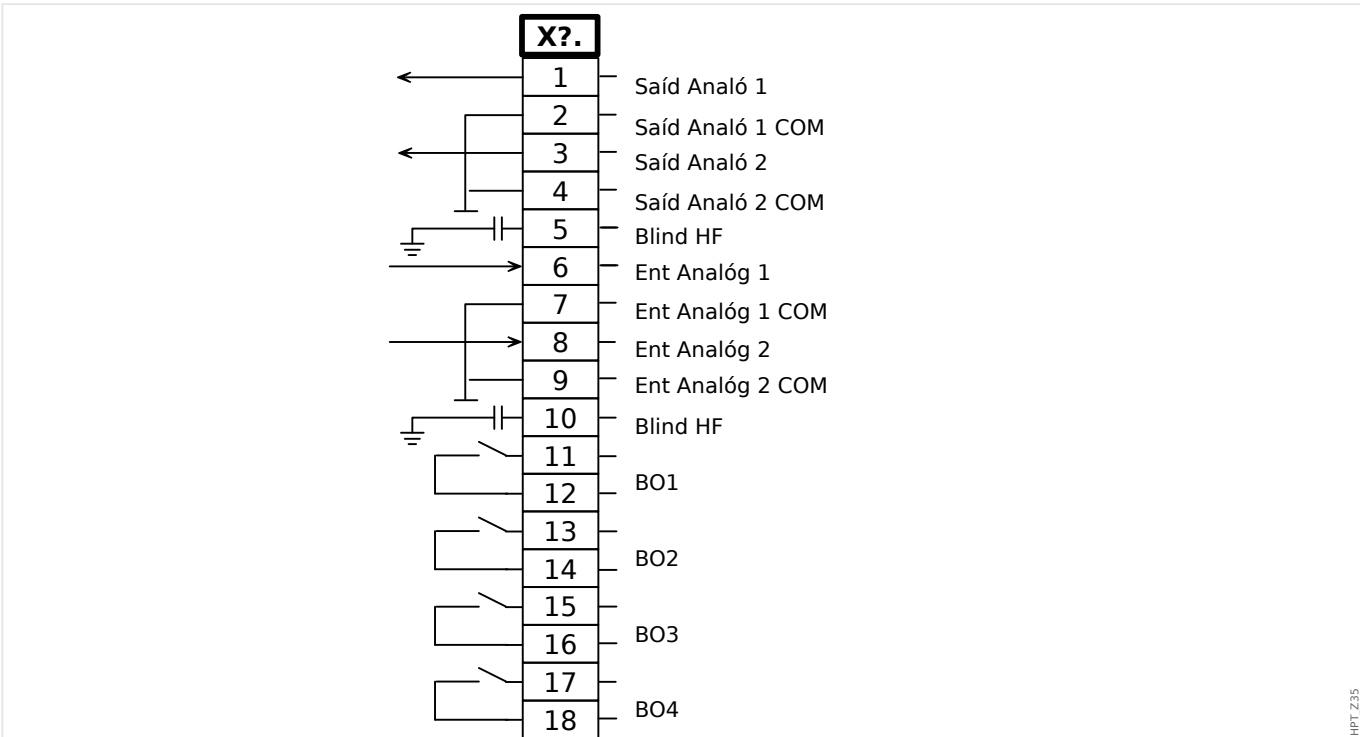
Fig. 38: Marcação de Terminal.
