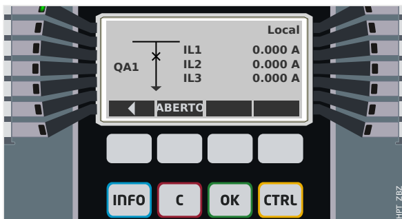
Fig. 119: Exemplo de página de controle, com o "Disjuntor" na posição fechada.
