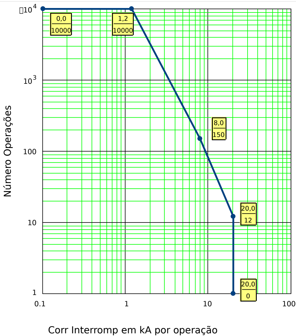
Fig. 124: Curva Manutenção de Disjuntor para Disjuntor normal 25kV
