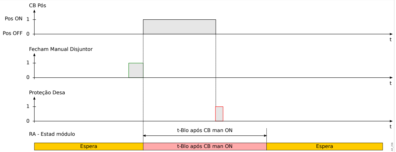
Fig. 106: Disparo de proteção enquanto o tempo de bloqueio de fechamento manual está cronometrando.
