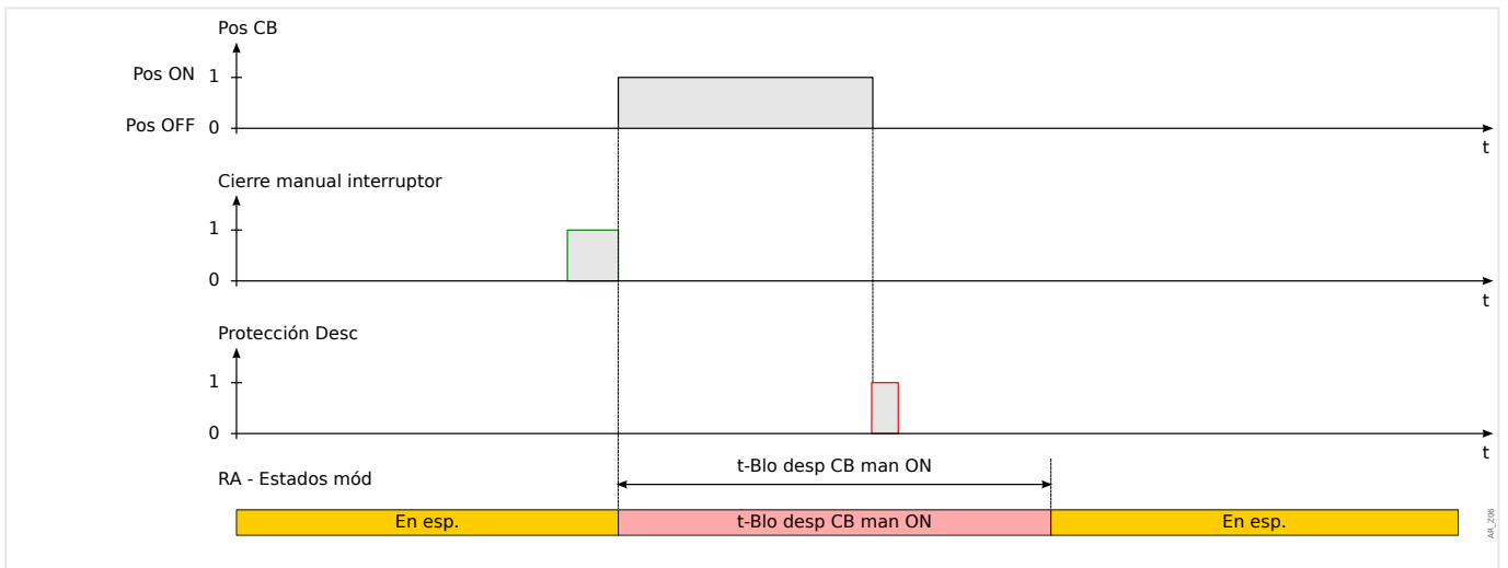
Fig. 106: Desconexión de protección mientras transcurre el tiempo de bloqueo de cierre manual.
