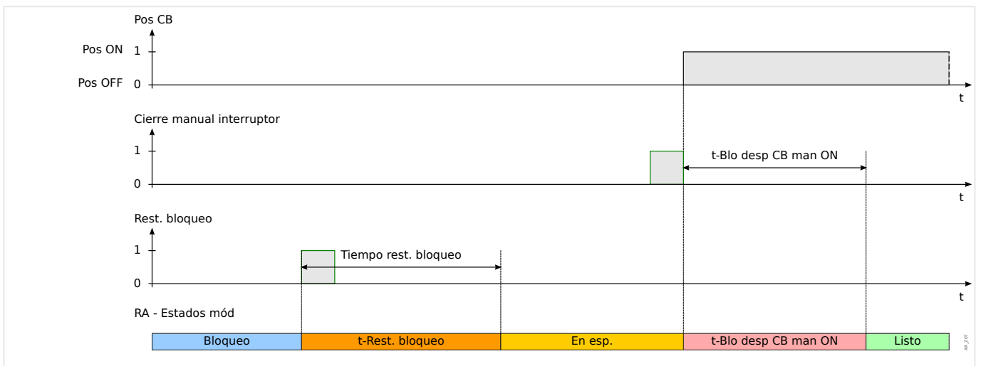
Fig. 107: Lógica de reinicio de bloqueo de AR en caso de que el reinicio de bloqueo llegue antes de que se cierre el interruptor manualmente.
