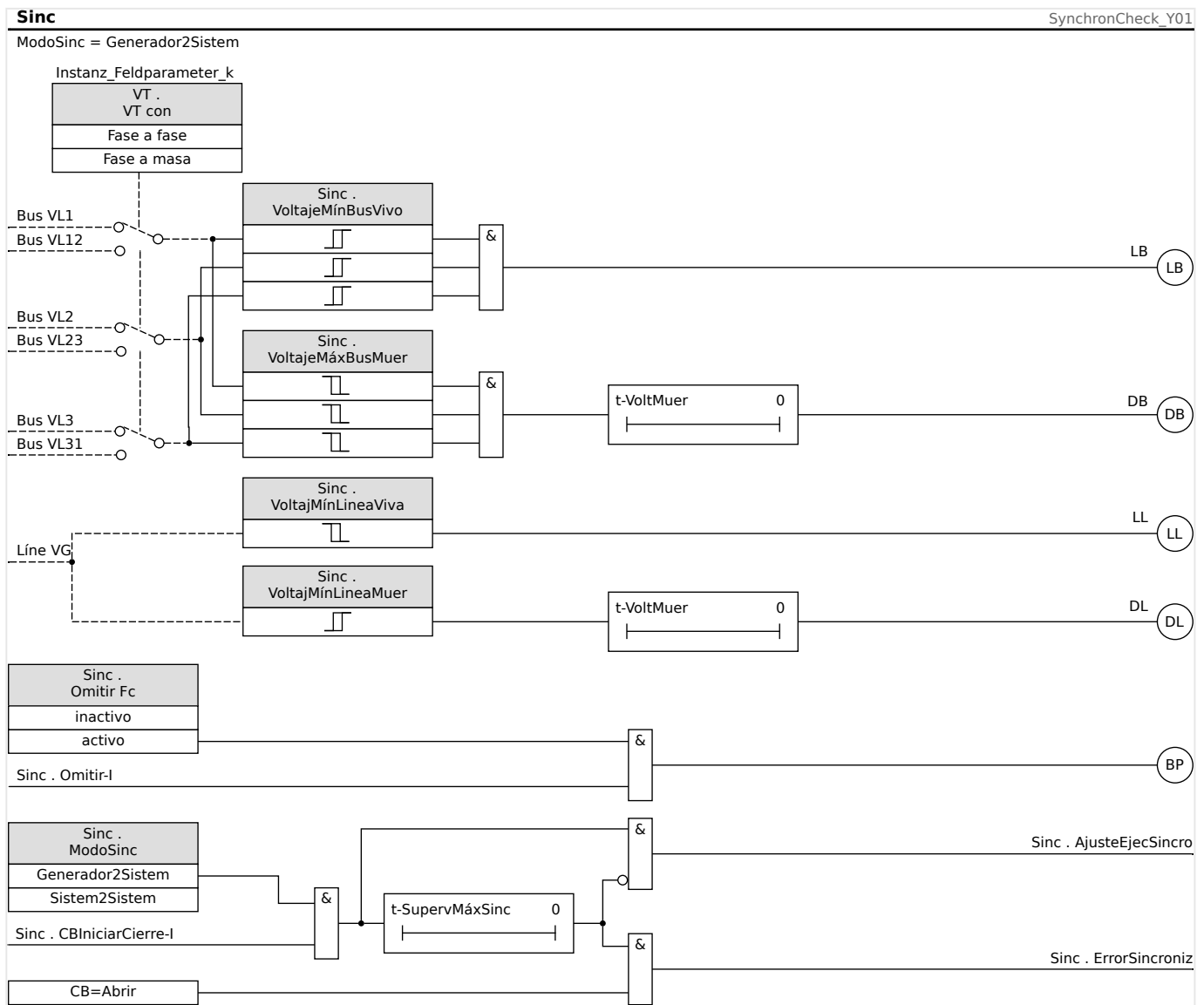
Fig. 111: Funcionalidad del módulo »Sinc«, «Generador2Sistem».
