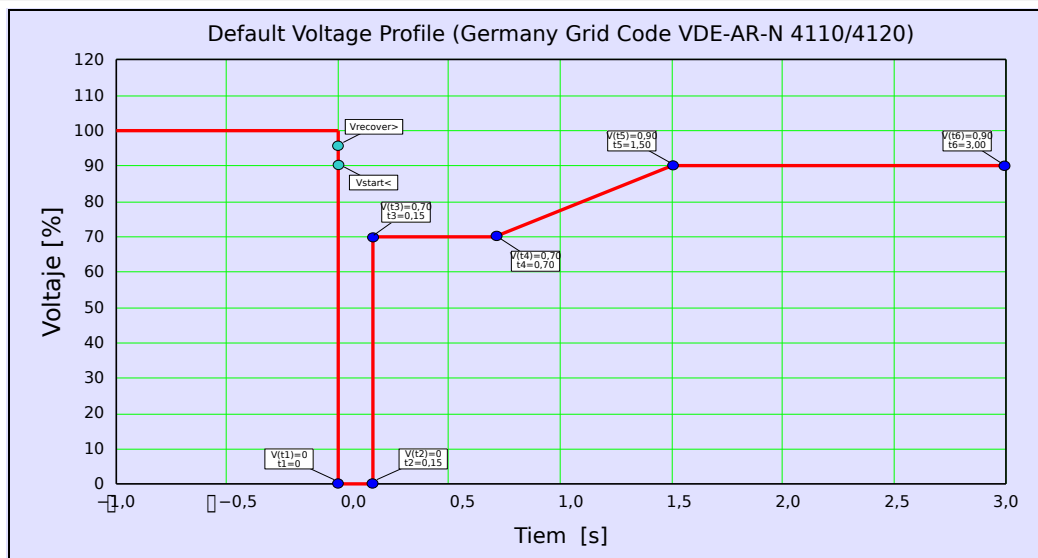
Fig. 80: Perfil de LVRT predeterminado (Tipo I).
