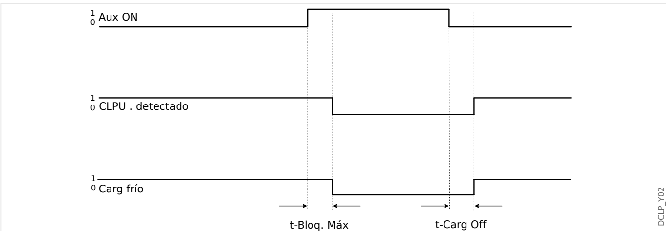
Fig. 113: Modo de ejemplo: Posición de interruptor.
