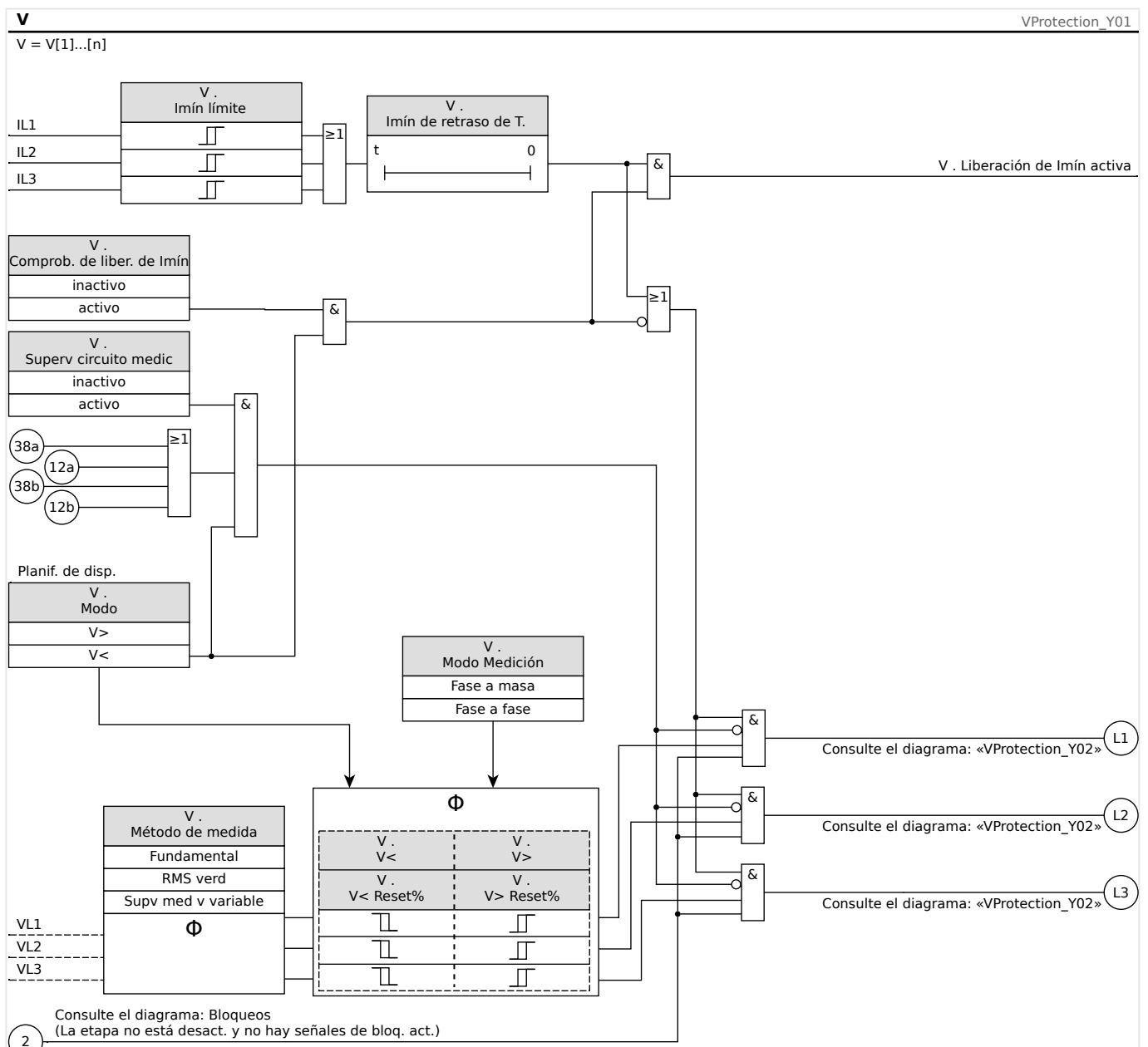
Fig. 74: Funcionalidad del módulo de protección de tensión, parte 1.
