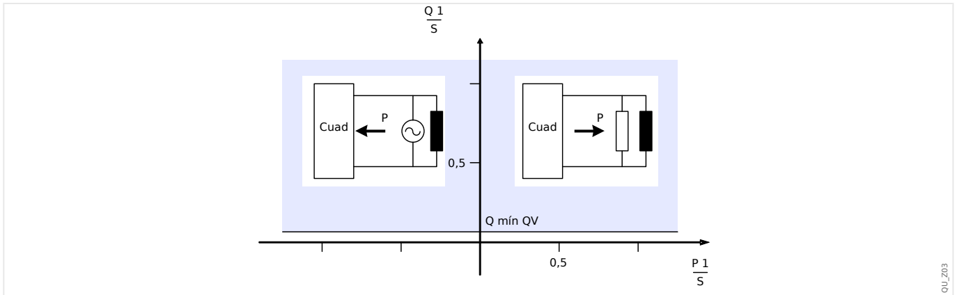
Fig. 92: Método 2: Supervisión de potencia reactiva pura.
