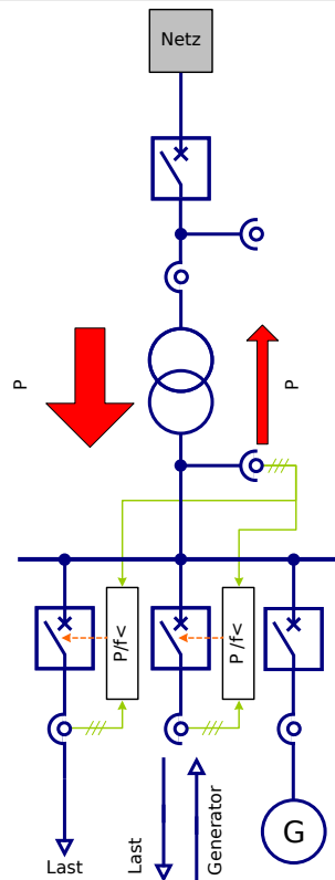
Abb. 96: Dezentrale Automatische Frequenzentlastung in Netzen mit zeitweiser Rückspeisung.
