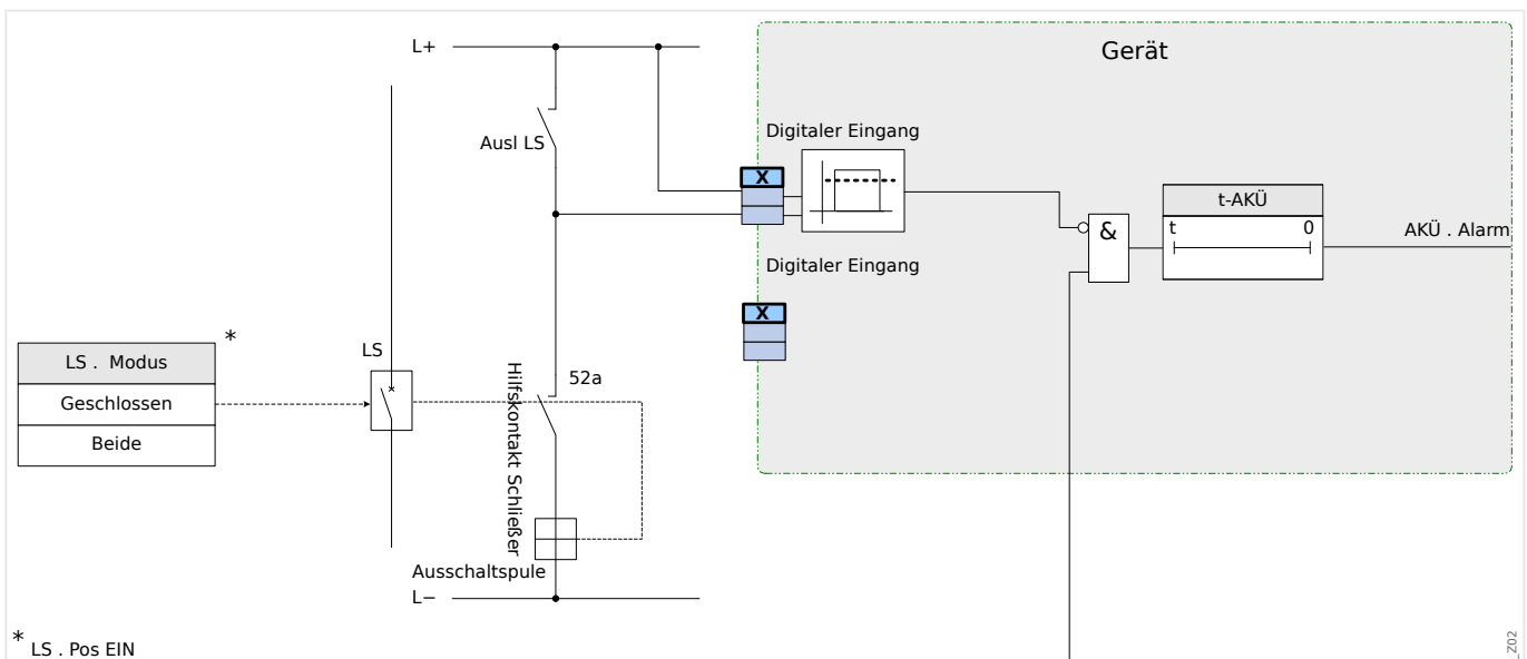
Abb. 116: Anschlussbeispiel: Auslösekreisüberwachung mit einem Hilfskontakt »Hiko EIN« (52a).
