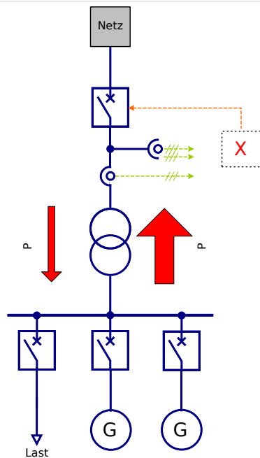
Abb. 97: Zentraler Einsatz in Teilnetzen mit überwiegender Rückspeisung.
