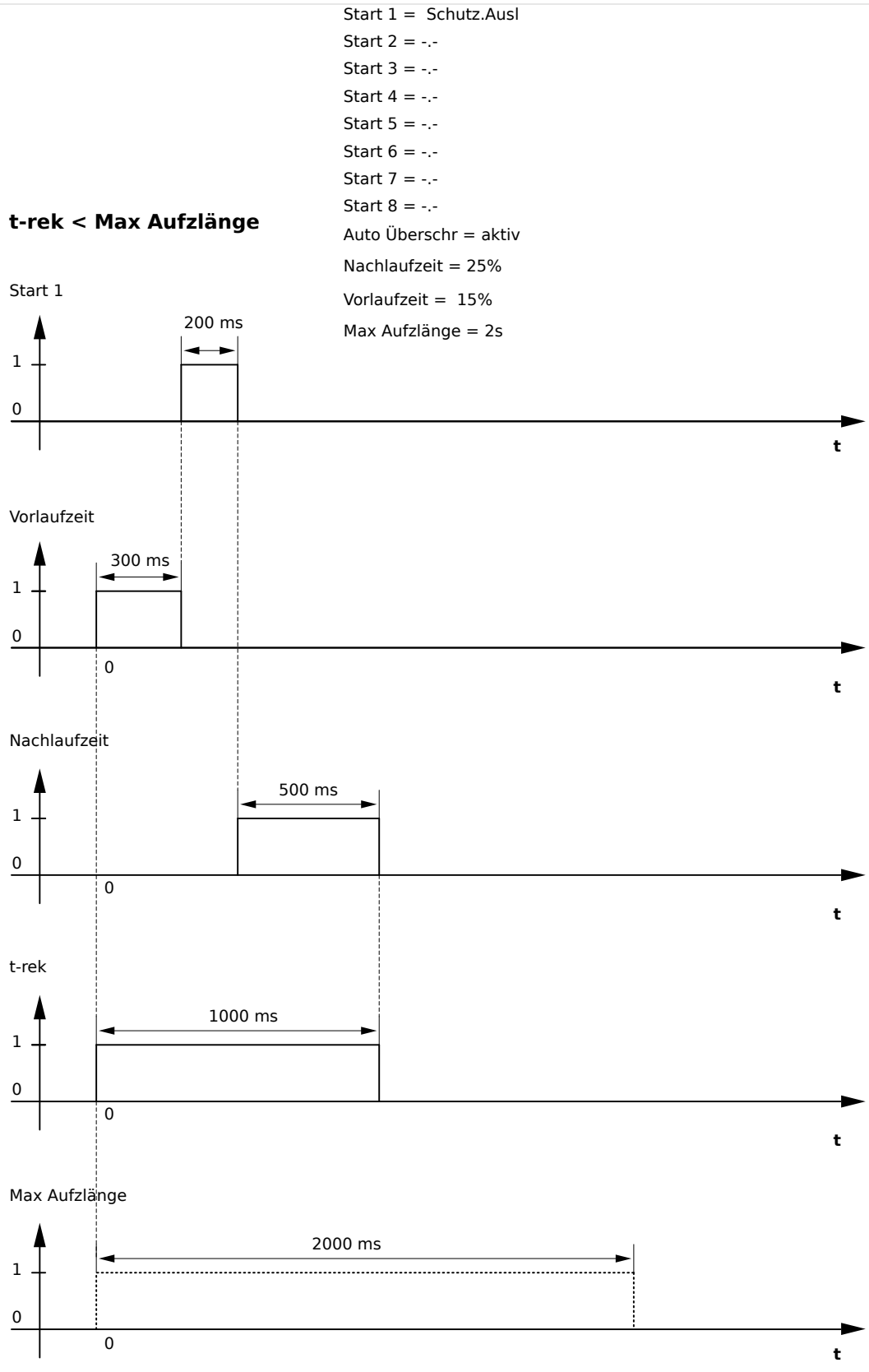
Abb. 128: Beispiel II Störschreiber-Ablaufdiagramm
