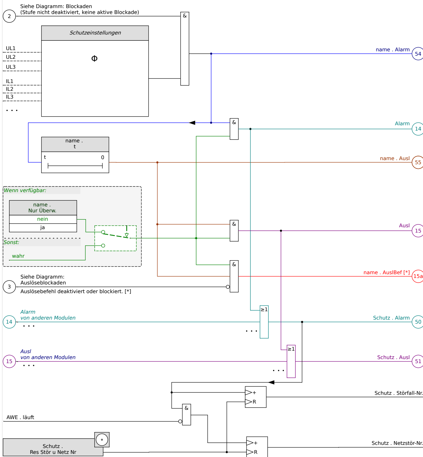
Abb. 61: Grobe Skizze der Funktionalität einer HighPROTEC-Schutzfunktion.
