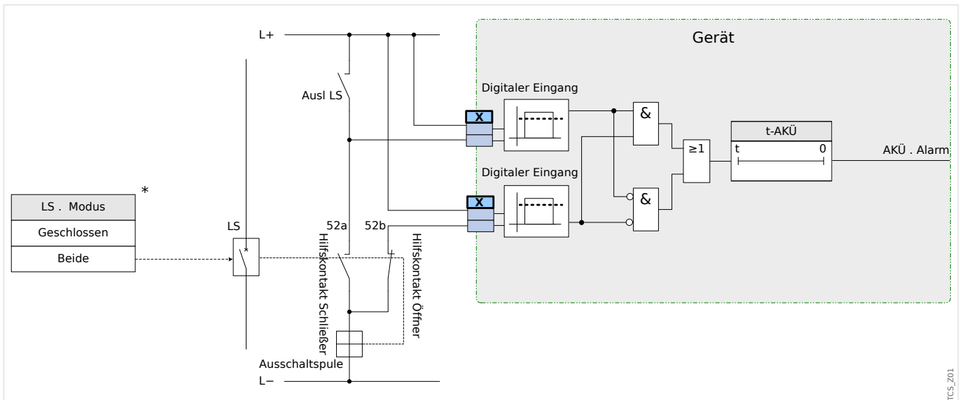
Abb. 115: Anschlussbeispiel (Empfehlung): Auslösekreisüberwachung mit zwei Hilfskontakten »Hiko EIN« (52a) und »Hiko AUS« (52b).
