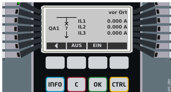
Abb. 120: Beispiel einer Steuer-Seite mit „Leistungsschalter“ in Störstellung (bzw. unplausiblem Zustand).
