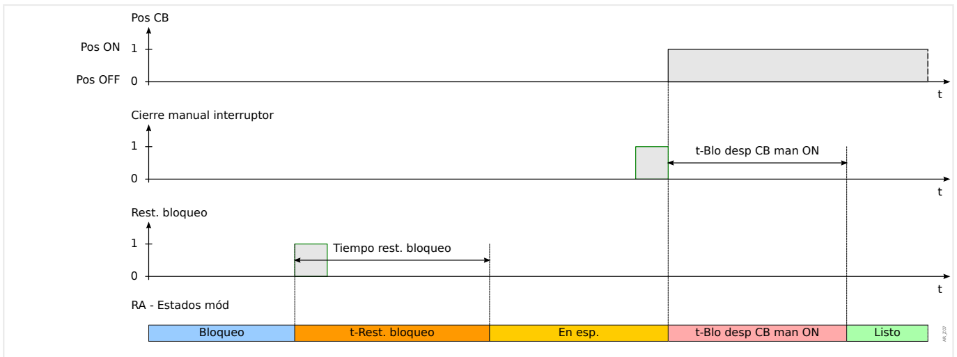
Fig. 106: Lógica de reinicio de bloqueo de AR en caso de que el reinicio de bloqueo llegue antes de que se cierre el interruptor manualmente.
