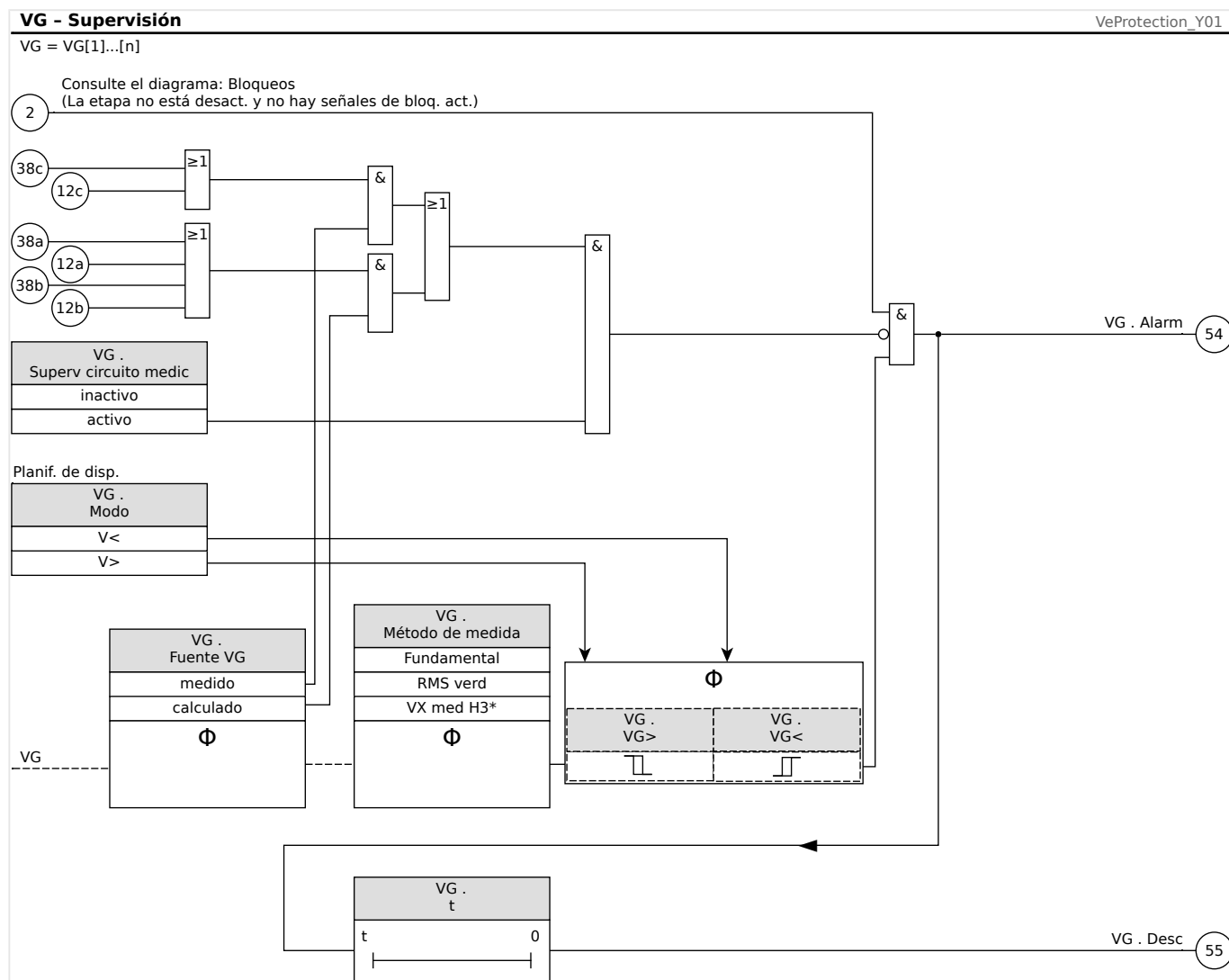
Fig. 80: VG, VX Supervisión de tensión, parte 1 (función de supervisión, decisión de desconexión).
