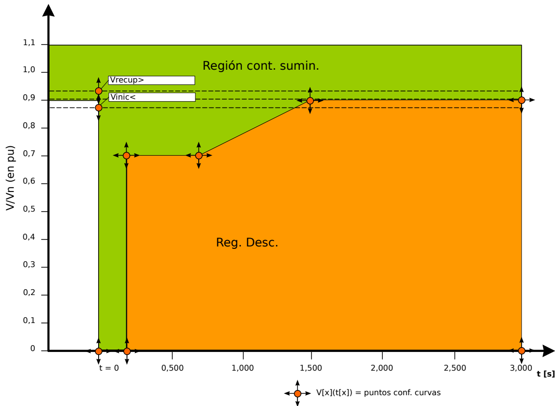
Fig. 78: Regiones de continuidad y desconexión.
