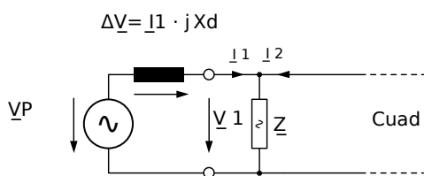
Fig. 83: Circuito equivalente en generador sincrónico en paralelo con la red de suministro eléctrico.
