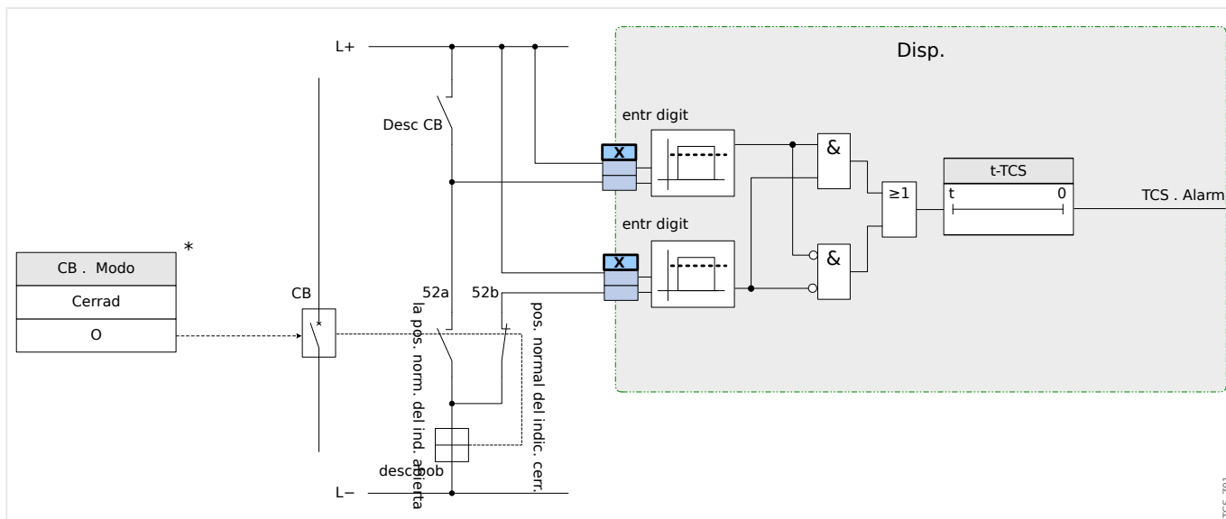
Fig. 114: Ejemplo de conexión: Supervisión del circuito de desconexión con dos contactos auxiliares CB »Aux ON« (52a) and »Aux OFF« (52b).
