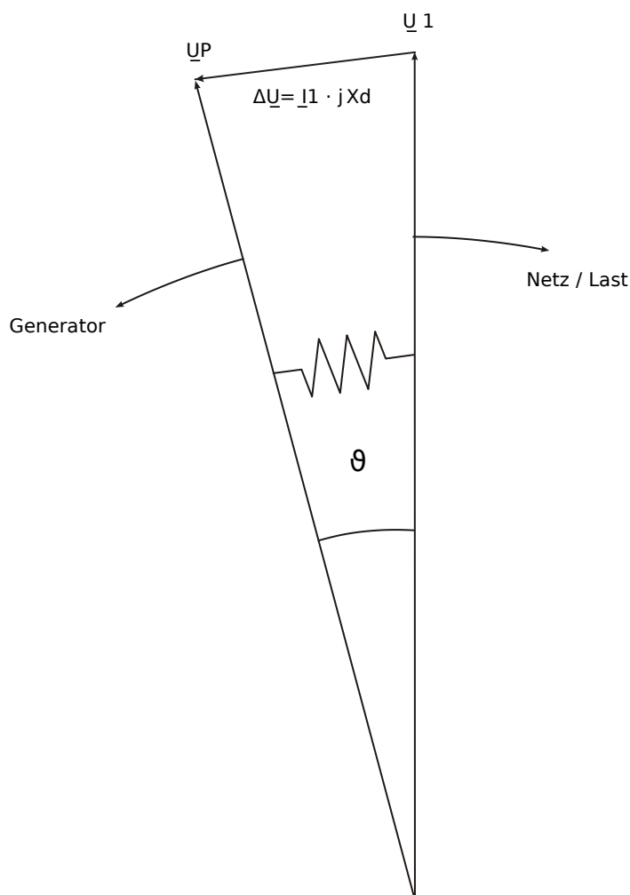
Abb. 90: Polradwinkel bei konstanter Belastung des Generators.
