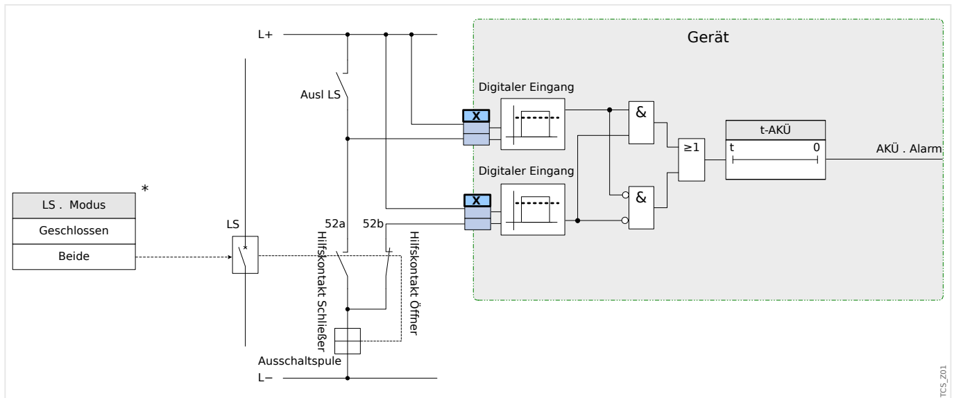
Abb. 117: Anschlussbeispiel (Empfehlung): Auslösekreisüberwachung mit zwei Hilfskontakten »Hiko EIN« (52a) und »Hiko AUS« (52b).
