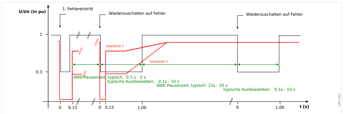
Abb. 111: Spannungsverlauf während einer zweischüssigen, nicht erfolgreichen AWE, aus: Technische Richtlinie, Erzeugungsanlagen am Mittelspannungsnetz, Ausgabe Juni 2008, BDEW Bundesverband der Energie- und Wasserwirtschaft e.V. (Page 89).
