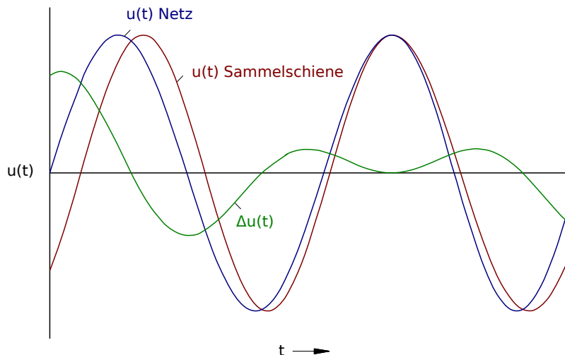
Abb. 96: Spannungsverlauf der Schwebespannung \Delta u(t) , vergrößert.
