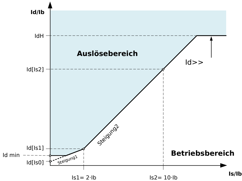
Abb. 75: Unstabilisierte Hochstromdifferenzialstufe I_{dH} .
