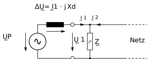
Abb. 89: Ersatzschaltbild netzparalleler Synchrongenerator
