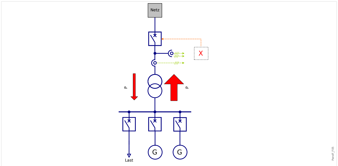
Abb. 106: Zentraler Einsatz in Teilnetzen mit überwiegender Rückspeisung.
