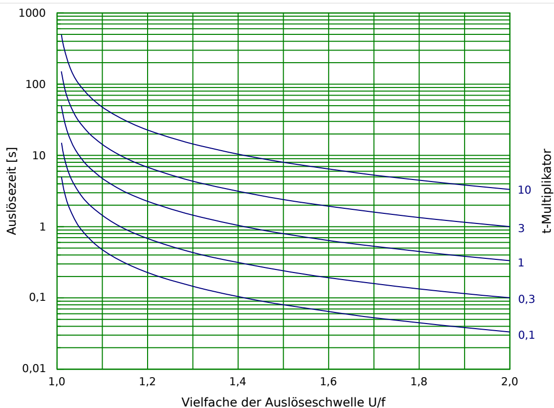
Abb. 81: Charakteristik/Kennlinie: INV A
