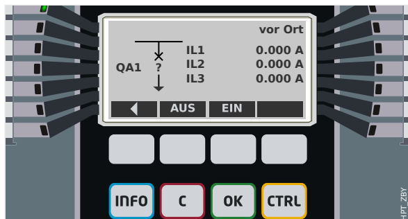
Abb. 122: Beispiel einer Steuer-Seite mit „Leistungsschalter“ in Störstellung (bzw. unplausiblem Zustand).
