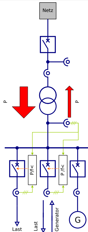
Abb. 105: Dezentrale Automatische Frequenzentlastung in Netzen mit zeitweiser Rückspeisung.
