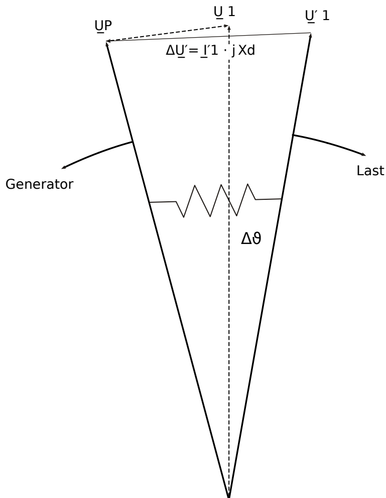
Abb. 92: Änderung des Polradwinkels bei plötzlicher Belastung des Generators.
