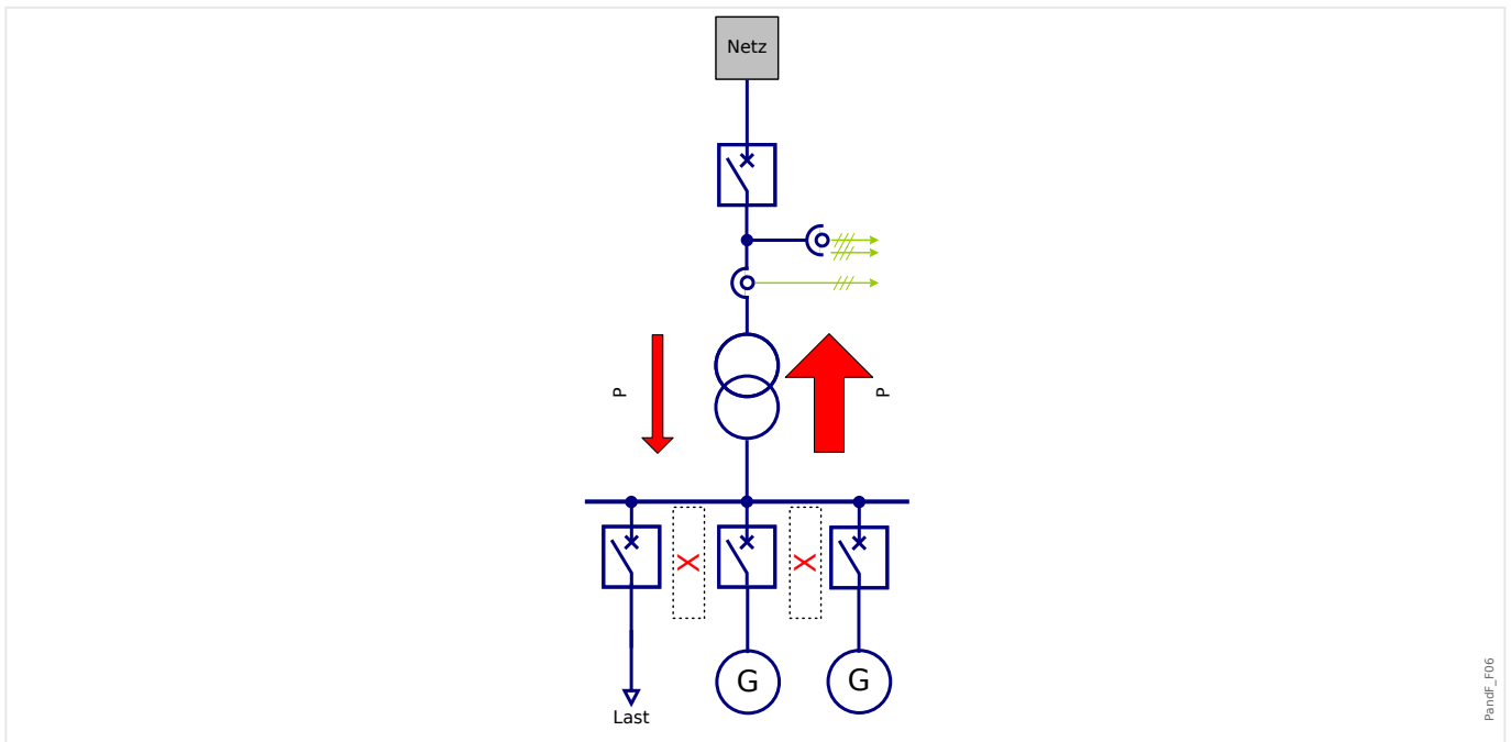
Abb. 107: Dezentraler Einsatz in Teilnetzen mit überwiegender Rückspeisung.
