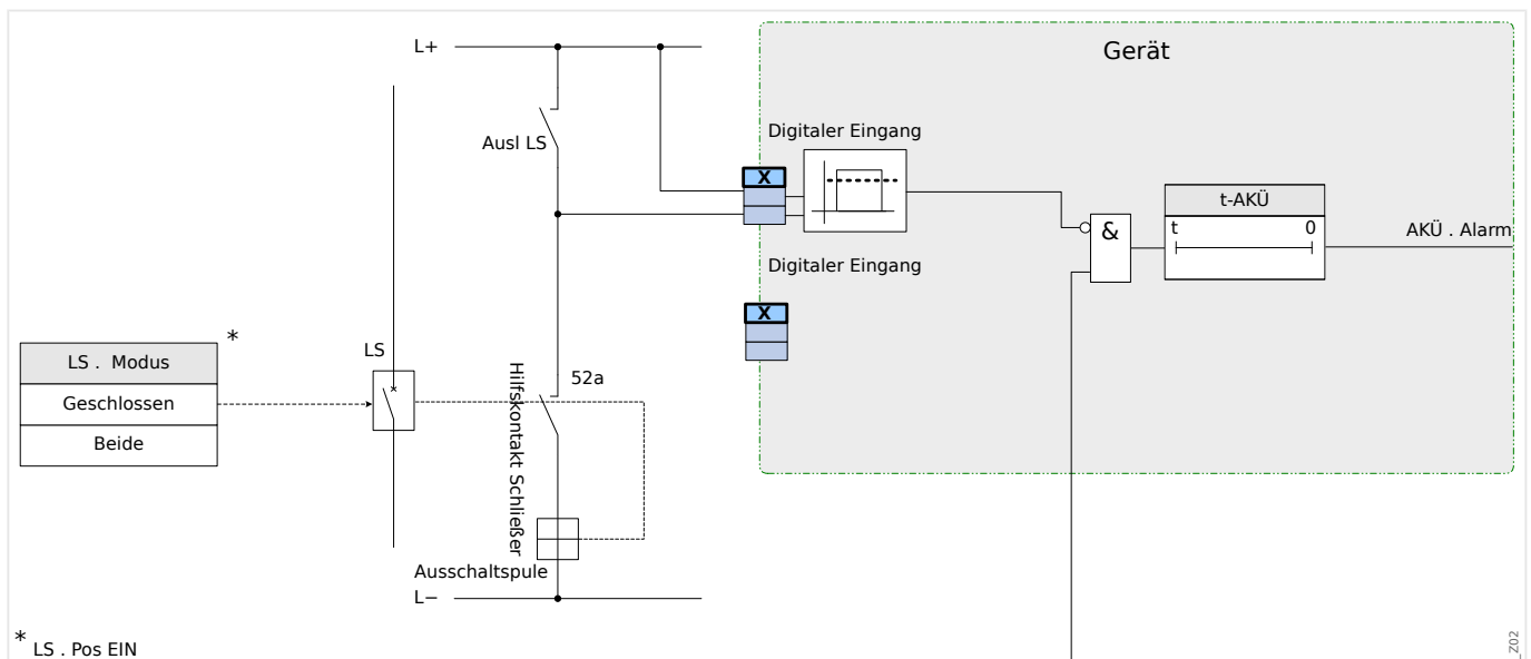
Abb. 118: Anschlussbeispiel: Auslösekreisüberwachung mit einem Hilfskontakt »Hiko EIN« (52a).
