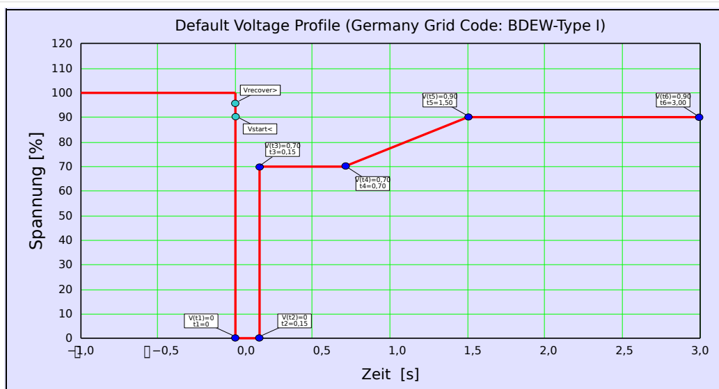
Abb. 113: LVRT-Werkseinstellung (BDEW-Typ-I).
