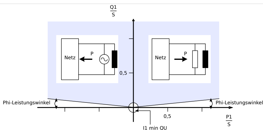
Abb. 100: Variante 1: Leistungswinkelüberwachung.
