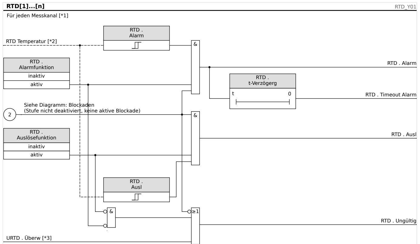
Abb. 116: Generelles RTD-Funktionsprinzip.
