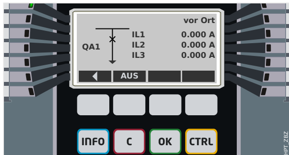
Abb. 121: Beispiel einer Steuer-Seite mit geschlossenem „Leistungsschalter“.
