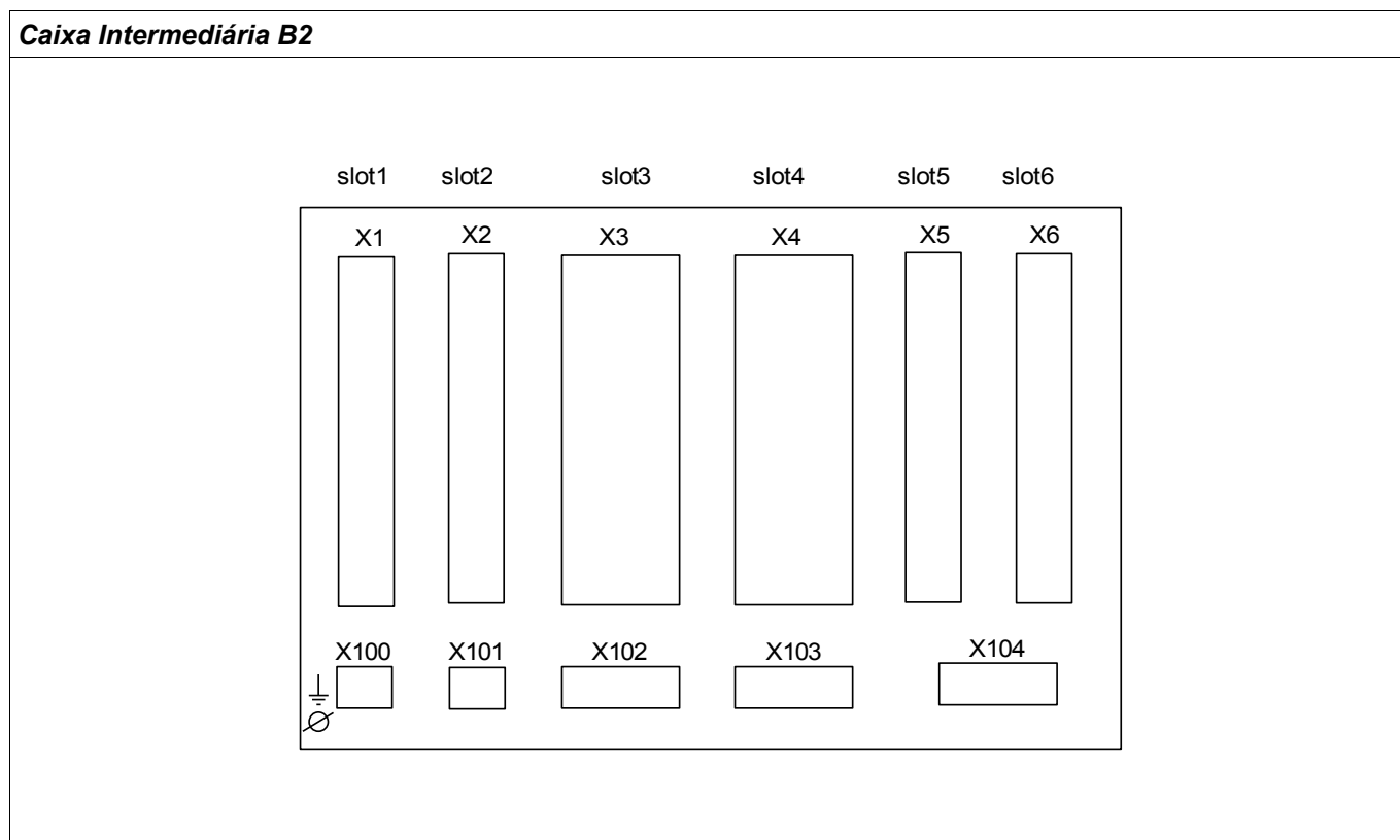
Vista traseira da caixa B2
