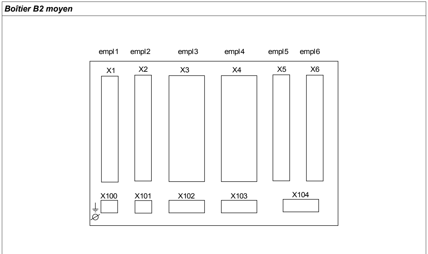
Vue arrière du boîtier B2
