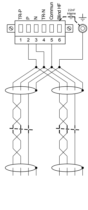
Blindage côté esclave bus connect aux résist terminaison de terre inutilisé
