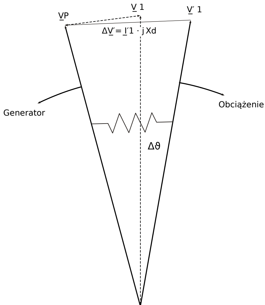
Rys. 103: Wektory napięcia przy awarii sieci.
