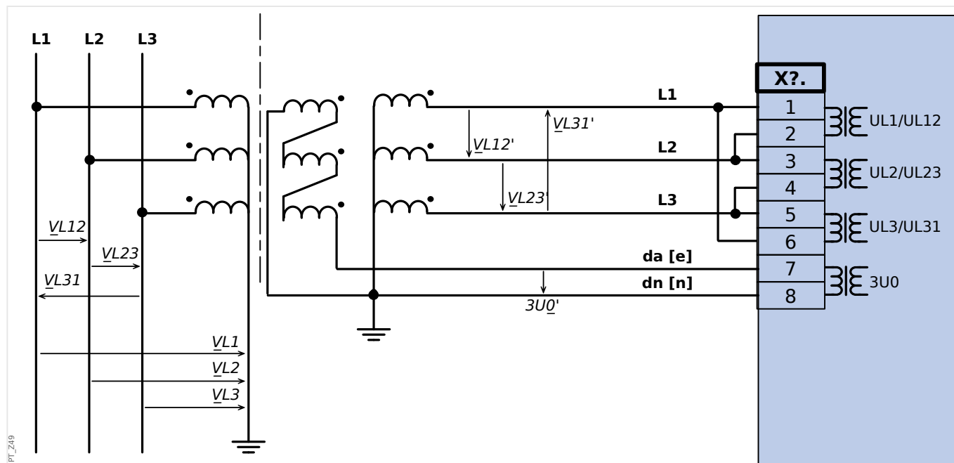
Rys. 37: Trójfazowy pomiar napięcia w układzie trójkąta: połączenie przewodów wejść pomiarowych: "połączenie w trójkąt" Pomiar 3U0 napięcia szczytkowego poprzez dodatkowe uzwojenia (e-n) w układzie otwartego trójkąta
