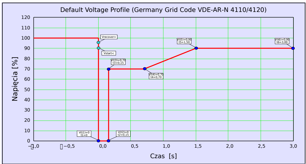
Rys. 124: Profil domyślny LVRT (typ I).
