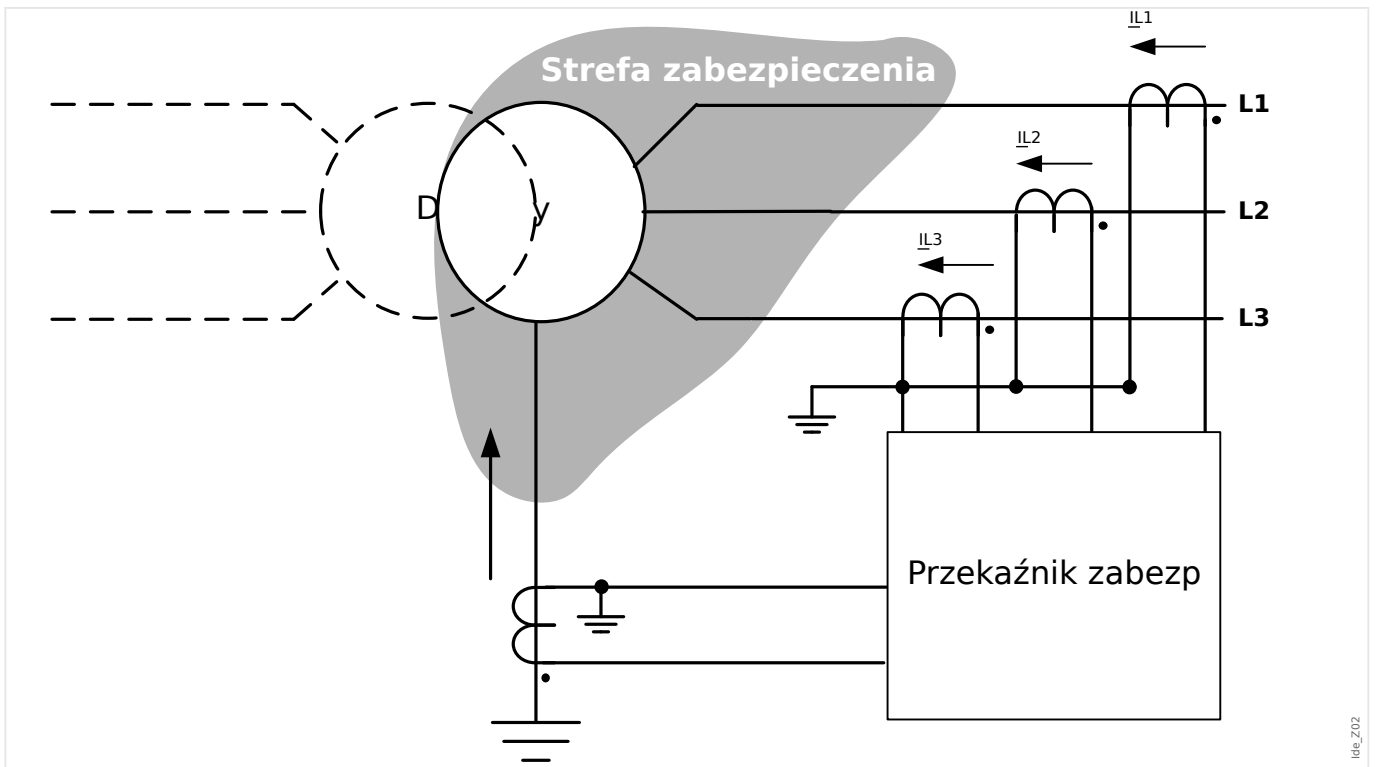
Rys. 79: Zasada działania zabezpieczenia różnicowego ziemnozwarciowego w uzwojeniach transformatorów połączonych w gwiazdę.
