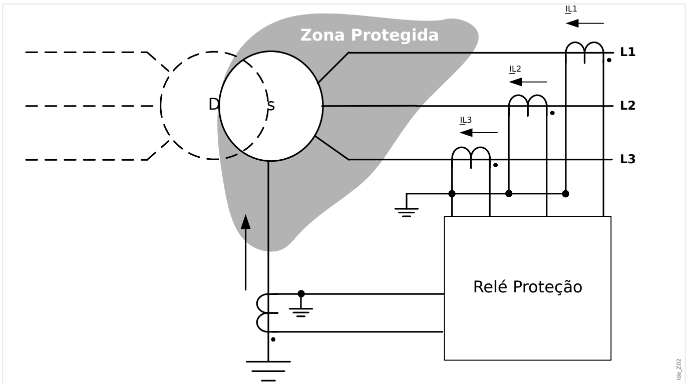
Fig. 77: Princípio de Proteção da Proteção Diferencial de Corrente de Aterramento no enrolamento lateral wye do transformador.
