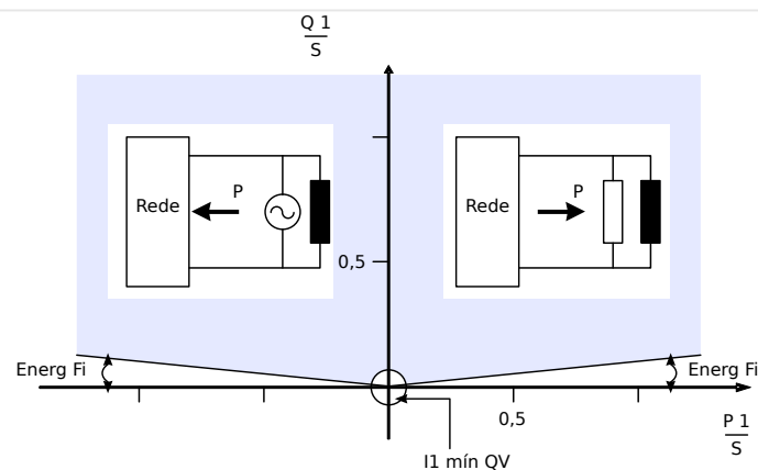
Fig. 101: Método 1: Supervisão Âng Energ.
