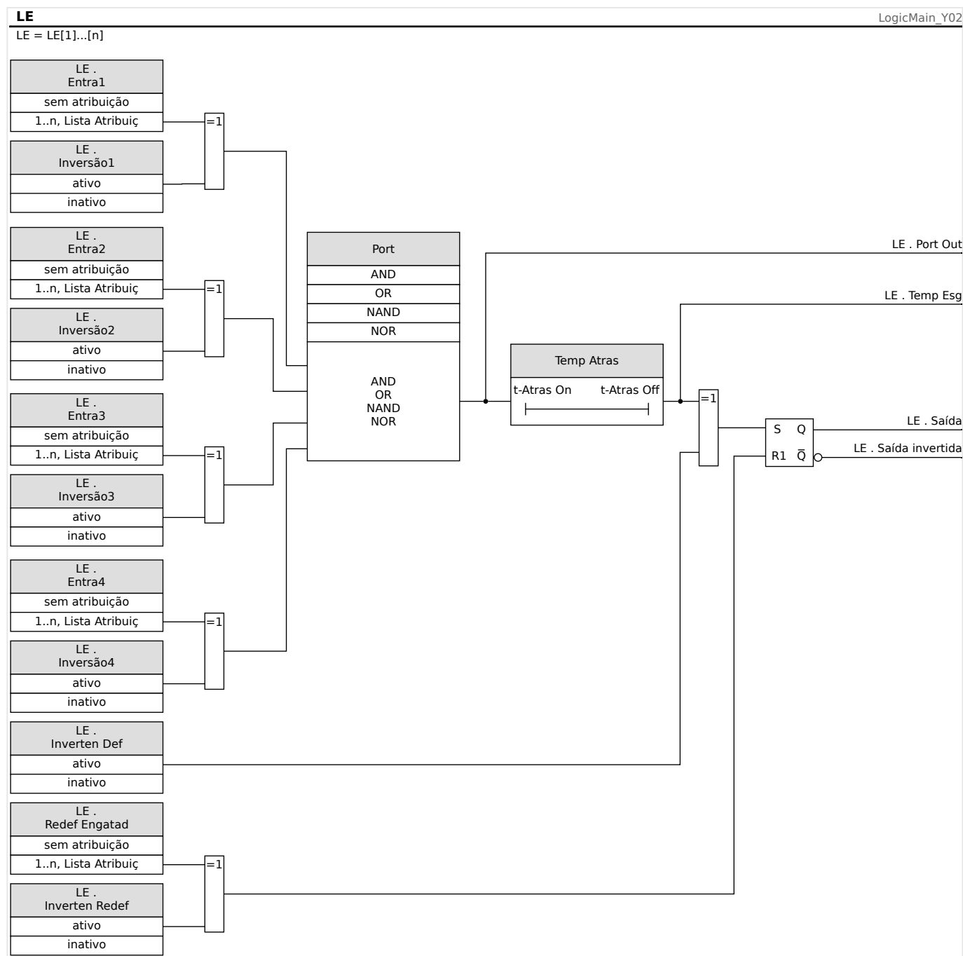
Fig. 134: Visão Geral Detalhada - Diagrama Lógico Geral.
