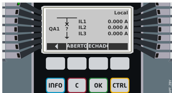
Fig. 123: Exemplo de página de controle, com o "Disjuntor" na posição de falha (ou implausível).
