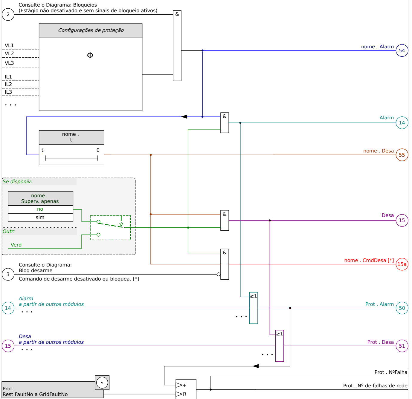
Fig. 63: Esboço rápido da funcionalidade de qualquer HighPROTEC elemento de proteção.
