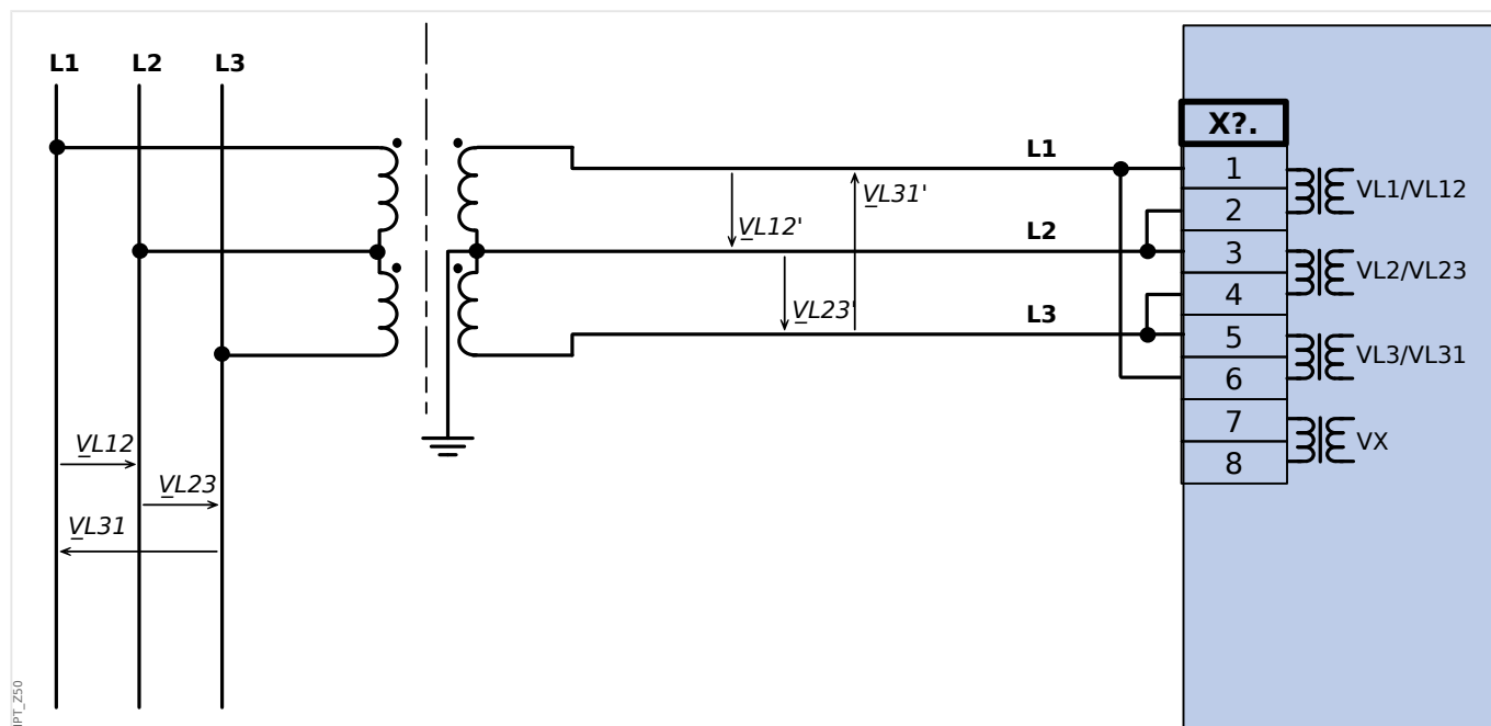
Fig. 38: Medição de tensão bifásica - fiação das entradas de medição: "Delta Aber"
