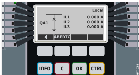
Fig. 122: Exemplo de página de controle, com o "Disjuntor" na posição fechada.
