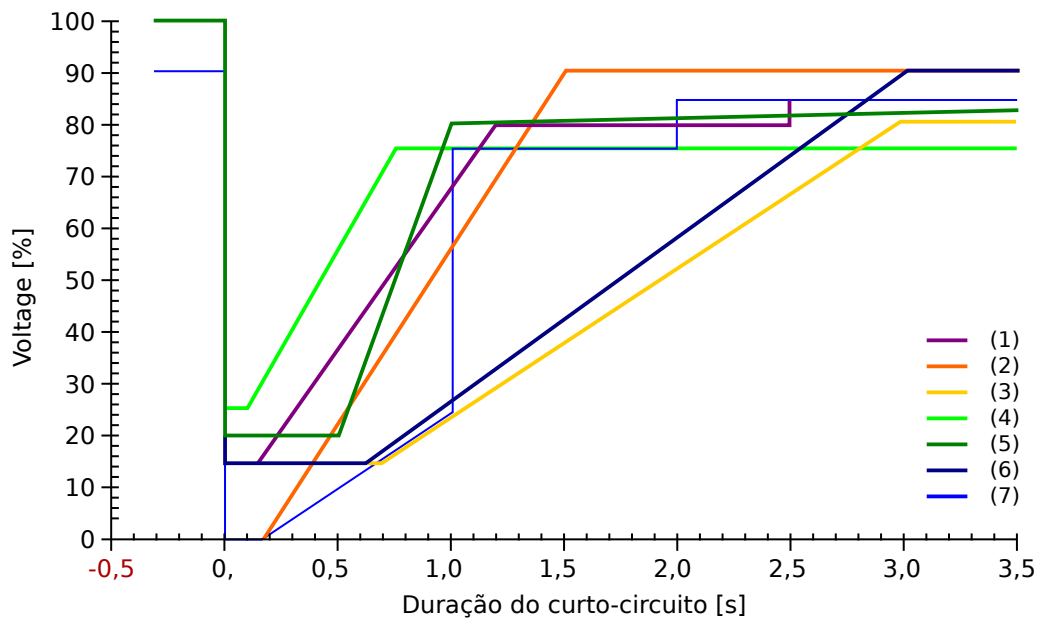
Fig. 111: Padrões LVRT; fonte: eBWK Bd. 60 (2008) Nr. 4. Autores: Dipl.-Ing. Thomas Smolka, Dr.-Ing. Karl-Heinz Weck, Zertifizierungstelle der FGH e.V., Mannheim, sowie Dipl.-Ing. (FH) Matthias Bartsch, Enercon GmbH, Aurich.
