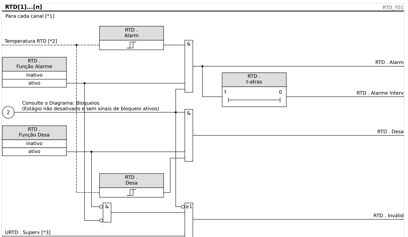
Fig. 117: O princípio geral de funcionamento (alarme atrasado, disparo sem atraso).
