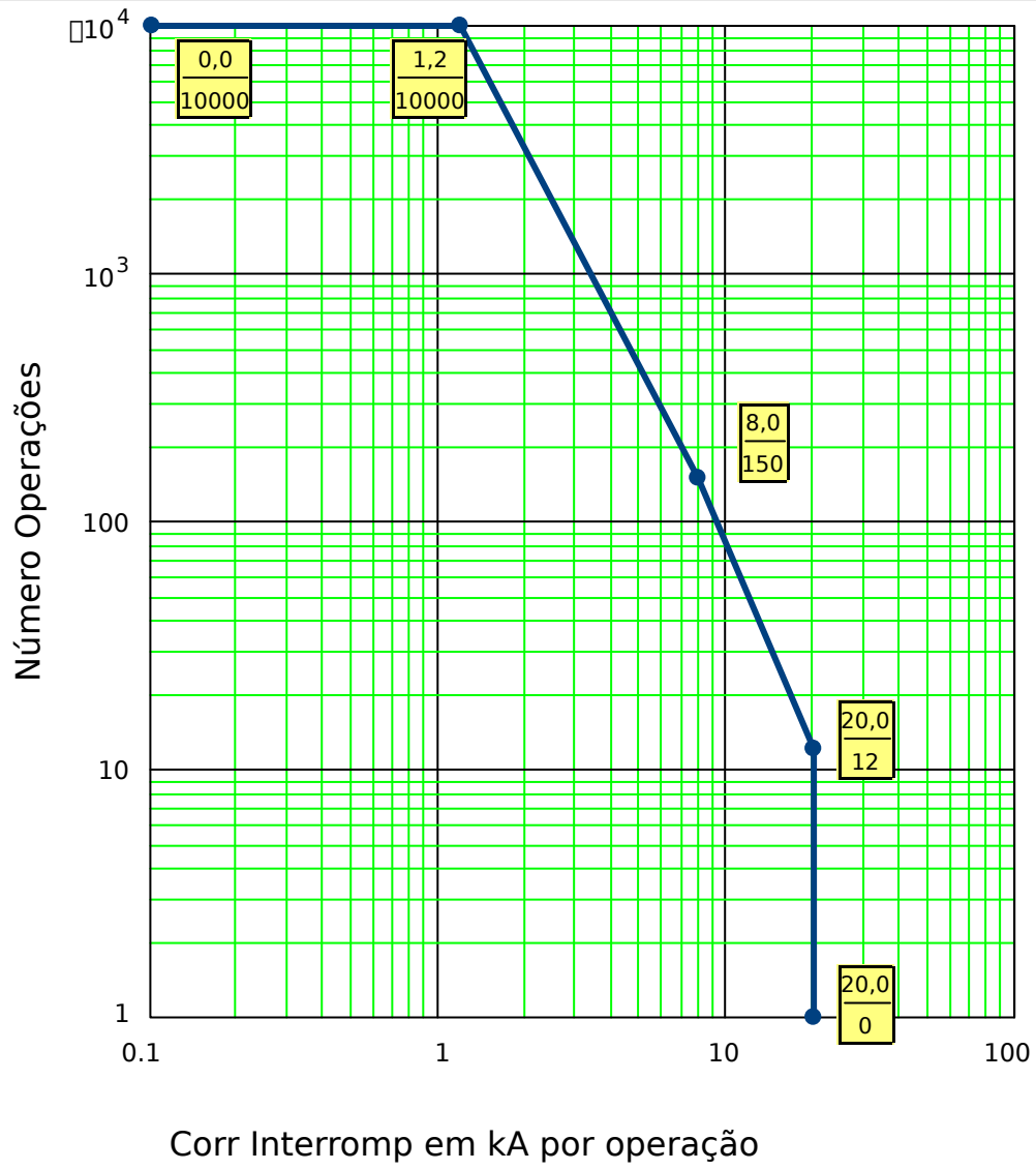
Fig. 127: Curva Manutenção de Disjuntor para Disjuntor normal 25kV
