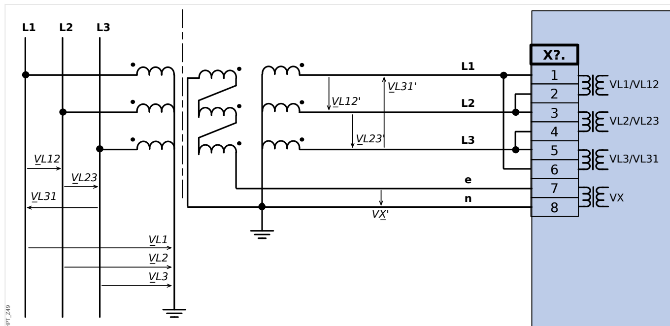
Fig. 37: Medição VG tensão residual por meio de "delta aberto" (e-n) de circuito auxiliar
