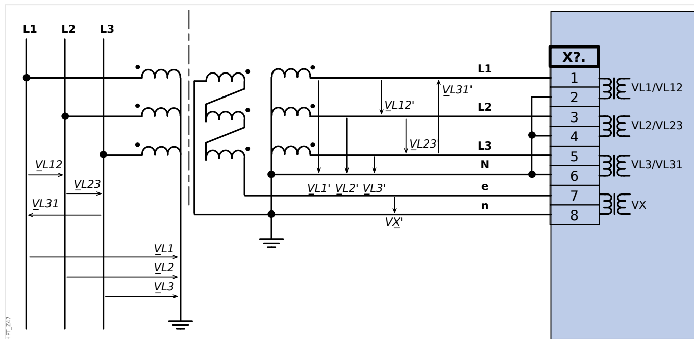
Fig. 35: VT Wye com conexão Broken Delta.
