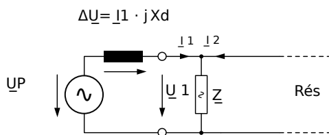
Fig. 90: Circuit équivalent au niveau du générateur synchrone en parallèle avec le réseau.
