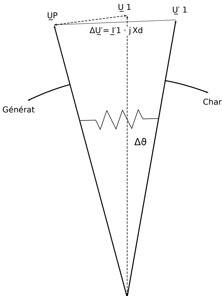
Fig. 93: Vecteurs de tension en cas de coupure de réseau.
