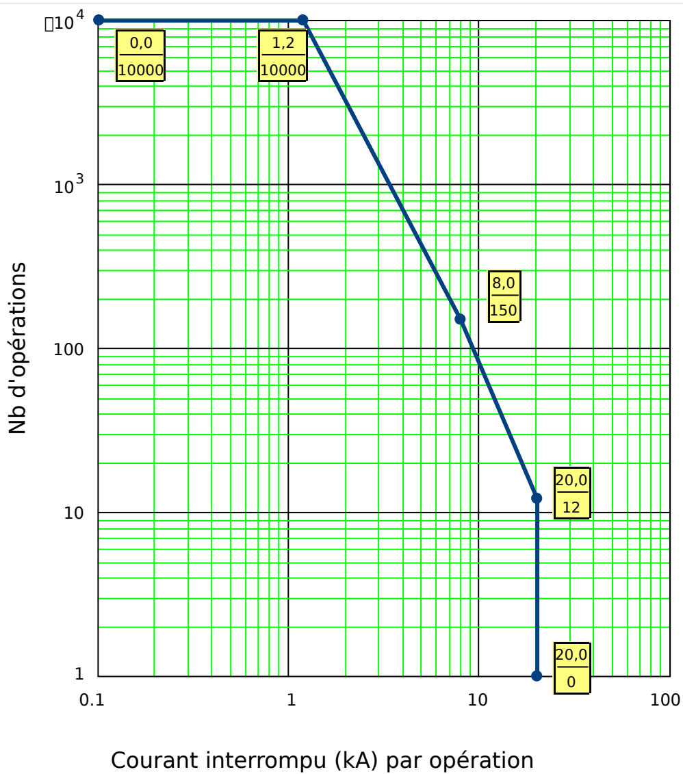
Fig. 127: Courbe de maintenance du disj pour un disj 25 ~kV typique
