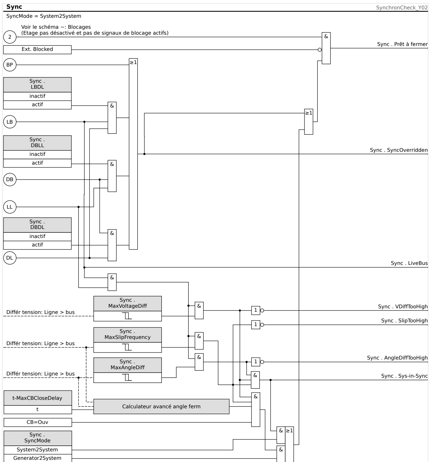
Fig. 99: Fonctionnalité du module «Sync», « System2System ».
