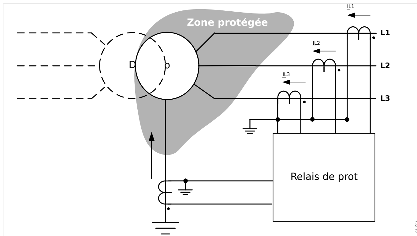
Fig. 77: Principe de protection différentielle du courant à la terre connecté à la partie en étoile de l'enroulement d'un transformateur
