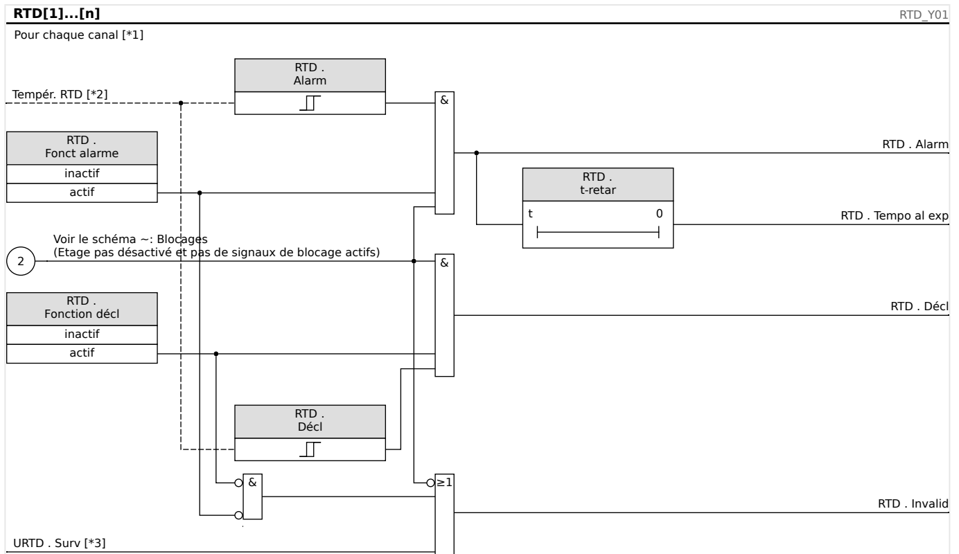
Fig. 117: Principe de fonctionnement général (alarme retardée, déclenchement non retardé).
