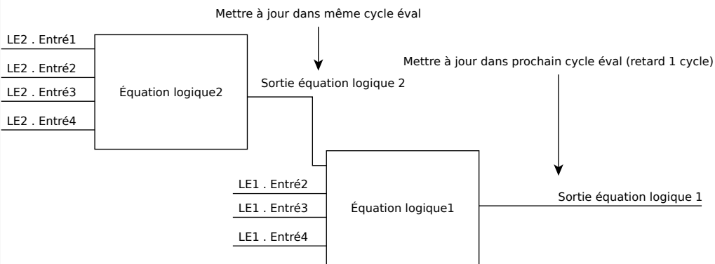
Fig. 138: En cascade ordre décroissant
