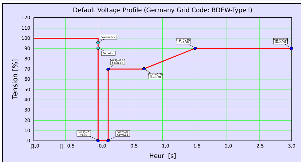
Fig. 114: Profil LVRT prédéfini en usine (BDEW-Type I).
