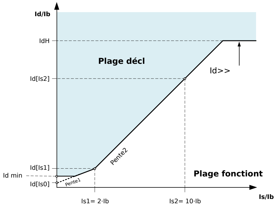
Fig. 76: Valeur IdH d'étape de niveau supérieur et non limitée de protection différentielle
