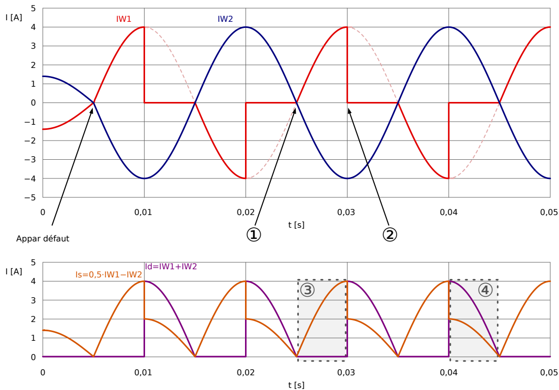
Fig. 75: Caractéristique de I_d et I_s avec saturation côté CT W1 pour un défaut externe.
