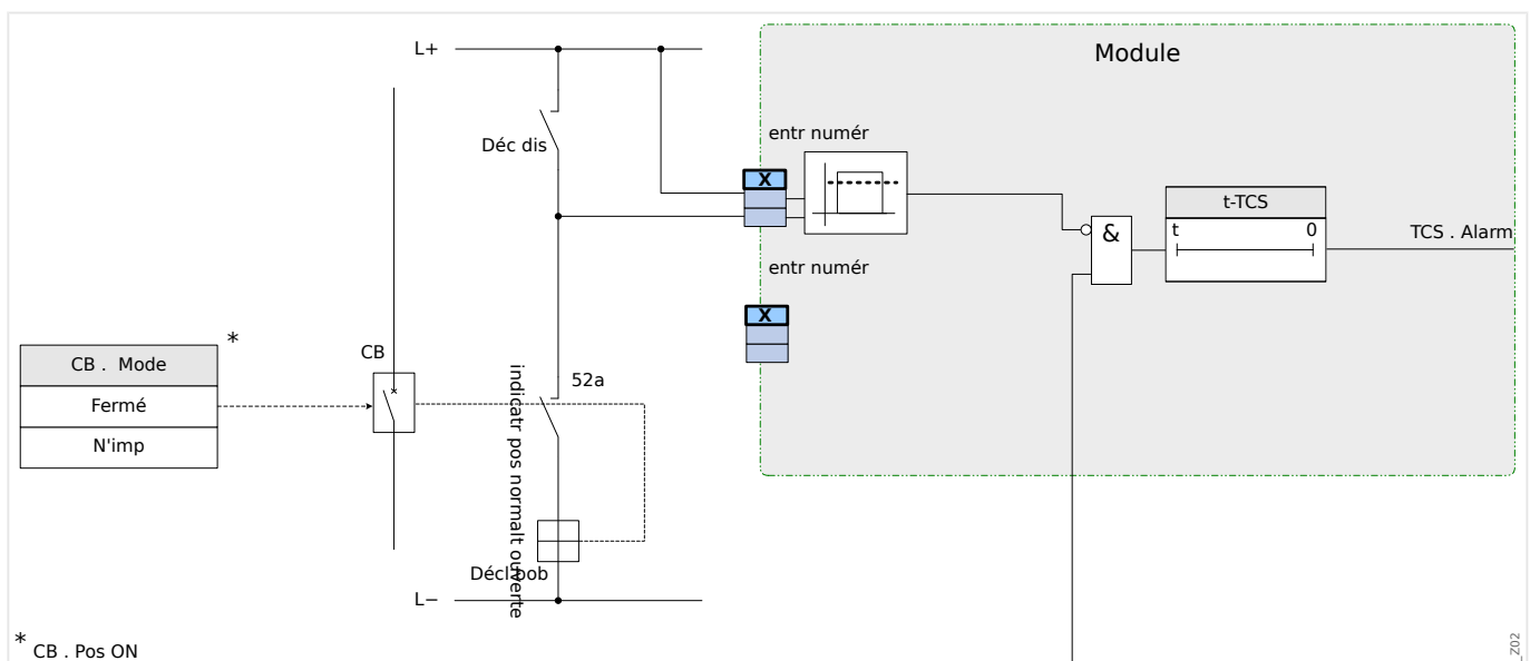
Fig. 119: Exemple de connexion : Surveillance du circuit de déclenchement avec un contact auxiliaire de disjoncteur «Aux ON» (52a).
