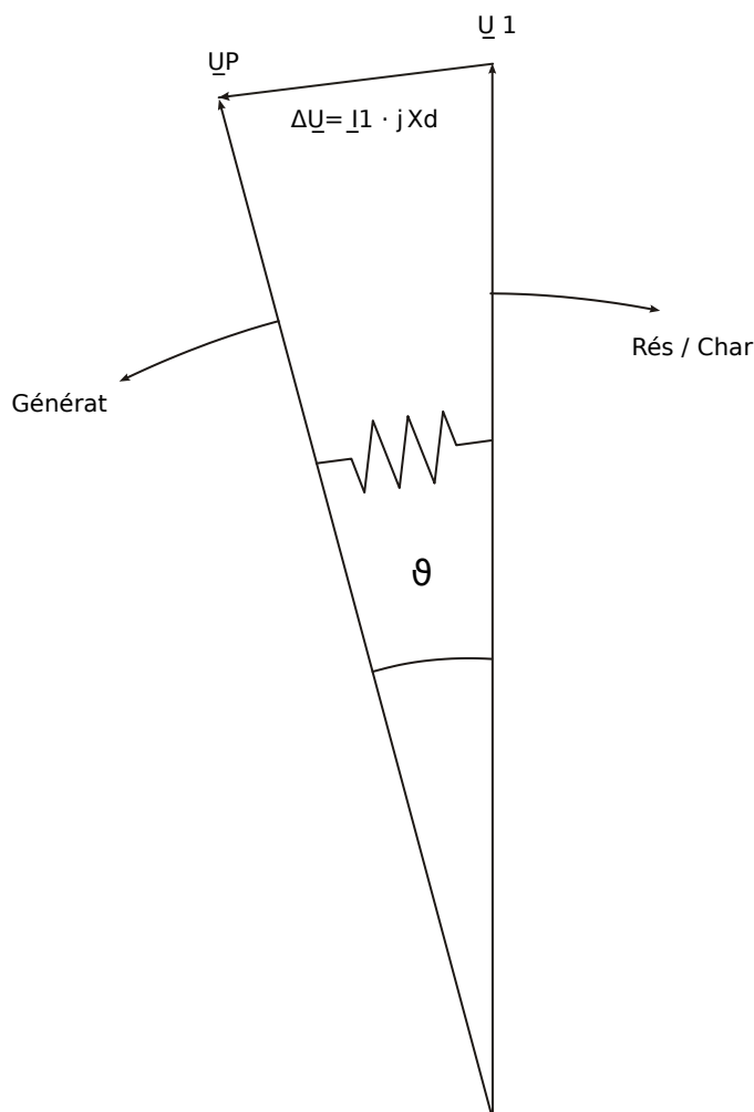
Fig. 91: Vecteurs de tension en fonctionnement parallèle du réseau.
