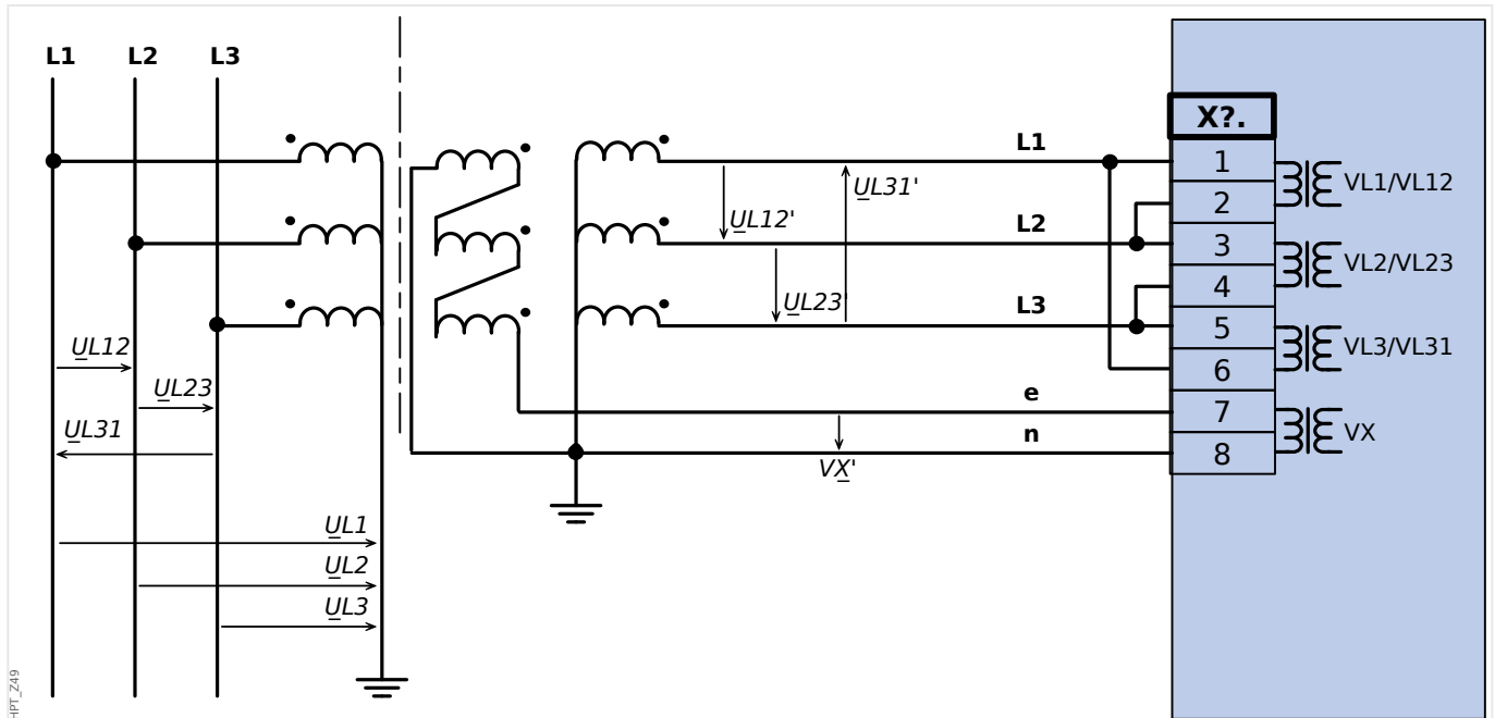
Fig. 37: Mesure de tension triphasée - câblage des entrées de mesure : "delta-connection" (Connexion en triangle). Mesure tension résid VG via enroults auxiliaires (e-n) "triangle fermé"
