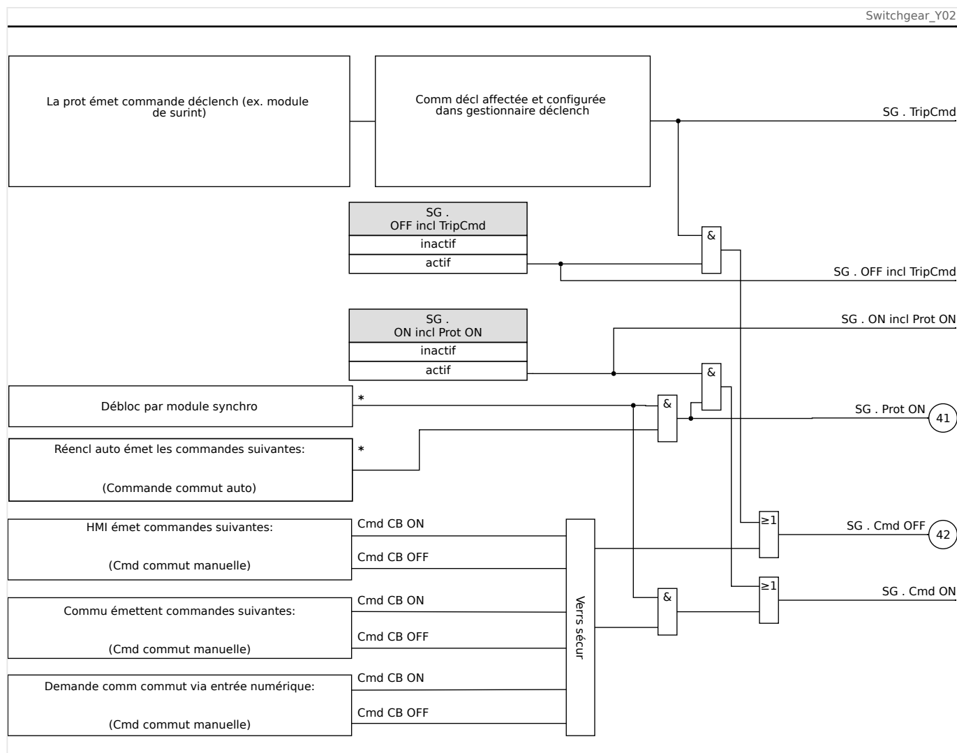
Fig. 125: Verrouillages (Parties identifiées par « * » : la disponibilité dépend du type de dispositif commandé.)
