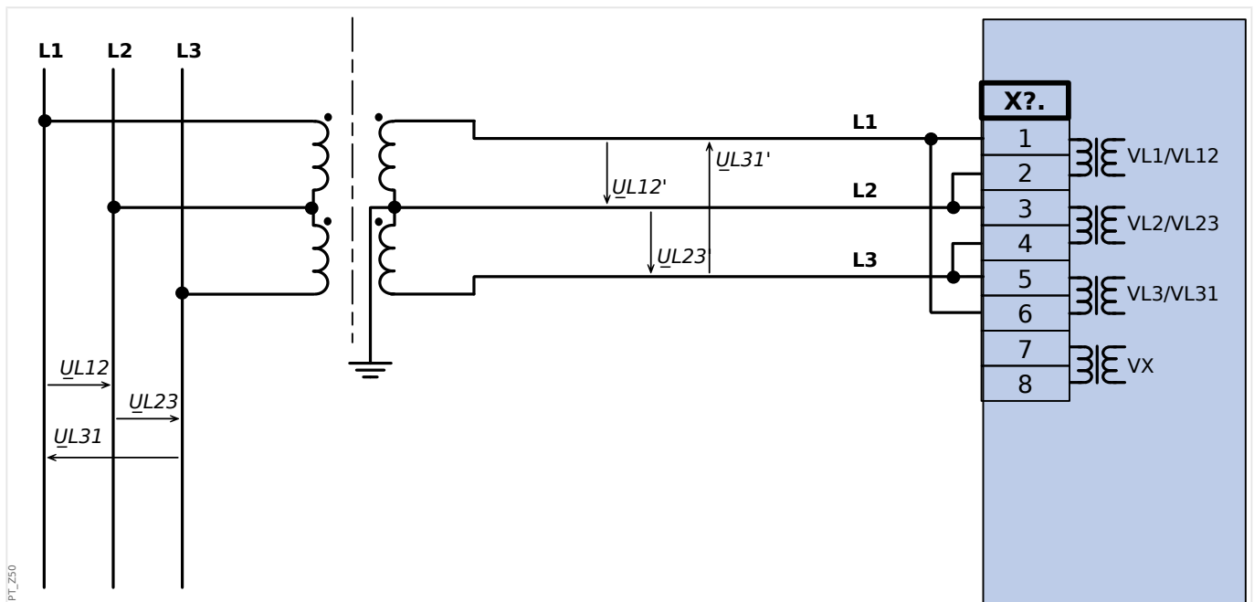
Fig. 38: Mesure de tension biphasée - câblage des entrées de mesure: "Triangle ouvert"
