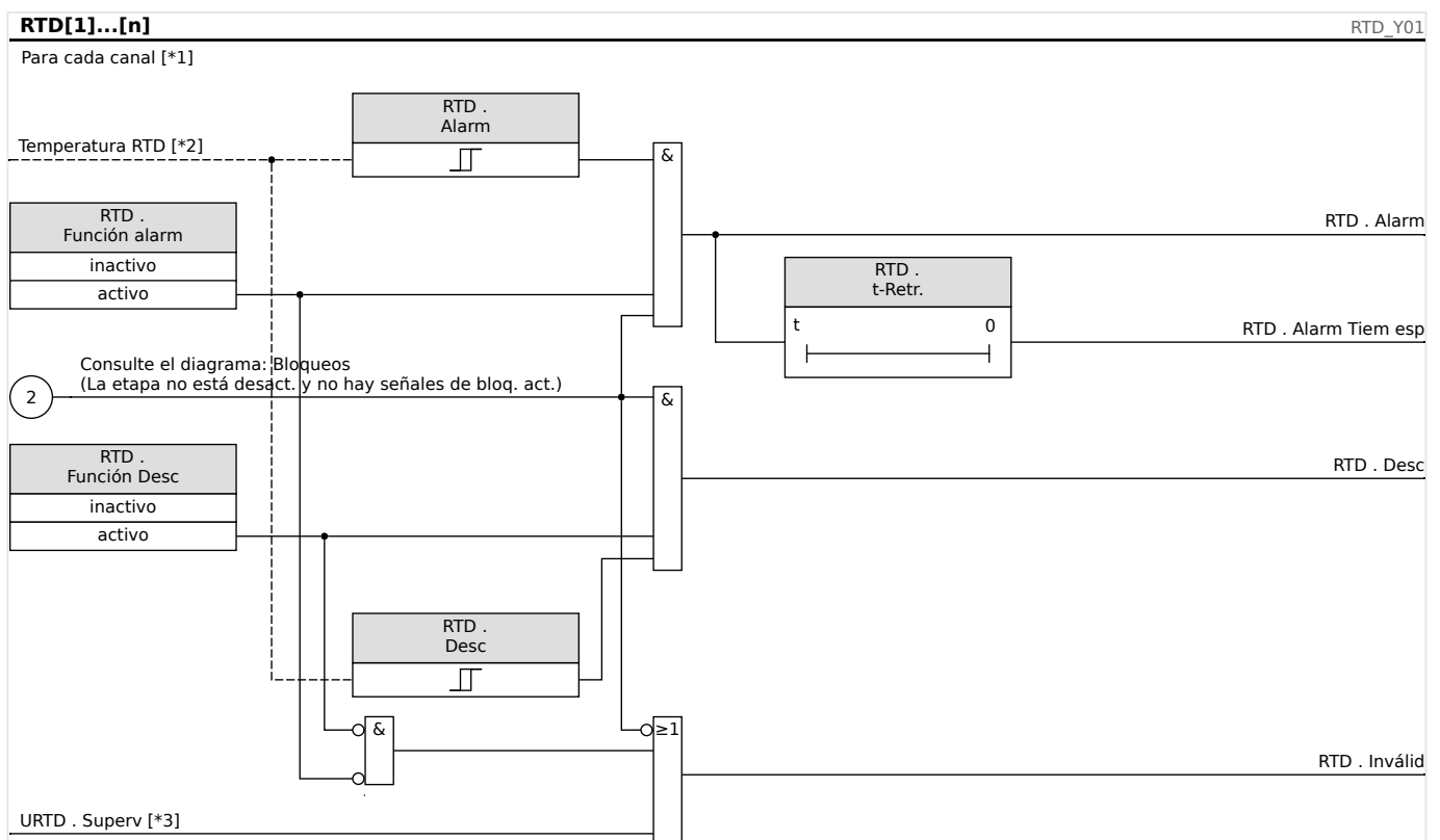
Fig. 117: El principio de funcionamiento general (alarma retrasada, desconexión sin retraso).
