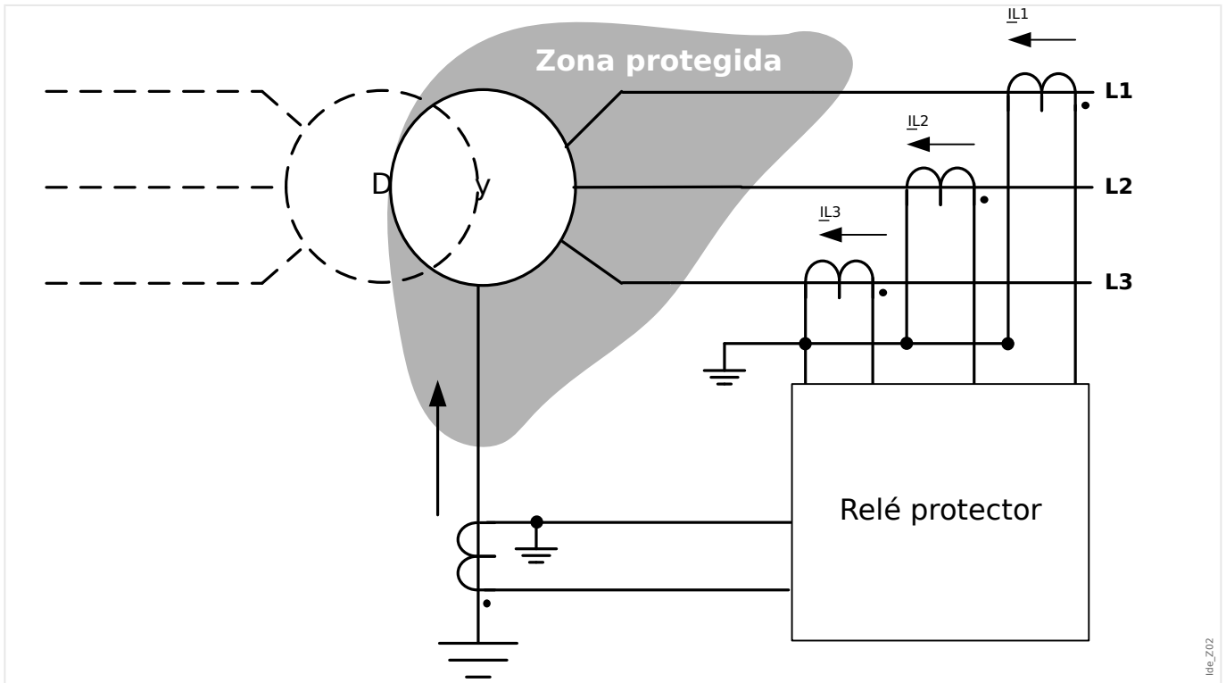
Fig. 77: Principio de protección de la protección de diferencial de corriente de tierra conectada al bobinado del lado wye del transformador
