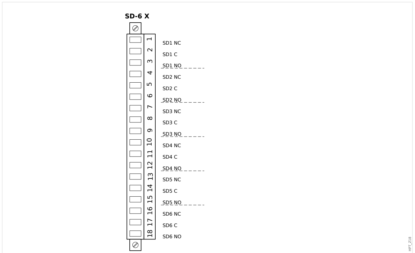
Fig. 13: Asignación electromecánica
