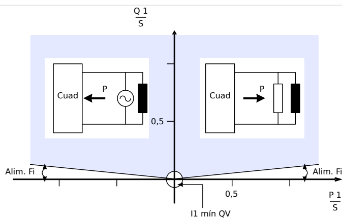
Fig. 101: Método 1: Supervisión de ángulo de potencia
