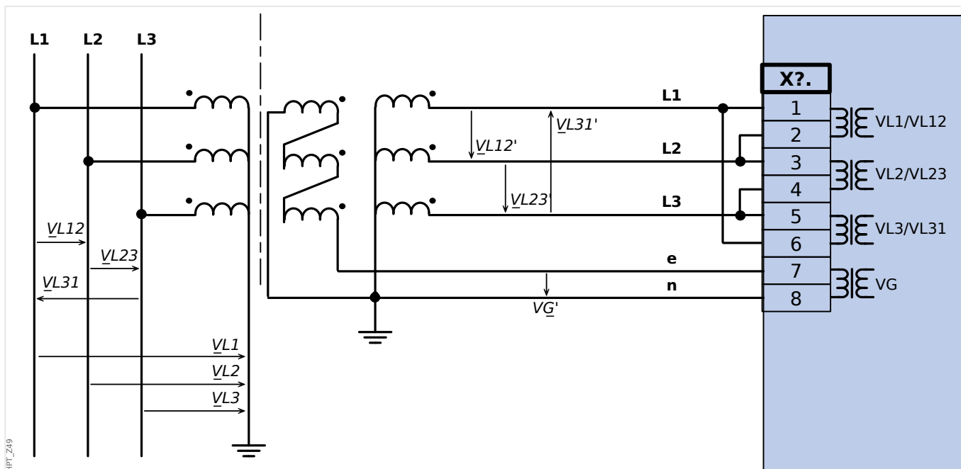
Fig. 37: Medida de tensión trifásica (cableado de las entradas de medición: "conexión delta") Medida del VG de voltaje residual a través de bobinas auxiliares (e-n) "delta roto"
