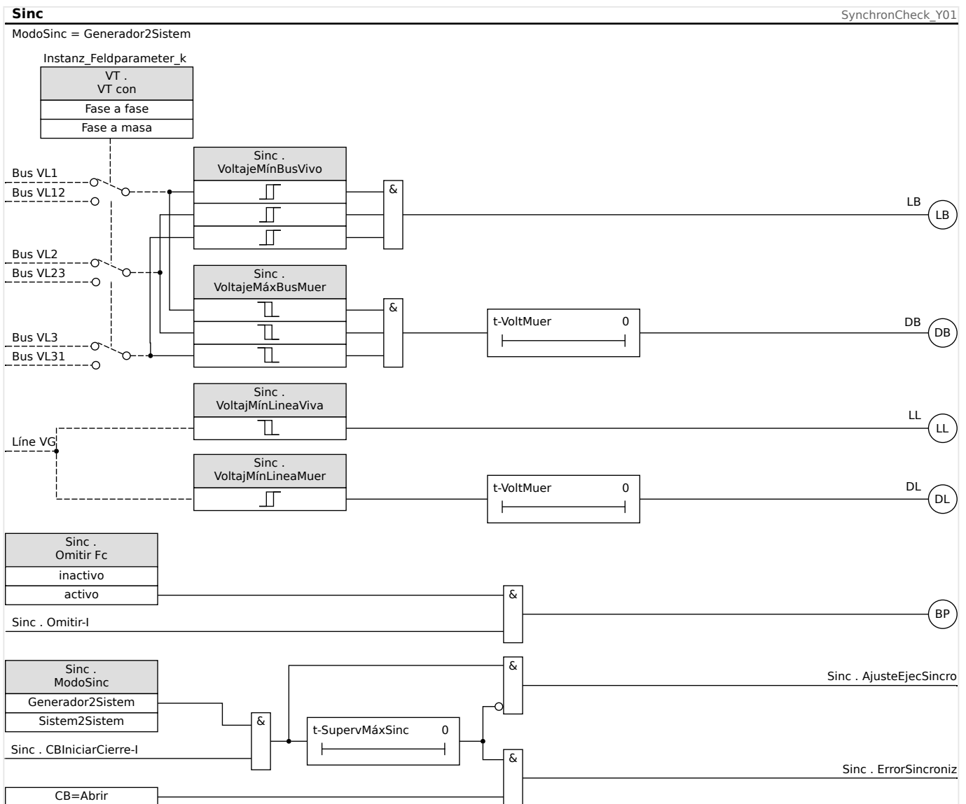
Fig. 98: Funcionalidad del módulo »Sinc«, «Generador2Sistem».
