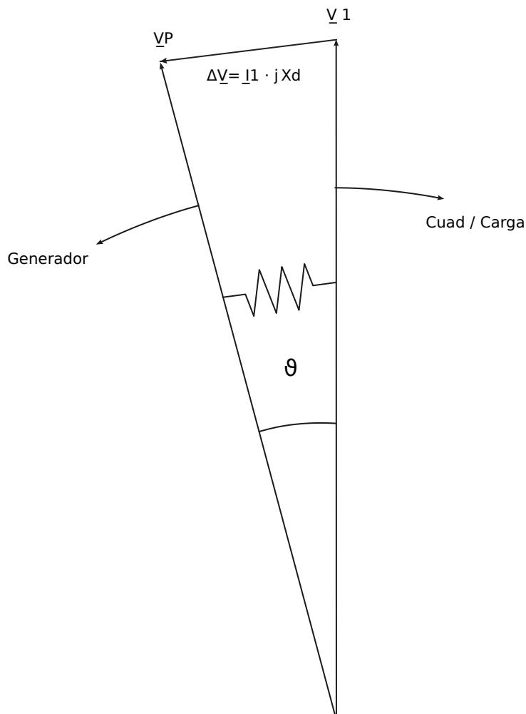
Fig. 91: Vectores de tensión en funcionamiento en paralelo con la red de suministro eléctrico.
