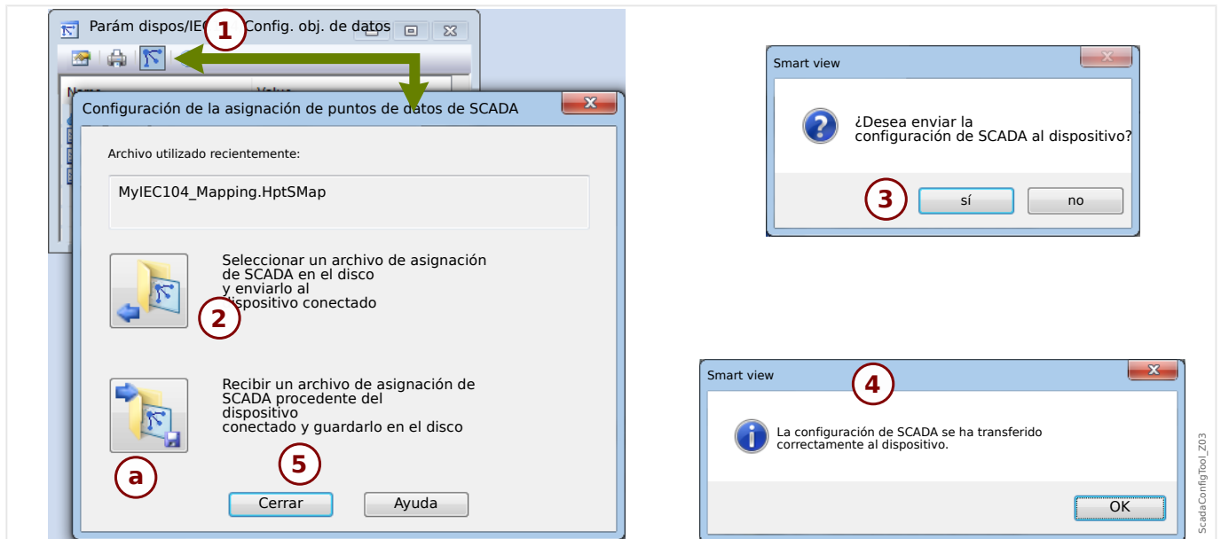
Fig. 61: Ejemplo de uso de Smart view para transferir el archivo *.HptSMap al dispositivo de protección.
