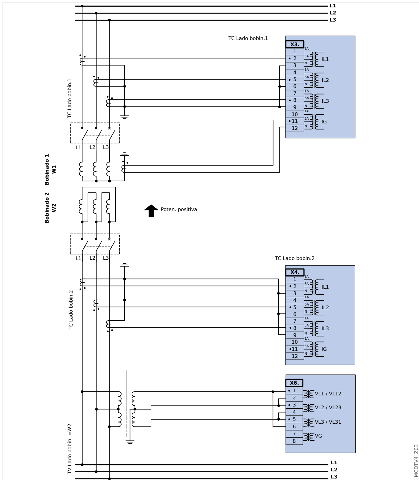
Fig. 40: Transformador DY con protección diferencial de fase, REF en W1 y VT en W2 (conexión V)
