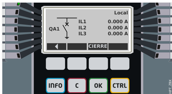
Fig. 124: Ejemplo de página de control, con el circuito en posición abierta.
