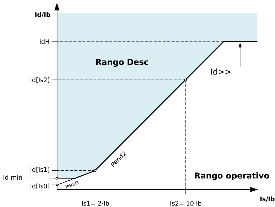
Fig. 76: Paso de protección de diferencial de ajuste alto no limitado I_{dH} .
