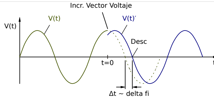
Fig. 94: Incremento vectorial de tensión.
