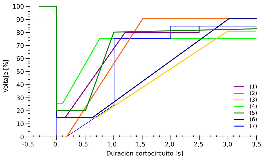
Fig. 111: Estándares de LVRT; fuente: eBWK Bd. 60 (2008) N.º 4. Autores: Dipl.-Ing. Thomas Smolka, Dr.-Ing. Karl-Heinz Weck, Zertifizierungstelle der FGH e.V., Mannheim, sowie Dipl.-Ing. (FH) Matthias Bartsch, Enercon GmbH, Aurich.
