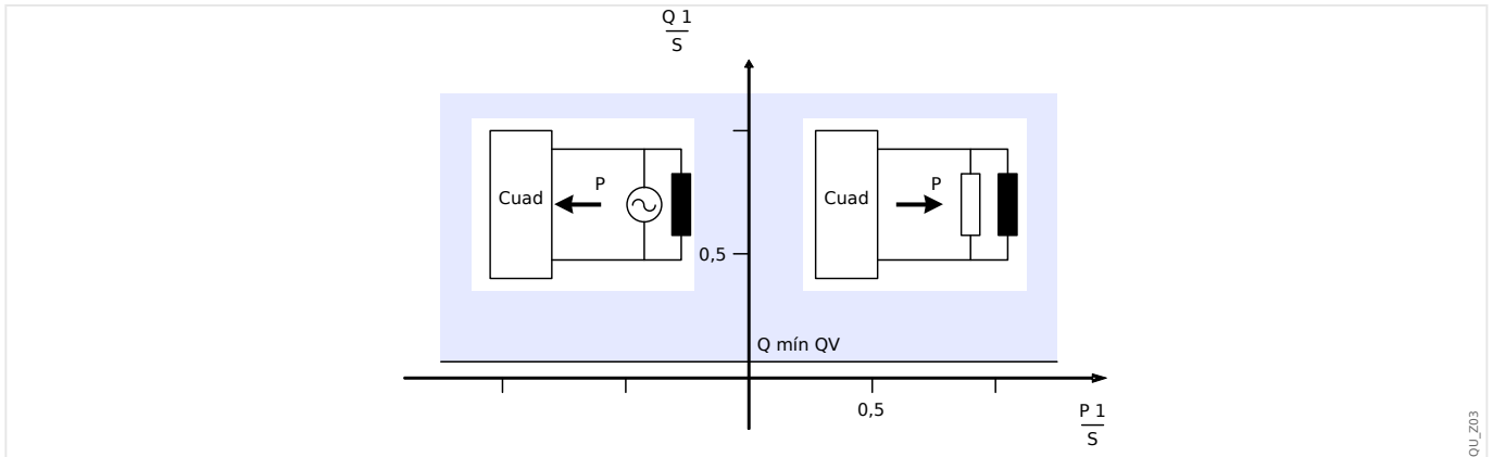
Fig. 102: Método 2: Supervisión de potencia reactiva pura.
