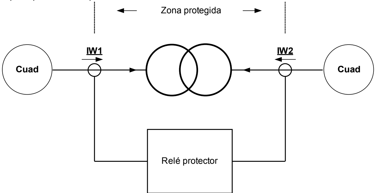
Principio de protección de la protección diferencial de corriente
