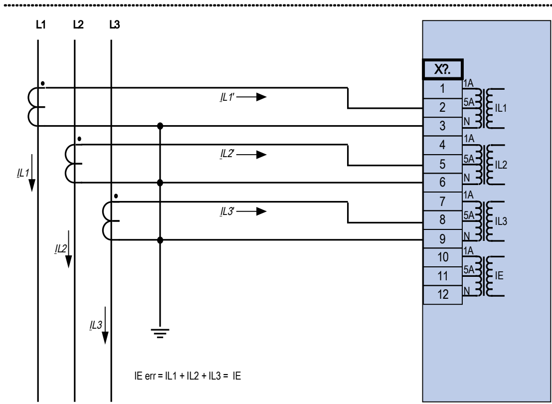
Dreiphasiger Stromwandleranschluss; In sekundär = 5 A.
