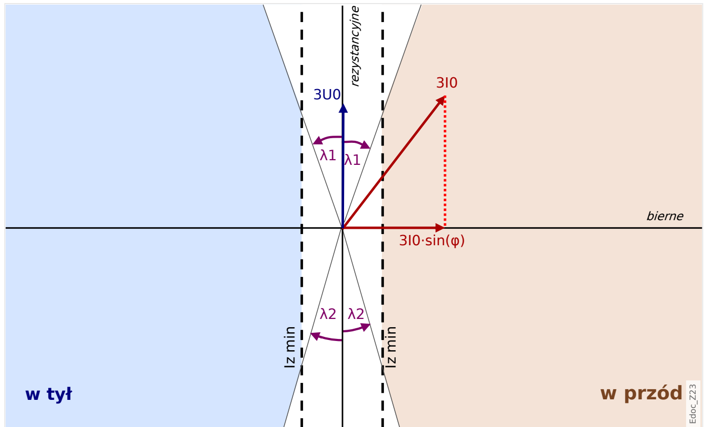
Rys. 70: Zasada określania kierunku metodą „ \sin(\phi) ”.
