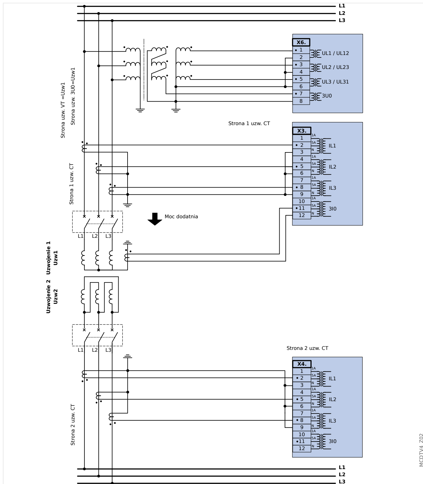
Rys. 39: Transformator DY z zabezpieczeniem różnicowoprądowym fazowym i ziemnozwarciowym tylko w W1.
