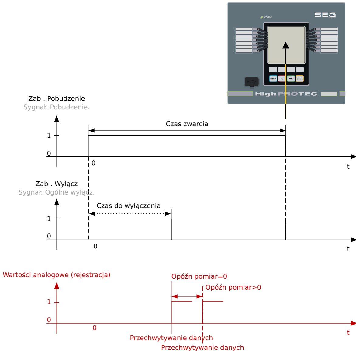
Rys. 142: Rejestrator zwarć: czasy (trwania).
