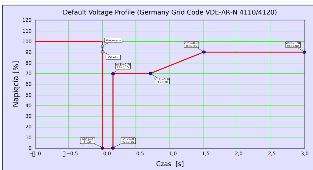
Rys. 124: Profil domyślny LVRT (typ I).
