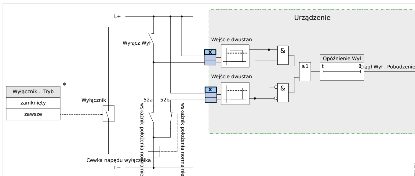
Rys. 128: Przykład okablowania: Układ kontroli ciągłości obwodów wyłącznika z dwoma stykami pomocniczymi wyłącznika „Położ ZAŁ” (52a) i „Położ WYŁ” (52b).
