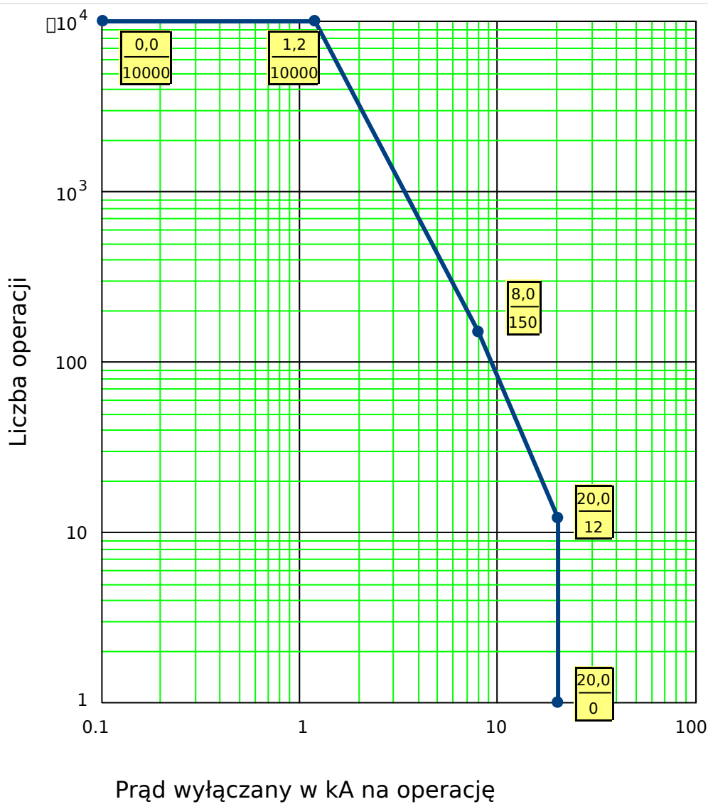
Rys. 137: Krzywa konserwacji wyłącznika typowego wyłącznika 25 kV
