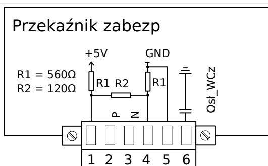
Rys. 47: Przypisanie elektromechaniczne
