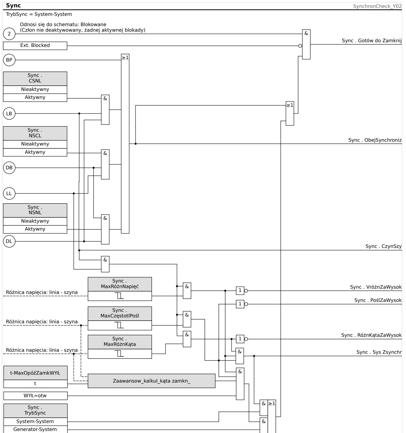
Rys. 109: Działanie modułu „Sync”, „System-System”.
