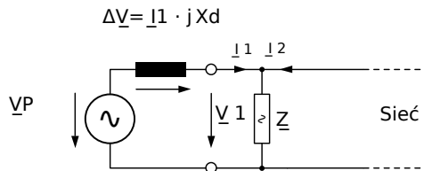
Rys. 100: Schemat zastępczy dla prądnicy synchronicznej pracującej równolegle z siecią.
