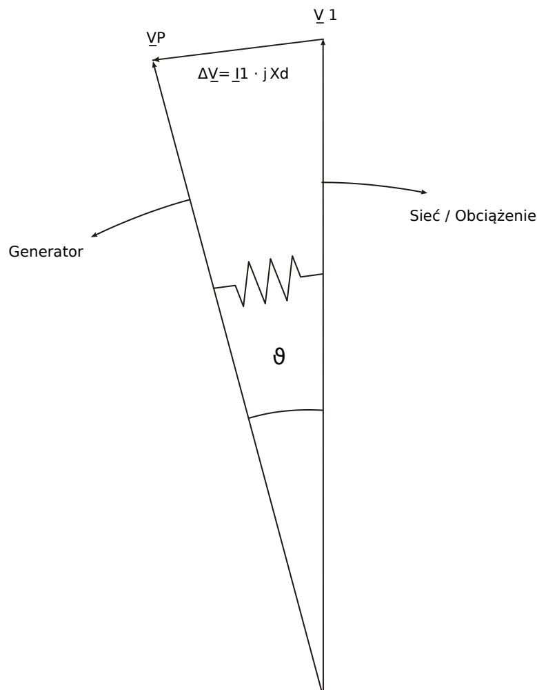
Rys. 101: Wektory napięcia przy pracy równoległej z siecią.
