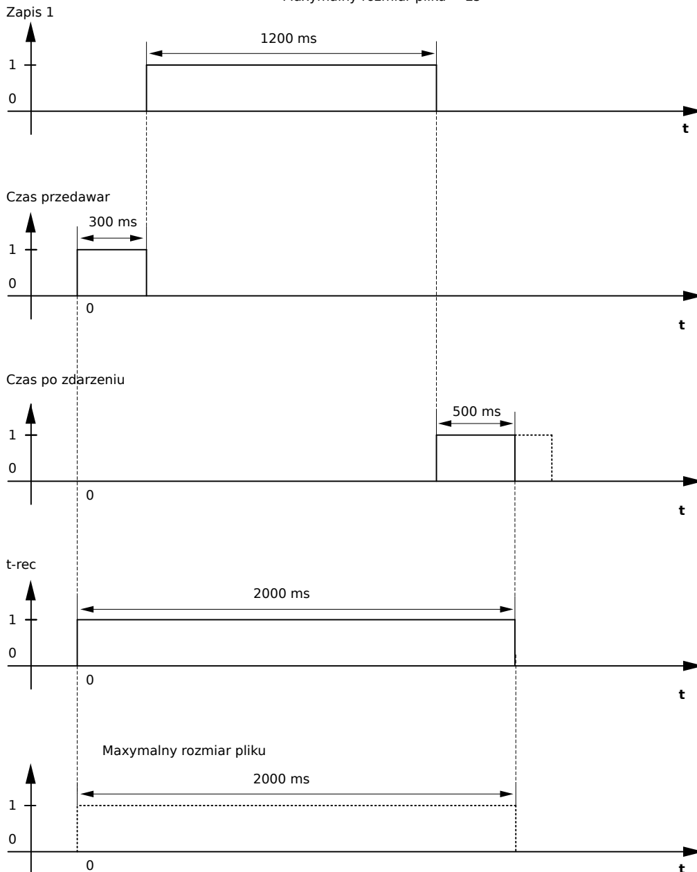
Rys. 140: Przykładowy wykres czasów pracy rejestratora zakłóceń I
