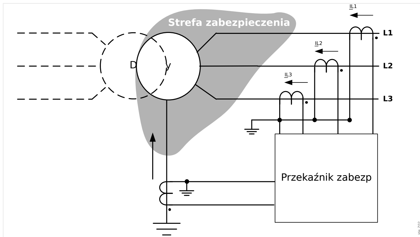
Rys. 79: Zasada działania zabezpieczenia różnicowego ziemnozwarciowego w uzwojeniach transformatorów połączonych w gwiazdę.
