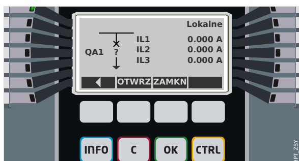
Rys. 133: Przykład strony sterowania z wyłącznikiem w pozycji zakłóconej (lub nieprawidłowej).
