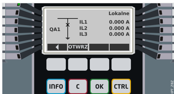
Rys. 132: Przykład strony sterowania z wyłącznikiem w pozycji zamkniętej.
