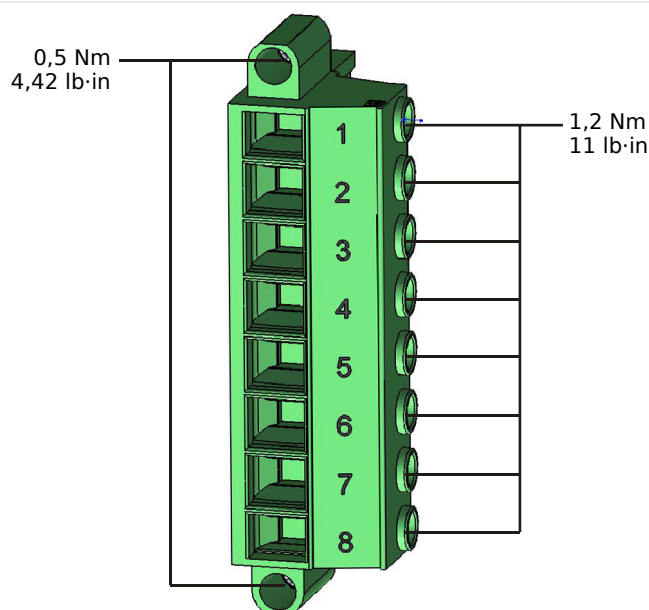
Rys. 151: Zaciski pomiaru napięcia karty pomiarowej „TU” (→ „2.8.1 TU – wejścia do pomiaru napięcia”).
