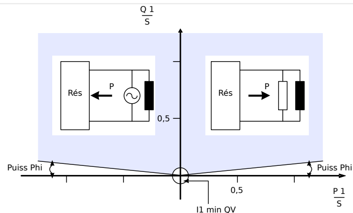
Fig. 111: Méthode 1 : Surveillance de l'angle de charge
