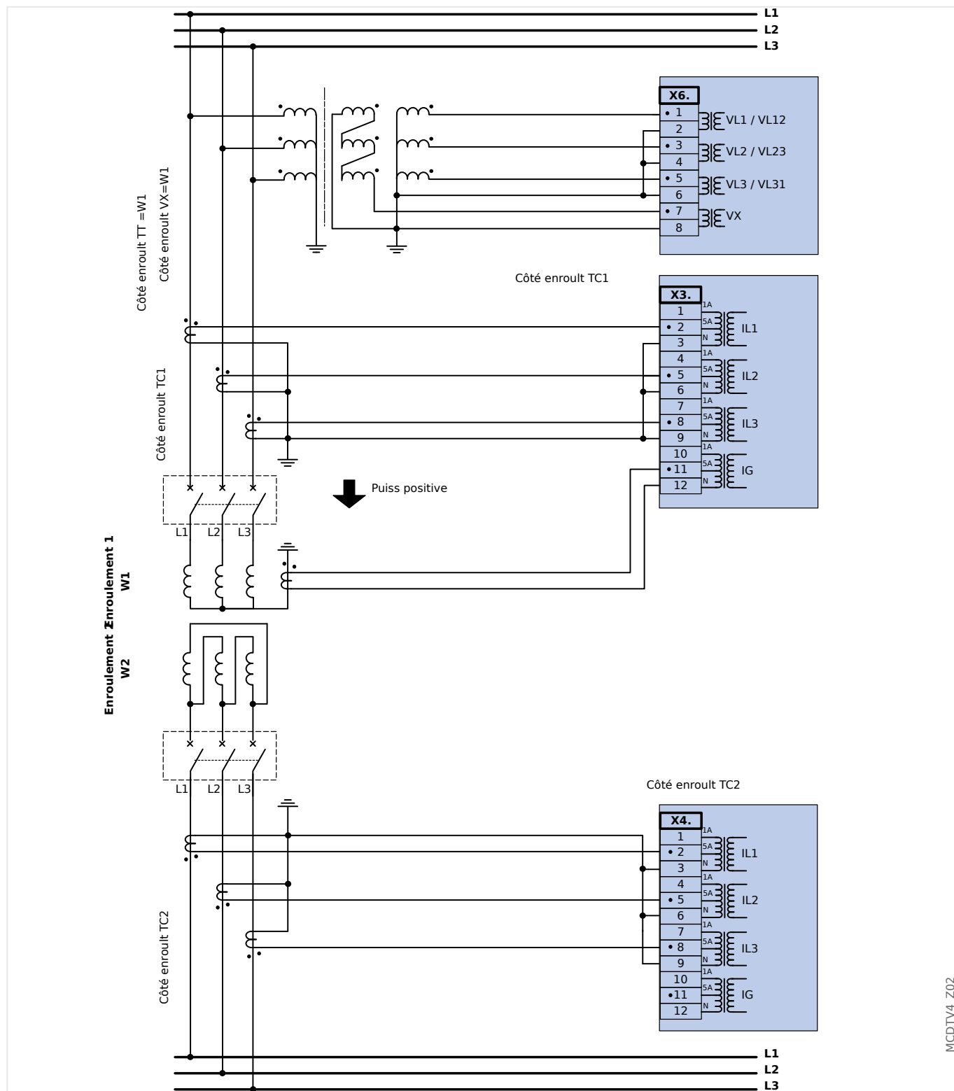
Fig. 39: Transformateur DY avec protection différentielle de phase et protection différentielle de terre sur la borne W1 uniquement.
