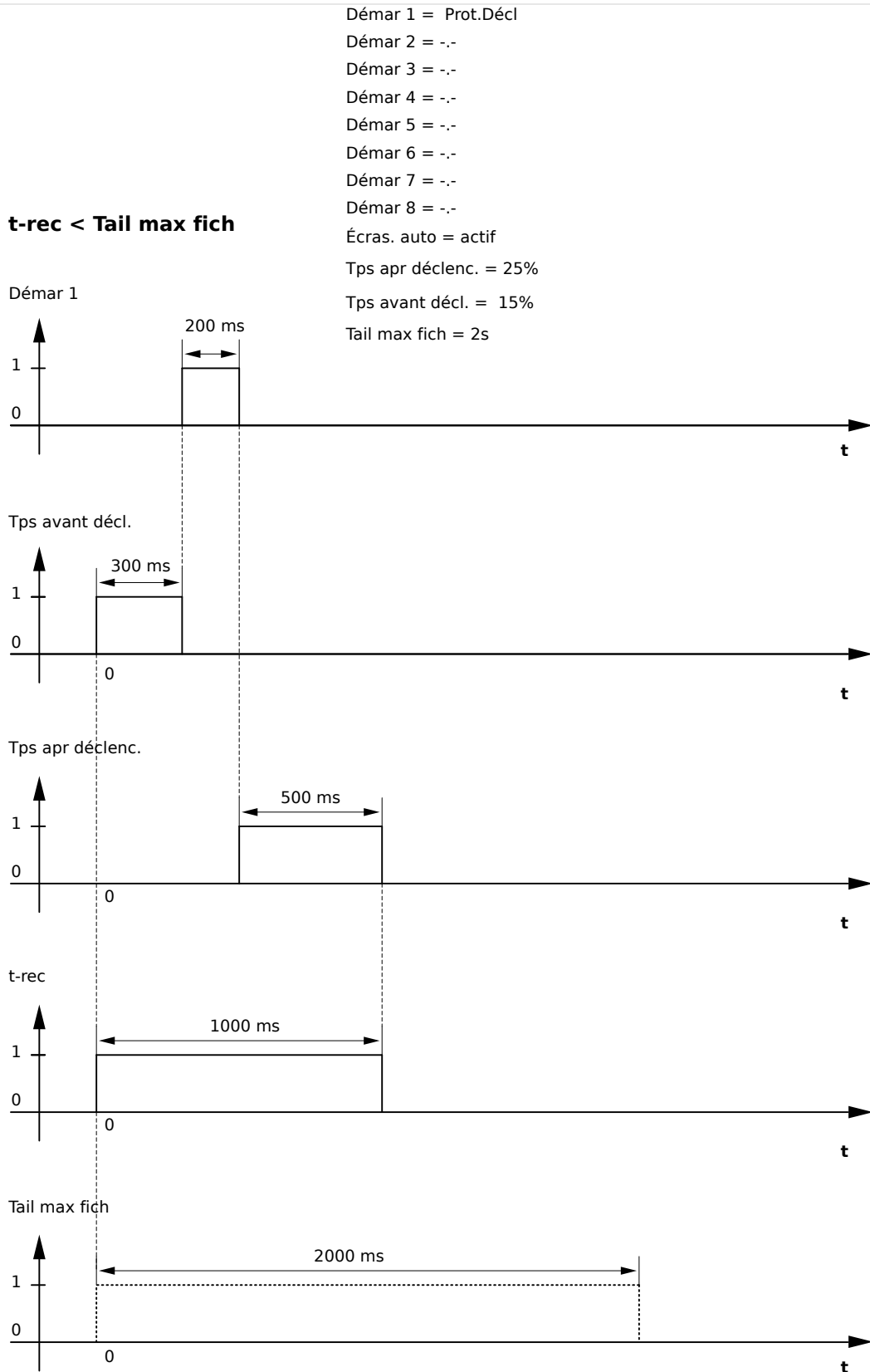
Fig. 141: Exemple de diagramme des temps de l'enregistreur de perturbations II
