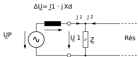
Fig. 100: Circuit équivalent au niveau du générateur synchrone en parallèle avec le réseau.
