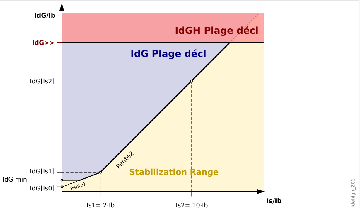
Fig. 80: Valeur d'excitation « I_dG » du courant différentiel à la terre en fonction du courant nominal « I_b » de l'objet de protection associé.
