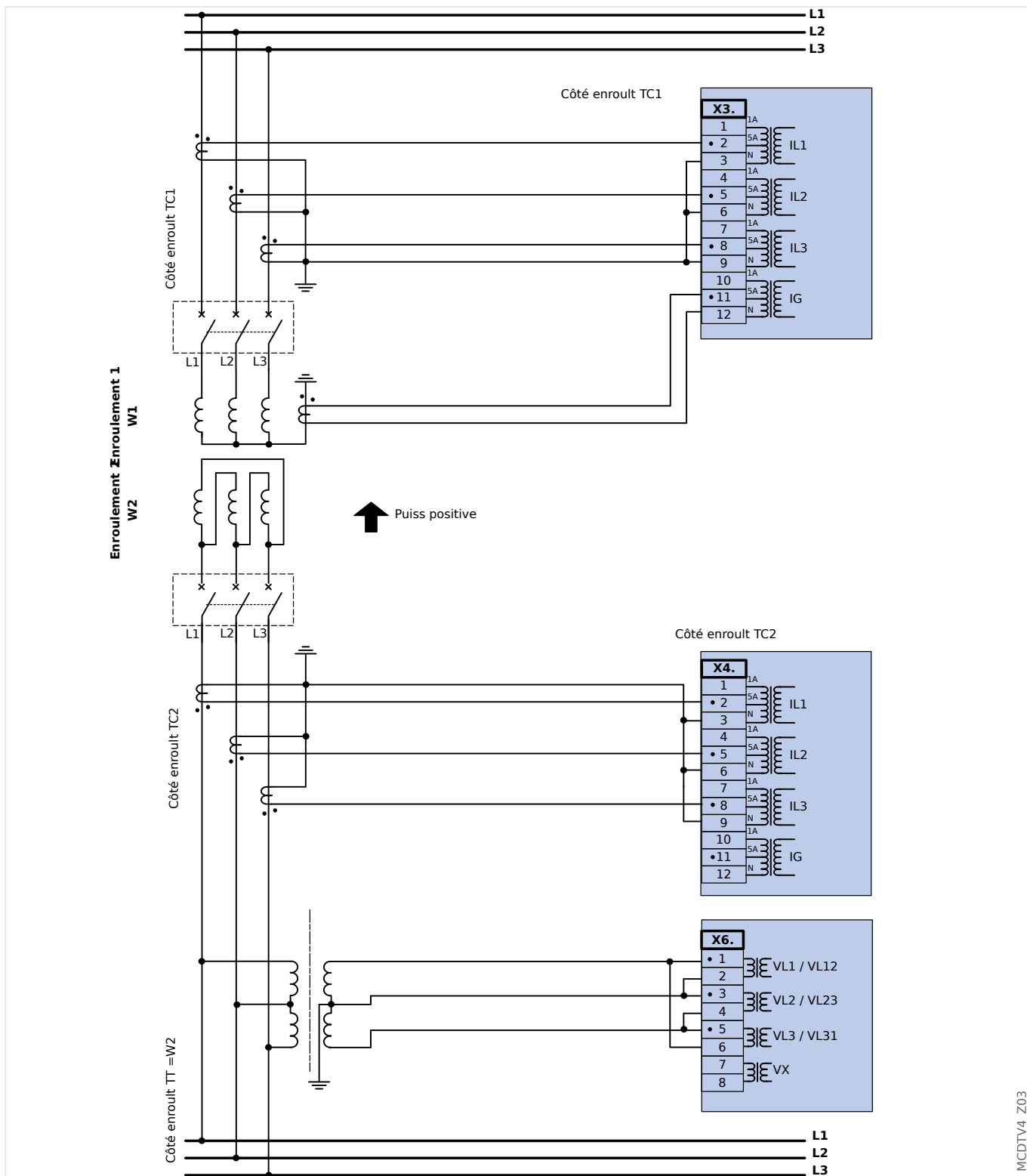
Fig. 40: Transformateur DY avec protection différentielle de phase, REF sur W1 et VT sur W2 (configuration en triangle ouvert).
