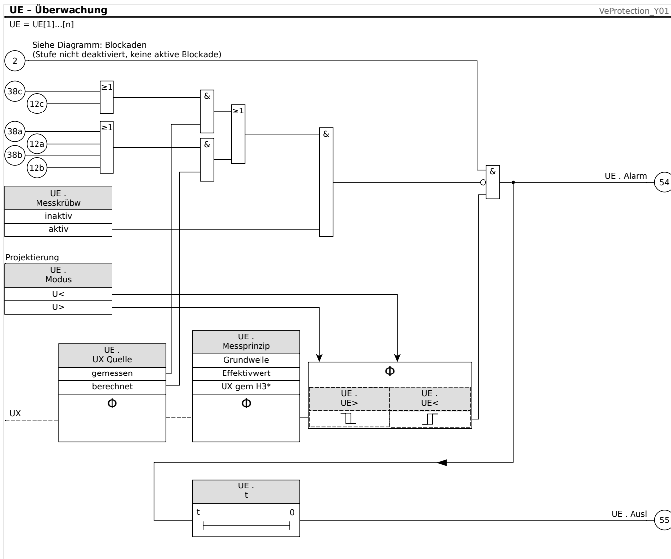
Abb. 114: UE/UX-Spannungsüberwachung, Teil 1 (Überwachungsfunktion, Auslöse-Entscheid).
