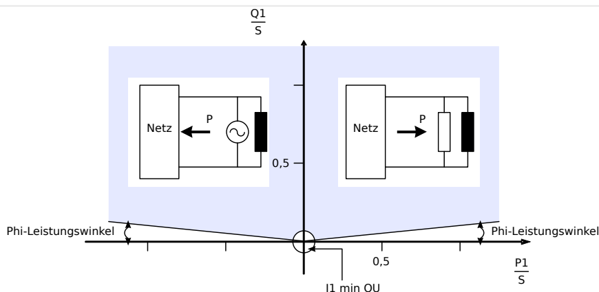
Abb. 127: Variante 1: Leistungswinkelüberwachung.
