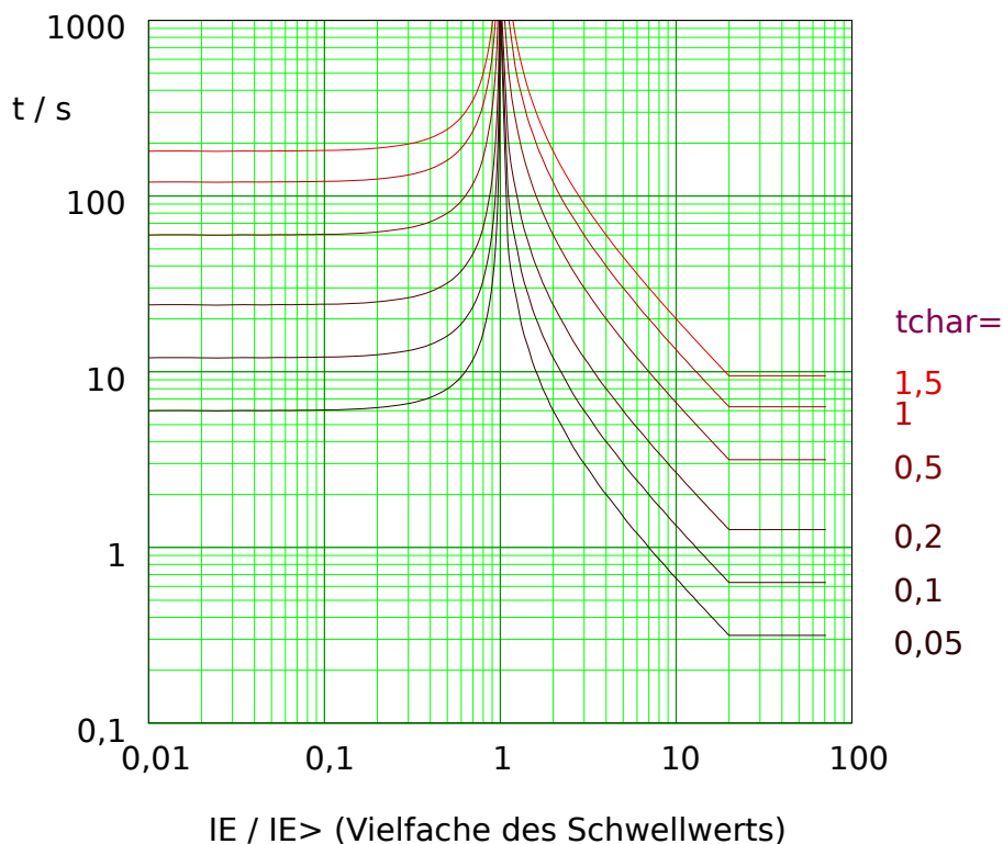
Abb. 95: LINV: Rückfallverzögerung (linke Hälfte, IE < IE_{max} ) und Auslöseverzögerung (rechte Hälfte, IE > IE_{max} ), Beispieldiagramm für IE_{max} = 20 \cdot IE_{nom} .
