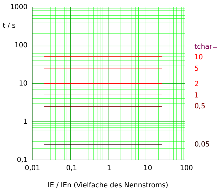
Abb. 101: Auslösekurve „Therm Flat“, wobei nur der Bereich IE > IE> jeweils anwendbar ist. Beispieldiagramm für gemessenen (nicht empfindlichen) Erdstrom.
