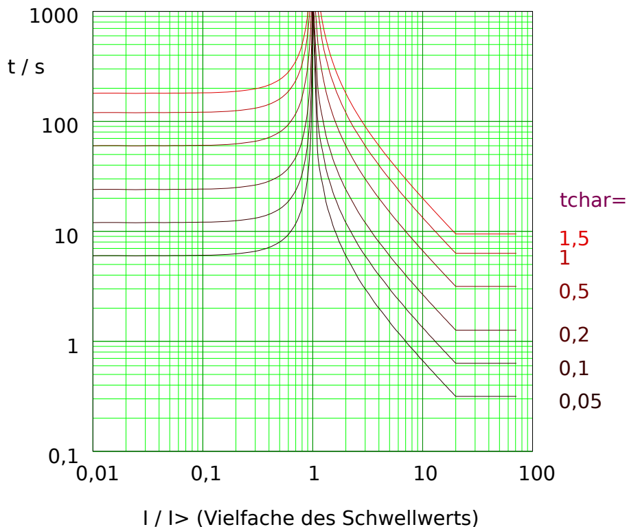
Abb. 83: LINV: Rückfallverzögerung (linke Hälfte, I < I_{max} ) und Auslöseverzögerung (rechte Hälfte, I > I_{max} ), Beispieldiagramm für I_{max} = 20 \cdot I_{nom} .
