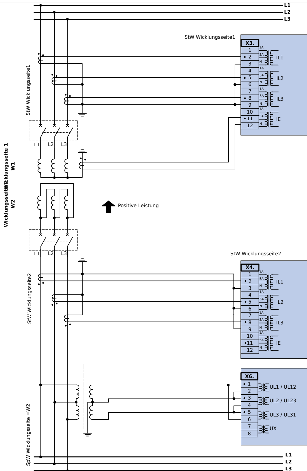
Abb. 40: DY-Transformator mit Phasendifferenzialschutz, REF auf W1 and SpW auf W2 (V-Schaltung).
