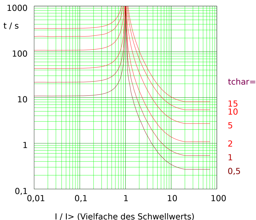
Abb. 85: VINV: Rückfallverzögerung (linke Hälfte, I < I> ) und Auslöseverzögerung (rechte Hälfte, I > I> ), Beispieldiagramm für I_{max} = 20 \cdot I> .
