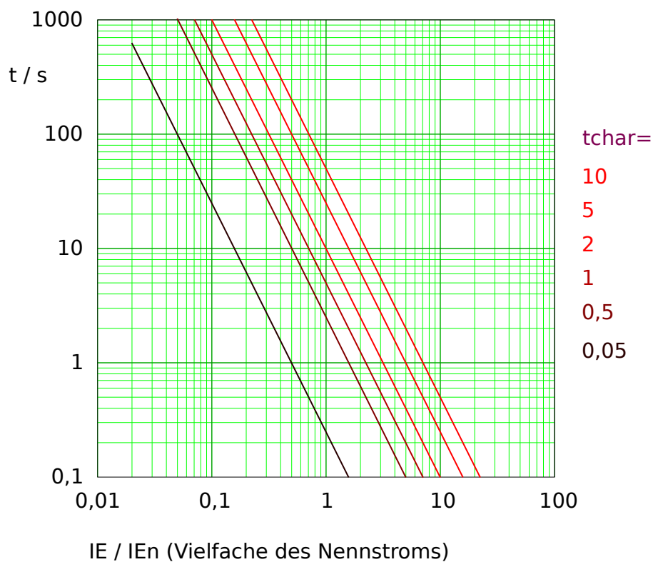
Abb. 103: Auslösekurve „I2T“, wobei nur der Bereich IE > IE_{n>} jeweils anwendbar ist. Beispieldiagramm für gemessenen (nicht empfindlichen) Erdstrom.
