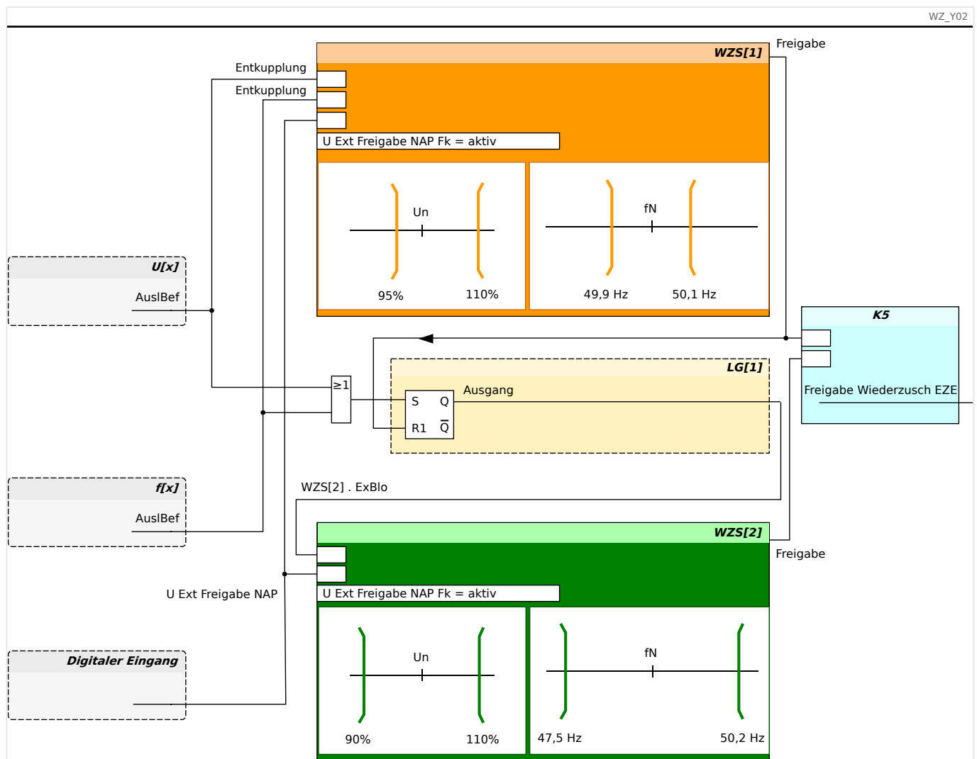
Abb. 129: Applikationsbeispiel für ein Zuschalten in Abhängigkeit von einer vorherigen Schutzauslösung.
