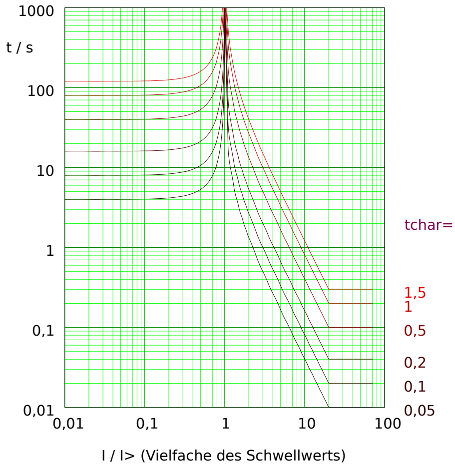
Abb. 82: EINV: Rückfallverzögerung (linke Hälfte, I < I_{>} ) und Auslöseverzögerung (rechte Hälfte, I > I_{>} ), Beispieldiagramm für I_{max} = 20 \cdot I_{>} .
