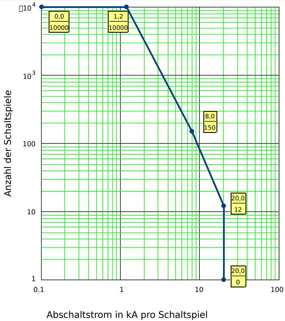
Abb. 154: Wartungskurve für einen typischen 25 kV Leistungsschalter
