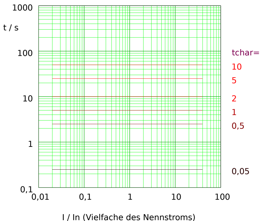
Abb. 88: Auslösekurve „Therm Flat“, wobei nur der Bereich I > I_0 jeweils anwendbar ist.
