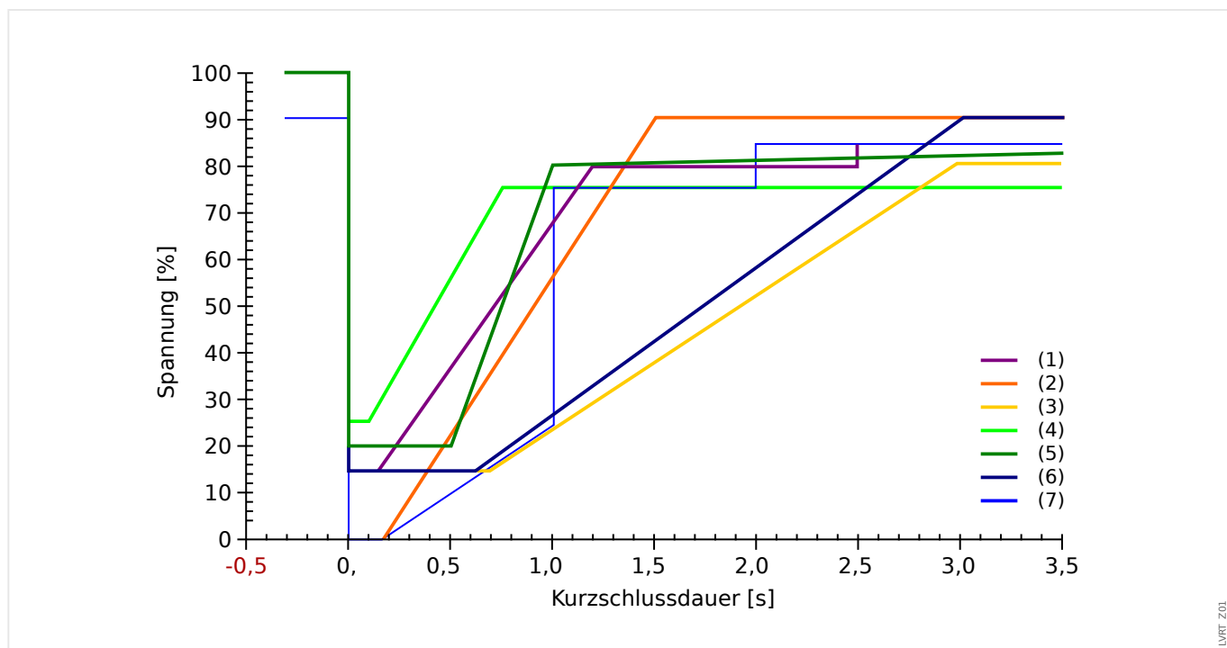
Abb. 138: Nationale LVRT-Standards, aus: eBWK Bd. 60 (2008) Nr. 4. Autoren: Dipl.-Ing. Thomas Smolka, Dr.-Ing. Karl-Heinz Weck, Zertifizierungstelle der FGH e.V., Mannheim, sowie Dipl.-Ing. (FH) Matthias Bartsch, Enercon GmbH, Aurich.
