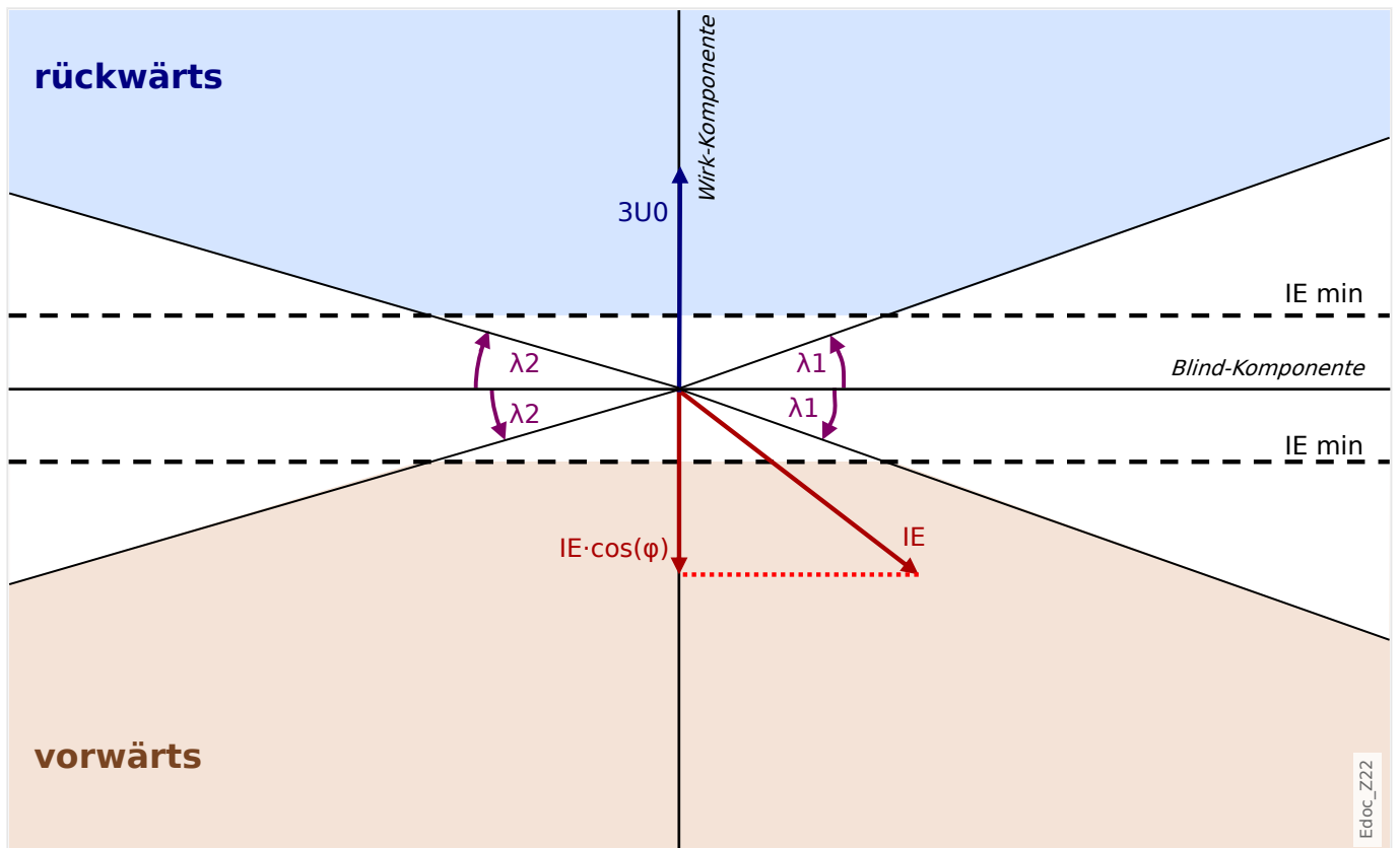
Abb. 68: Richtungserkennung nach der Methode „ \cos(\phi) “.
