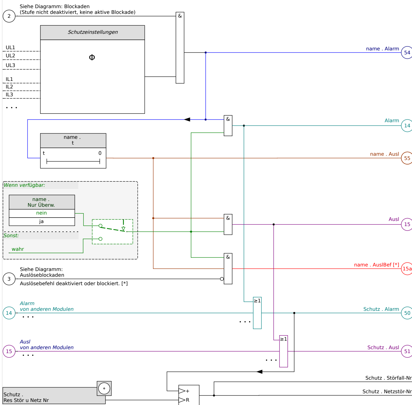
Abb. 64: Grobe Skizze der Funktionalität einer HighPROTEC-Schutzfunktion.
