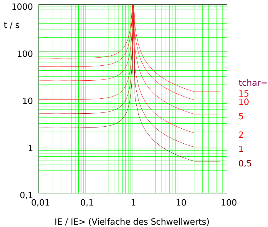
Abb. 96: MINV: Rückfallverzögerung (linke Hälfte, IE < IE> ) und Auslöseverzögerung (rechte Hälfte, IE > IE> ), Beispieldiagramm für I_{E,max} = 20 \cdot IE> .
