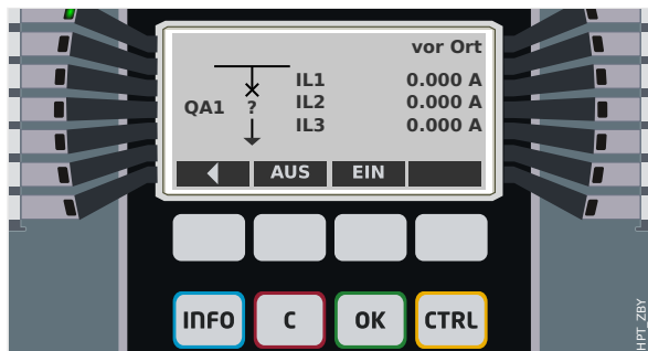
Abb. 150: Beispiel einer Steuer-Seite mit „Leistungsschalter“ in Störstellung (bzw. unplausiblem Zustand).
