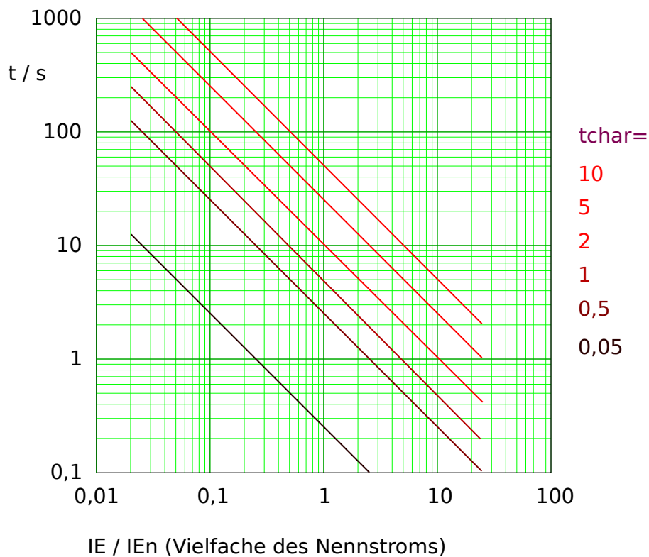
Abb. 102: Auslösekurve „IT“, wobei nur der Bereich IE > IE_n jeweils anwendbar ist. Beispieldiagramm für gemessenen (nicht empfindlichen) Erdstrom.
