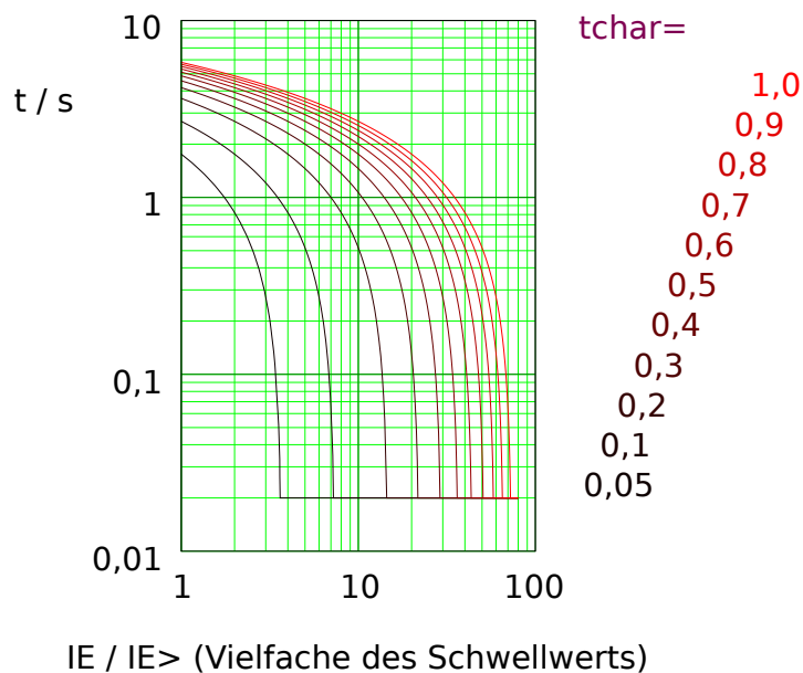
Abb. 100: RXIDG: Auslöseverzögerung, IE > IE > .
