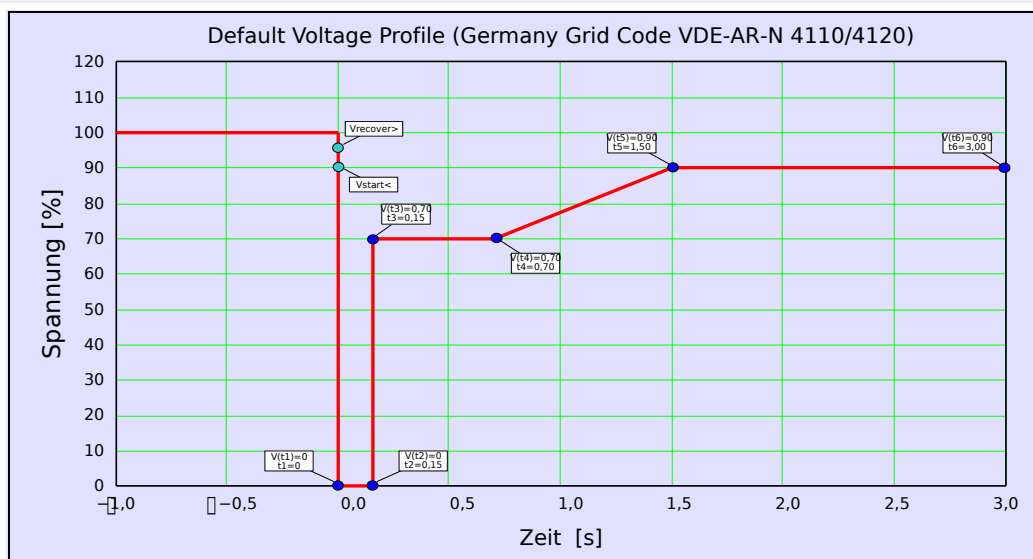
Abb. 141: LVRT-Werkseinstellung (Typ I).
