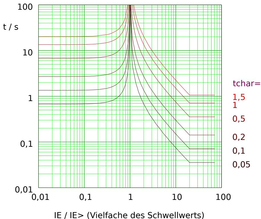
Abb. 93: VINV: Rückfallverzögerung (linke Hälfte, IE < IE_{max} ) und Auslöseverzögerung (rechte Hälfte, IE > IE_{max} ), Beispieldiagramm für IE_{max} = 20 \cdot IE_{nom} .
