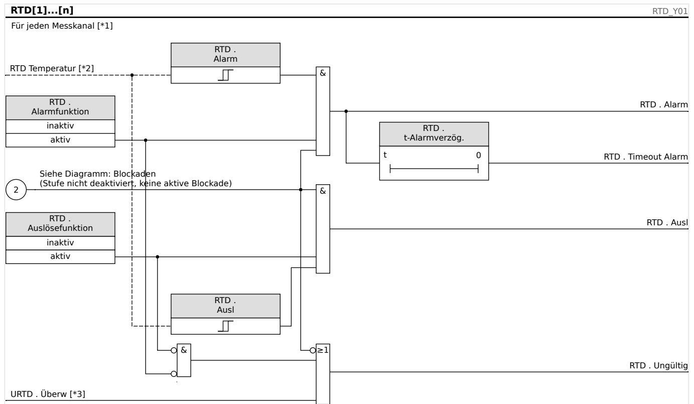
Abb. 144: Generelles RTD-Funktionsprinzip.
