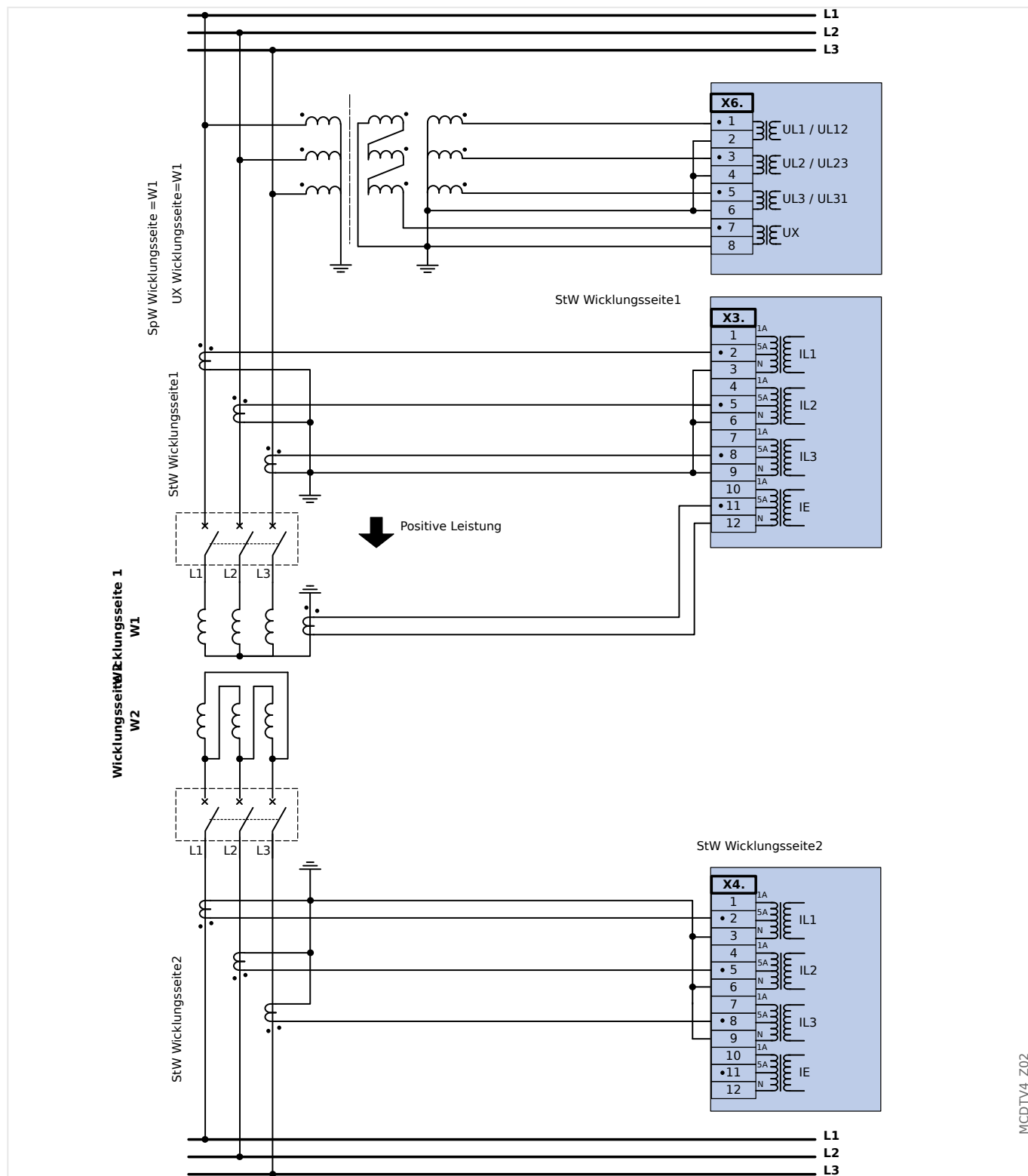
Abb. 39: DY-Transformator mit Phasendifferenzialschutz und Erddifferenzialschutz auf der Seite W1.
