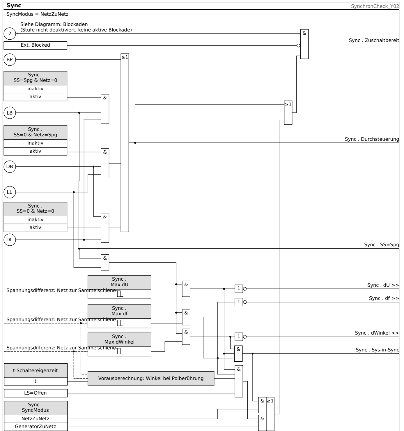
Abb. 125: Funktionalität des »Sync«-Moduls, „NetzZuNetz“.
