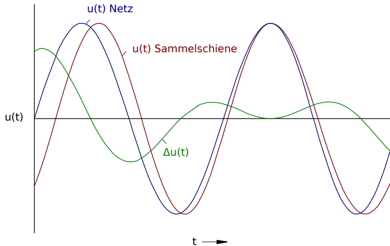
Abb. 123: Spannungsverlauf der Schwebespannung \Delta u(t) , vergrößert.
