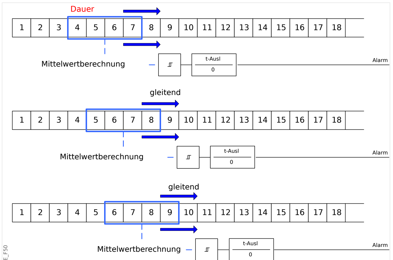
Abb. 155: Statistikmethode = gleitend
