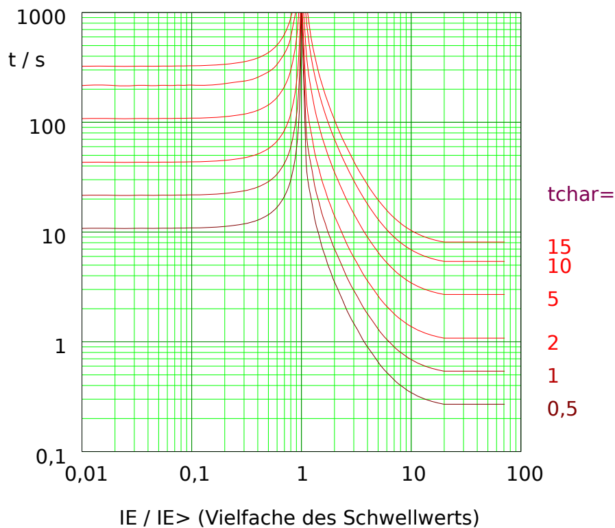
Abb. 97: VINV: Rückfallverzögerung (linke Hälfte, IE < IE> ) und Auslöseverzögerung (rechte Hälfte, IE > IE> ), Beispieldiagramm für I_{E,max} = 20 \cdot IE> .
