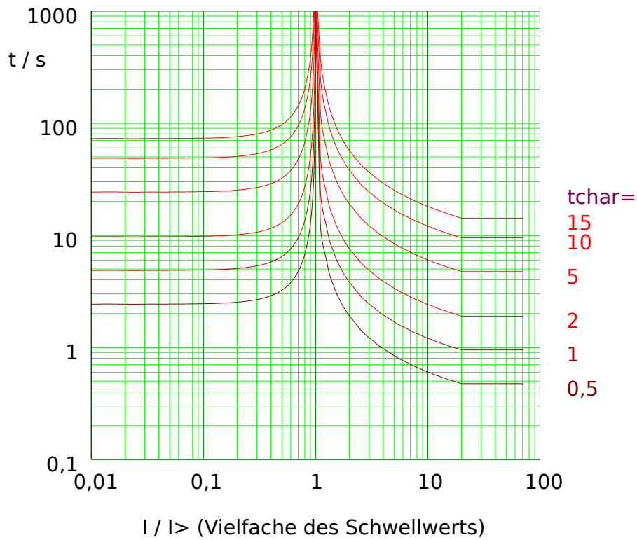
Abb. 84: MINV: Rückfallverzögerung (linke Hälfte, I < I > ) und Auslöseverzögerung (rechte Hälfte, I > I > ), Beispieldiagramm für I_{max} = 20 \cdot I > .
