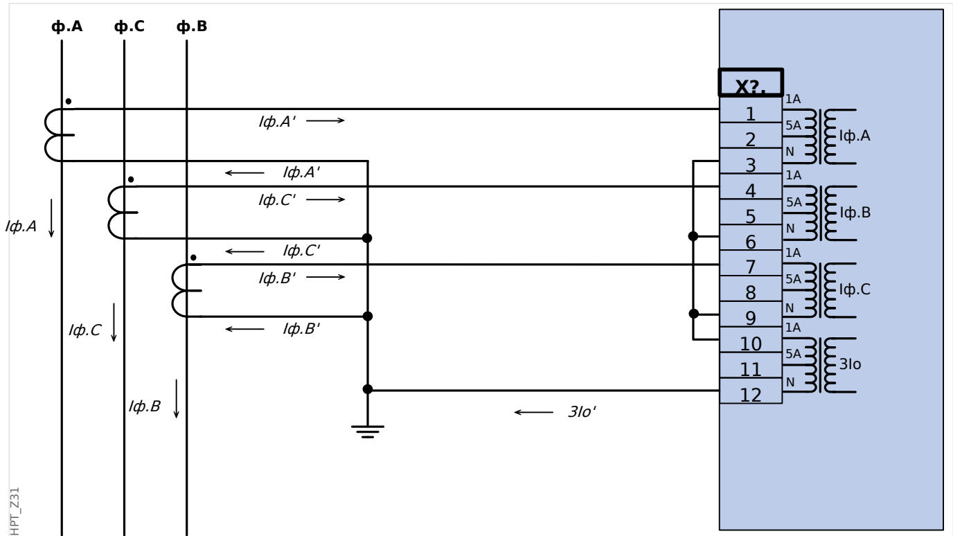
Рис. 25: Измерение фазных токов по схеме «полной» звезды; I_n вторичн. = 1 А. Ток на землю, измеряемый через соединение по схеме Холмгринна 3I_o . ном.втор. = 1 А.
