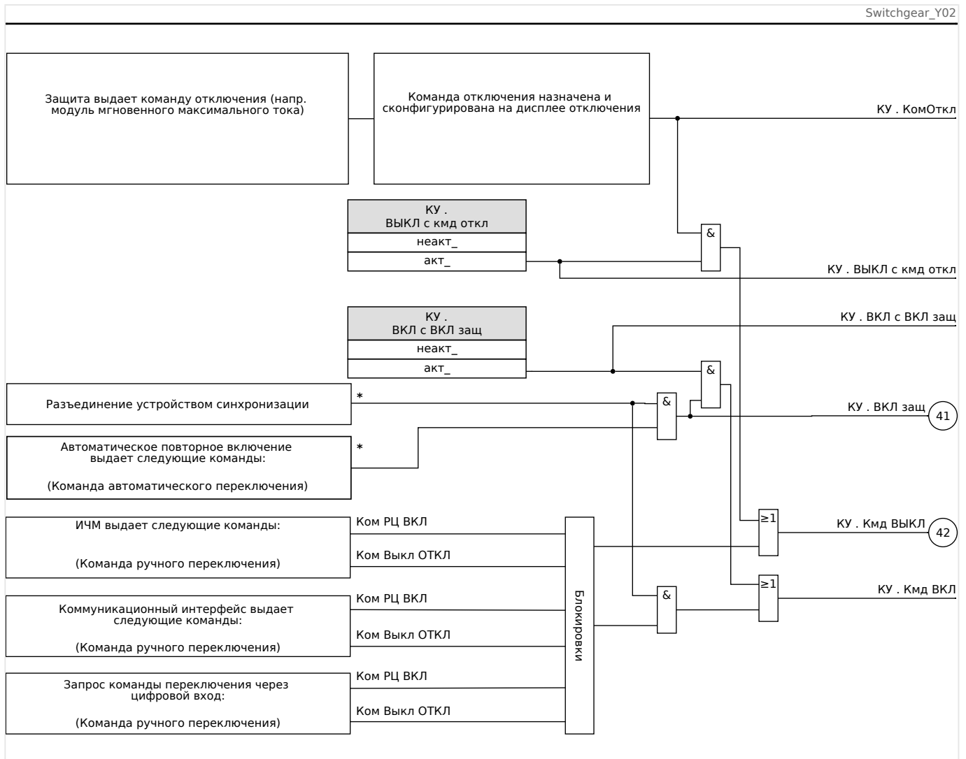
Рис. 127: Блокировки. (Детали, отмеченные «*»: наличие зависит от заказанного типа устройства.)
