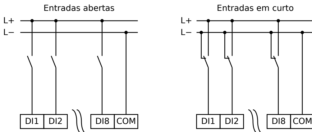
Fig. 144: Estado seguro das entradas digitais
