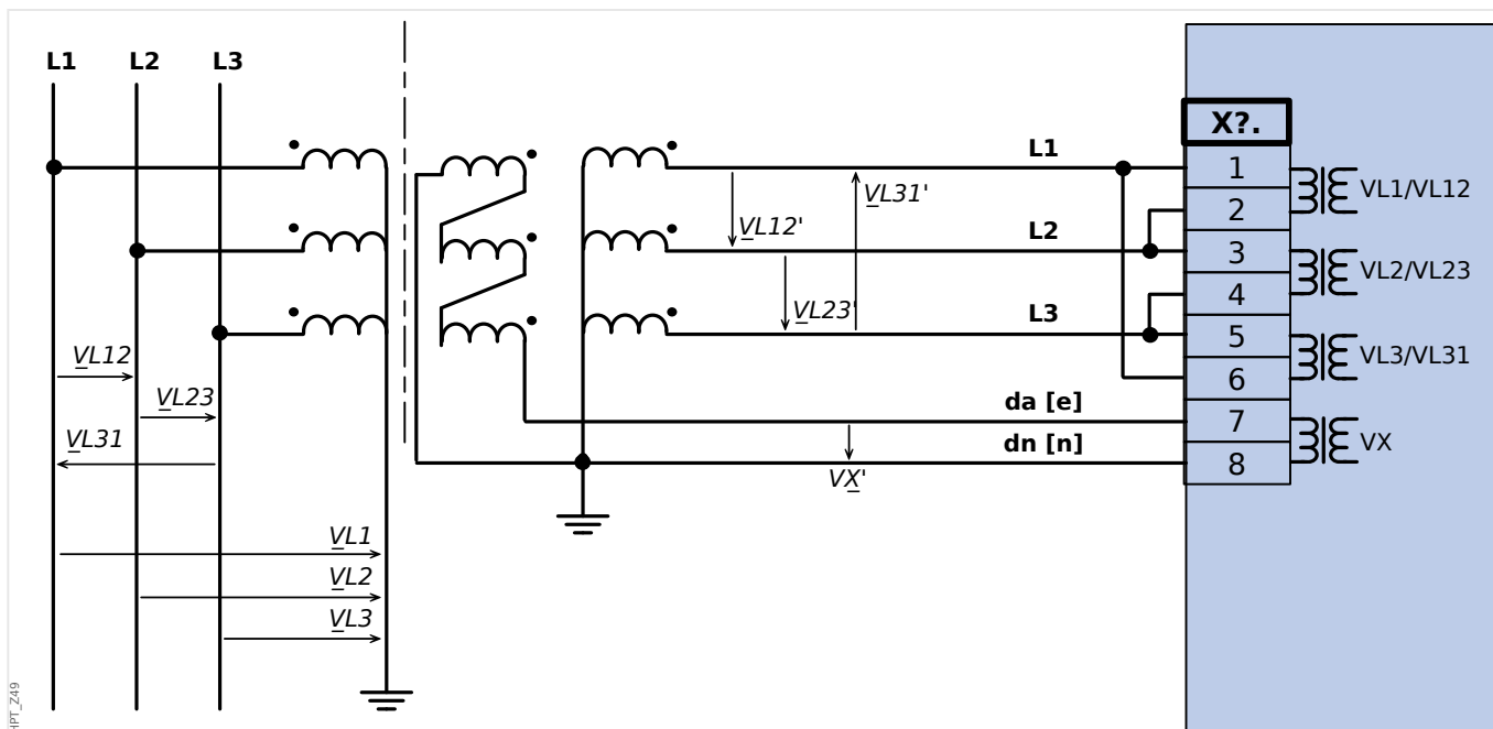
Fig. 37: Medição VG voltagem residual por meio de "delta aberto" (e-n) de circuito auxiliar
