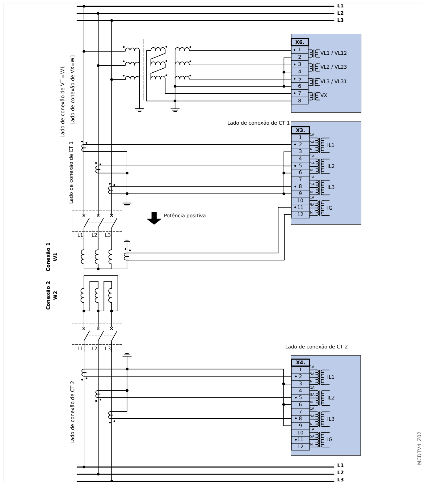
Fig. 39: Transformador DY com Proteção Diferencial de Fase e Proteção Diferencial de Terra no W1 apenas.
