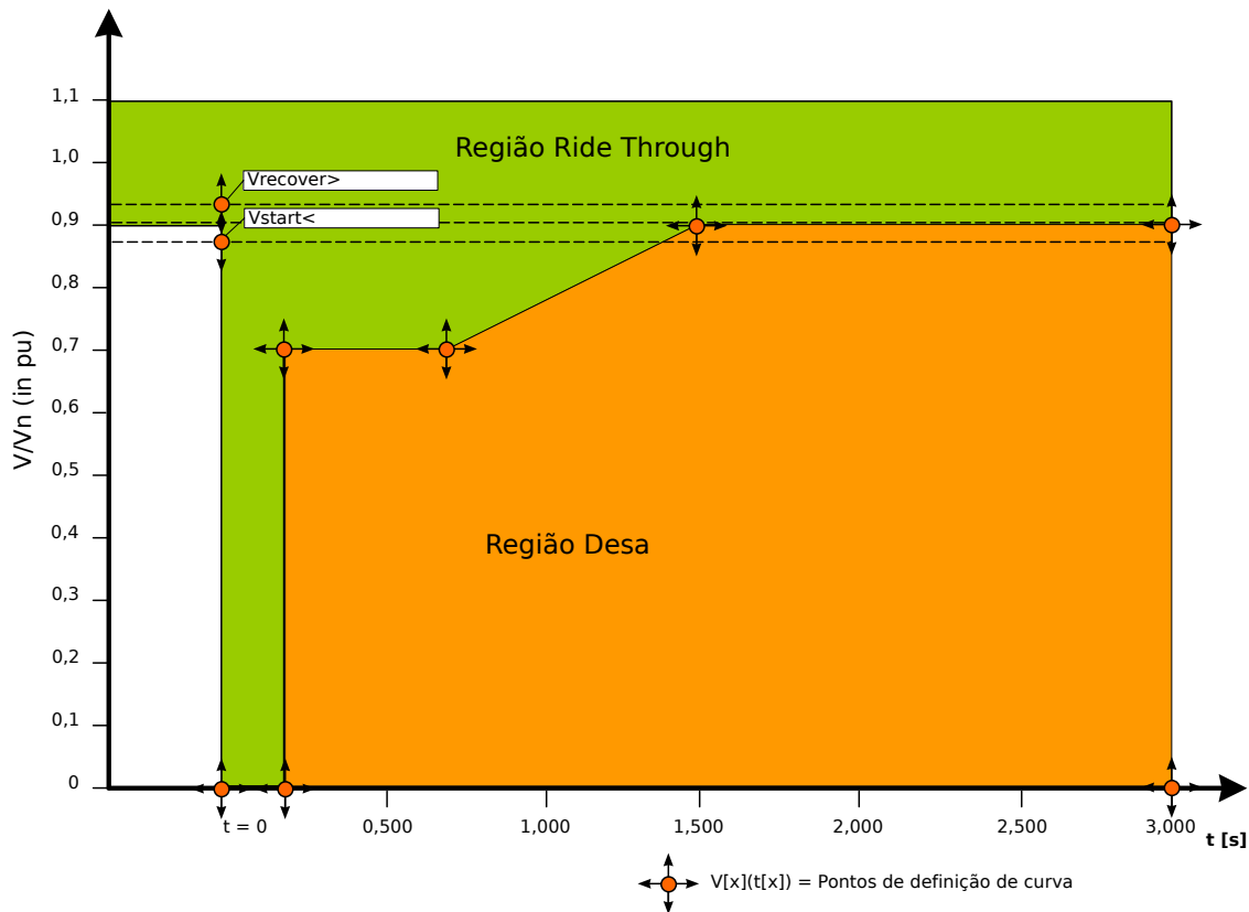
Fig. 115: Região de “passagem” e região de “disparo”.
