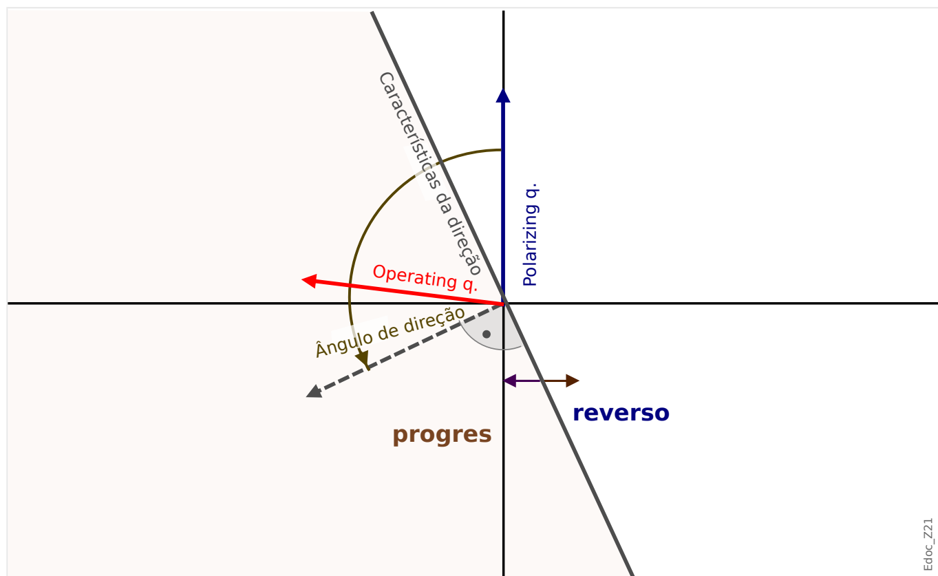
Fig. 67: Princípio de determinação da direção para todos os métodos, exceto “ \cos(\phi) ”, “ \sin(\phi) ”.
