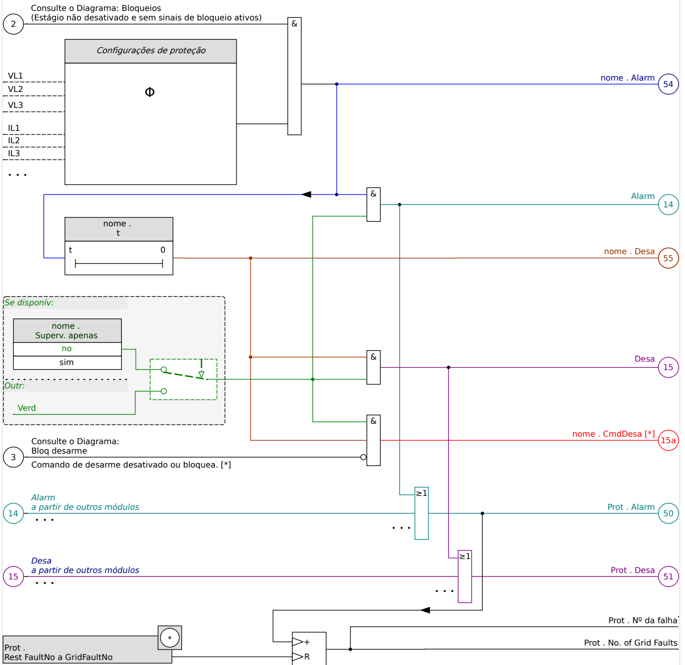
Fig. 64: Esboço rápido da funcionalidade de qualquer HighPROTEC elemento de proteção.
