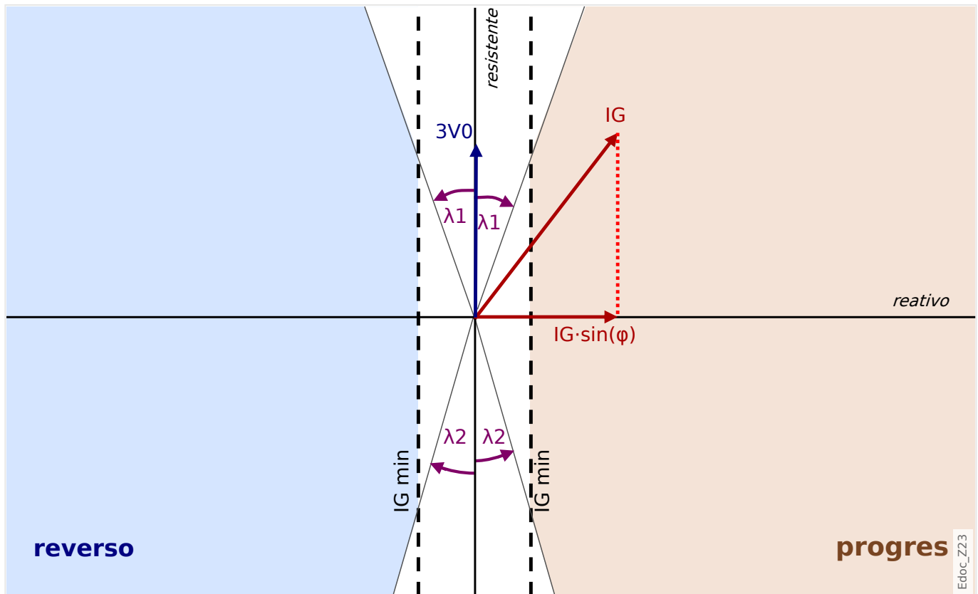
Fig. 70: Princípio de determinação da direção para o método " \sin(\phi) ".
