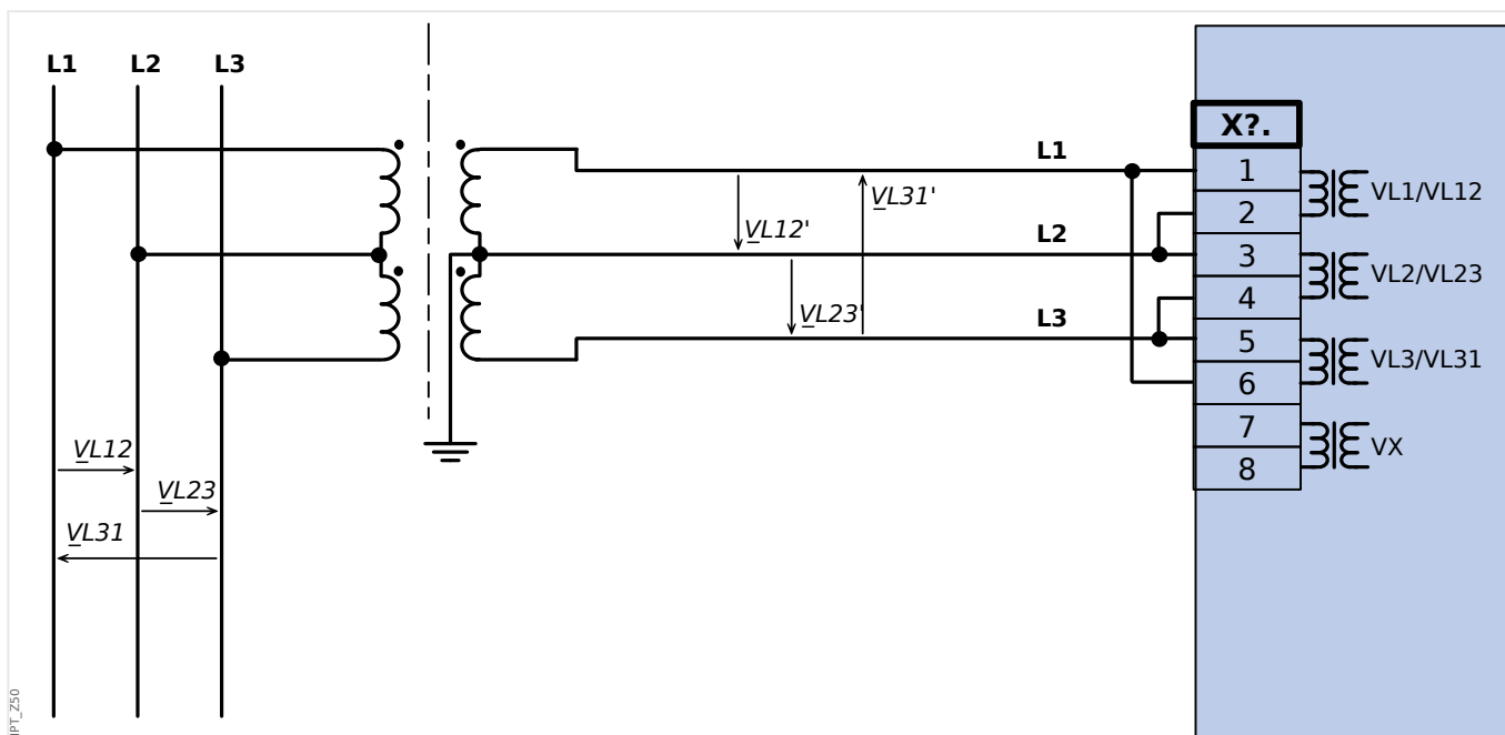
Fig. 38: Medição de voltagem bifásica - fiação das entradas de medição: "Delta Aber"
