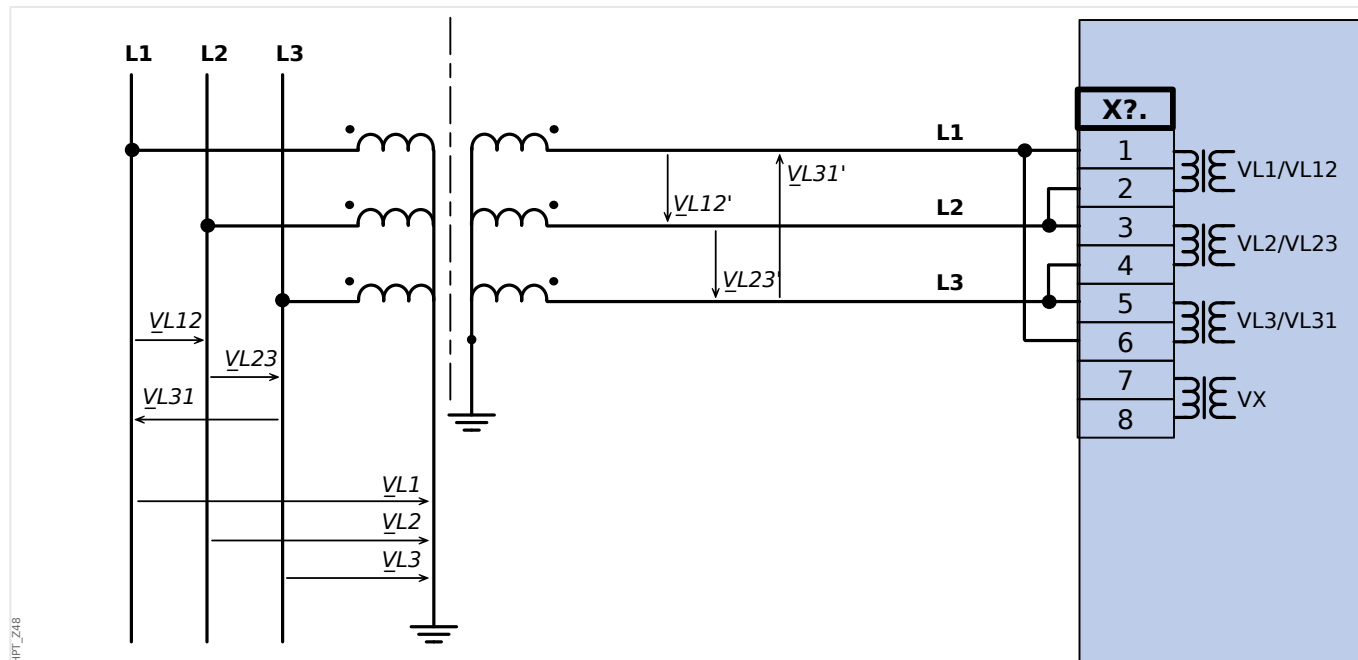
Fig. 36: Medição de tensão trifásica - fiação das entradas de medição: "conexão-delta"
