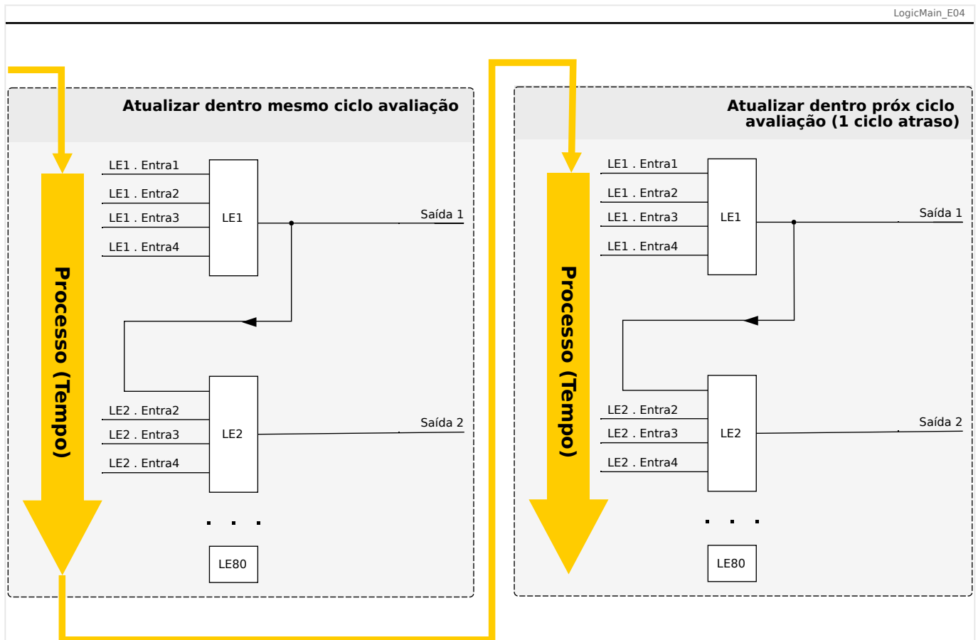
Fig. 138: Em cascata crescente.
