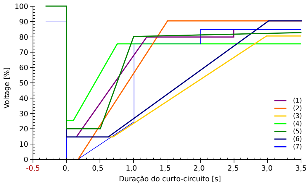
Fig. 113: Padrões LVRT; fonte: eBWK Bd. 60 (2008) Nr. 4. Autores: Dipl.-Ing. Thomas Smolka, Dr.-Ing. Karl-Heinz Weck, Zertifizierungstelle der FGH e.V., Mannheim, sowie Dipl.-Ing. (FH) Matthias Bartsch, Enercon GmbH, Aurich.
