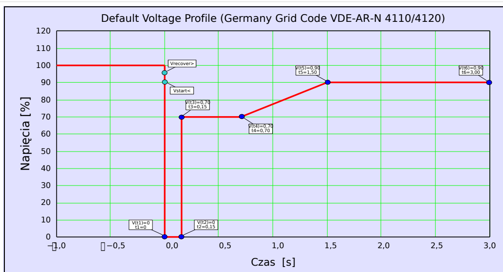
Rys. 116: Profil domyślny LVRT (typ I).
