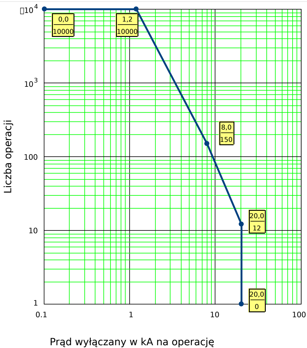
Rys. 129: Krzywa konserwacji wyłącznika typowego wyłącznika 25 kV
