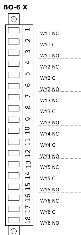
Rys. 13: Przepisanie elektromechaniczne
