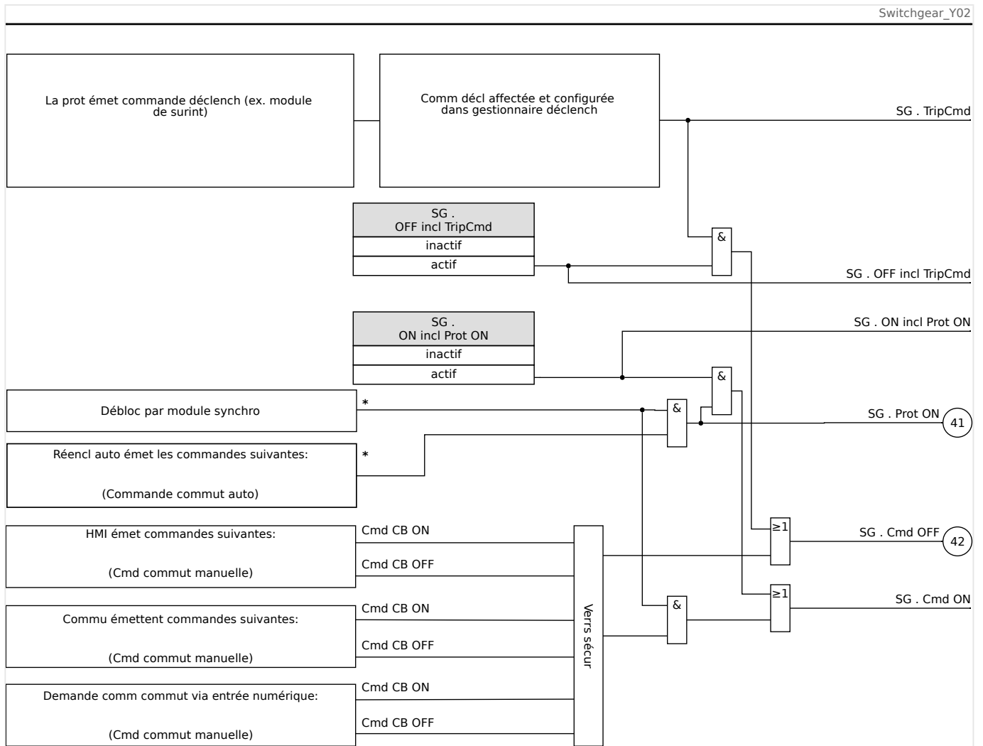
Fig. 127: Verrouillages (Parties identifiées par « * » : la disponibilité dépend du type de dispositif commandé.)
