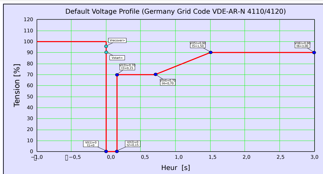
Fig. 116: Profil LVRT prédéfini en usine (Type I).
