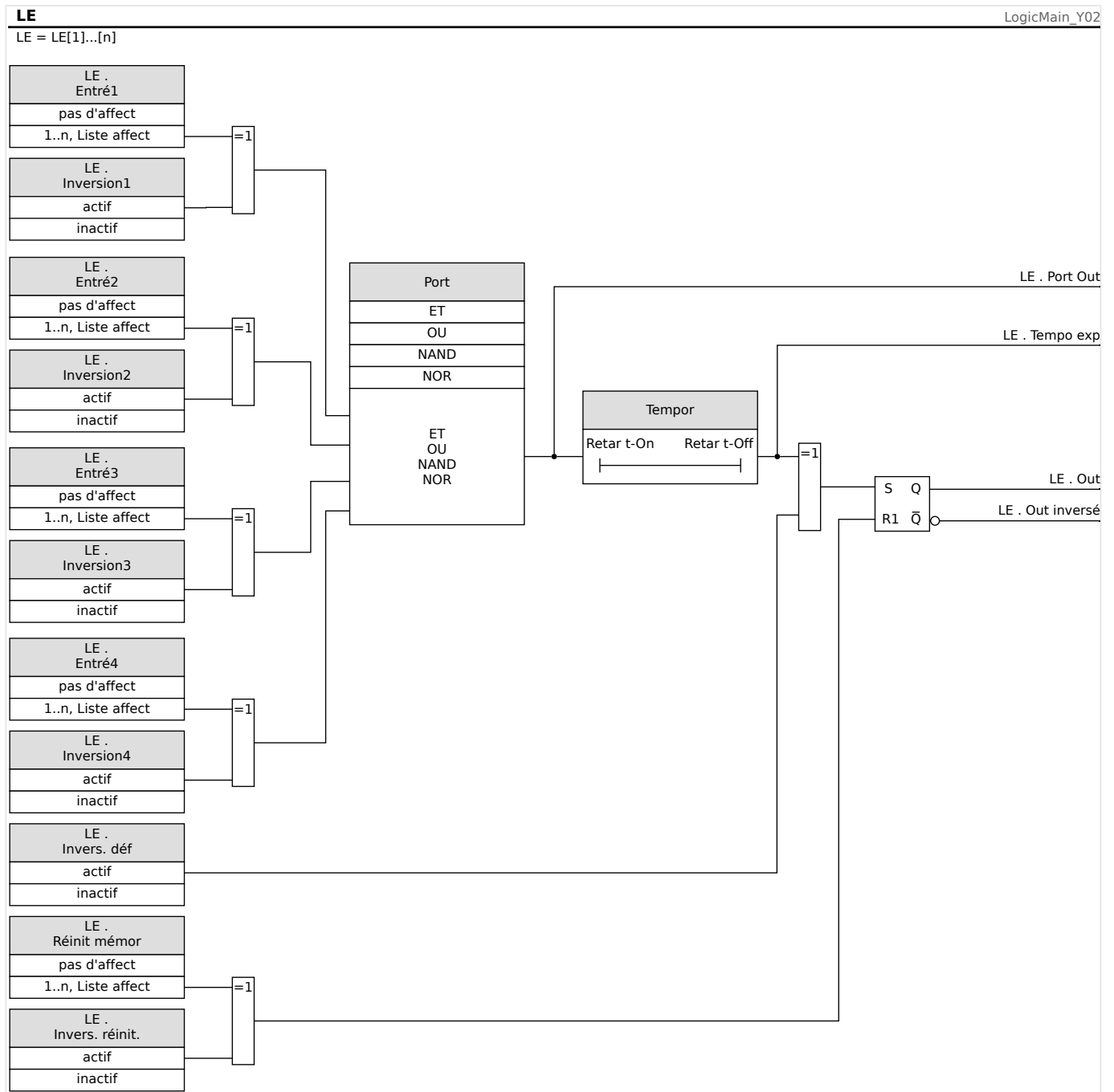
Fig. 136: Présentation détaillée - Diagramme logique global.
