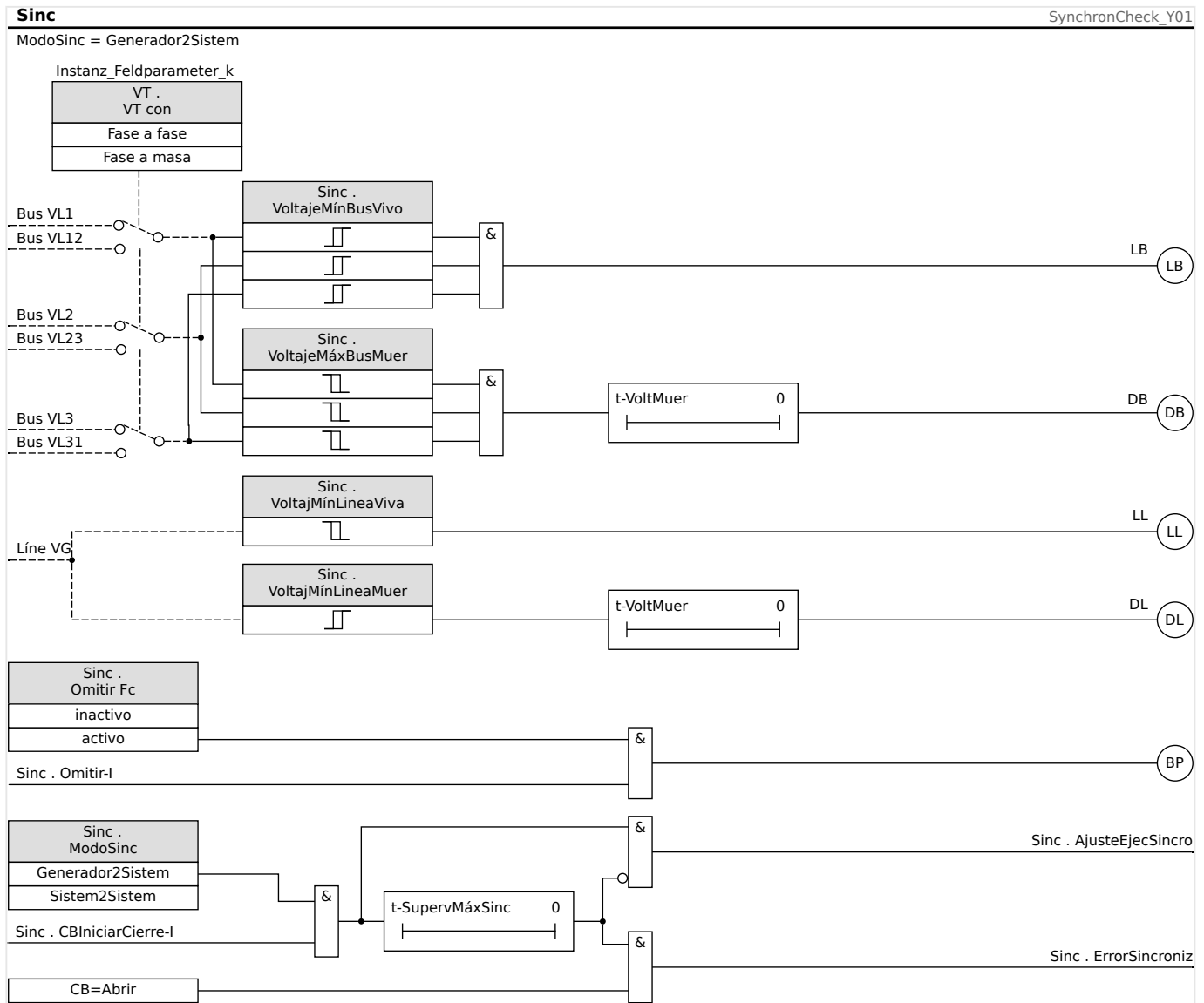
Fig. 100: Funcionalidad del módulo »Sinc«, «Generador2Sistem».
