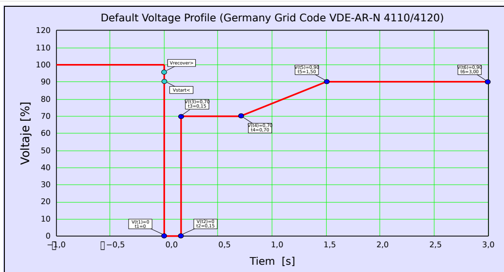
Fig. 116: Perfil de LVRT predeterminado (Tipo I).
