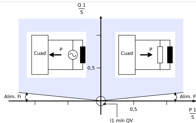
Fig. 103: Método 1: Supervisión de ángulo de potencia
