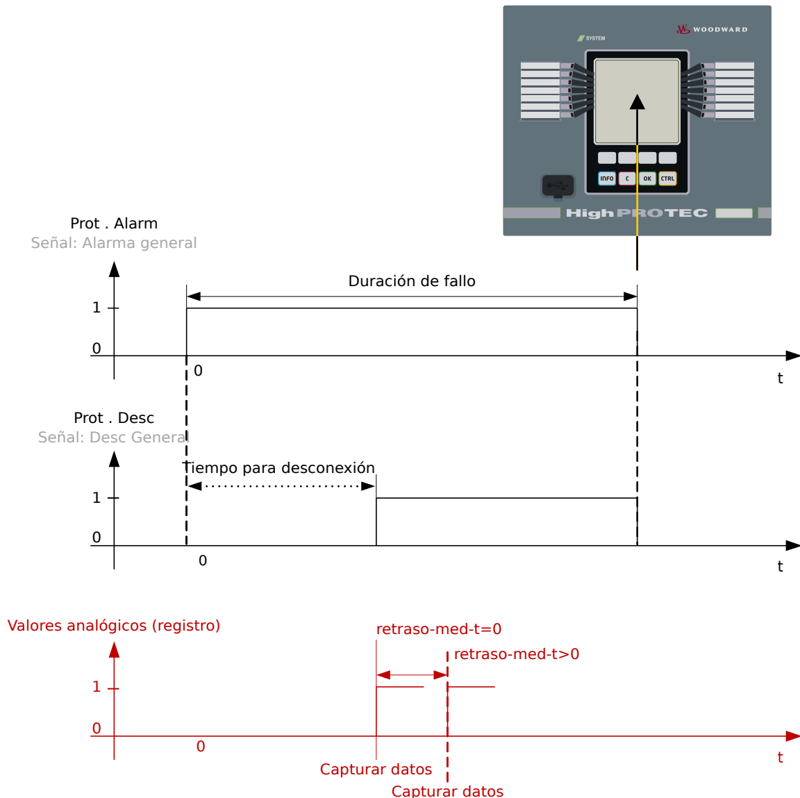
Fig. 134: Registrador de fallos: tiempos y duraciones.
