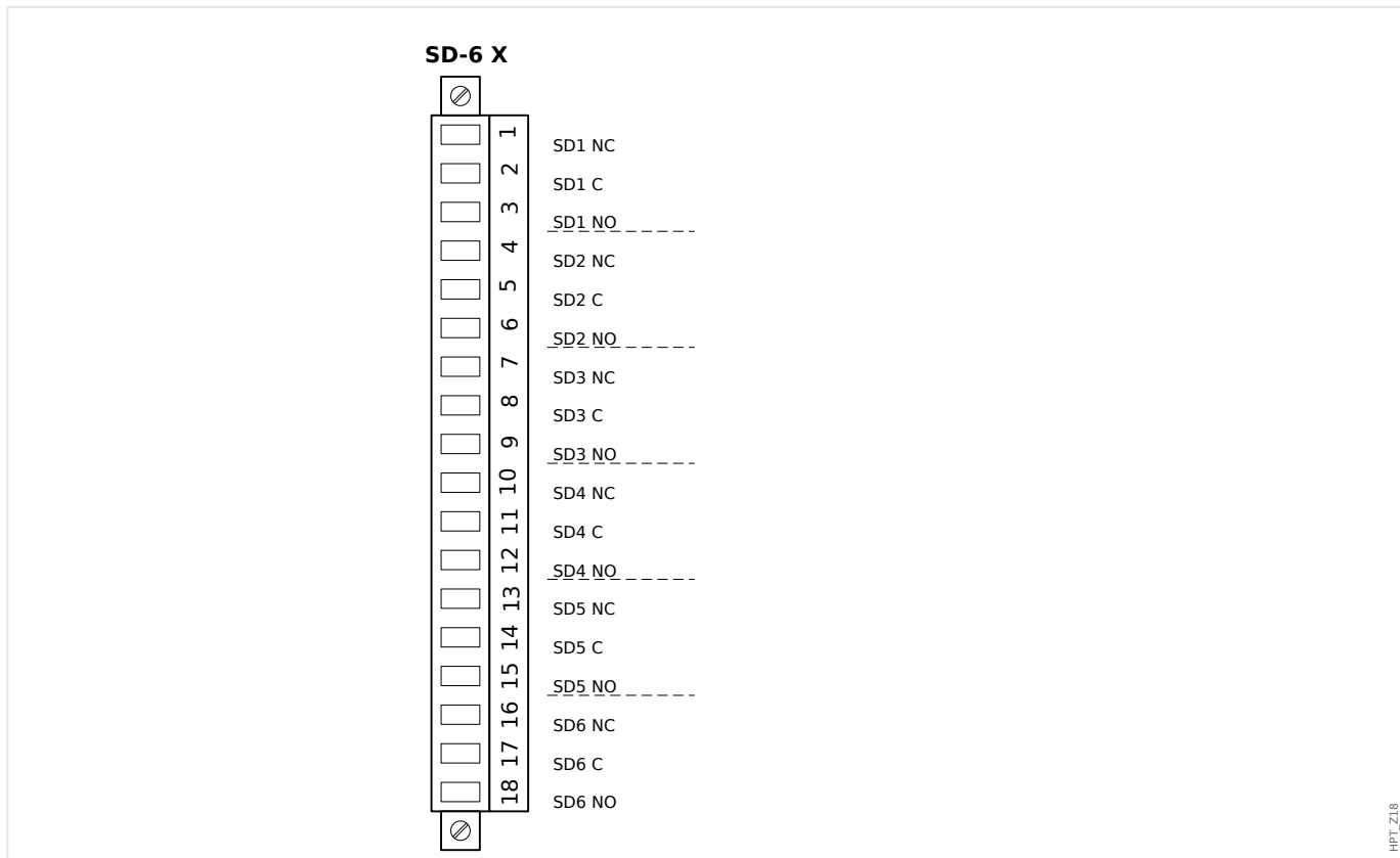
Fig. 13: Asignación electromecánica
