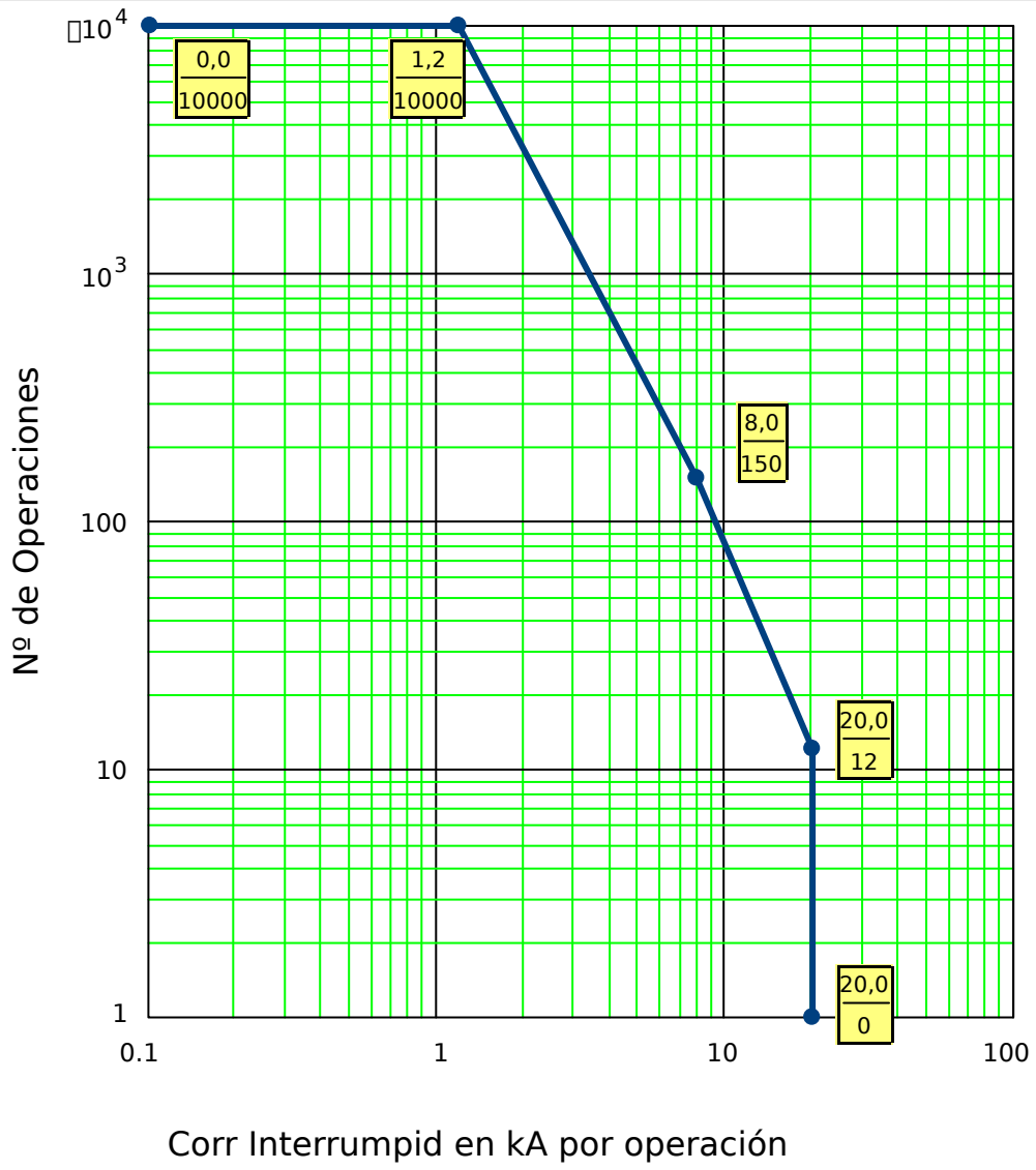
Fig. 129: Curva Mantenim Interruptor para Interrupt Circuito típico 25kV
