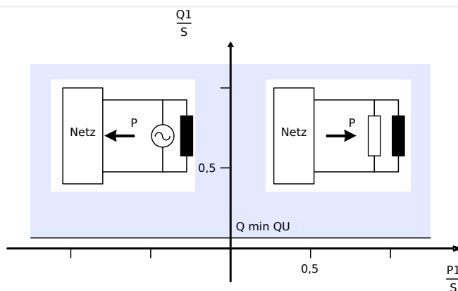
Abb. 103: Variante 2: Reine Blindleistungsschwellwertüberwachung.
