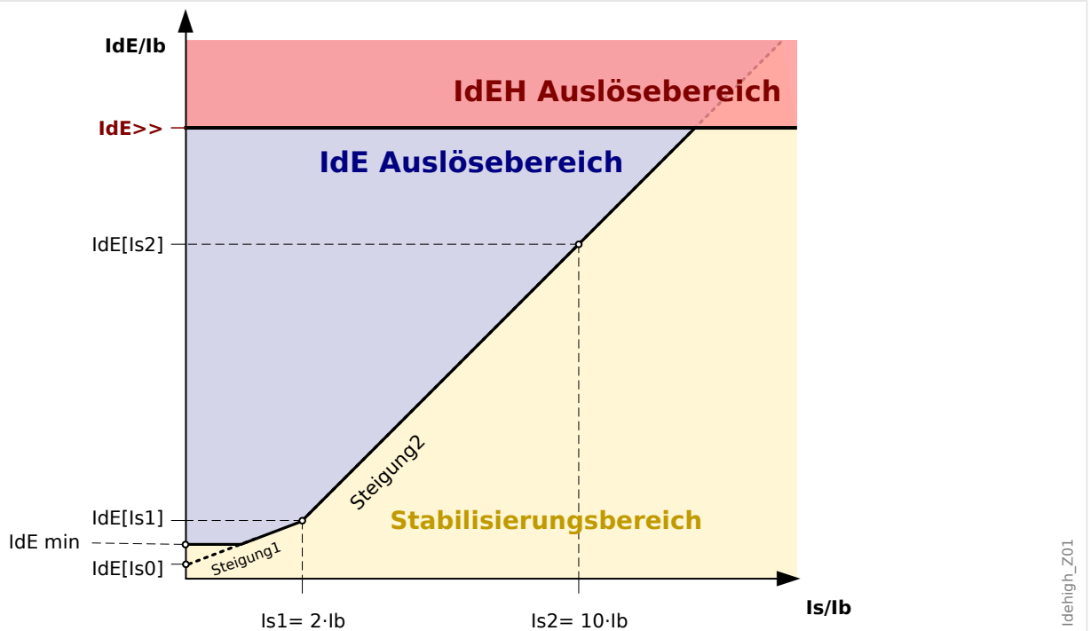
Abb. 79: Ansprechwert »IdE>>« des Erddifferenzialstromes bezogen auf den Nennstrom »lb« des entsprechenden Schutzobjektes.
