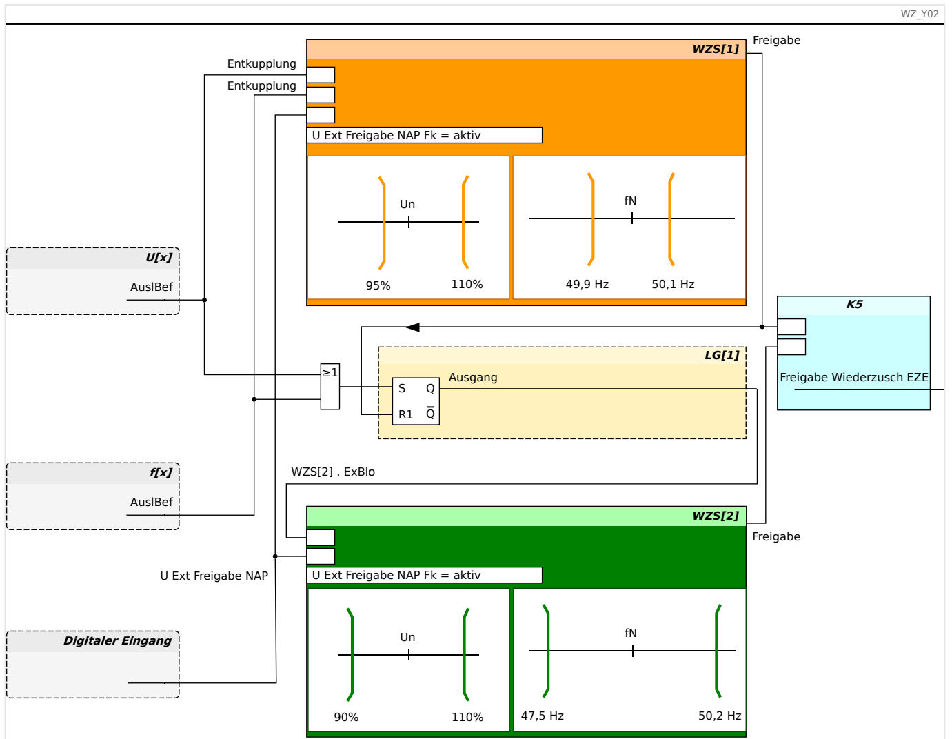
Abb. 104: Applikationsbeispiel für ein Zuschalten in Abhängigkeit von einer vorherigen Schutzauslösung.
