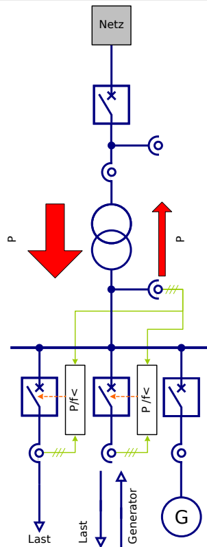
Abb. 108: Dezentrale Automatische Frequenzentlastung in Netzen mit zeitweiser Rückspeisung.
