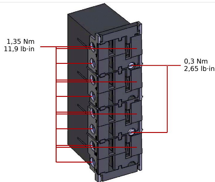
Рис. 142: Штепсельные соединения со встроенными закорачивающими перемычками (стандартные токовые входы)
