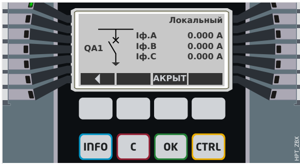
Рис. 124: Пример страницы управления, выключатель в разомкнутом положении.
