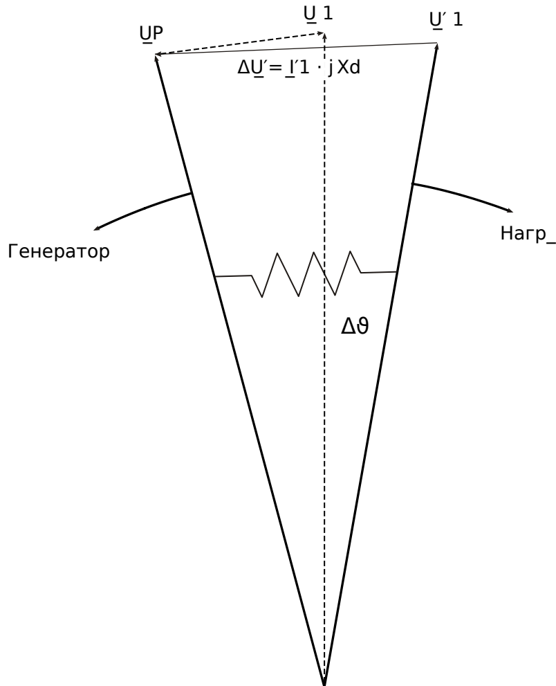
Рис. 93: Векторы напряжения при сбое электросети.
