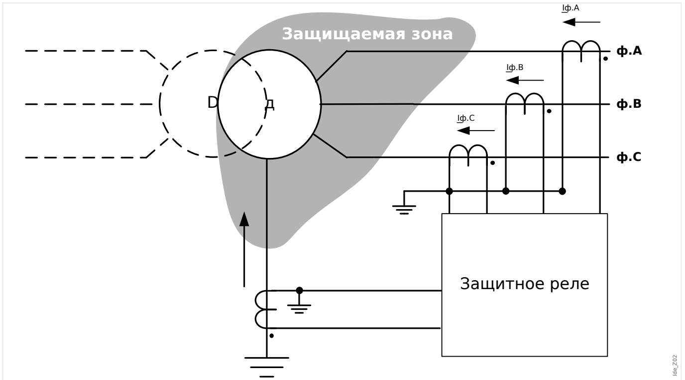
Рис. 77: Принцип работы дифференциальной токовой защиты обмоток трансформаторов, соединенных по схеме «звезда».
