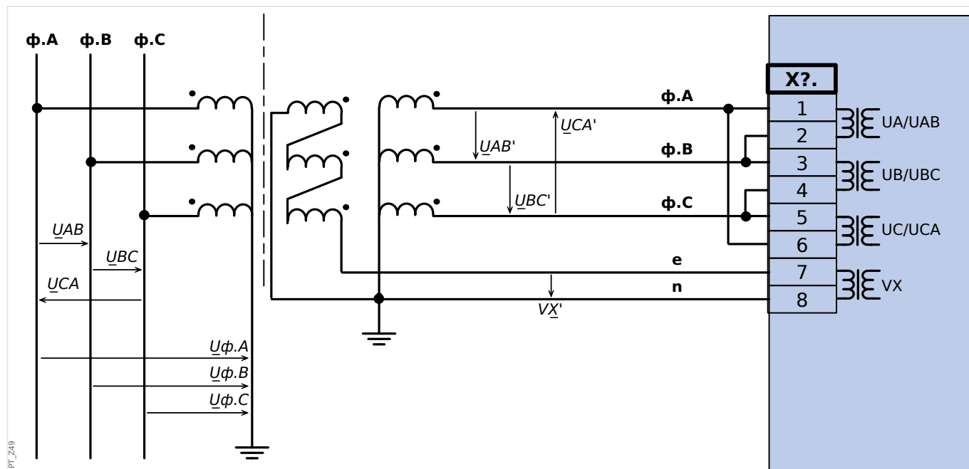
Рис. 37: Измерение трехфазного напряжения - схема измерительных входов: "соединение треугольником" Измерение напряжения нулевой последовательности V_G через вспомогательные обмотки (e-n) («открытый треугольник»)
