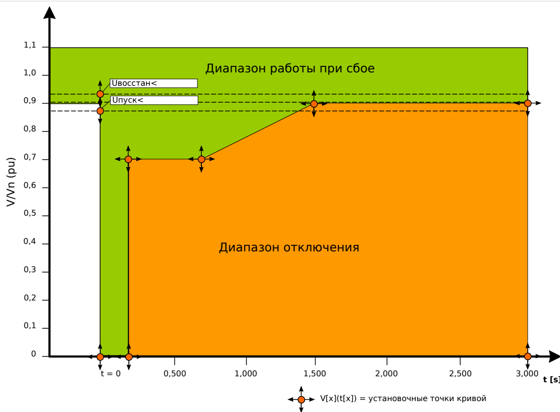
Рис. 113: Область продолжения работы и область отключения.
