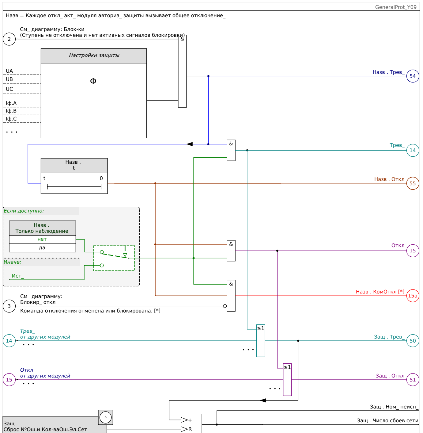
Рис. 63: Примерная схема функций любого элемента защиты HighPROTEC.
