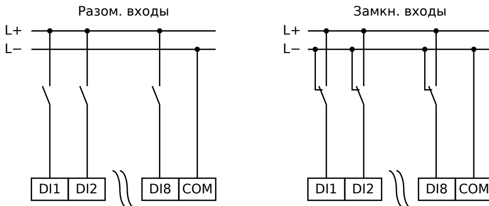
Рис. 144: Безопасное состояние цифровых входов
