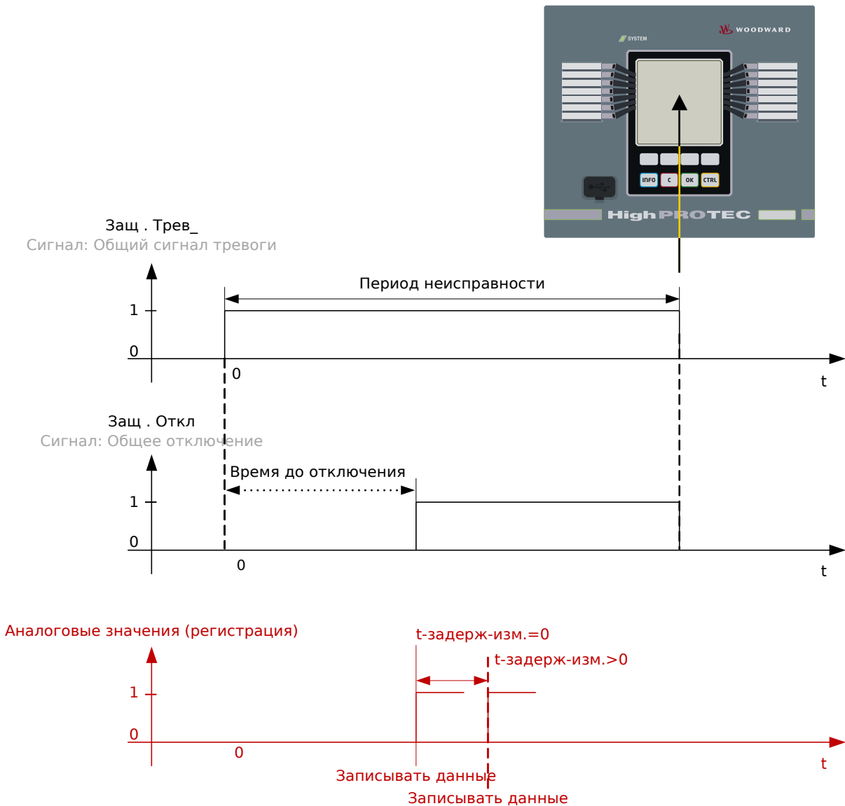
Рис. 132: Регистратор неисправностей: время и длительность.
