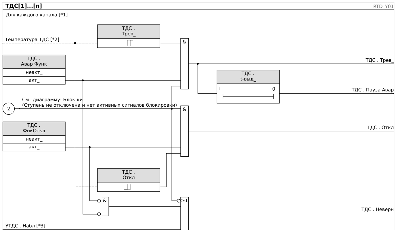
Рис. 117: Общий принцип работы (аварийный сигнал с задержкой, отключение без задержки).
