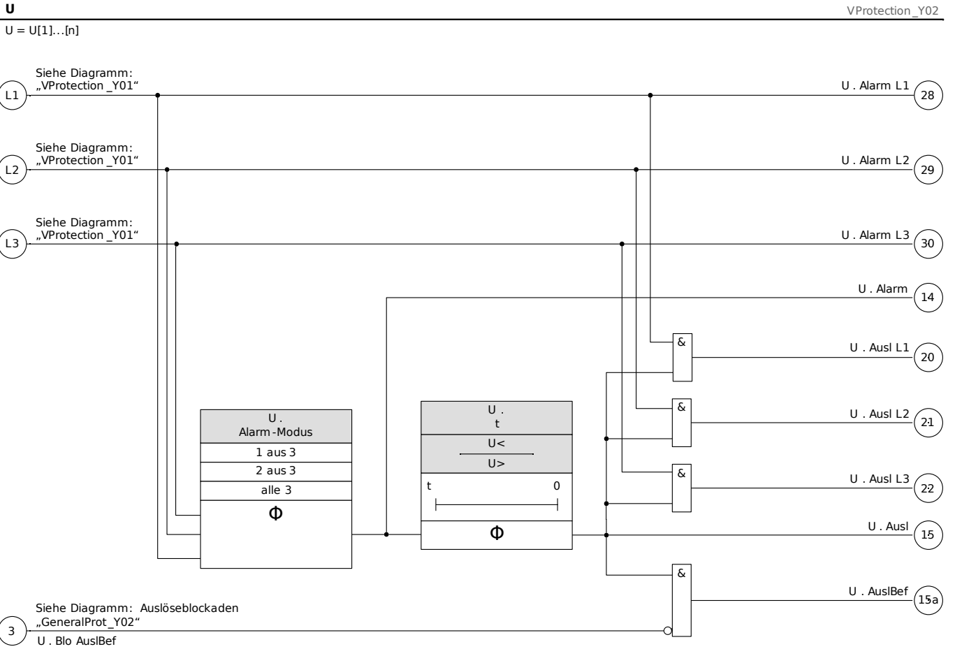
Funktionalität des Spannungsschutzmoduls, Teil 2.
