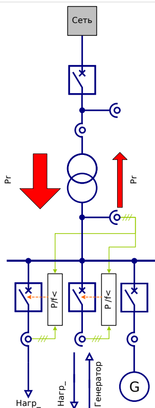
Рис. 118: Децентрализованная автоматическая частотная разгрузка в сетях с временным электроснабжением.
