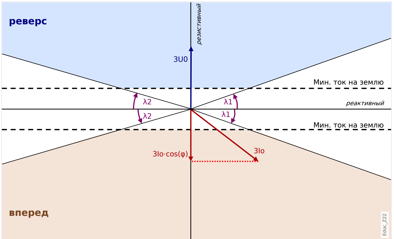
Рис. 67: Принцип определения направления для метода « \cos(\phi) ».
