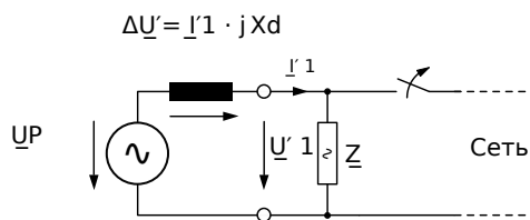
Рис. 104: Эквивалентная цепь при сбое электросети.
