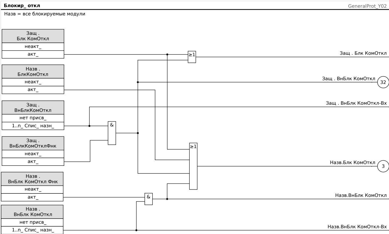
Рис. 71: Активация и деактивация команды отключения модуля защиты
