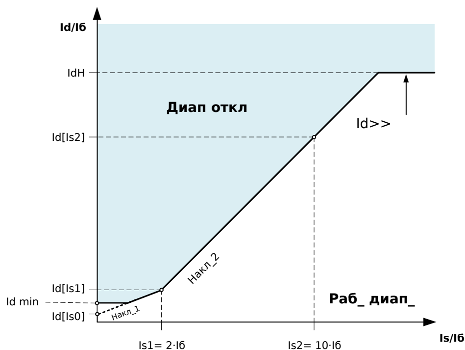
Рис. 77: Этап неограниченной дифференциальной защиты с высокой уставкой I_{dH} .
