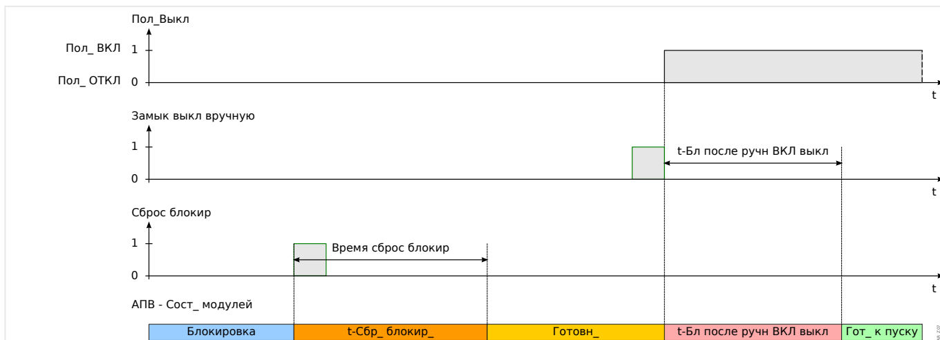
Рис. 96: Логика сброса блокировки АПВ при получении команды сброса блокировки перед замыканием выключателя вручную.
