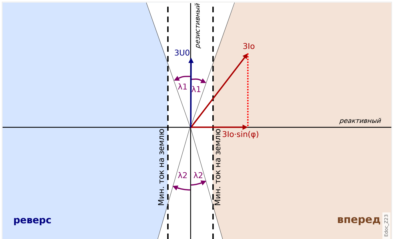
Рис. 68: Принцип определения направления для метода «sin(φ)».
