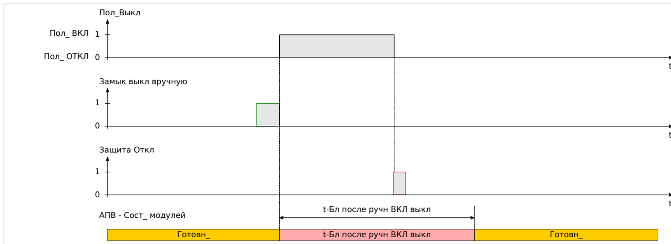
Рис. 95: Отключение защиты во время работы таймера блокировки замыкания вручную.
