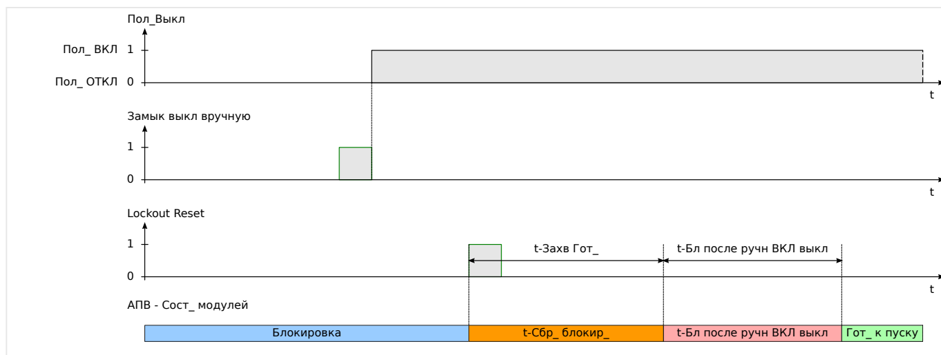
Рис. 97: Логика сброса блокировки АПВ при получении команды сброса блокировки после замыкания выключателя вручную.
