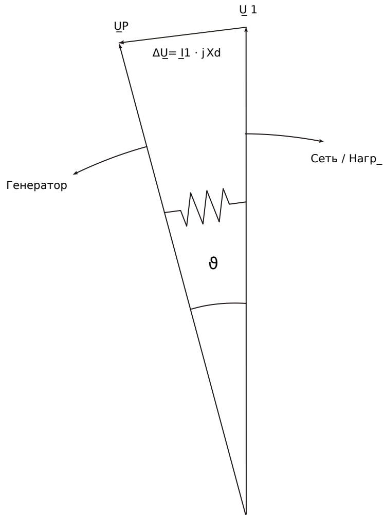
Рис. 103: Векторы напряжения в параллельной работе с электросетью.
