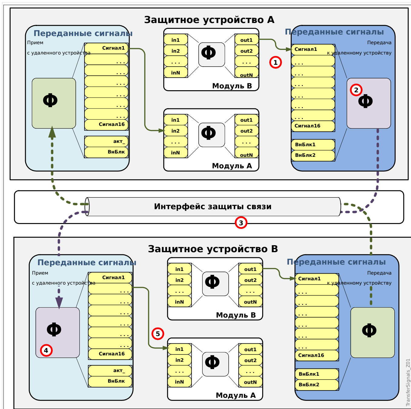
Рис. 82: Принцип работы «Передача сигнала».
