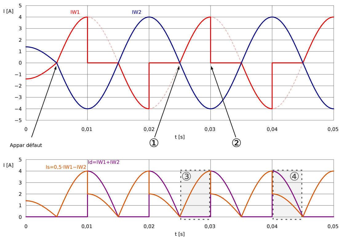
Fig. 76: Caractéristique de I_d et I_s avec saturation côté CT W1 pour un défaut externe.
