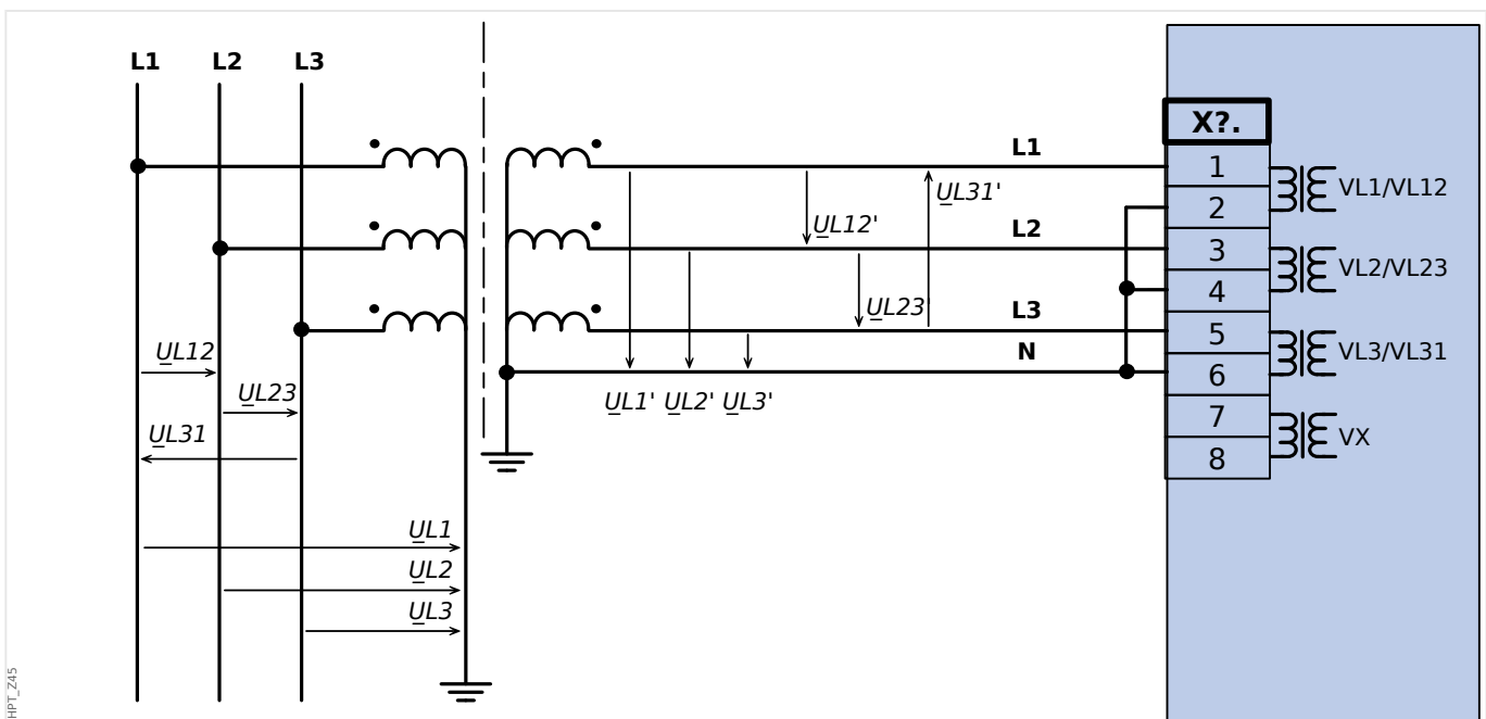
Fig. 30: VT Wye : Mesure de tension triphasée - câblage des entrées de mesure: "connex étoile"
