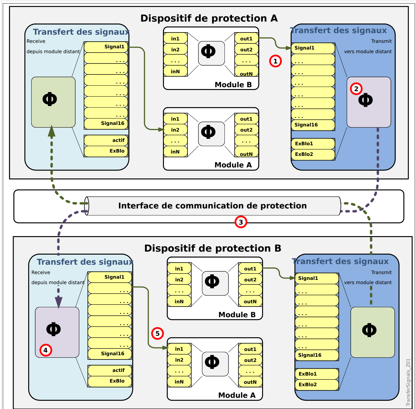
Fig. 82: Principe de la fonctionnalité «Sig-Trans».
