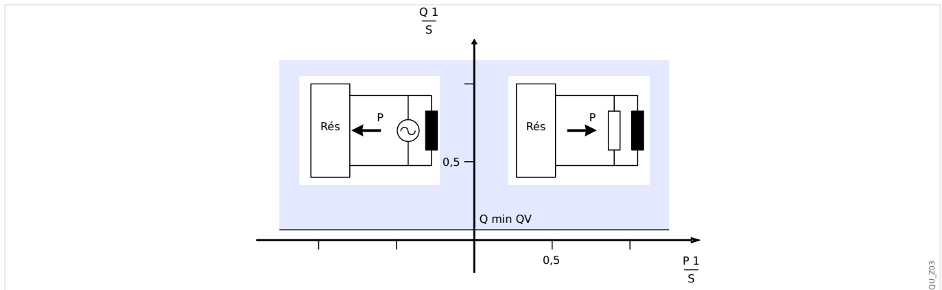
Fig. 114: Méthode 2 : Surveillance de la puissance réactive pure
