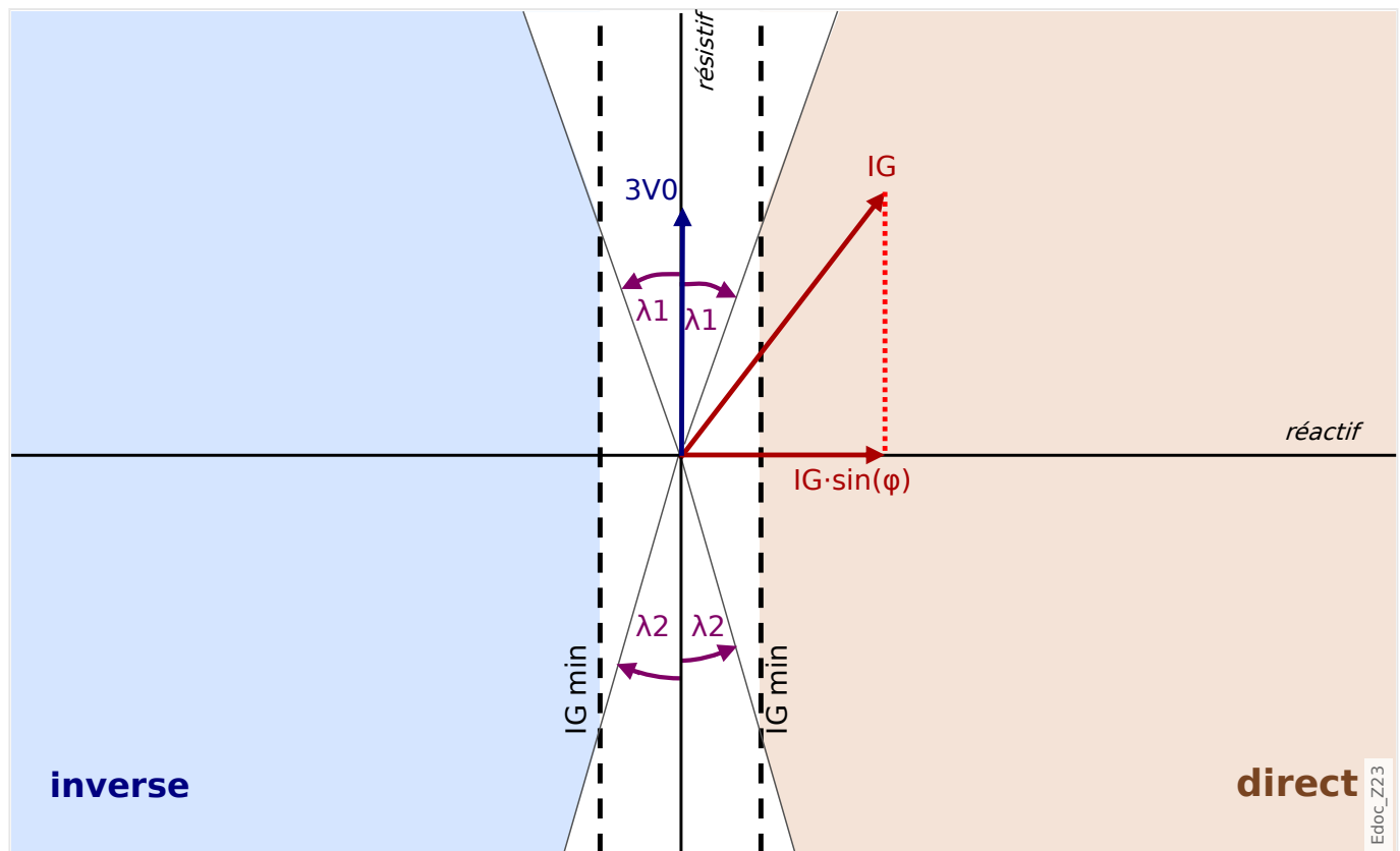
Fig. 68: Principe de détermination de la direction pour la méthode « \sin(\phi) ».
