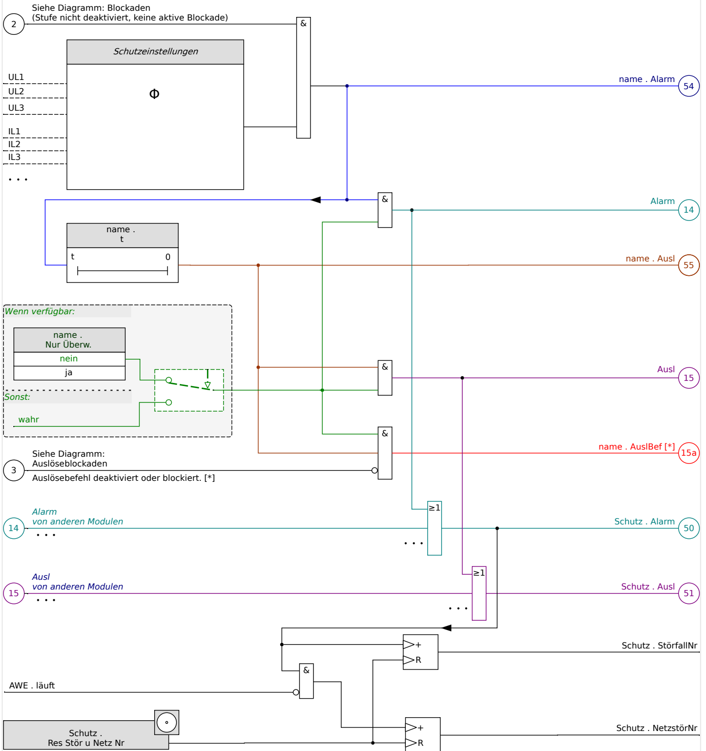
Abb. 62: Grobe Skizze der Funktionalität einer HighPROTEC-Schutzfunktion.
