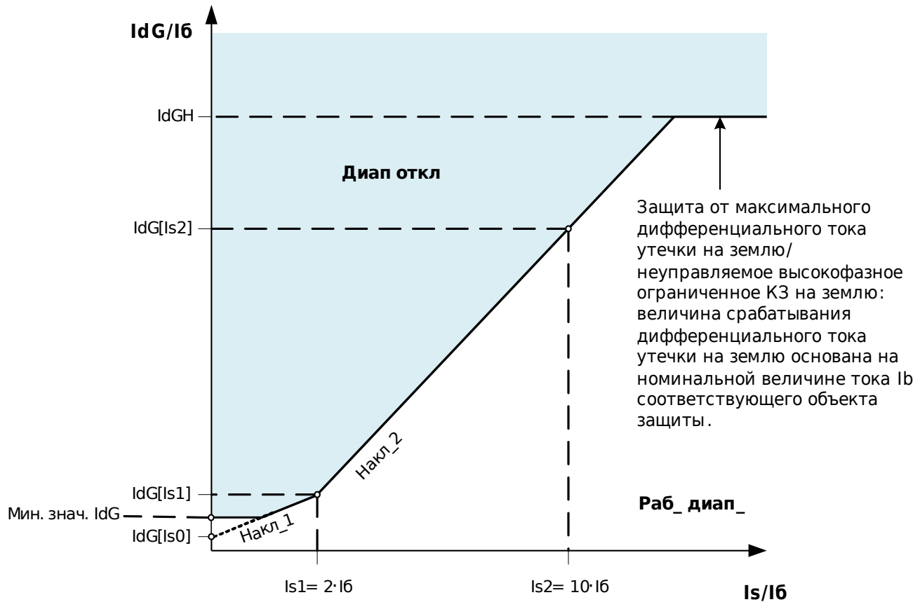
Неуправляемый элемент дифференциальной защиты с высокой установкой IdGH
