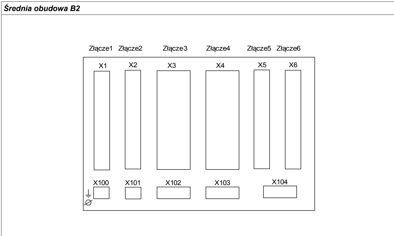
Widok obudowy B2 z tyłu
