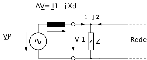
Fig. 112: Circuito equivalente no gerador síncrono em paralelo com a rede.
