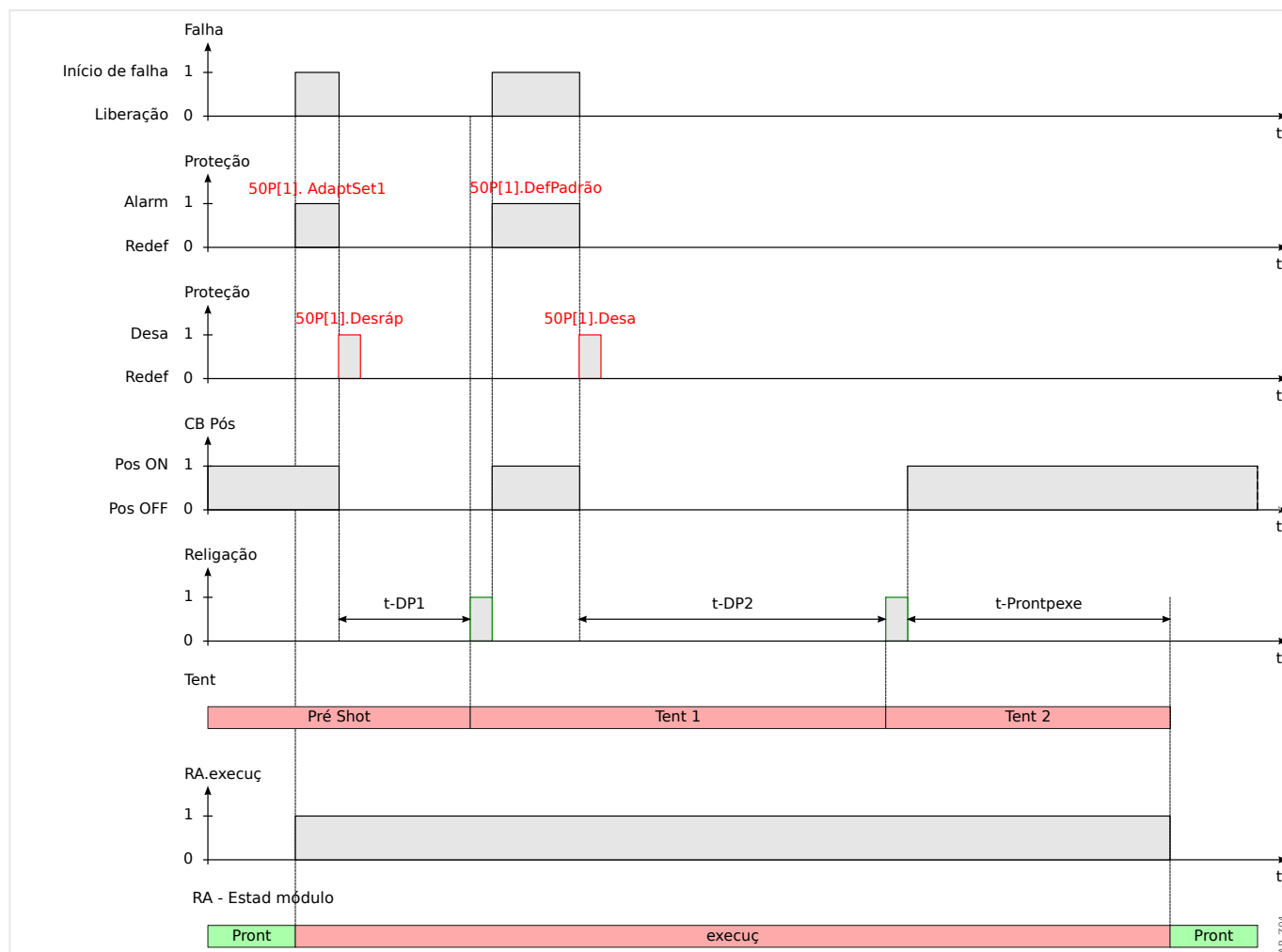
Fig. 103: Diagrama de temporização de religamento automático para esquema de religamento de 2 tentativas bem-sucedidas com aceleração na pré tentativa
