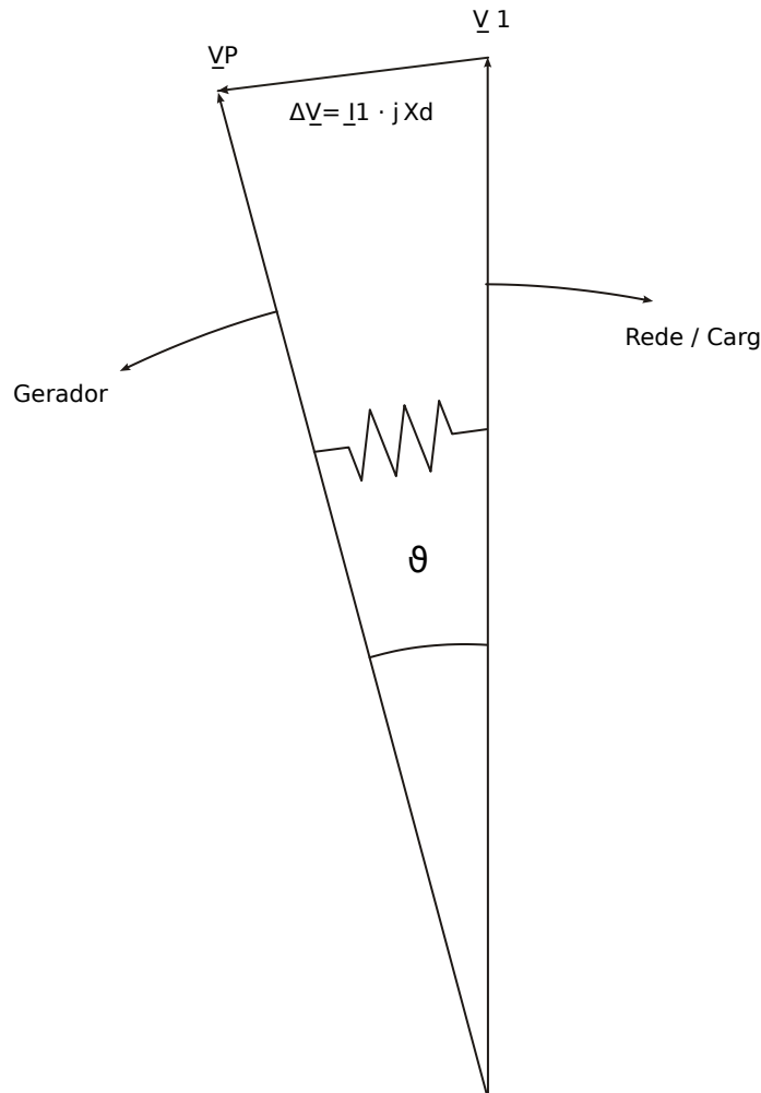
Fig. 113: Vetores de voltagem em operação paralela.
