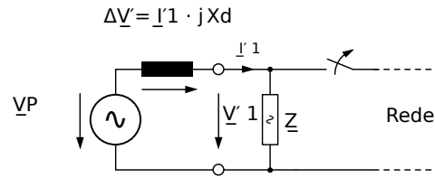
Fig. 114: Circuito equivalente em falha da rede
