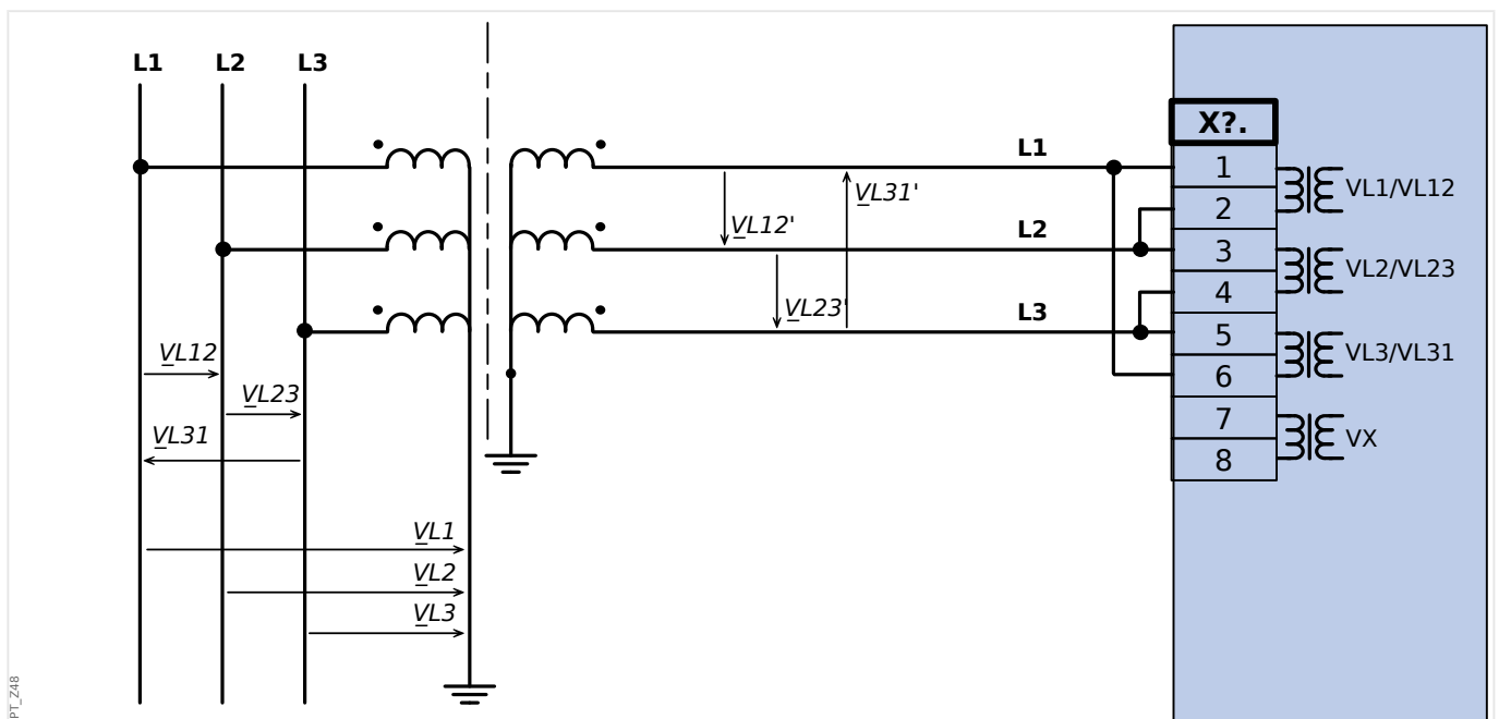
Fig. 32: Medição de tensão trifásica - fiação das entradas de medição: "conexão-delta"
