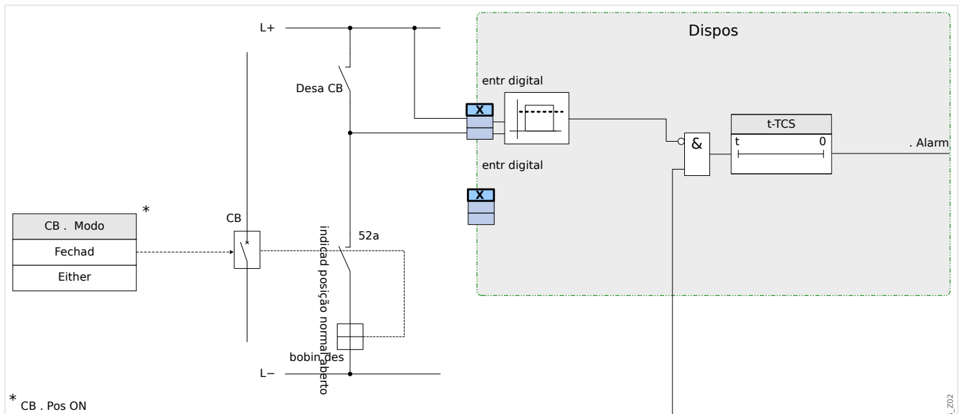
Fig. 140: Exemplo de conexão: Supervisão do circuito de disparo com apenas um contato CB auxiliar »Aux ON« (52a).
