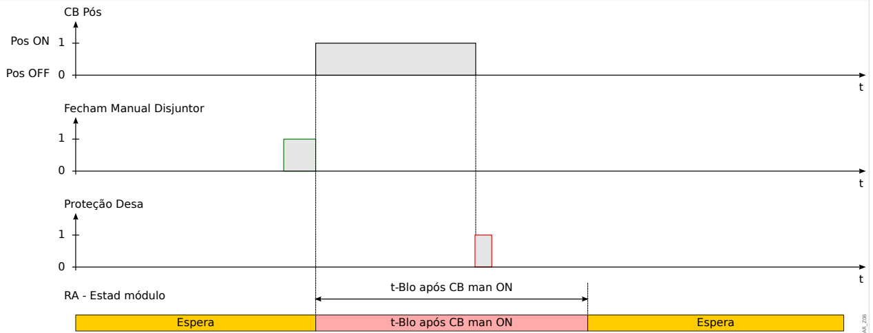
Fig. 105: Disparo de proteção enquanto o tempo de bloqueio de fechamento manual está cronometrando.
