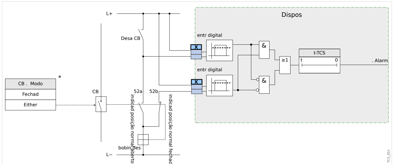
Fig. 139: Exemplo de conexão: Supervisão do circuito de disparo com dois contatos CB auxiliares »Aux ON« (52a) e »Aux OFF« (52b).
