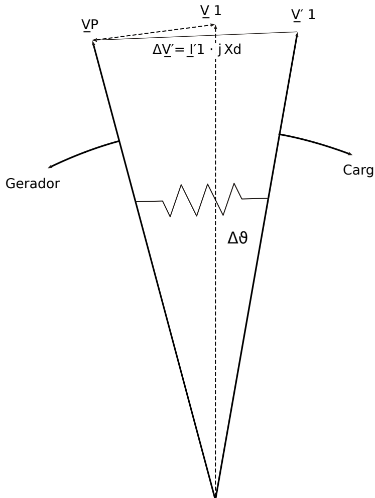
Fig. 115: Vetores de tensão em falha da rede
