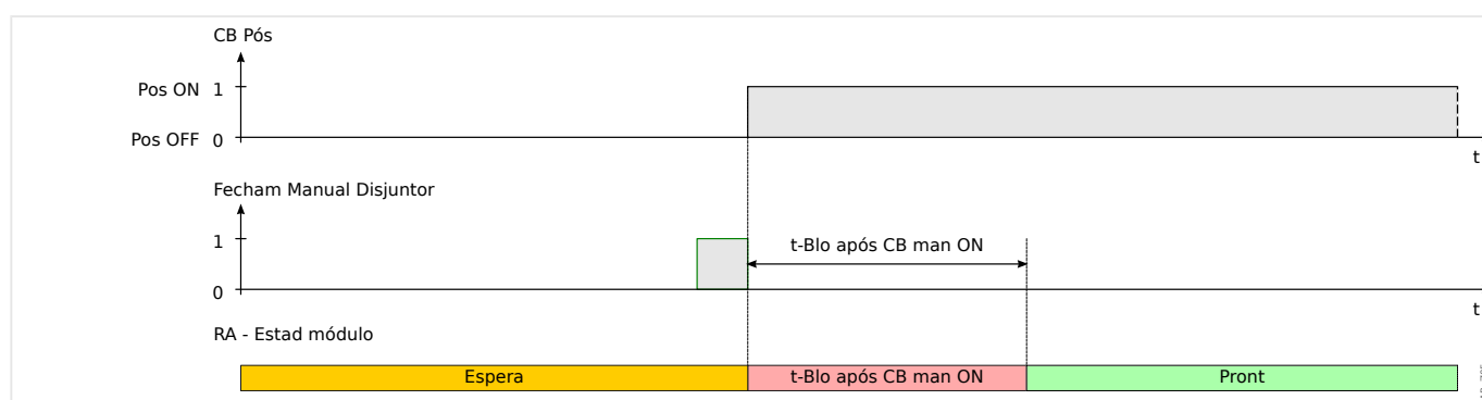
Fig. 104: Estados de religamento automático durante fechamento manual do disjuntor
