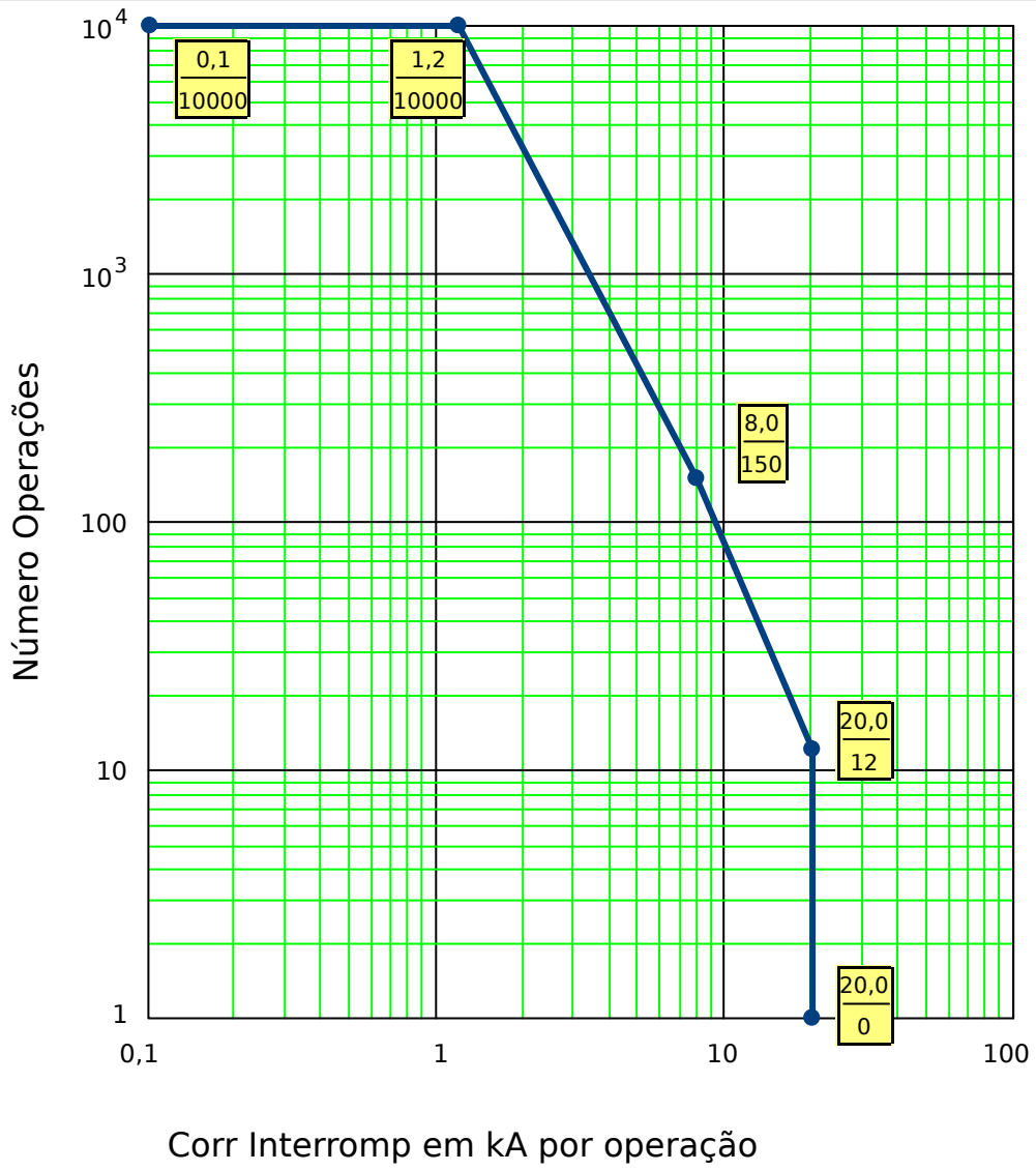
Fig. 148: Curva Manutenção de Disjuntor para Disjuntor normal 25kV
