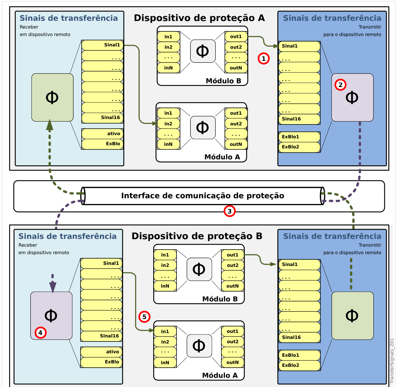
Fig. 84: Princípio da funcionalidade do »Trans-Sinal«.
