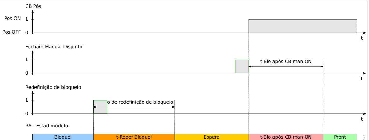
Fig. 106: A lógica de reinicialização de travamento no caso do reinício do travamento vir antes do fechamento manual do disjuntor
