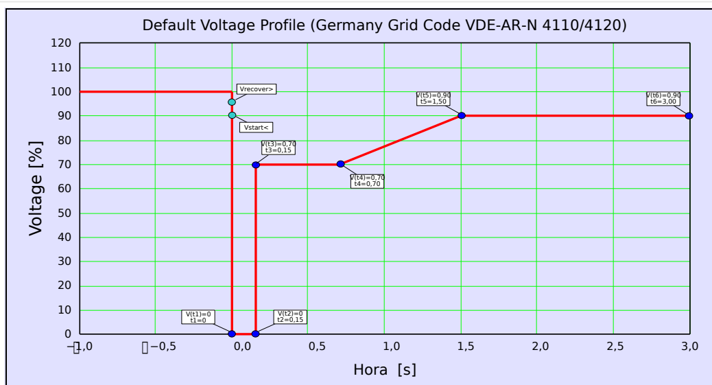
Fig. 136: Perfil padrão do LVRT (Tipo I).
