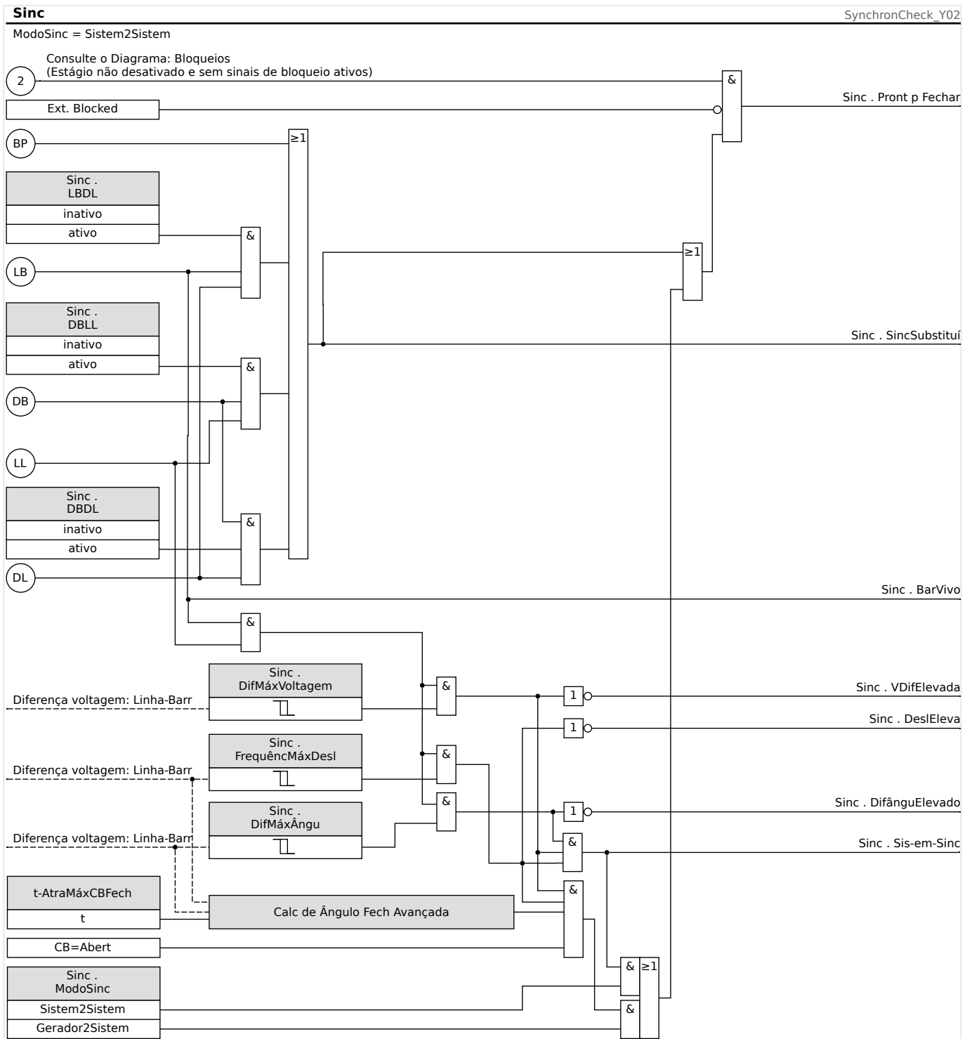
Fig. 121: Funcionalidade do módulo »Sinc«, "Sistem2Sistem".
