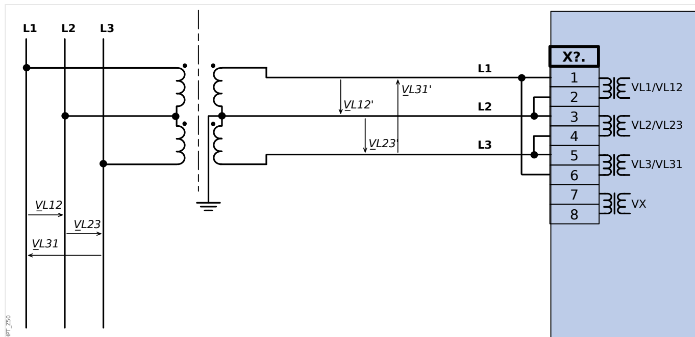
Fig. 34: Medição de voltagem bifásica - fiação das entradas de medição: "Delta Aber"
