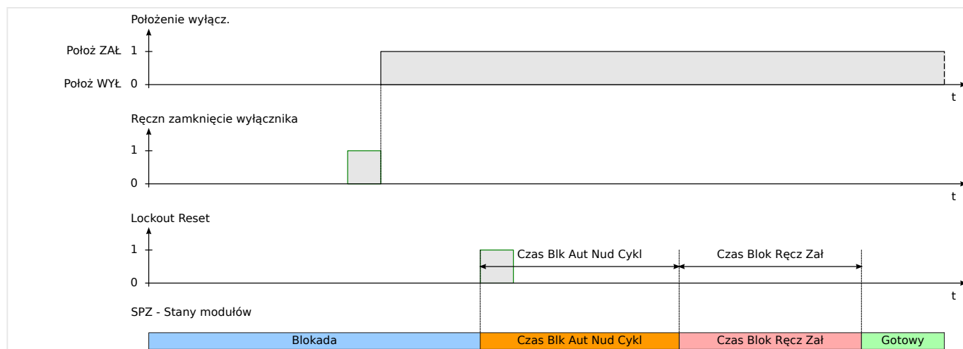
Rys. 107: Logika resetowania blokady automatyki SPZ w przypadku odebrania sygnału resetowania blokady po ręcznym zamknięciu wyłącznika.
