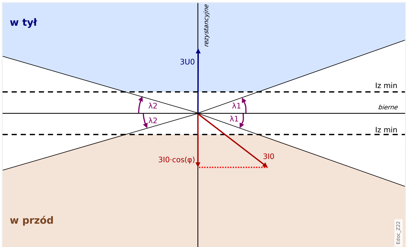
Rys. 68: Zasada określania kierunku metodą „ \cos(\phi) ”.
