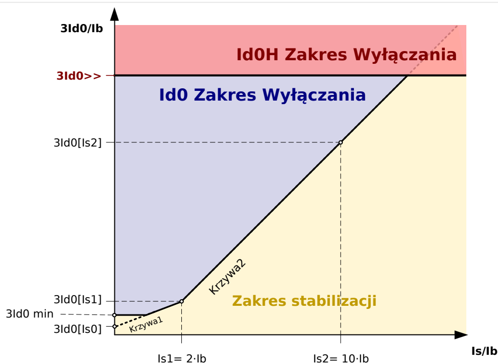
Rys. 81: Wartość pobudzenia „3Id0>>” prądu różnicowego doziemnego w oparciu o prąd znamionowy „lb” obiektu zabezpieczanego.
