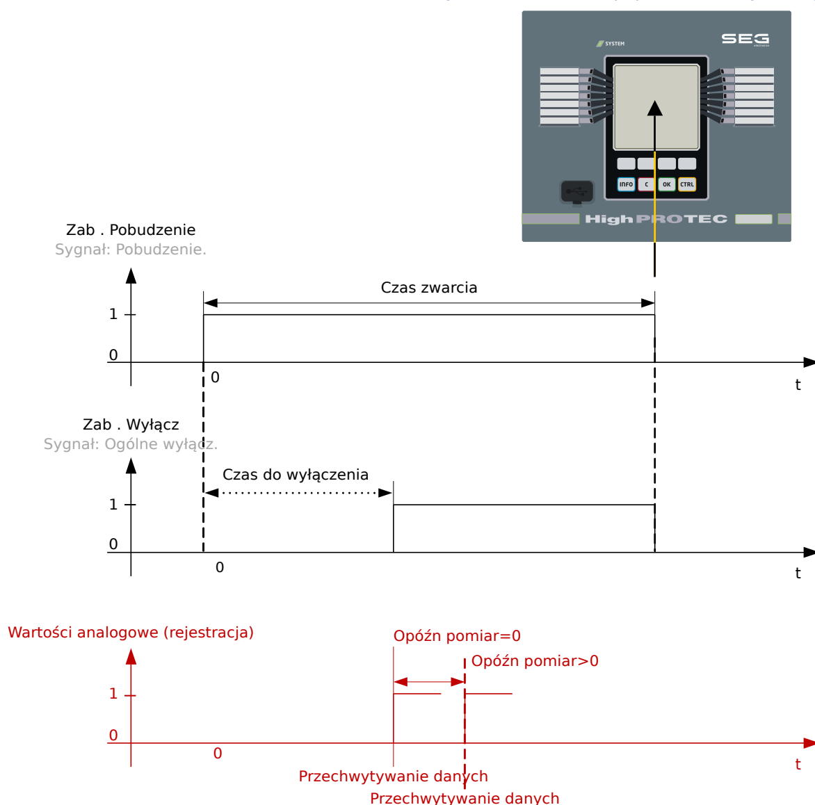
Rys. 153: Rejestrator zwarć: czasy (trwania).
