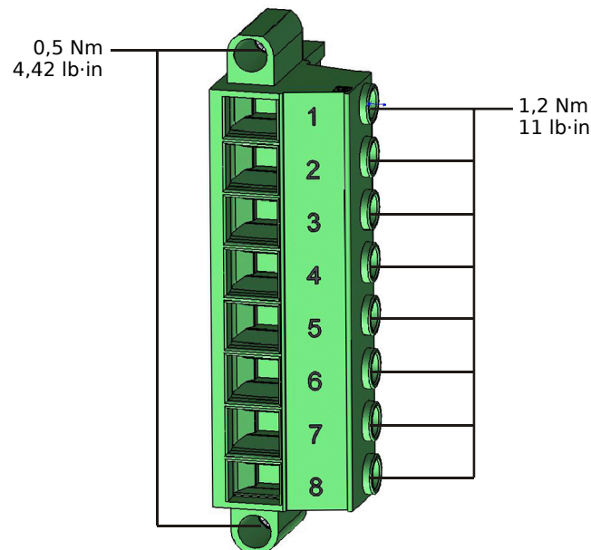
Rys. 162: Zaciski pomiaru napięcia karty pomiarowej „TU” (↳ „3.6.1 TU – wejścia do pomiaru napięcia”).
