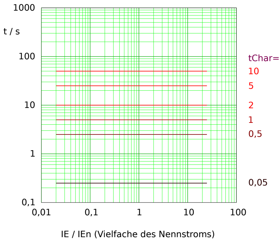
Abb. 106: Auslösekurve „Therm Flat“, wobei nur der Bereich IE > I_{E>} jeweils anwendbar ist. Beispieldiagramm für gemessenen (nicht empfindlichen) Erdstrom.
