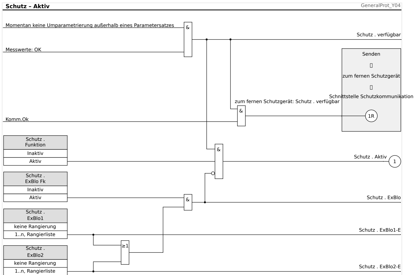
Abb. 63: Verfügbarkeit des Schutzes in Abhängigkeit von der Schutzkommunikation von Leitungsdifferentialschutzgeräten.
