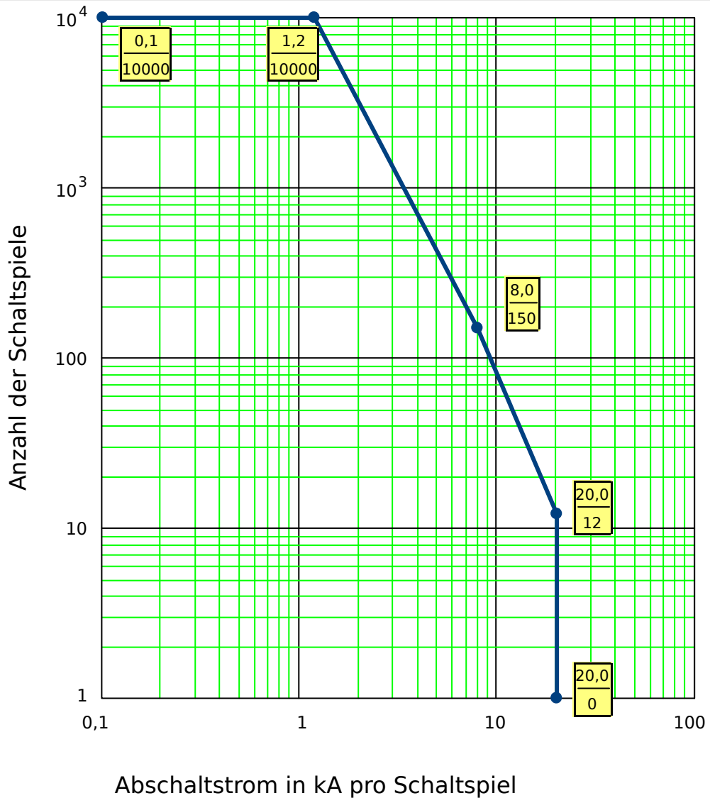
Abb. 166: Wartungskurve für einen typischen 25 kV Leistungsschalter
