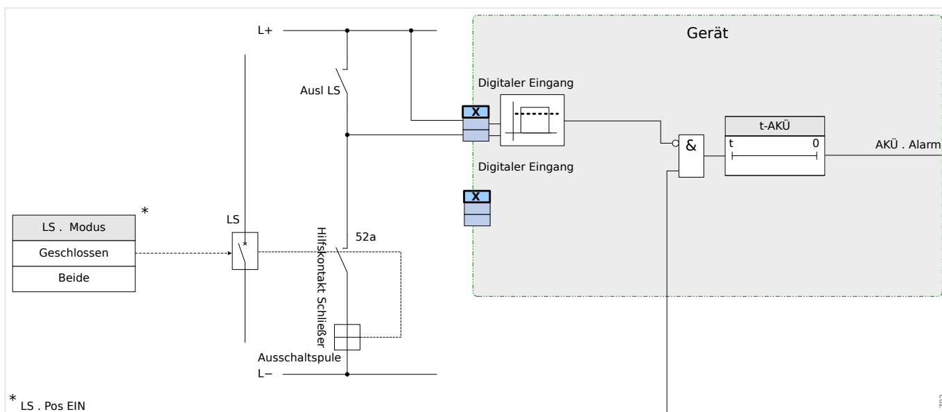
Abb. 158: Anschlussbeispiel: Auslösekreisüberwachung mit einem Hilfskontakt »Hiko EIN« (52a).
