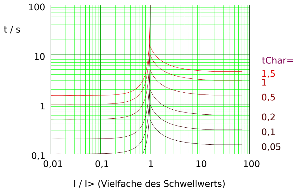
Abb. 89: RINV: Rückfallverzögerung (linke Hälfte, I < I_{>} ) und Auslöseverzögerung (rechte Hälfte, I > I_{>} ), Beispieldiagramm für I_{max} = 20 \cdot I_{>} .
