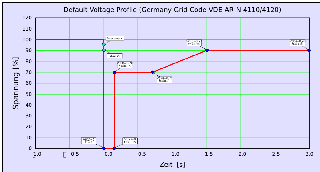
Abb. 154: LVRT-Werkseinstellung (Typ I).
