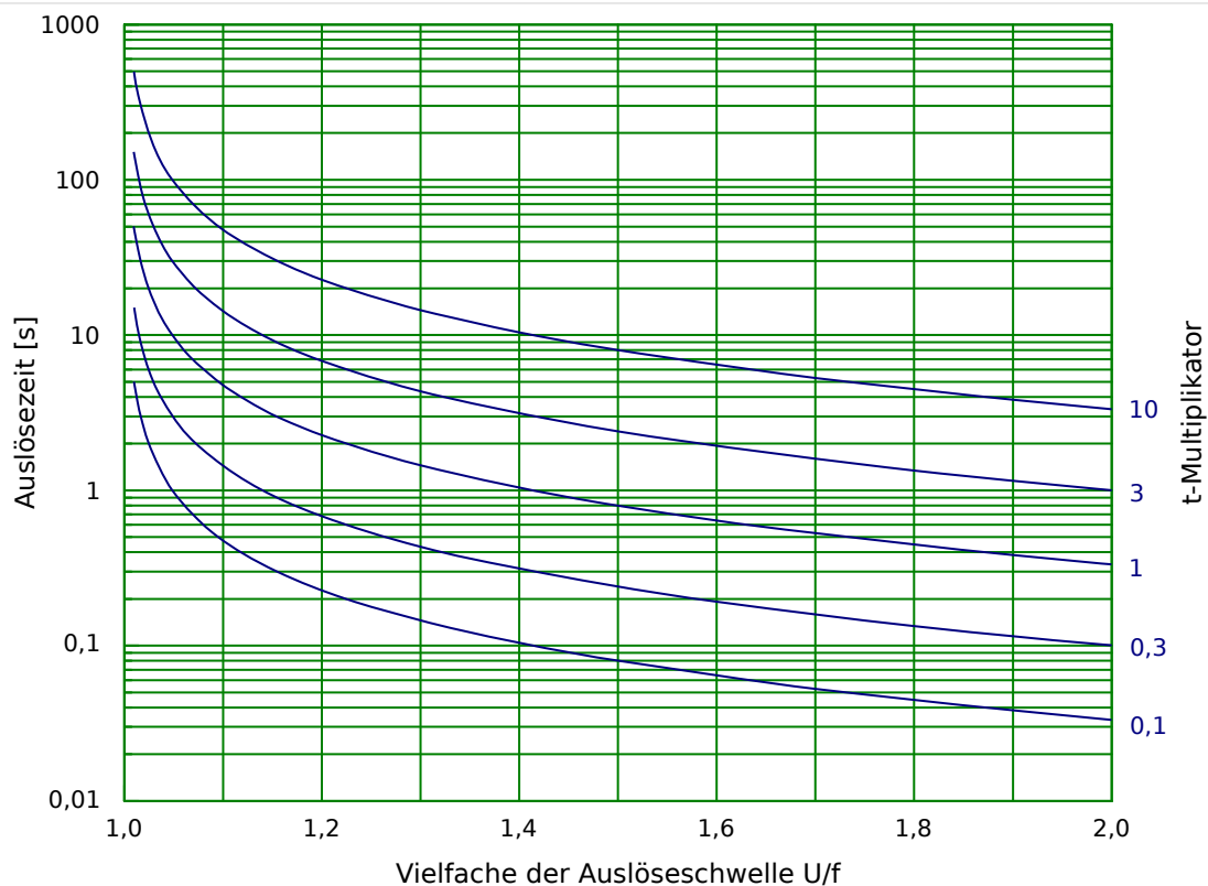
Abb. 113: Charakteristik/Kennlinie: INV A
