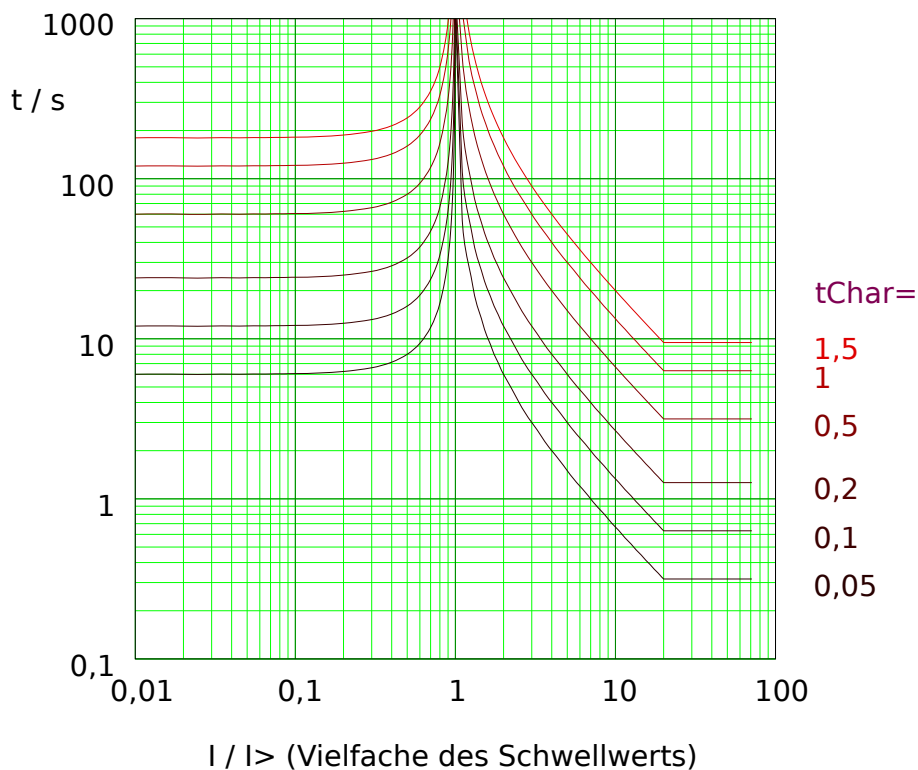
Abb. 88: LINV: Rückfallverzögerung (linke Hälfte, I < I_N ) und Auslöseverzögerung (rechte Hälfte, I > I_N ), Beispieldiagramm für I_{max} = 20 \cdot I_N .
