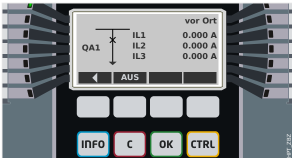
Abb. 161: Beispiel einer Steuer-Seite mit geschlossenem „Leistungsschalter“.
