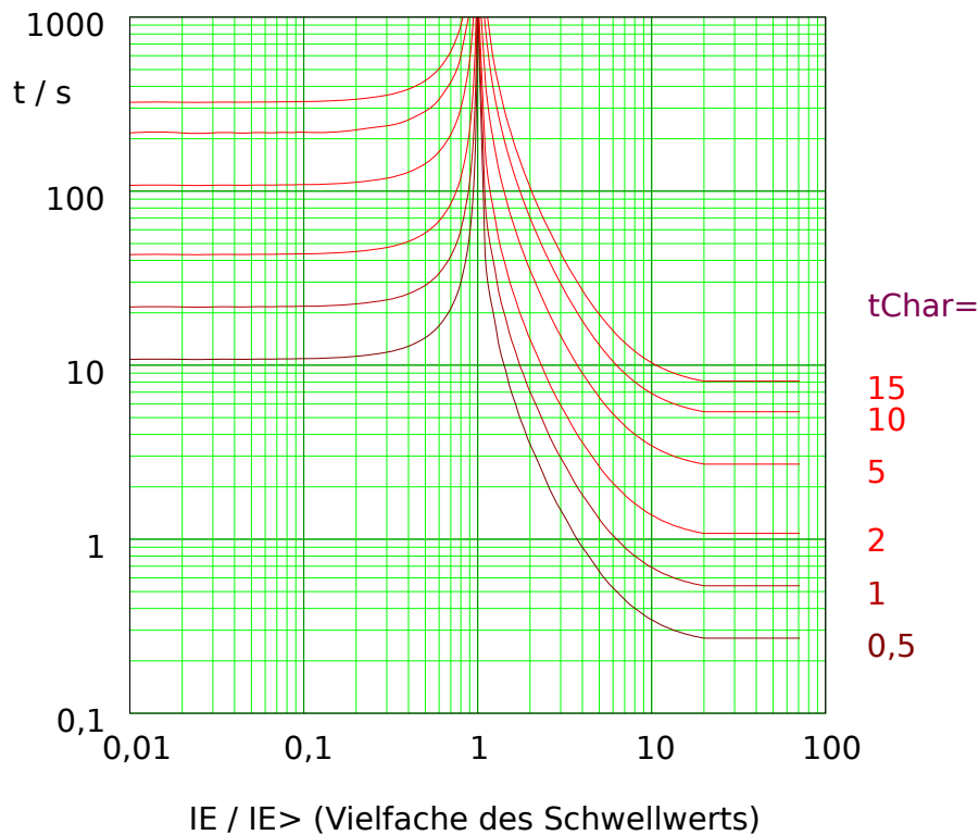
Abb. 103: VINV: Rückfallverzögerung (linke Hälfte, IE < I_{E>} ) und Auslöseverzögerung (rechte Hälfte, IE > I_{E>} ), Beispieldiagramm für I_{max} = 20 \cdot I_{E>} .
