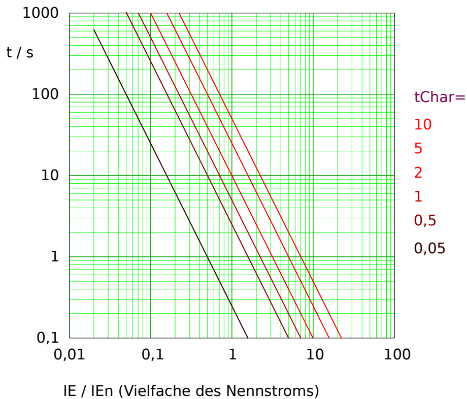
Abb. 108: Auslösekurve „I2T“, wobei nur der Bereich IE > I_{E>} jeweils anwendbar ist. Beispieldiagramm für gemessenen (nicht empfindlichen) Erdstrom.
