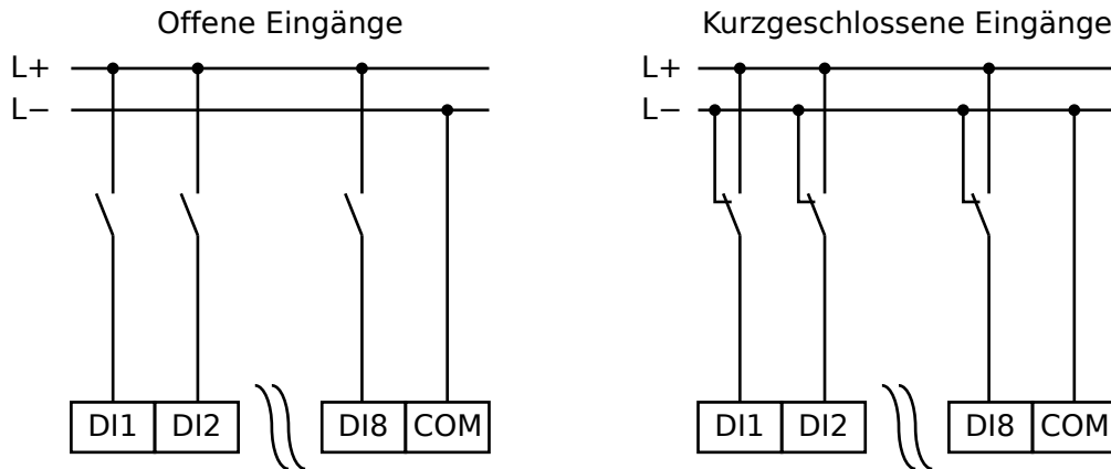
Abb. 183: Sicherer Zustand der digitalen Eingänge
