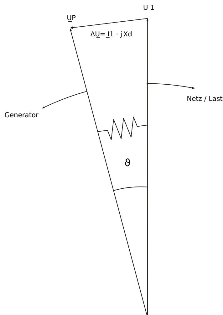
Abb. 130: Polradwinkel bei konstanter Belastung des Generators.
