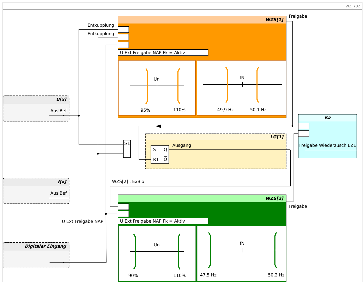
Abb. 142: Applikationsbeispiel für ein Zuschalten in Abhängigkeit von einer vorherigen Schutzauslösung.
