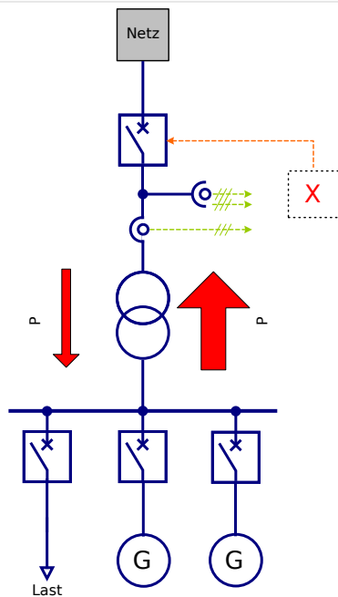
Abb. 147: Zentraler Einsatz in Teilnetzen mit überwiegender Rückspeisung.
