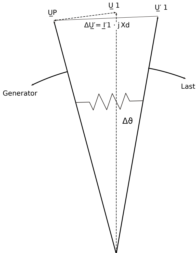
Abb. 132: Änderung des Polradwinkels bei plötzlicher Belastung des Generators.
