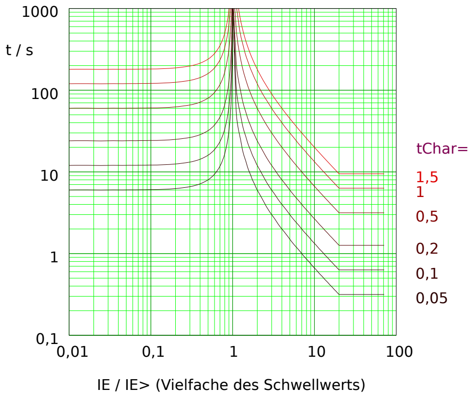
Abb. 100: LINV: Rückfallverzögerung (linke Hälfte, IE < I_{E>} ) und Auslöseverzögerung (rechte Hälfte, IE > I_{E>} ), Beispieldiagramm für I_{max} = 20 \cdot I_{E>} .
