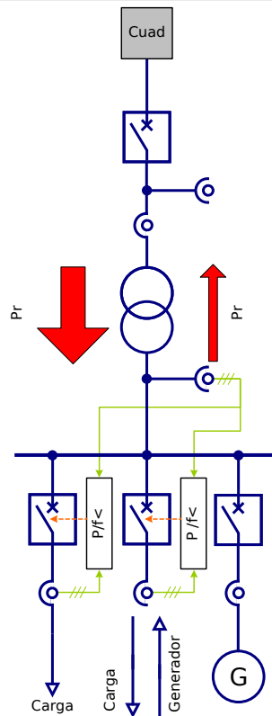
Fig. 118: Reducción de carga descentralizada por subfrecuencia en redes eléctricas con alimentación temporal.
