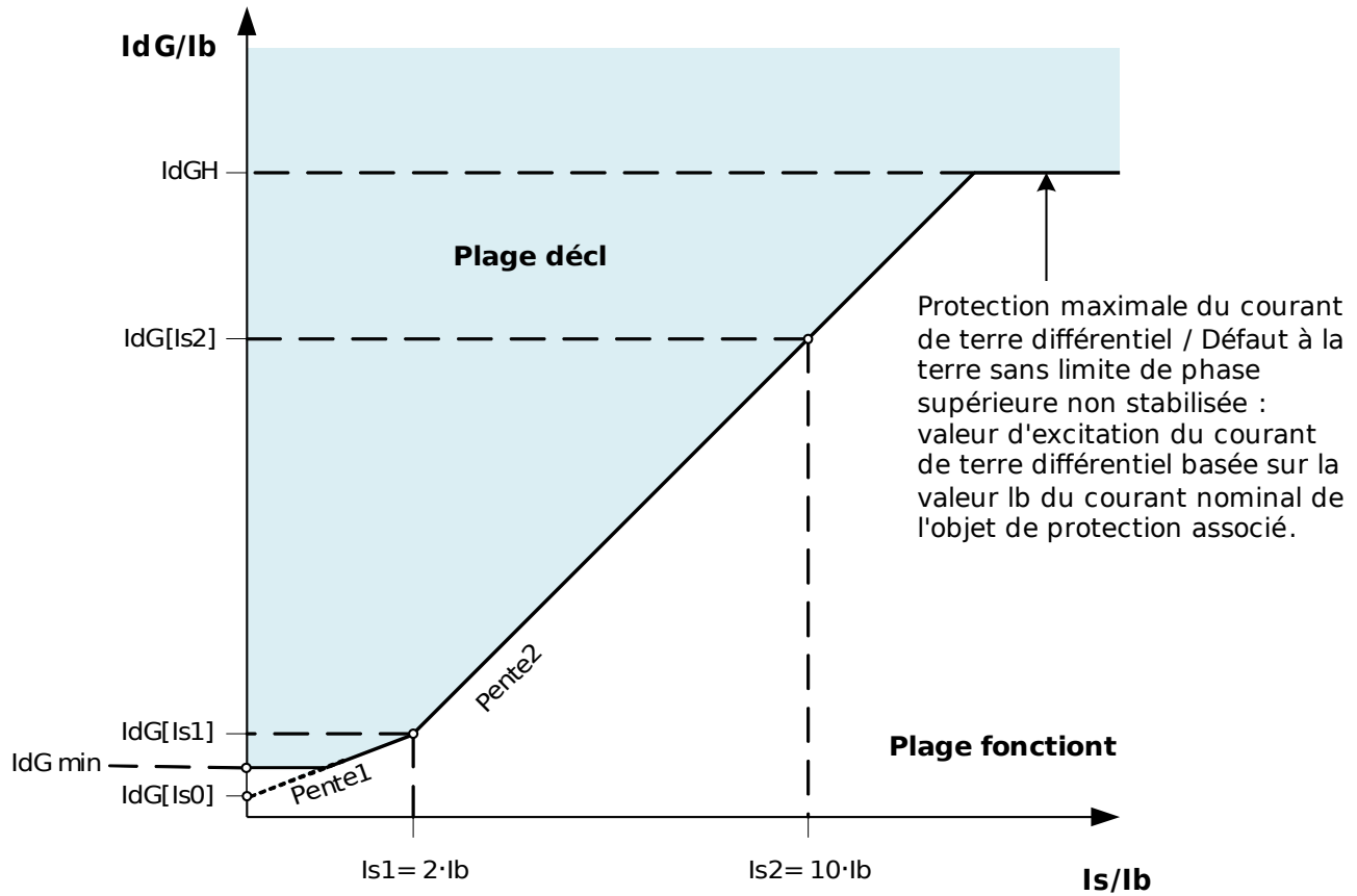
Élément de protection différentielle non stabilisé de niveau supérieur IdGH
