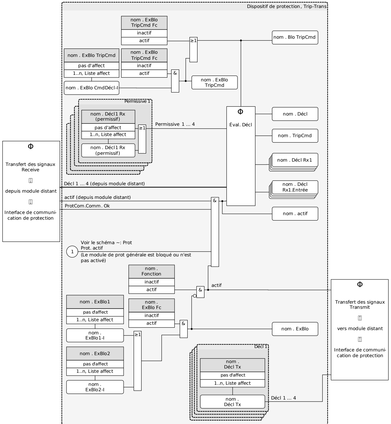
Fonctionnalité du module Trip-Trans La sous-routine « Éval. Décl » est détaillée dans le schéma suivant.
