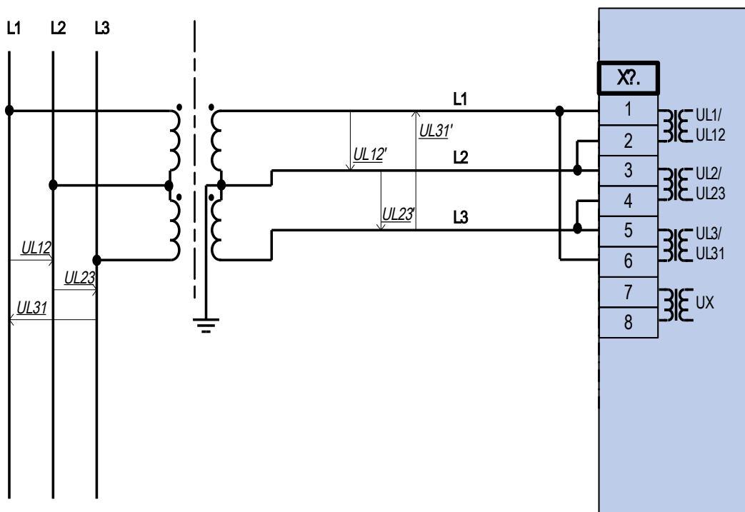
Zwei Spannungswandler mit Geräteanschluss in V-Schaltung
