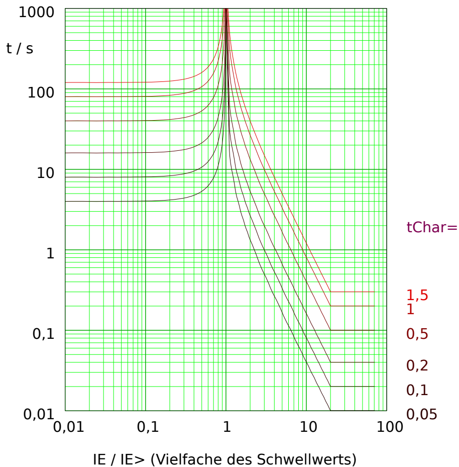
Abb. 103: EINV: Rückfallverzögerung (linke Hälfte, IE < I_{E>} ) und Auslöseverzögerung (rechte Hälfte, IE > I_{E>} ), Beispieldiagramm für I_{max} = 20 \cdot I_{E>} .
