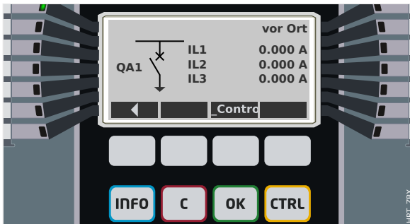
Abb. 166: Beispiel einer Steuer-Seite mit geöffnetem „Leistungsschalter“.
