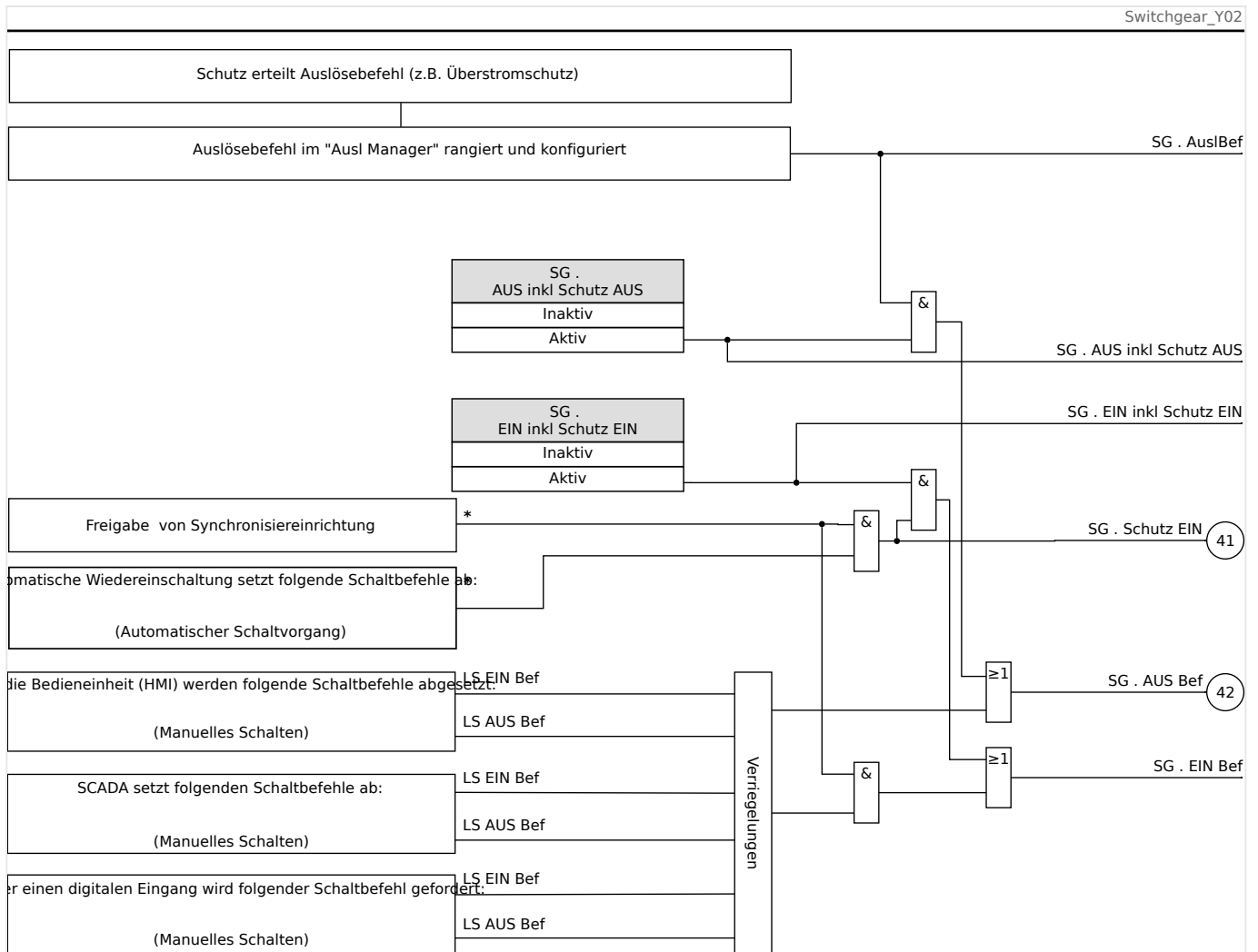
Abb. 167: Verriegelungen. (Für die mit „*“ markierten Teile gilt: Verfügbarkeit hängt von der bestellten Gerätevariante ab.)
