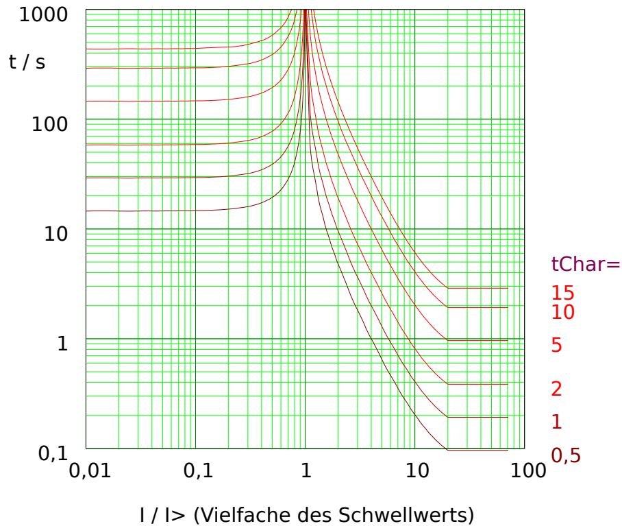
Abb. 96: EINV: Rückfallverzögerung (linke Hälfte, I < I_{>} ) und Auslöseverzögerung (rechte Hälfte, I > I_{>} ), Beispieldiagramm für I_{max} = 20 \cdot I_{>} .
