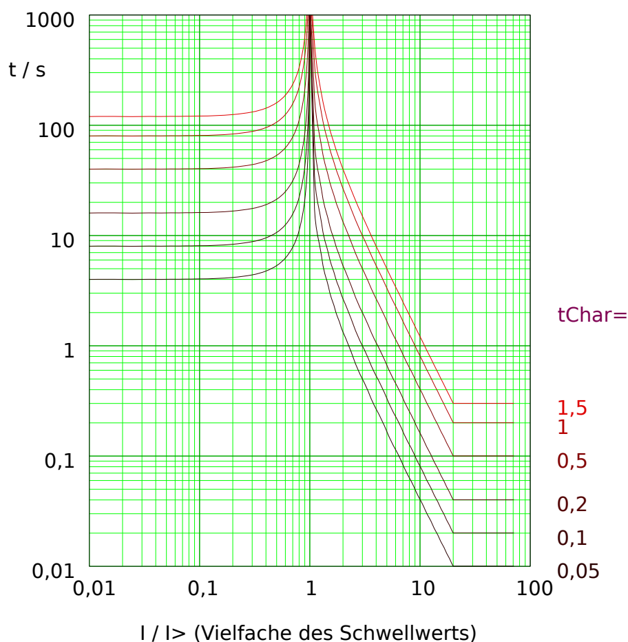
Abb. 91: EINV: Rückfallverzögerung (linke Hälfte, I < I_{>} ) und Auslöseverzögerung (rechte Hälfte, I > I_{>} ), Beispieldiagramm für I_{max} = 20 \cdot I_{>} .
