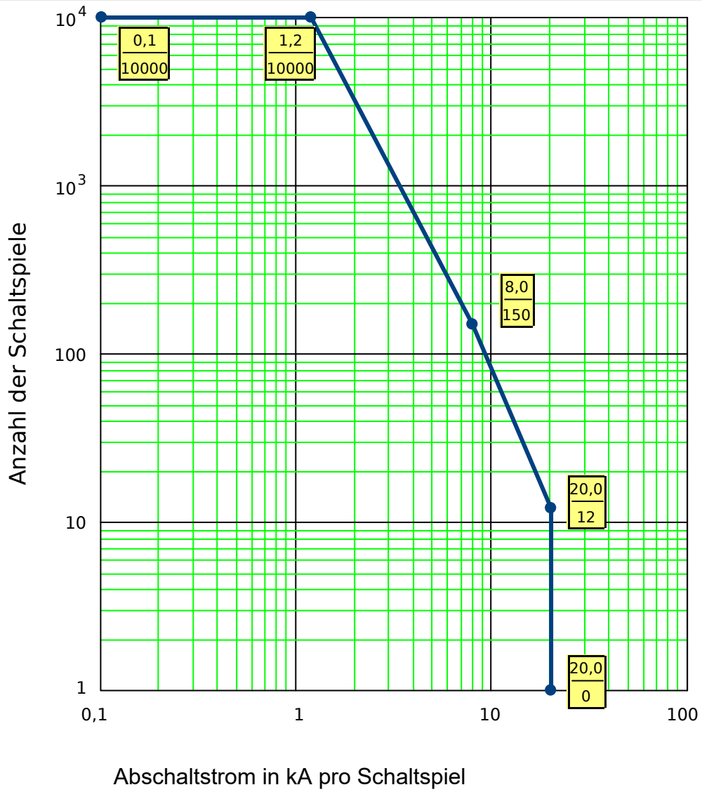
Abb. 169: Wartungskurve für einen typischen 25 kV Leistungsschalter
