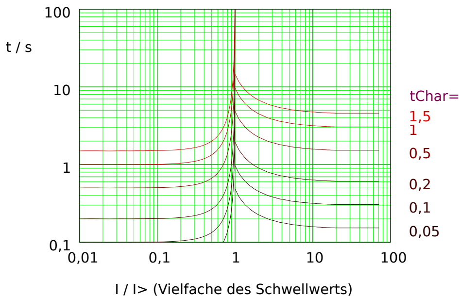
Abb. 93: RINV: Rückfallverzögerung (linke Hälfte, I < I_{>} ) und Auslöseverzögerung (rechte Hälfte, I > I_{>} ), Beispieldiagramm für I_{max} = 20 \cdot I_{>} .
