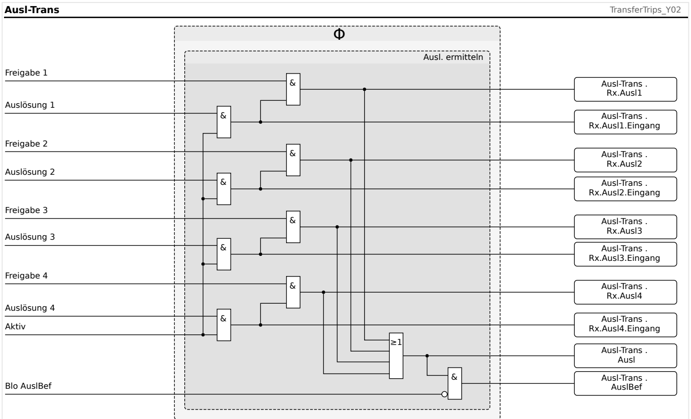
Abb. 87: Funktionalität des Moduls »Ausl-Trans« (Teil 2).
