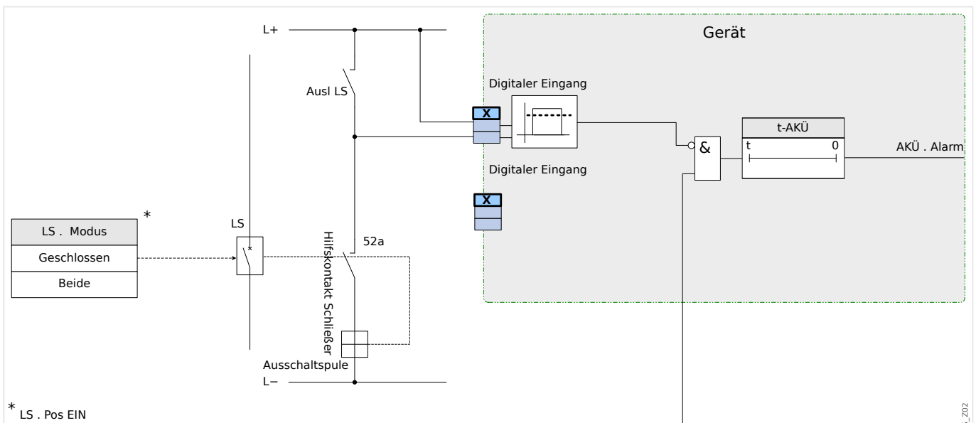
Abb. 160: Anschlussbeispiel: Auslösekreisüberwachung mit einem Hilfskontakt »Hiko EIN« (52a).
