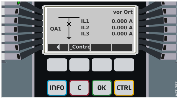
Abb. 164: Beispiel einer Steuer-Seite mit geschlossenem „Leistungsschalter“.
