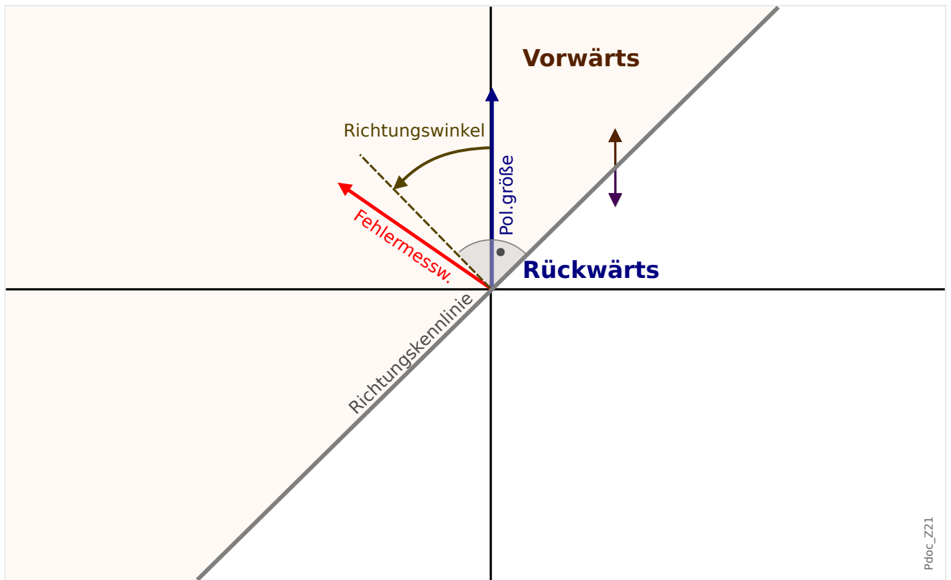
Abb. 66: Prinzip der Richtungserkennung von Phasenfehlern.
