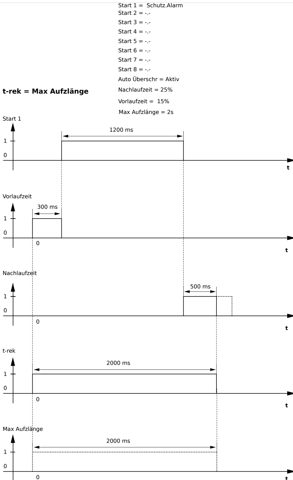
Abb. 172: Beispiel I Störschreiber-Ablaufdiagramm
