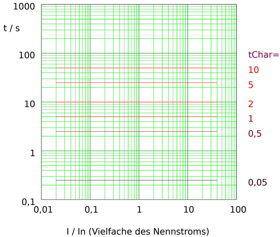
Abb. 97: Auslösekurve „Therm Flat“, wobei nur der Bereich I > I_{>} jeweils anwendbar ist.
