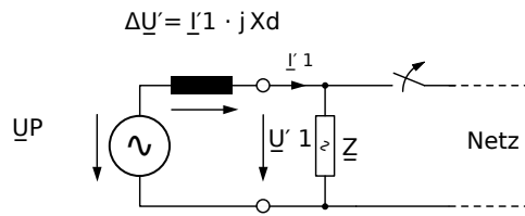
Abb. 135: Ersatzschaltbild Synchrongenerator bei Netzausfall.
