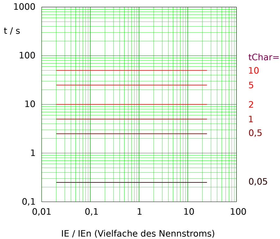
Abb. 110: Auslösekurve „Therm Flat“, wobei nur der Bereich IE > I_{E>} jeweils anwendbar ist. Beispieldiagramm für gemessenen (nicht empfindlichen) Erdstrom.
