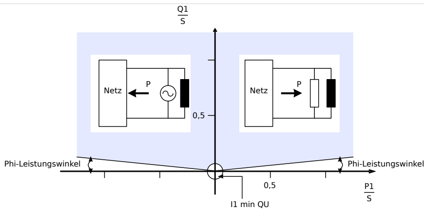
Abb. 145: Variante 1: Leistungswinkelüberwachung.
