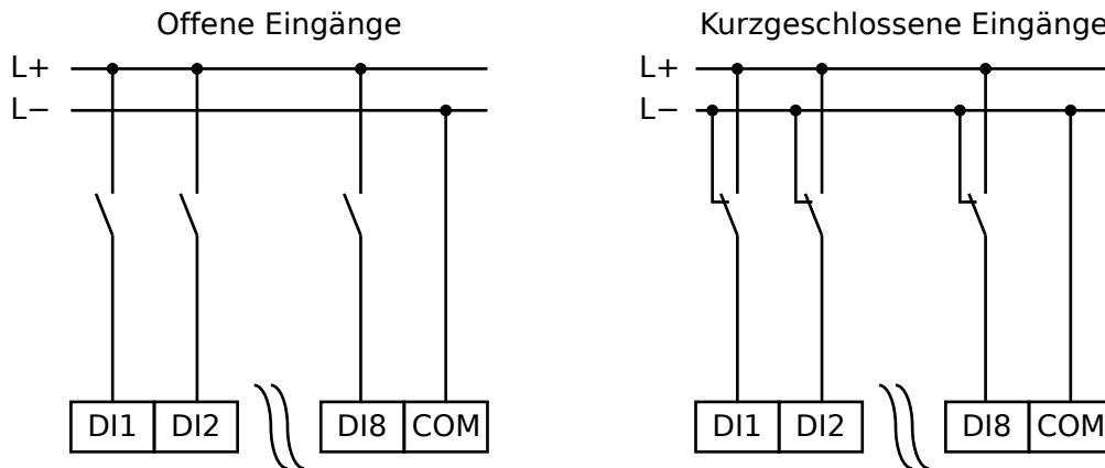
Abb. 186: Sicherer Zustand der digitalen Eingänge
