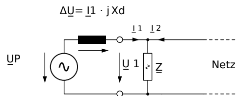
Abb. 133: Ersatzschaltbild netzparalleler Synchrongenerator
