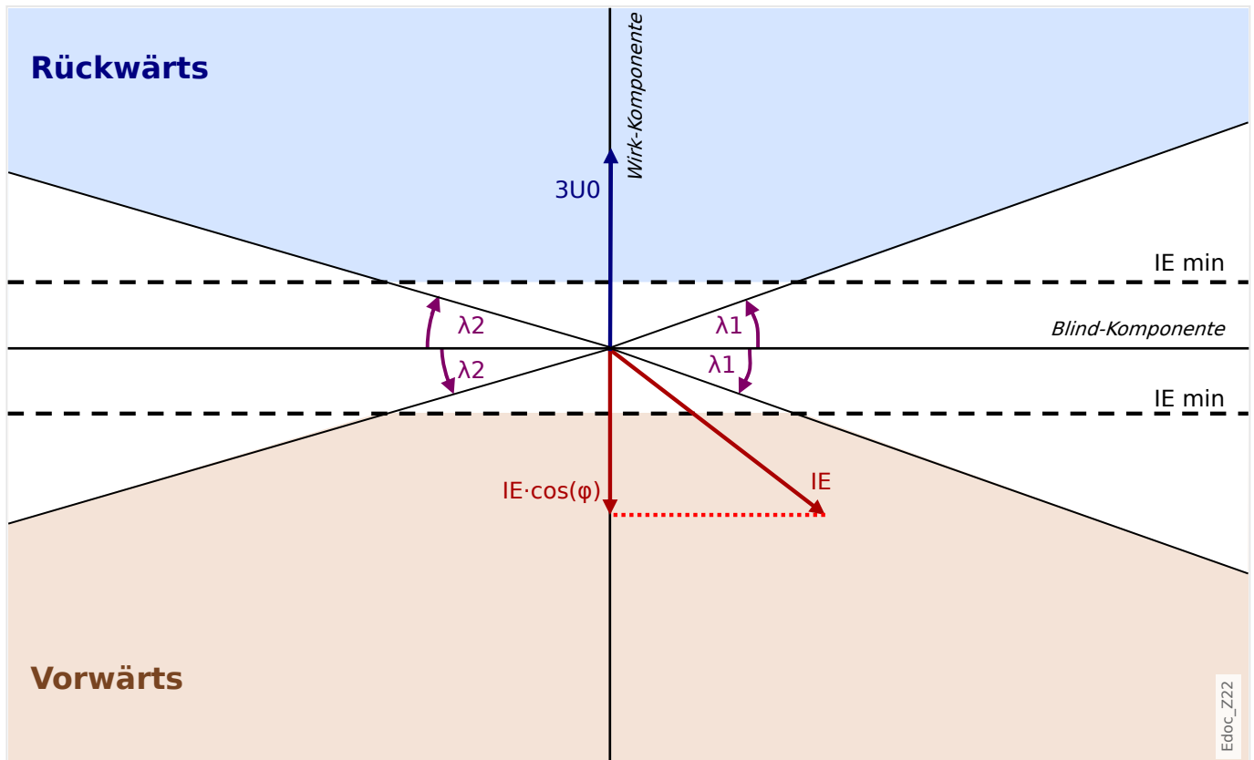
Abb. 69: Richtungserkennung nach der Methode „ \cos(\phi) “.
