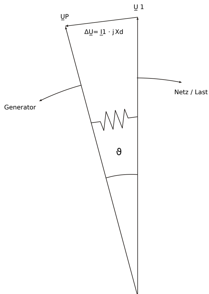
Abb. 134: Polradwinkel bei konstanter Belastung des Generators.
