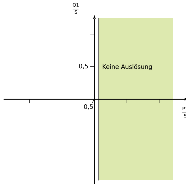
Abb. 151: Variante 2 (Reine Wirkleistungsschwellwertüberwachung): »UFLA Methode« = „Reine Wirkleistungsschwelle“.
