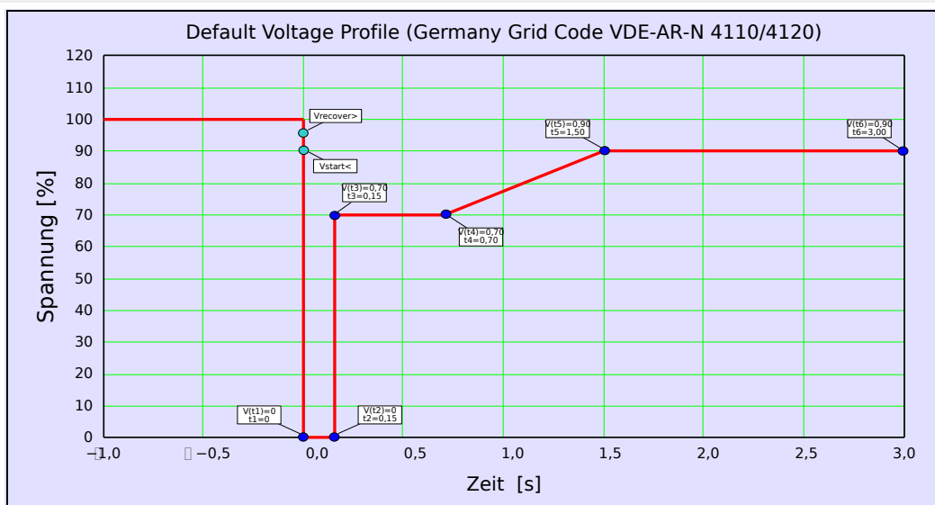
Abb. 155: LVRT-Werkseinstellung (Typ I).
