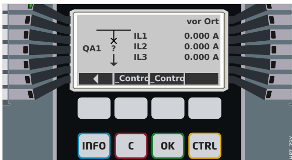
Abb. 165: Beispiel einer Steuer-Seite mit „Leistungsschalter“ in Störstellung (bzw. unplausiblem Zustand).
