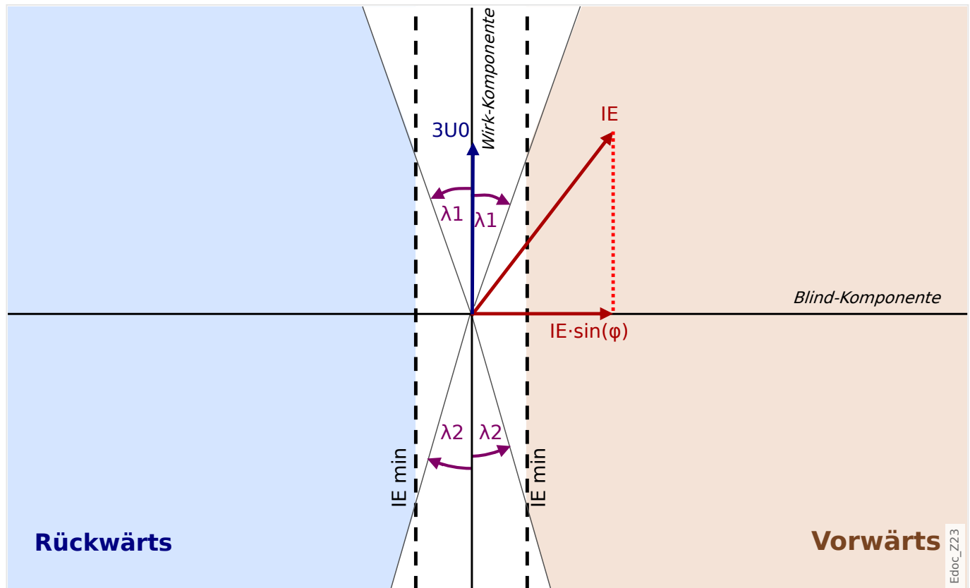
Abb. 70: Richtungserkennung nach der Methode „ \sin(\phi) “.
