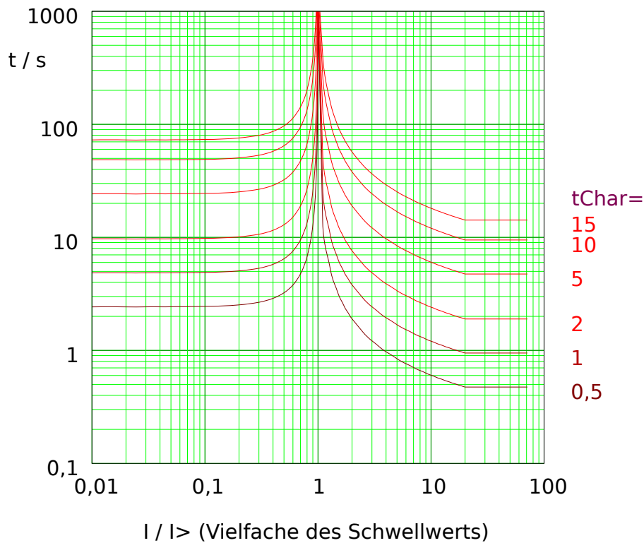
Abb. 94: MINV: Rückfallverzögerung (linke Hälfte, I < I_{>} ) und Auslöseverzögerung (rechte Hälfte, I > I_{>} ), Beispieldiagramm für I_{max} = 20 \cdot I_{>} .
