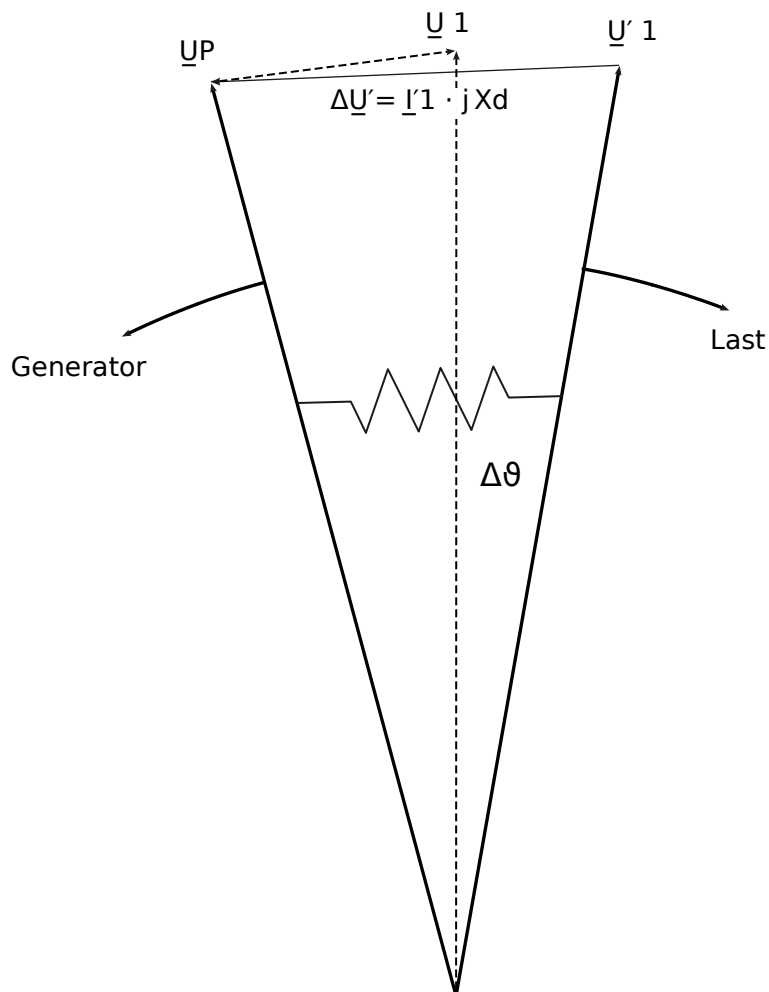
Abb. 136: Änderung des Polradwinkels bei plötzlicher Belastung des Generators.
