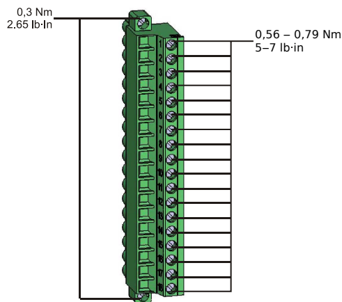
Рис. 163: Измерительные контакты плат измерения напряжения «TU-OR5» и «TU-DI8».
