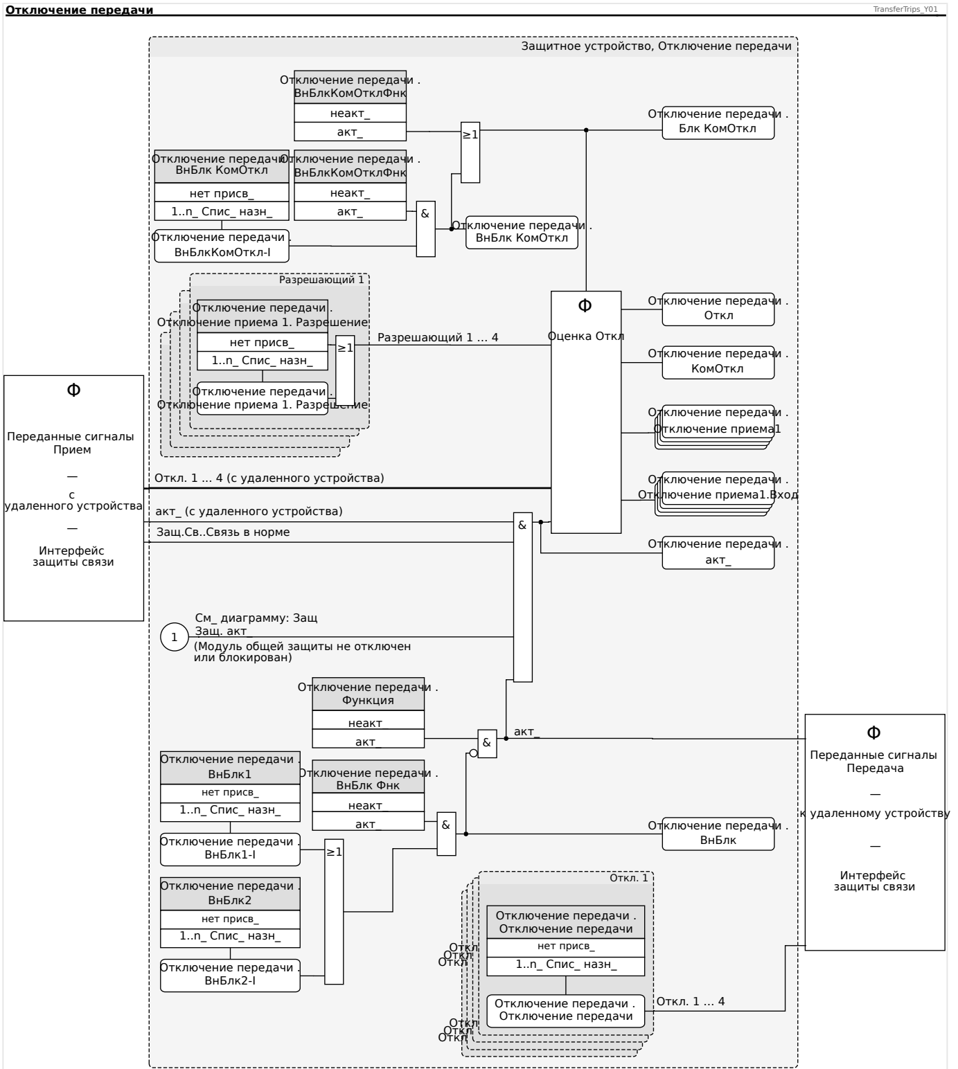
Рис. 82: Принцип работы модуля «Отключение передачи». Подпрограмма пробного отключения в подробностях представлена на приведенной далее схеме.
