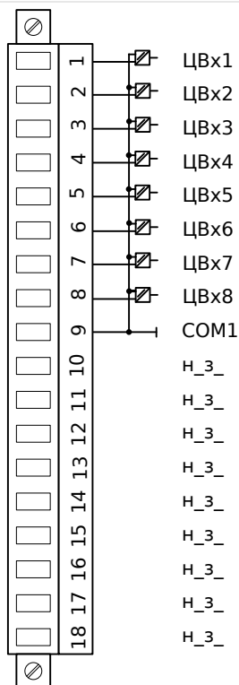
Рис. 40: Электромеханическая адресация.
