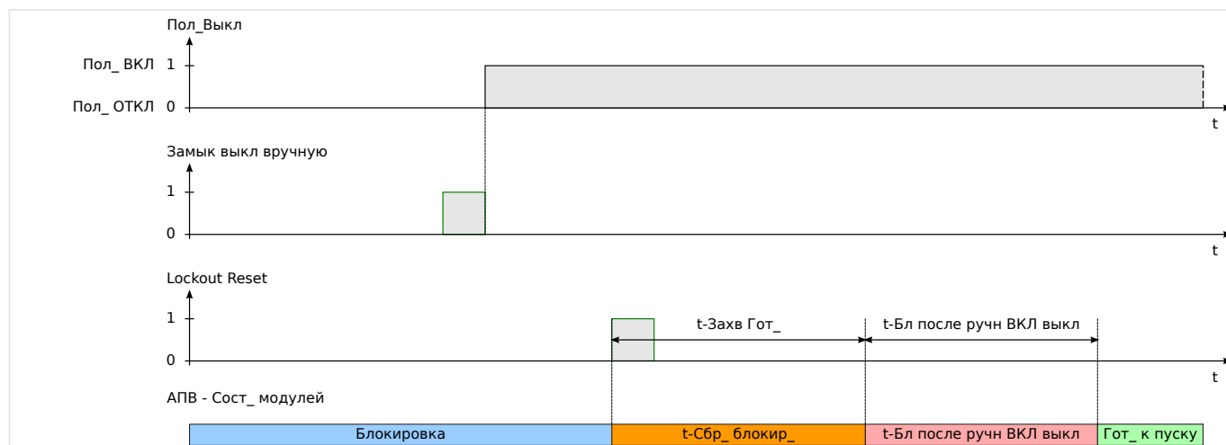
Рис. 107: Логика сброса блокировки АПВ при получении команды сброса блокировки после замыкания выключателя вручную.
