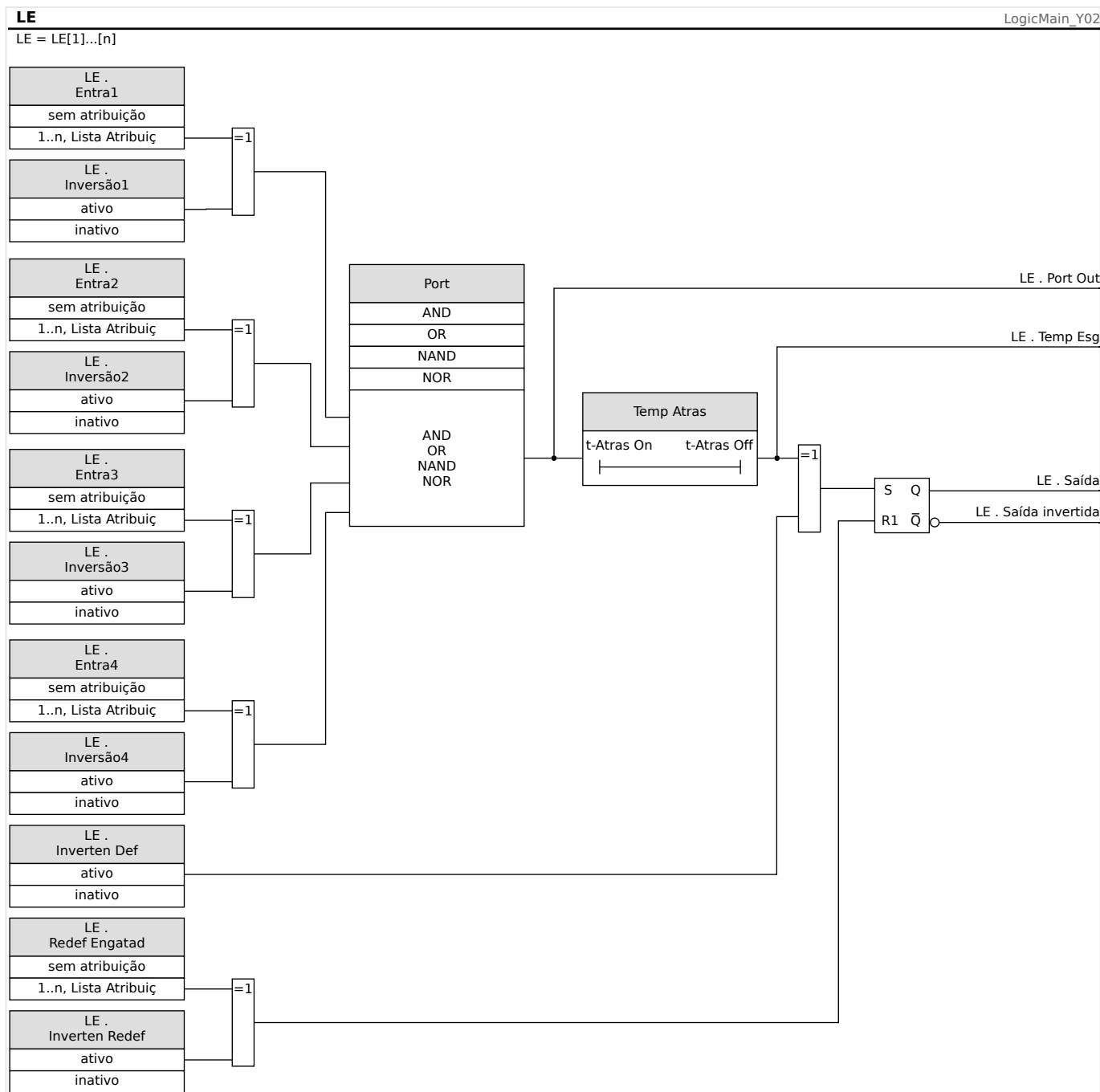
Fig. 155: Visão Geral Detalhada - Diagrama Lógico Geral.
