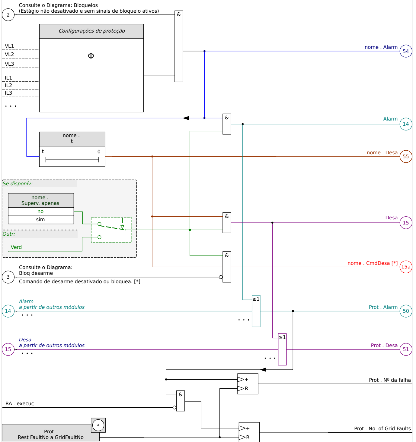
Fig. 63: Esboço rápido da funcionalidade de qualquer HighPROTEC elemento de proteção.
