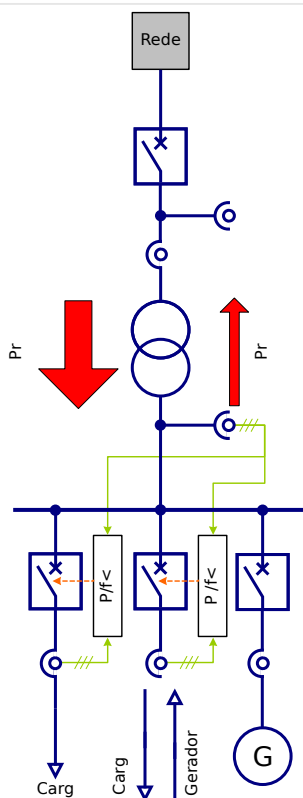
Fig. 128: Eliminação de carga de subfrequência descentralizada em redes com fornecimento temporário de energia.
