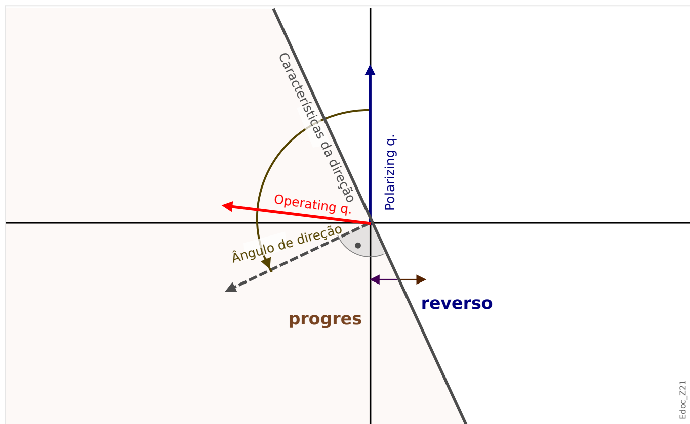
Fig. 66: Princípio de determinação da direção para todos os métodos, exceto “ \cos(\phi) ”, “ \sin(\phi) ”.
