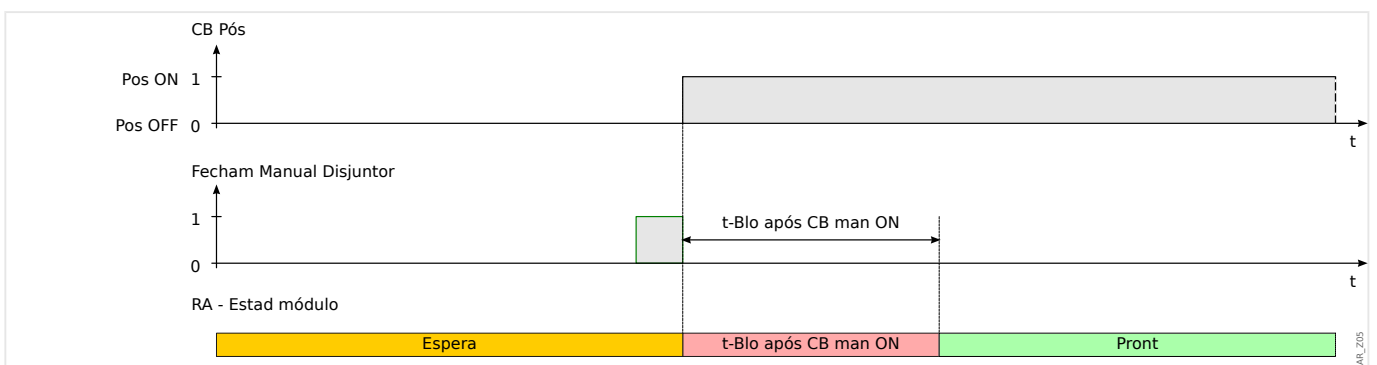
Fig. 104: Estados de religamento automático durante fechamento manual do disjuntor
