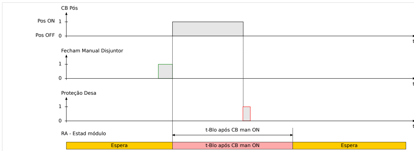
Fig. 105: Disparo de proteção enquanto o tempo de bloqueio de fechamento manual está cronometrando.
