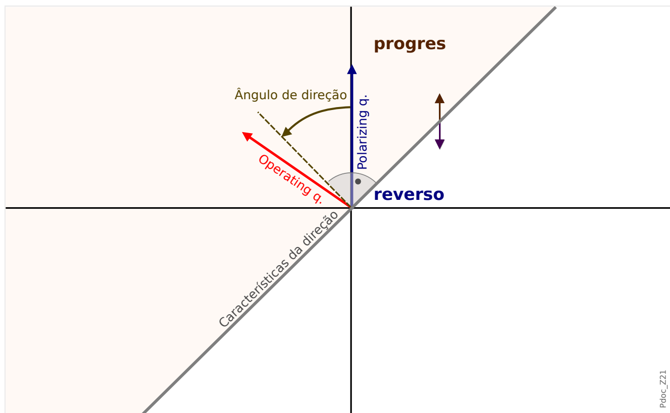
Fig. 64: Princípio de detecção da direção de falhas de fase
