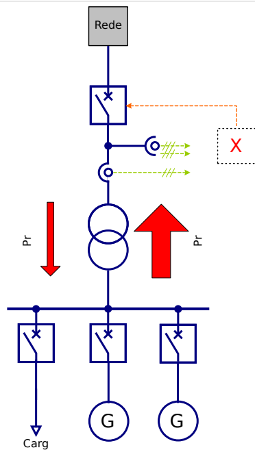
Fig. 129: Uso centralizado em redes com fonte de alimentação predominante.
