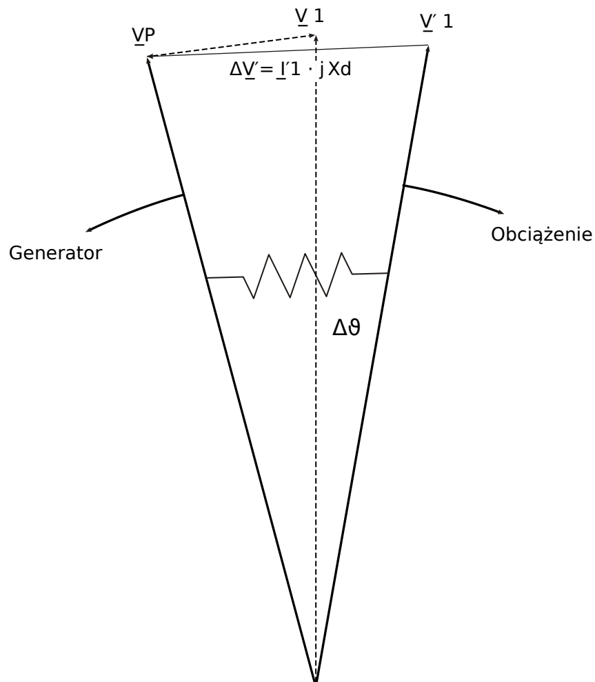
Rys. 115: Wektory napięcia przy awarii sieci.
