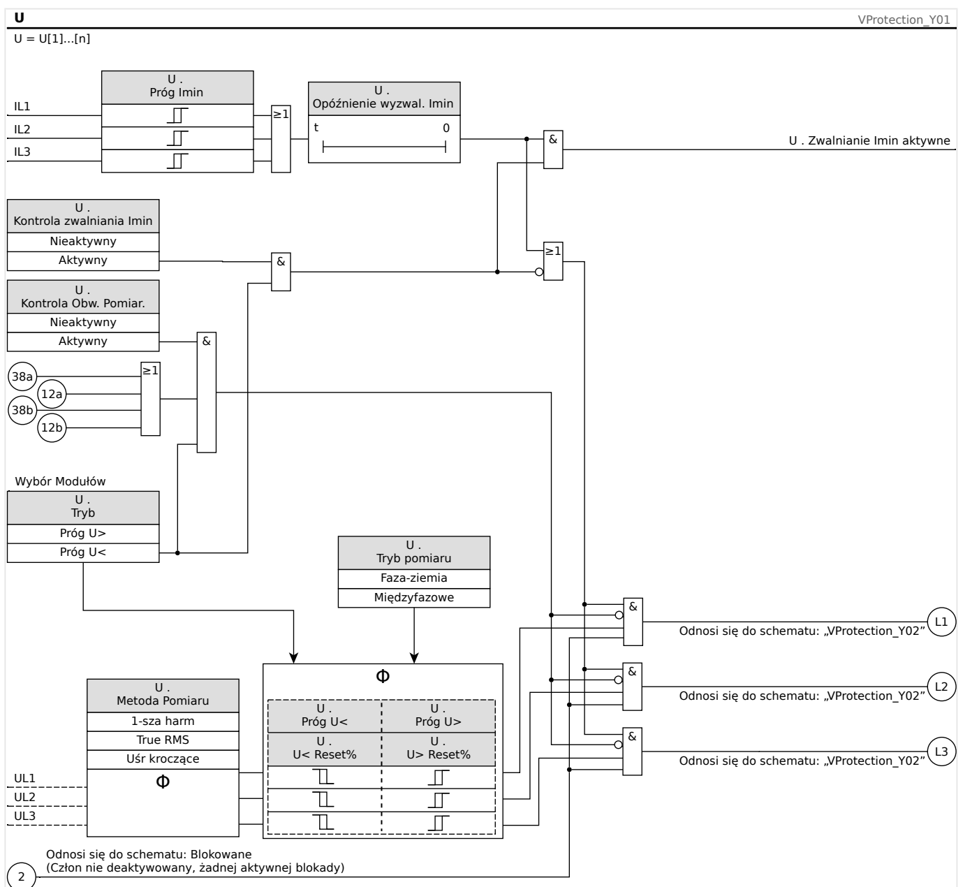
Rys. 108: Działanie modułu zabezpieczenia napięciowego, część 1.
