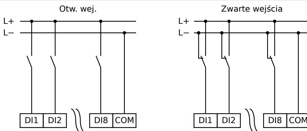
Rys. 164: Stan bezpieczny wejść dwustanowych
