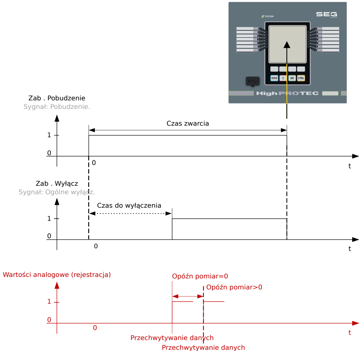
Rys. 153: Rejestrator zwarć: czasy (trwania).
