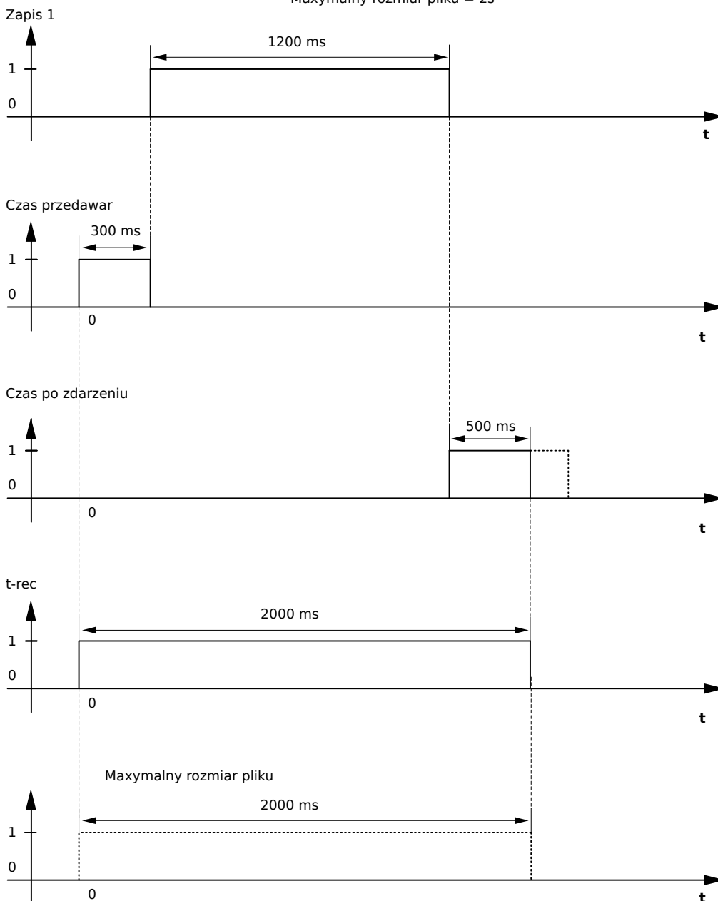
Rys. 151: Przykładowy wykres czasów pracy rejestratora zakłóceń I
