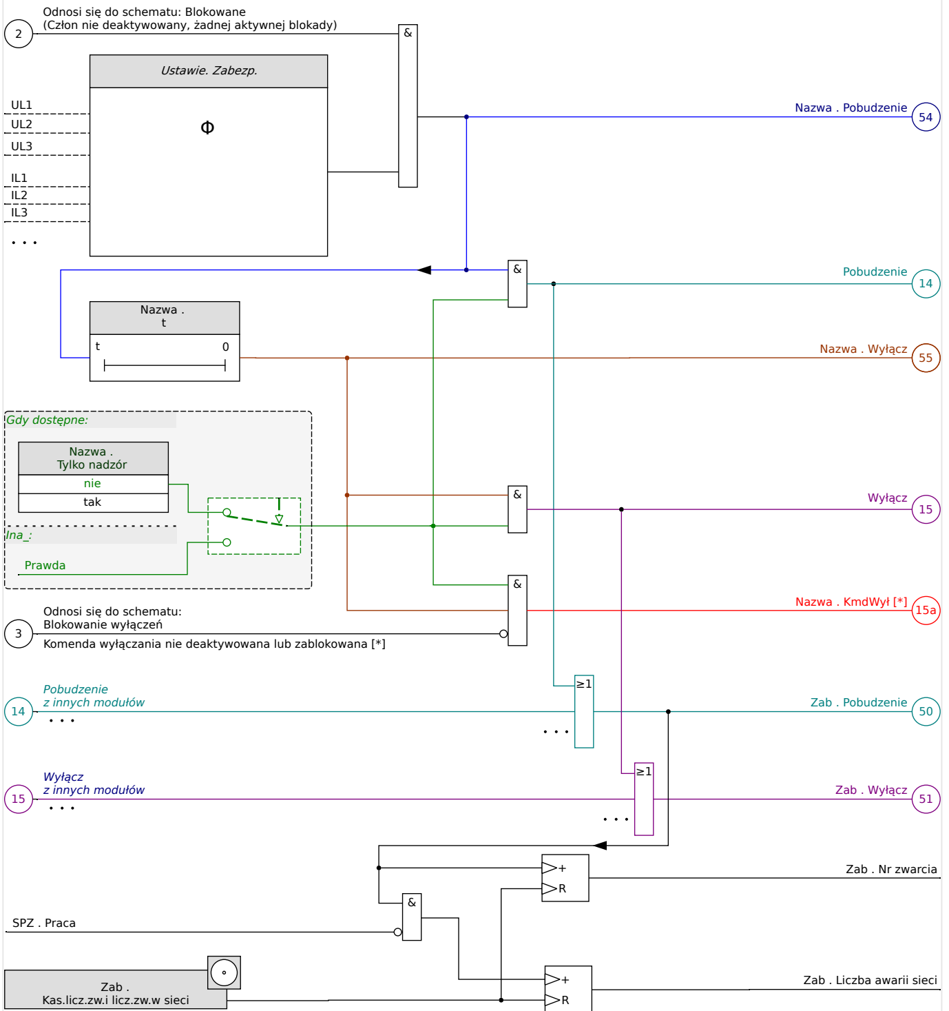
Rys. 63: Schemat ogólny działania każdego elementu zabezpieczającego HighPROTEC.
