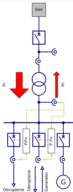
Rys. 128: Zdecentralizowane podczęstotliwościowe zmniejszanie obciążenia w sieciach z tymczasowym zasilaniem.
