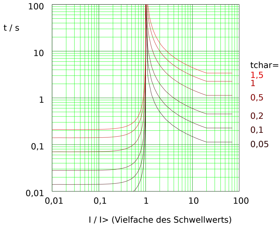
Abb. 84: NINV: Rückfallverzögerung (linke Hälfte, I < I_n ) und Auslöseverzögerung (rechte Hälfte, I > I_n ), Beispieldiagramm für I_{max} = 20 \cdot I_n .
