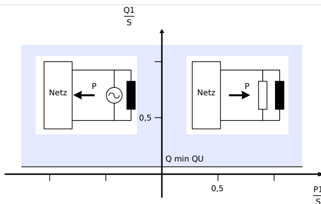
Abb. 140: Variante 2: Reine Blindleistungsschwellwertüberwachung.
