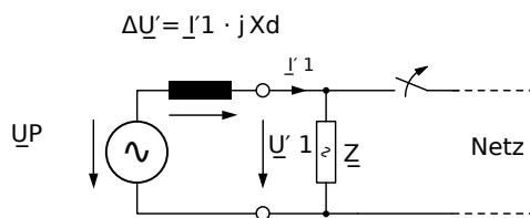
Abb. 130: Ersatzschaltbild Synchrongenerator bei Netzausfall.
