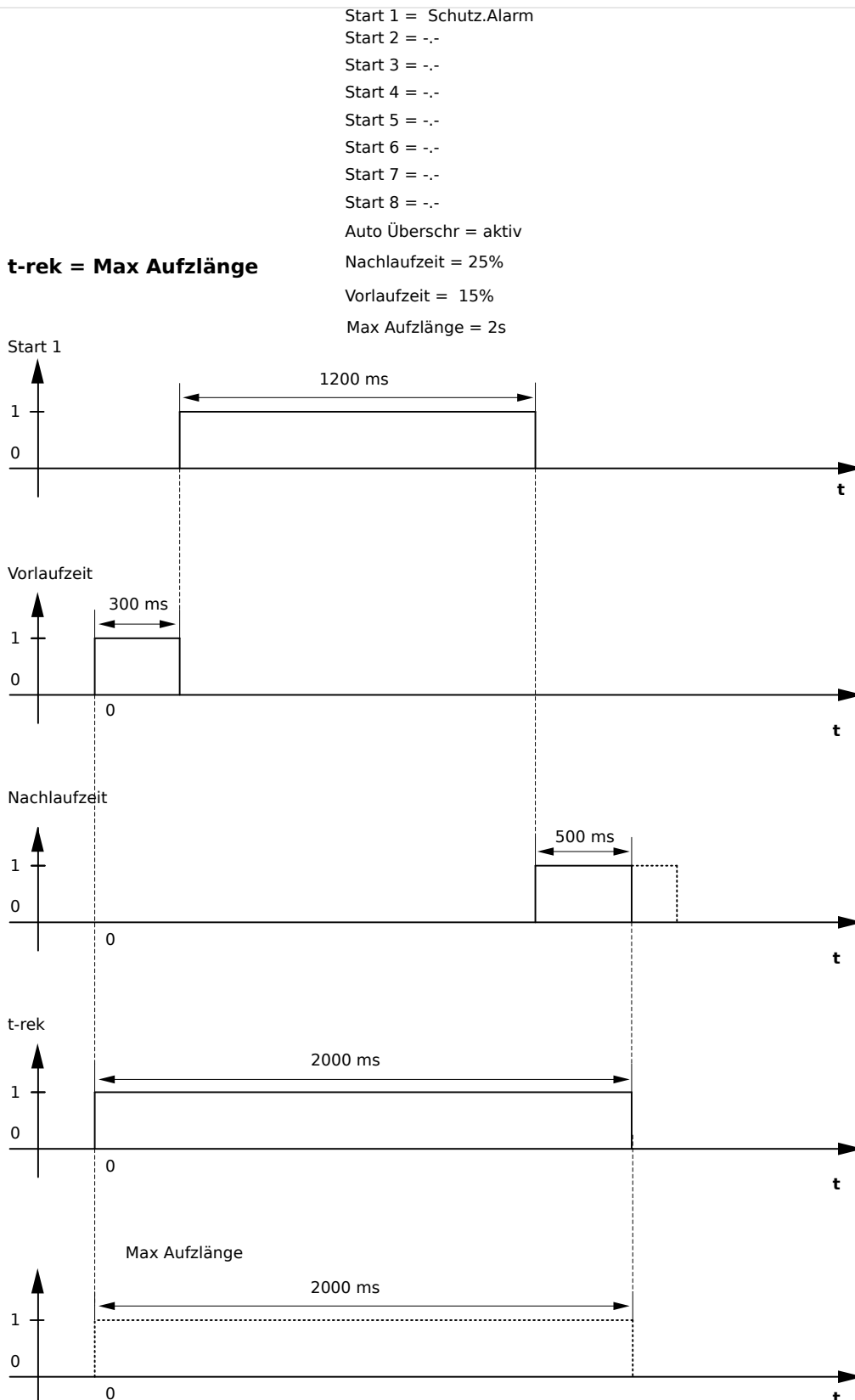
Abb. 168: Beispiel I Störschreiber-Ablaufdiagramm
