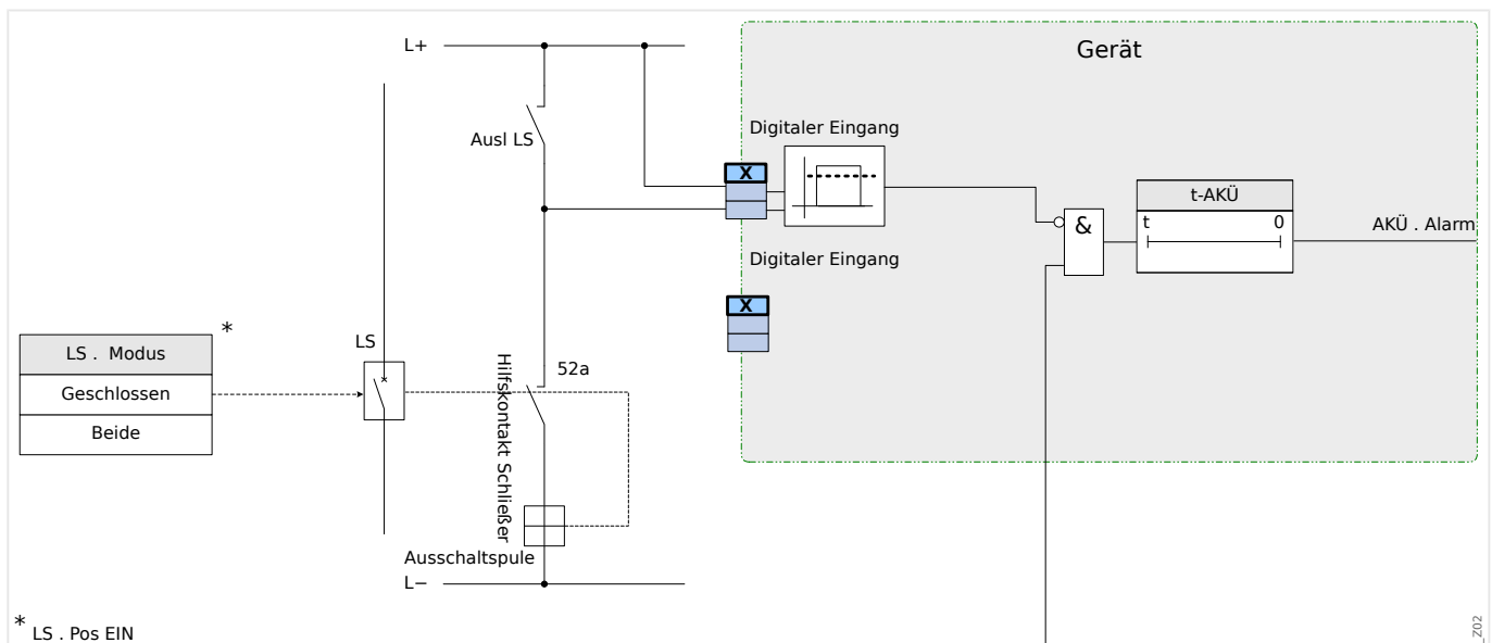
Abb. 157: Anschlussbeispiel: Auslösekreisüberwachung mit einem Hilfskontakt »Hiko EIN« (52a).
