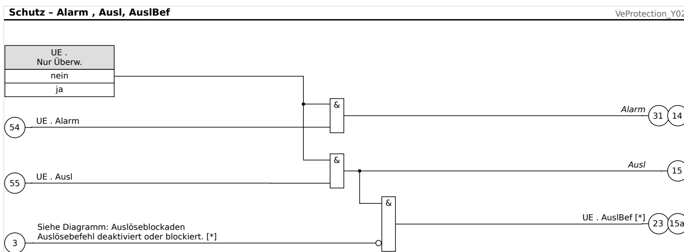
Abb. 127: UE/UX-Spannungsüberwachung, Teil 2 (Aus-Befehl und Anstoßen von Generalanregung und General-Auslösung).
