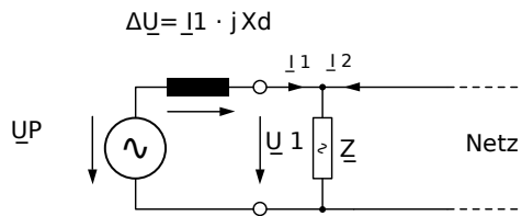
Abb. 128: Ersatzschaltbild netzparalleler Synchrongenerator
