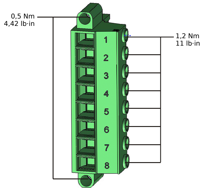
Abb. 179: Spannungsmesstecker der Spannungsmesskarte „TU“ (↳ „2.6.1 TU - Spannungsmesseingänge“).
