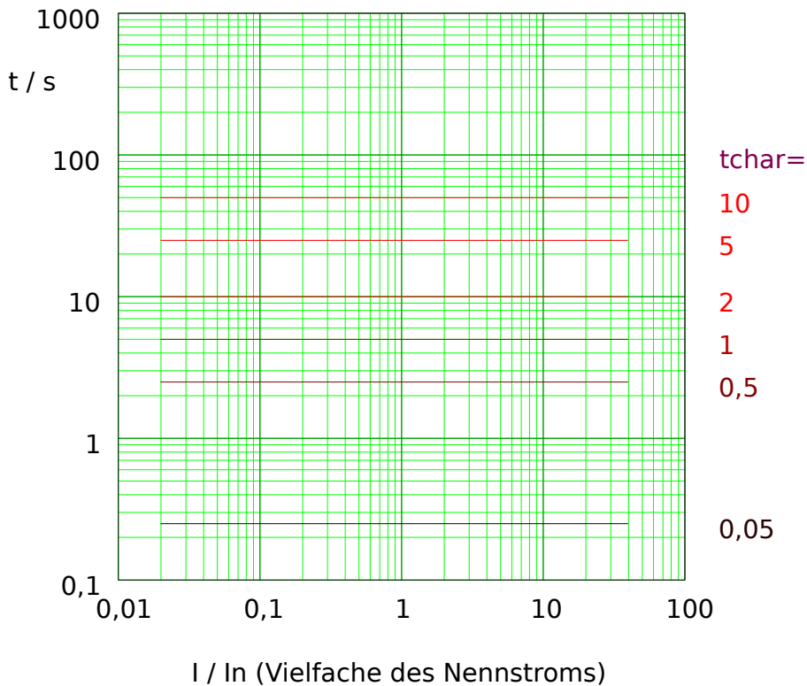
Abb. 92: Auslösekurve „Therm Flat“, wobei nur der Bereich I > I_n jeweils anwendbar ist.
