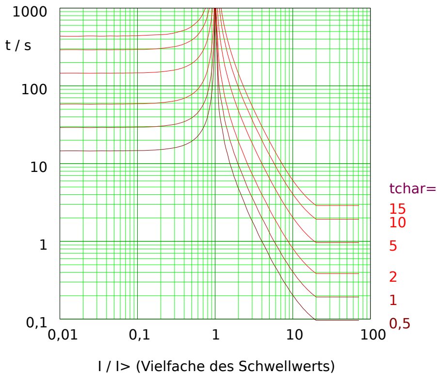
Abb. 90: EINV: Rückfallverzögerung (linke Hälfte, I < I> ) und Auslöseverzögerung (rechte Hälfte, I > I> ), Beispieldiagramm für I_{max} = 20 \cdot I> .
