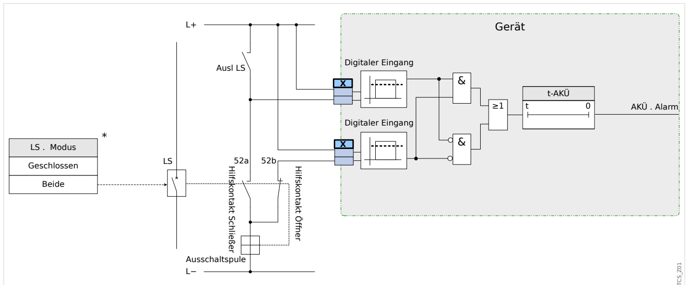
Abb. 156: Anschlussbeispiel (Empfehlung): Auslösekreisüberwachung mit zwei Hilfskontakten »Hiko EIN« (52a) und »Hiko AUS« (52b).
