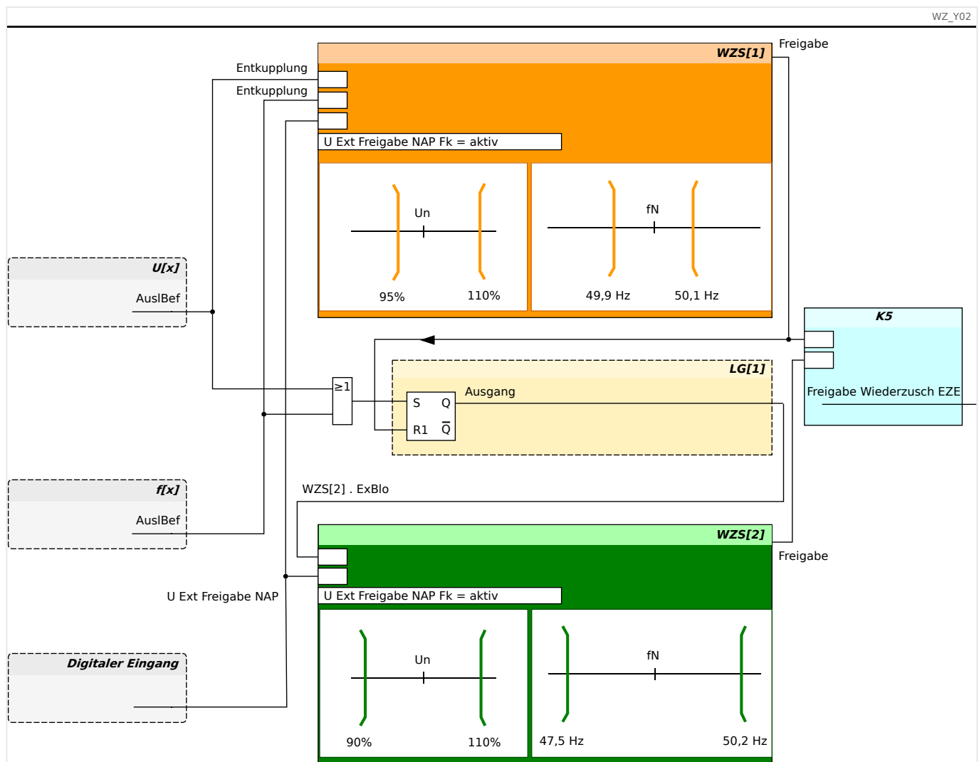
Abb. 141: Applikationsbeispiel für ein Zuschalten in Abhängigkeit von einer vorherigen Schutzauslösung.
