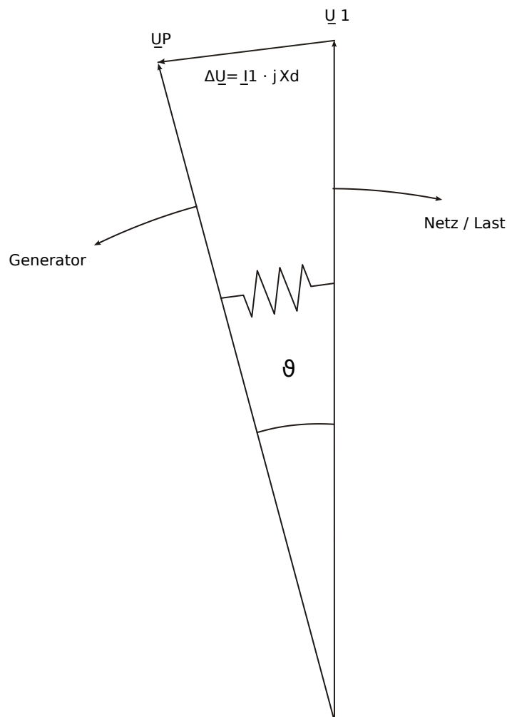
Abb. 129: Polradwinkel bei konstanter Belastung des Generators.
