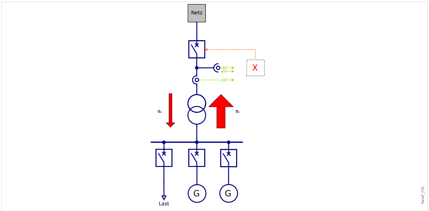
Abb. 146: Zentraler Einsatz in Teilnetzen mit überwiegender Rückspeisung.
