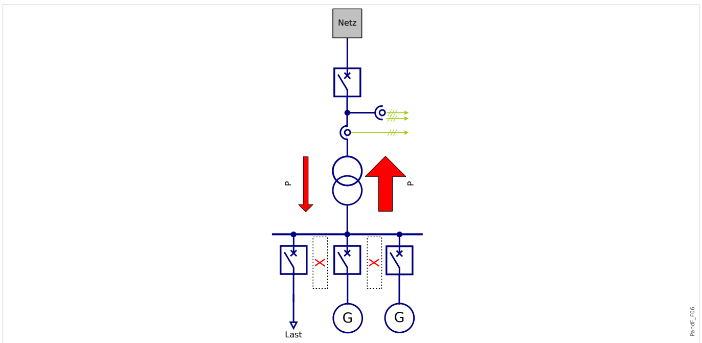
Abb. 147: Dezentraler Einsatz in Teilnetzen mit überwiegender Rückspeisung.
