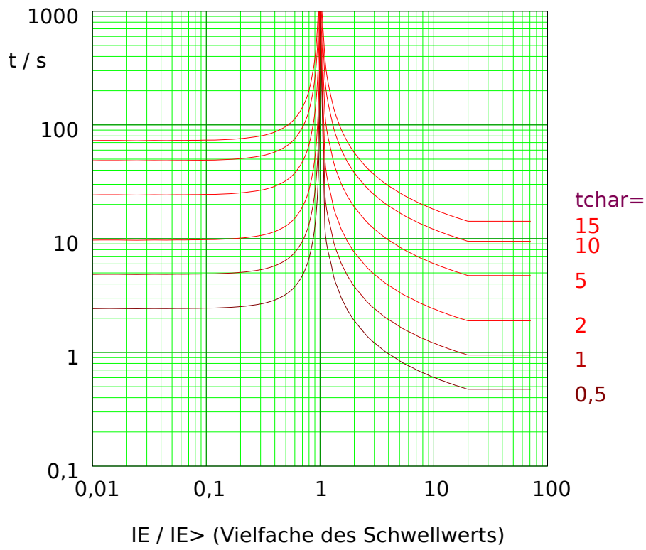
Abb. 100: MINV: Rückfallverzögerung (linke Hälfte, IE < IE_{>} ) und Auslöseverzögerung (rechte Hälfte, IE > IE_{>} ), Beispieldiagramm für I_{E,max} = 20 \cdot IE_{>} .
