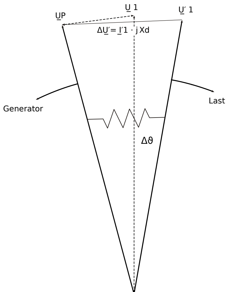
Abb. 131: Änderung des Polradwinkels bei plötzlicher Belastung des Generators.
