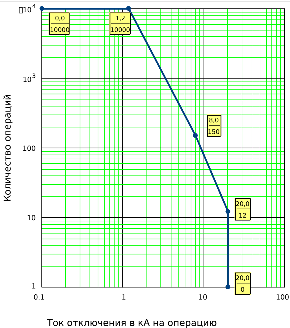
Рис. 138: Эксплуатационная кривая выключателя для типичного выключателя 25кВ
