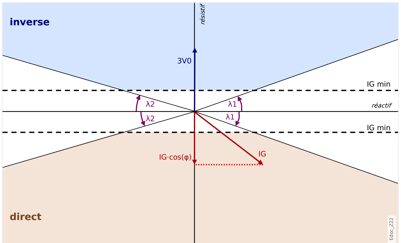
Fig. 67: Principe de détermination de la direction pour la méthode « \cos(\phi) ».
