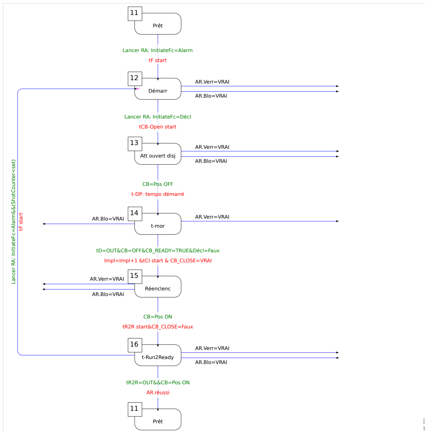
Fig. 91: Cycle d'exécution du AR (état 4).
