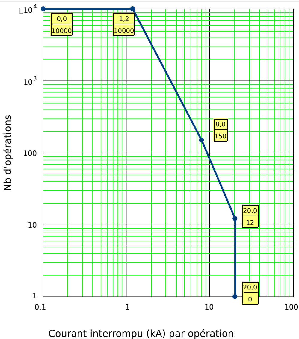
Fig. 138: Courbe de maintenance du disj pour un disj 25 ~kV typique
