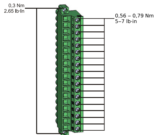
Fig. 155: Bornes de mesure de tension des cartes de mesure « TU-OR5 » et « TU-DI8 ».
