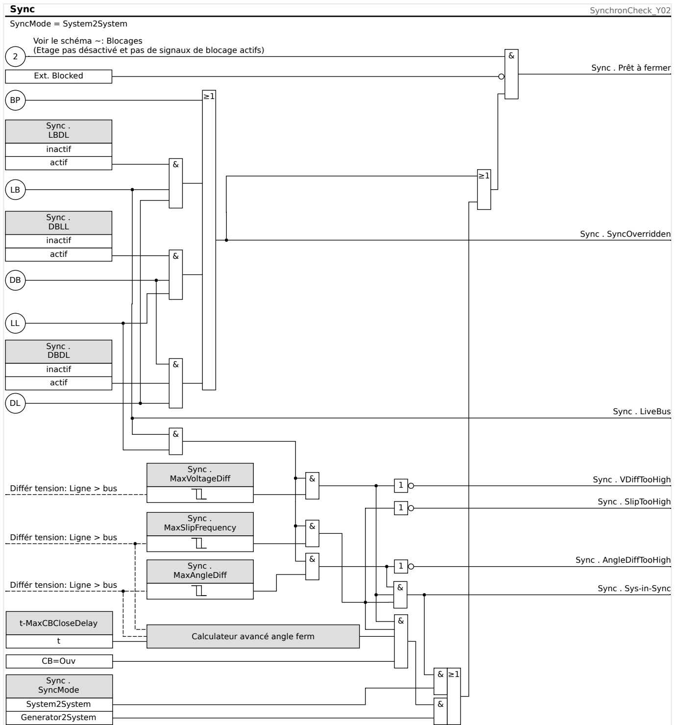
Fig. 111: Fonctionnalité du module «Sync», « System2System ».
