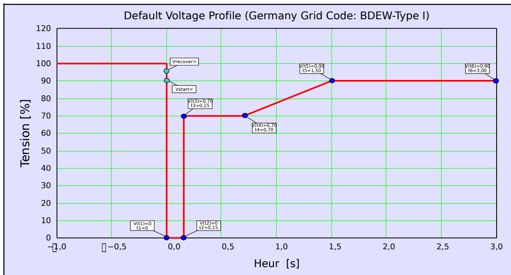
Fig. 126: Profil LVRT prédéfini en usine (BDEW-Type I).
