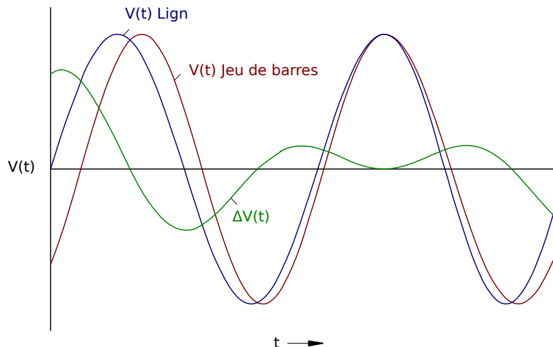
Fig. 109: Courbe de tension avec résolution agrandie
