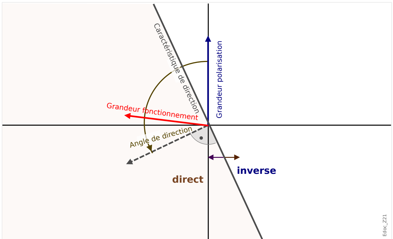
Fig. 65: Principe de détection de la direction pour toutes les méthodes excepté « \cos(\phi) », « \sin(\phi) ».
