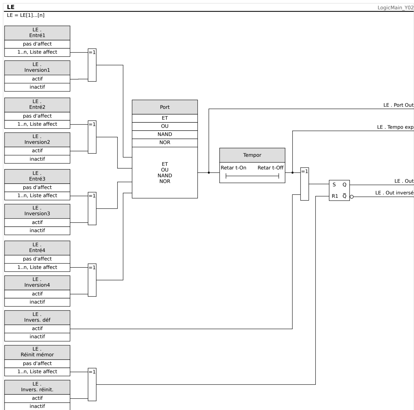
Fig. 145: Présentation détaillée - Diagramme logique global.
