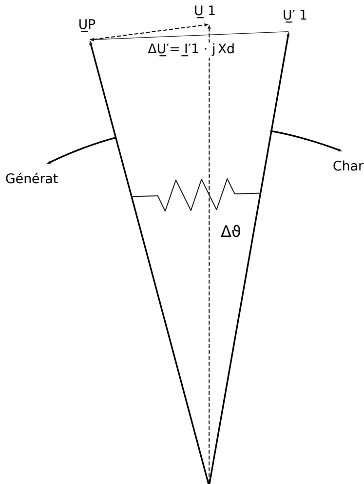
Fig. 105: Vecteurs de tension en cas de coupure de réseau.
