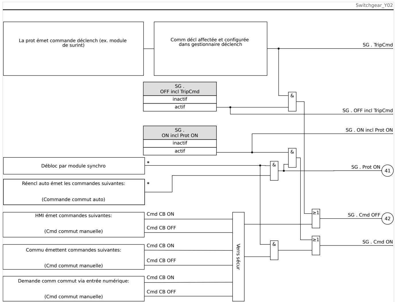
Fig. 136: Verrouillages (Parties identifiées par « * » : la disponibilité dépend du type de dispositif commandé.)
