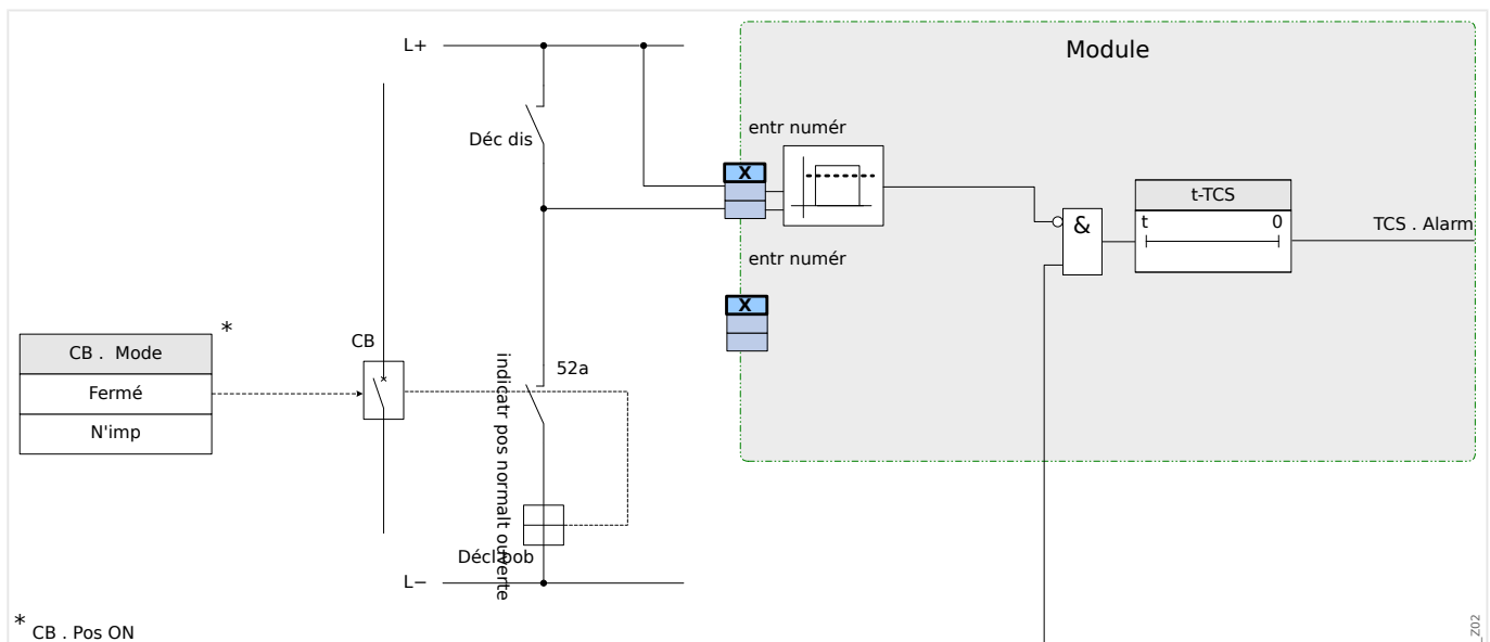
Fig. 130: Exemple de connexion : Surveillance du circuit de déclenchement avec un contact auxiliaire de disjoncteur «Aux ON» (52a).
