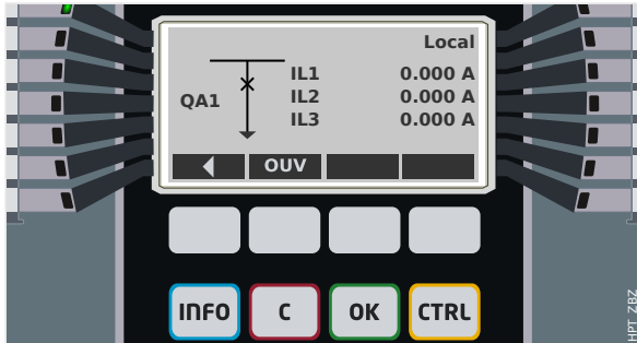
Fig. 133: Exemple de page de contrôle, avec le « disjoncteur » en position fermée.
