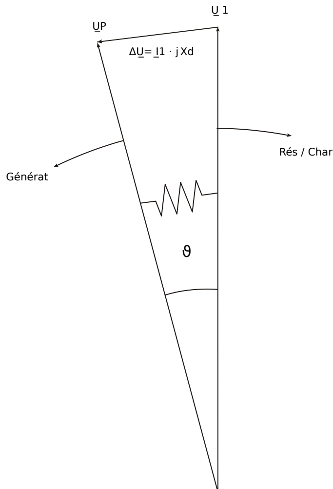
Fig. 103: Vecteurs de tension en fonctionnement parallèle du réseau.
