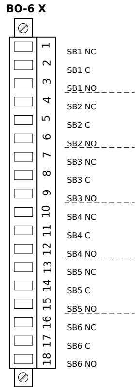
Fig. 13: Affectation électromécanique
