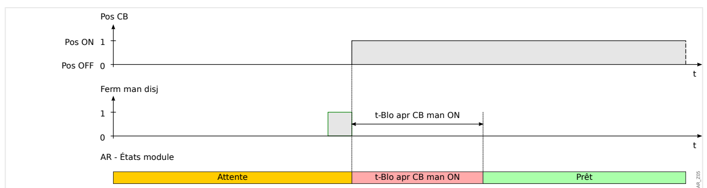
Fig. 94: États du réenclenchement automatique pendant la fermeture manuelle du disjoncteur.
