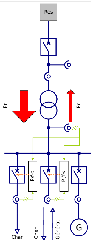
Fig. 118: Délestage de charge de sous-fréquence décentralisé au sein de réseaux avec alimentation temporaire.
