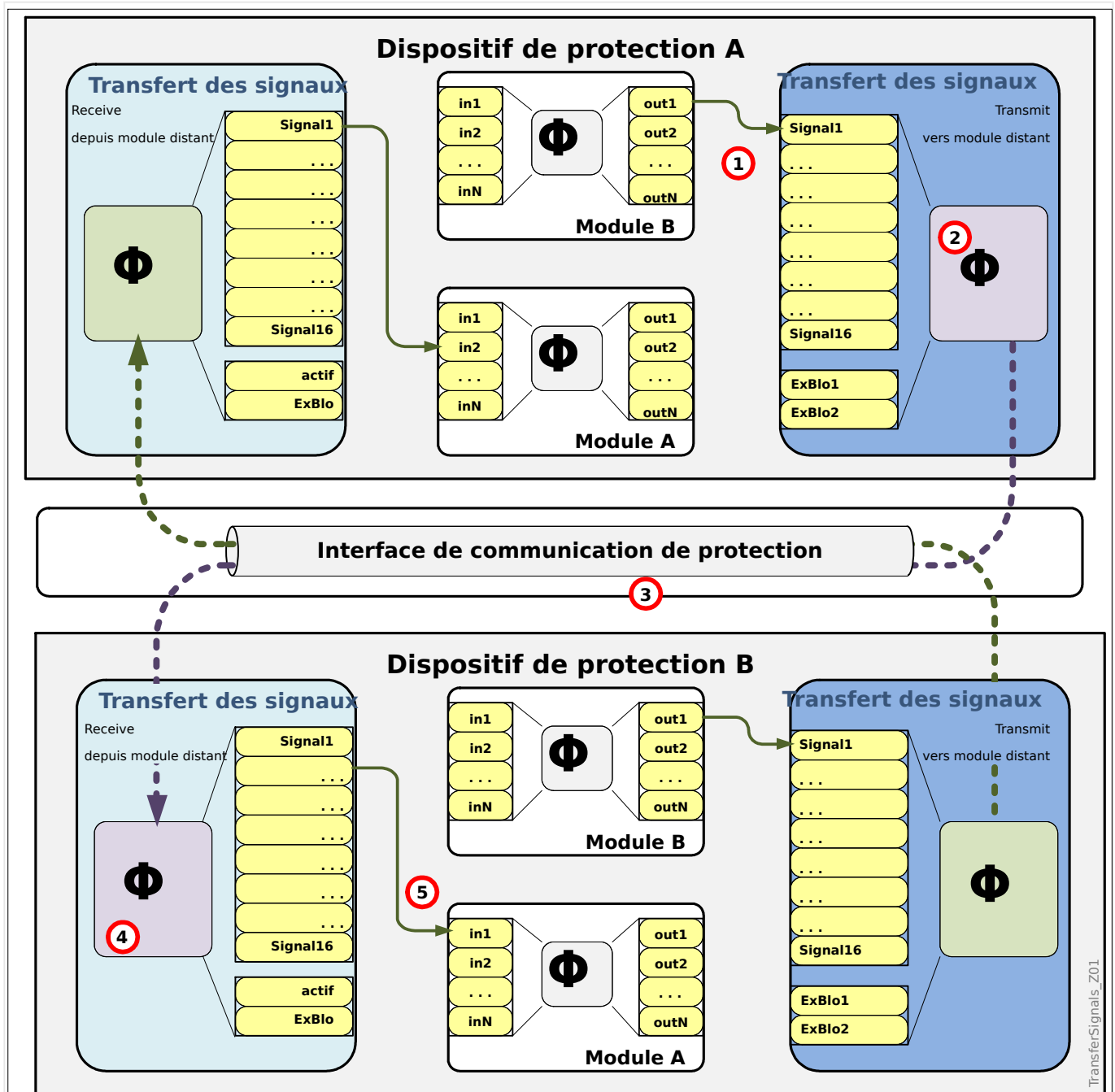
Fig. 82: Principe de la fonctionnalité «Sig-Trans».
