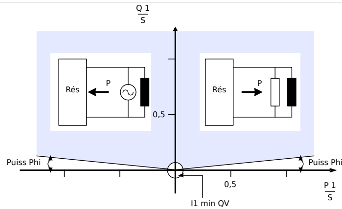
Fig. 113: Méthode 1 : Surveillance de l'angle de charge
