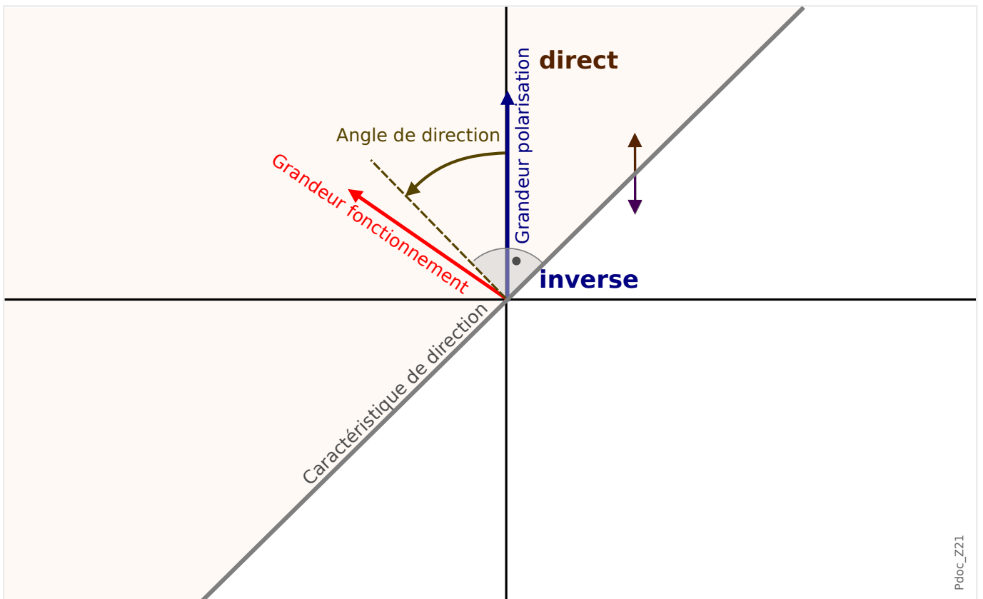
Fig. 63: Principe de la détection de la direction des défauts de phase.
