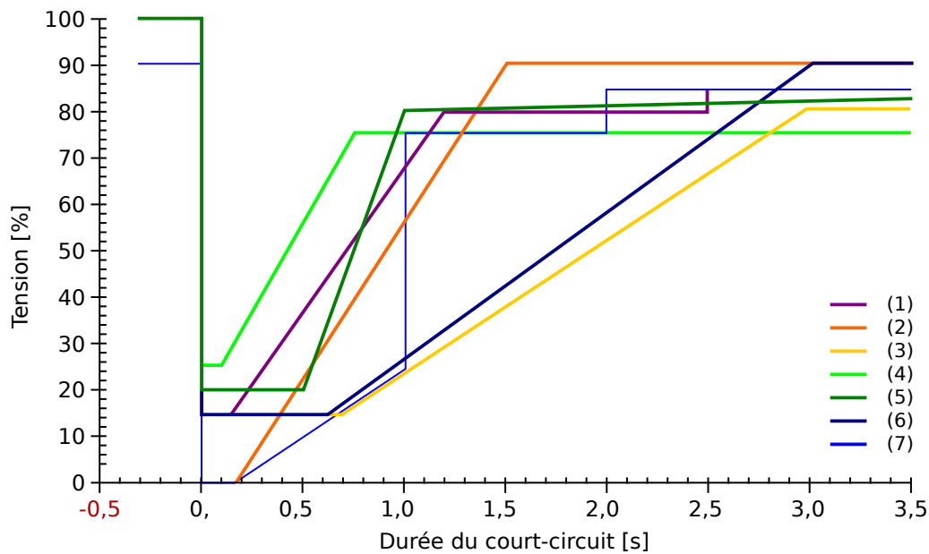
Fig. 123: Normes LVRT ; source : eBWK Bd. 60 (2008) N° 4. Auteurs: Dipl.-Ing. Thomas Smolka, Dr.-Ing. Karl-Heinz Weck, Zertifizierungstelle der FGH e.V., Mannheim, sowie Dipl.-Ing. (FH) Matthias Bartsch, Enercon GmbH, Aurich.
