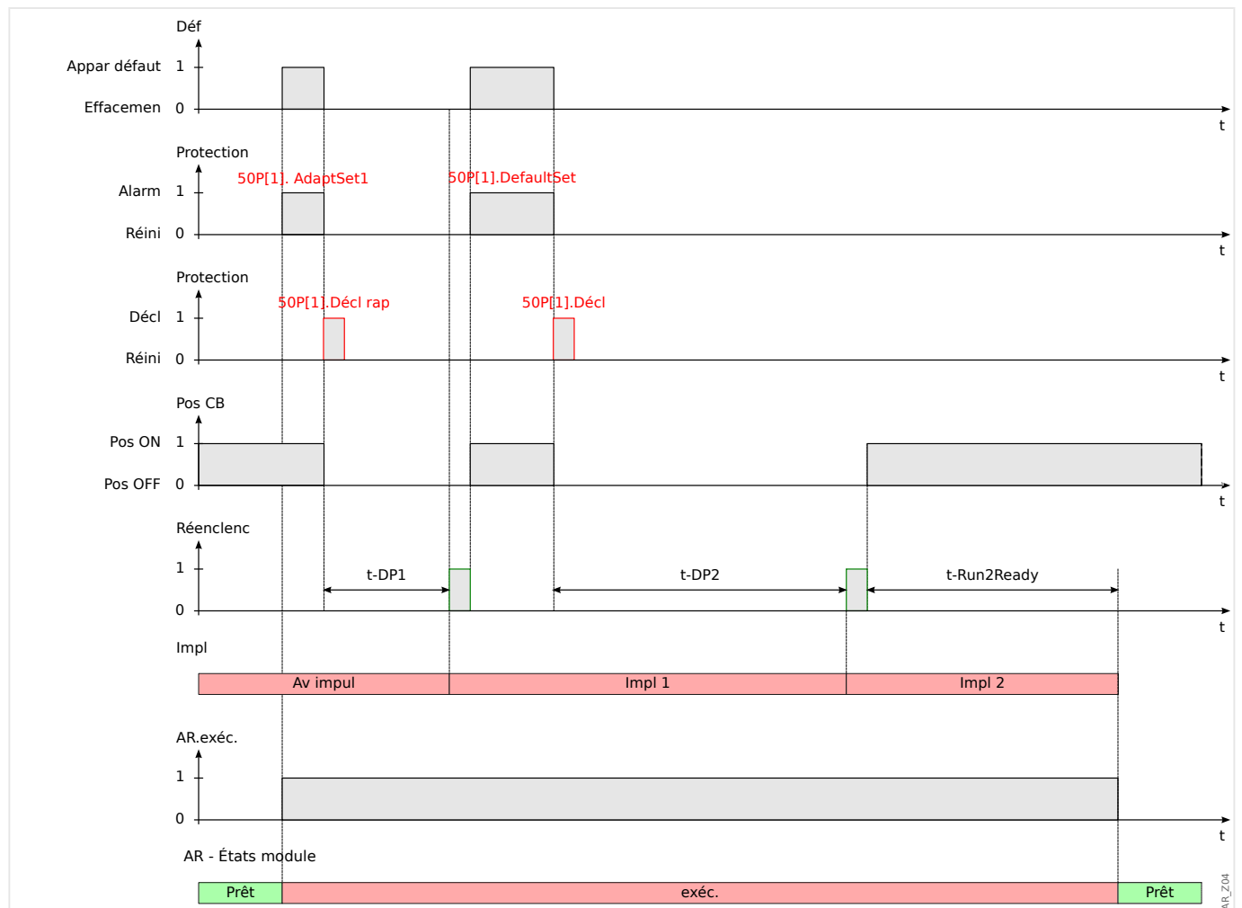
Fig. 93: Diagramme de temporisation de réenclenchement automatique pour un schéma de réenclenchement automatique à 2 impulsions réussi avec une accélération à la pré-impulsion.
