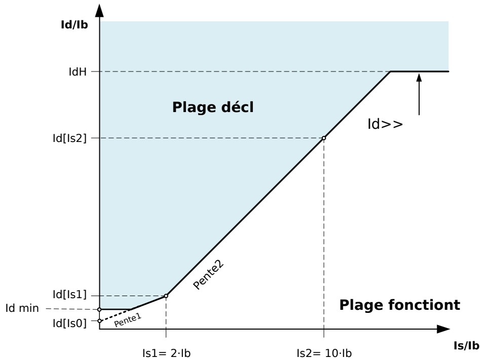
Fig. 77: Valeur IdH d'étape de niveau supérieur et non limitée de protection différentielle
