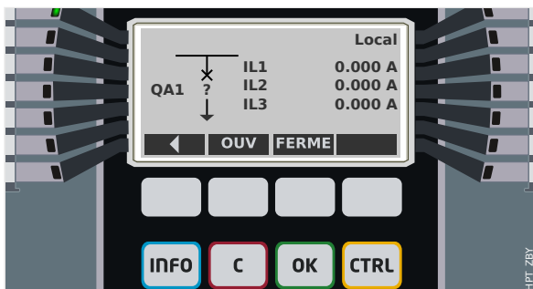
Fig. 134: Exemple de page de contrôle, avec le « disjoncteur » en position de dysfonctionnement (ou invraisemblable).
