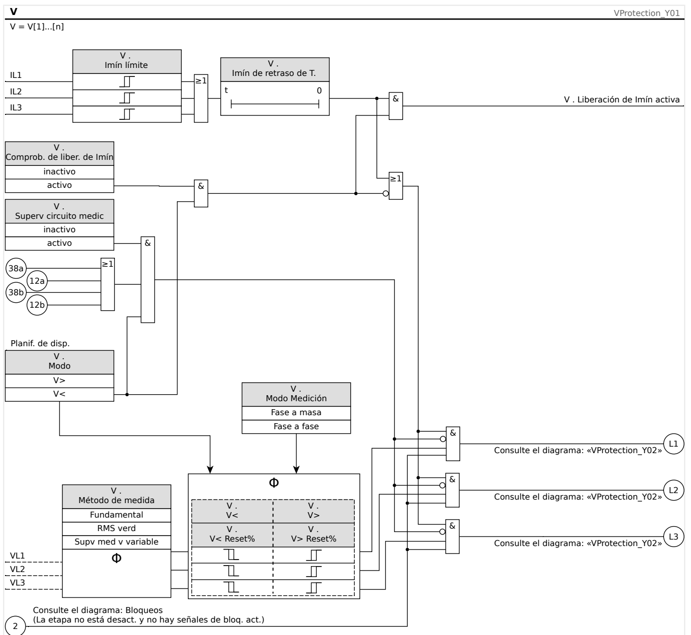
Fig. 98: Funcionalidad del módulo de protección de tensión, parte 1.
