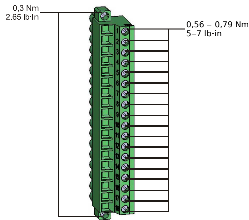
Fig. 155: Terminales de medición de tensión de tarjetas de medición “TU-OR5” y “TU-DI8” , ).
