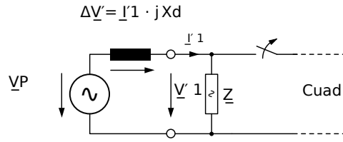
Fig. 104: Circuito equivalente en fallo de red eléctrica.
