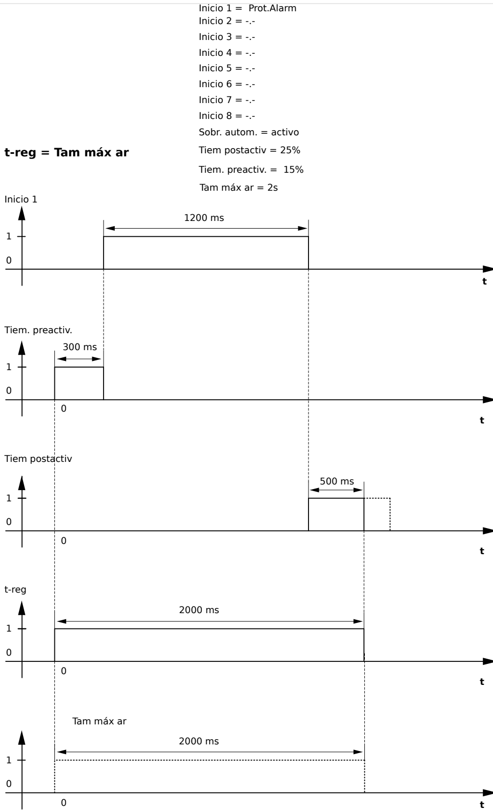
Fig. 141: Ejemplo 1: cuadro de intervalos del registrador de perturbaciones
