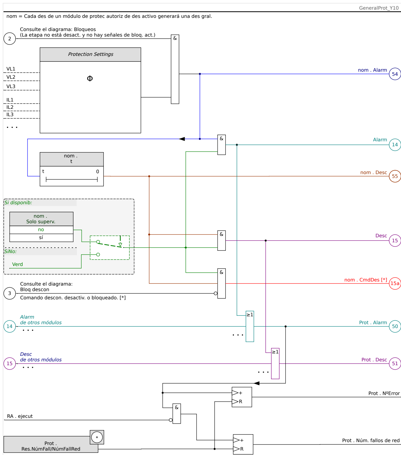
Fig. 62: Descripción a grandes rasgos de la funcionalidad de cualquier elemento de protección de HighPROTEC.
