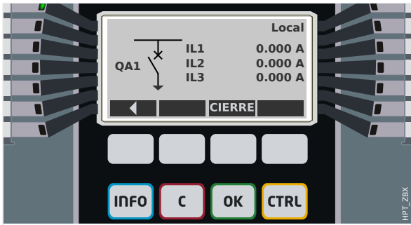
Fig. 135: Ejemplo de página de control, con el circuito en posición abierta.
