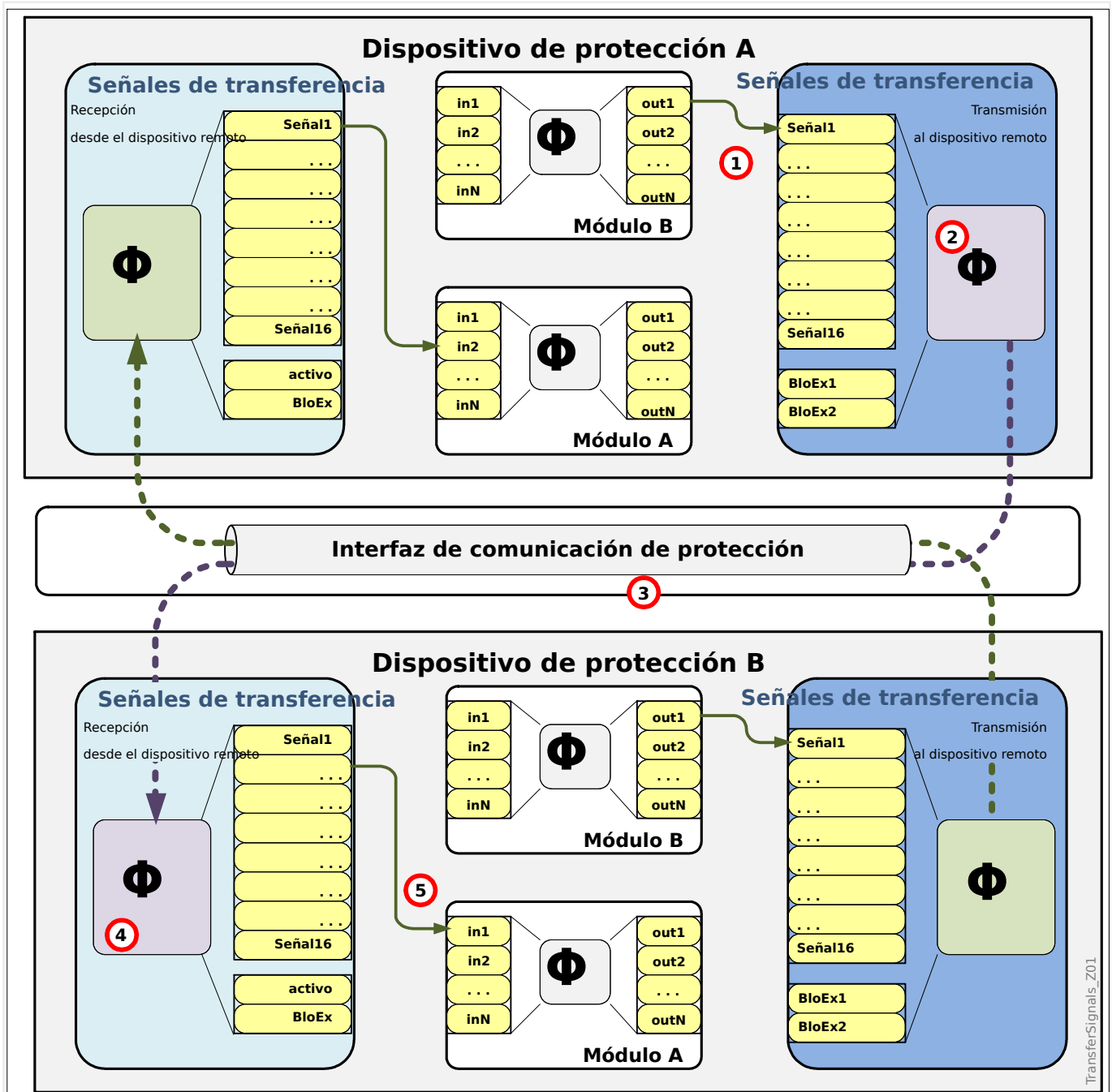
Fig. 82: Principio de funcionalidad de «Transf. señal».
