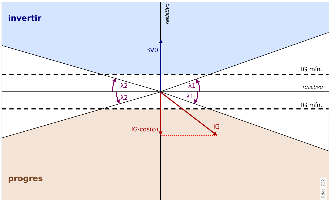
Fig. 67: Principio para determinar la dirección en el método "cos(φ)".
