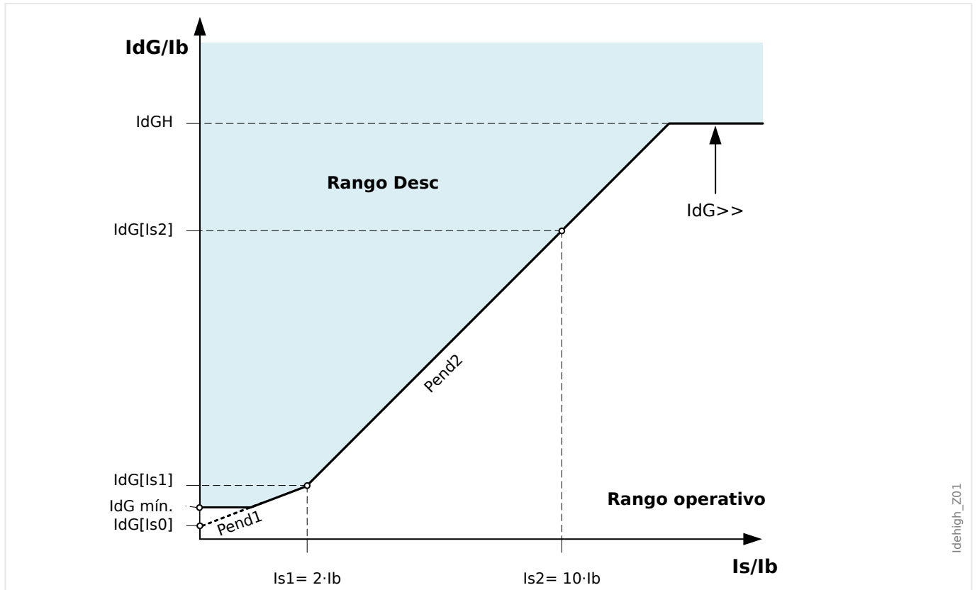
Fig. 79: Valor de selección »IdG>>« de la corriente de diferencial de tierra basada en la corriente nominal »lb« del objeto de protección relacionado.
