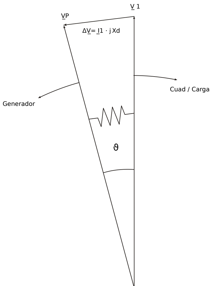
Fig. 103: Vectores de tensión en funcionamiento en paralelo con la red de suministro eléctrico.
