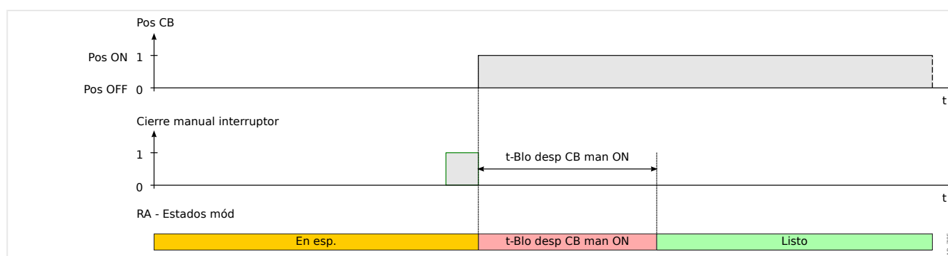
Fig. 94: Estados de reconexión automática durante el cierre manual del interruptor.
