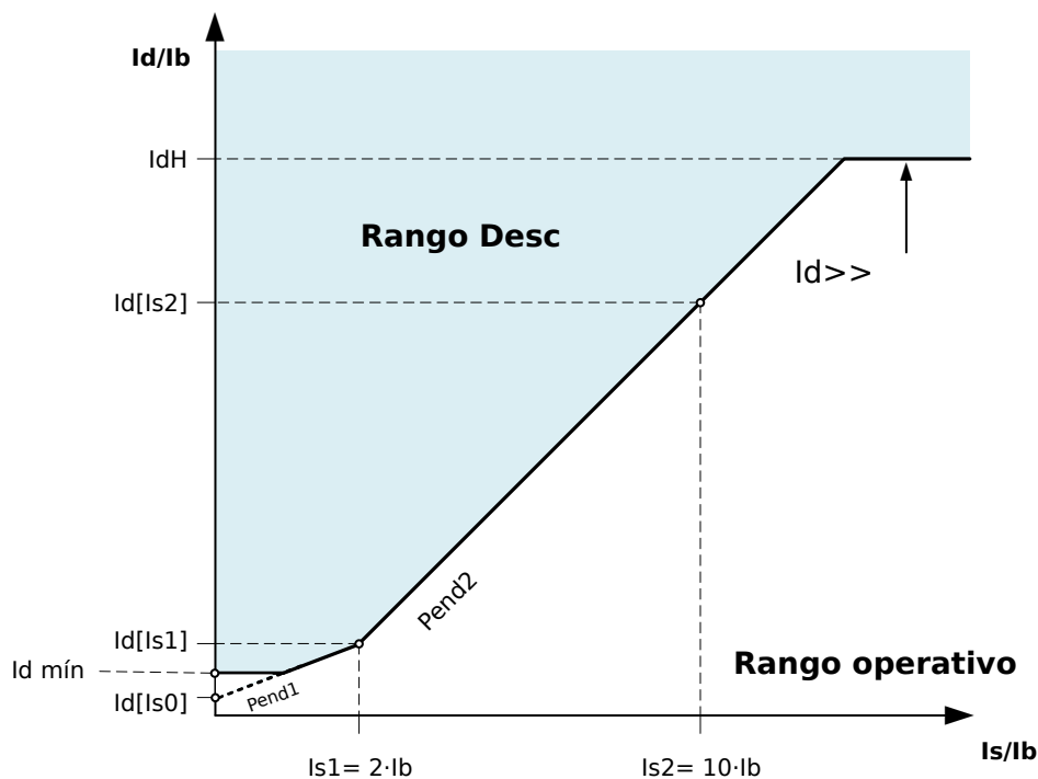
Fig. 77: Paso de protección de diferencial de ajuste alto no limitado IdH.
