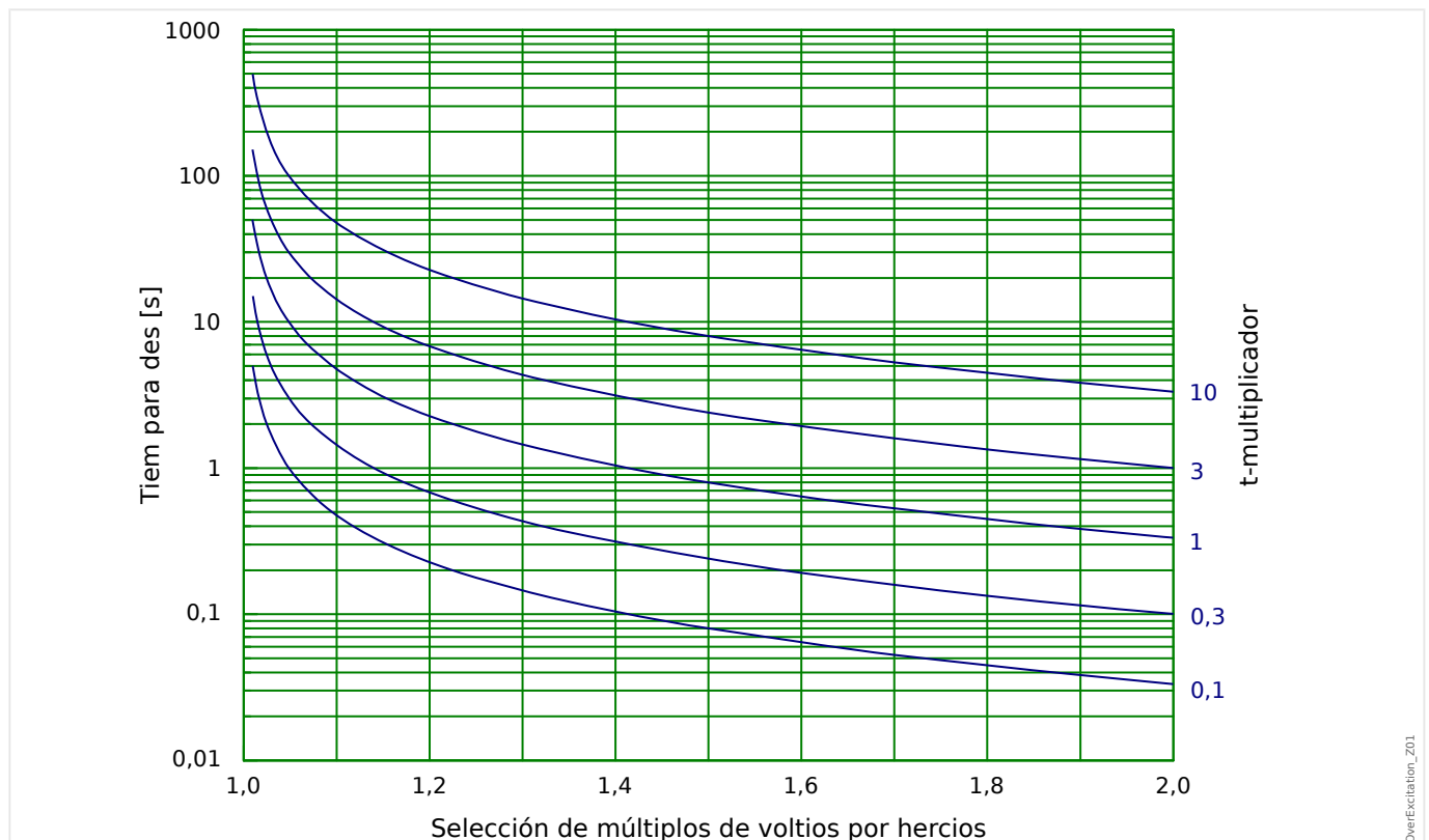
Fig. 86: Características/Forma curva: INV A
