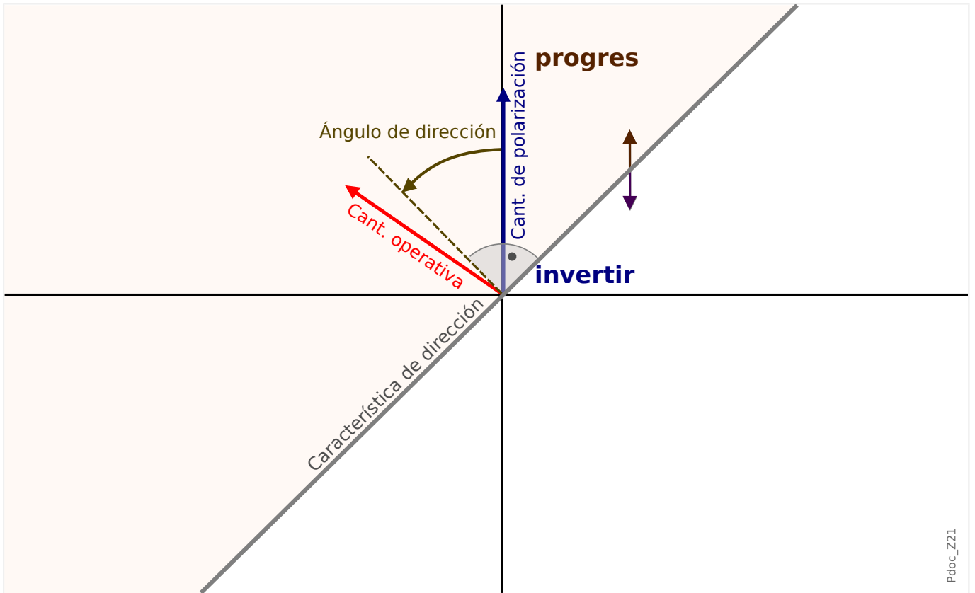
Fig. 63: Principio de detección de dirección de fallo de fase
