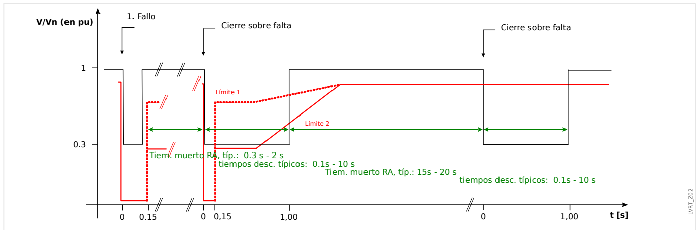
Fig. 124: Recorrido de la curva de tensión durante dos intentos fallidos de reconexión automática; fuente: Technische Richtlinie, Erzeugungsanlagen am Mittelspannungsnetz, Ausgabe Juni 2008, BDEW Bundesverband der Energie- und Wasserwirtschaft e.V. (Página 89).
