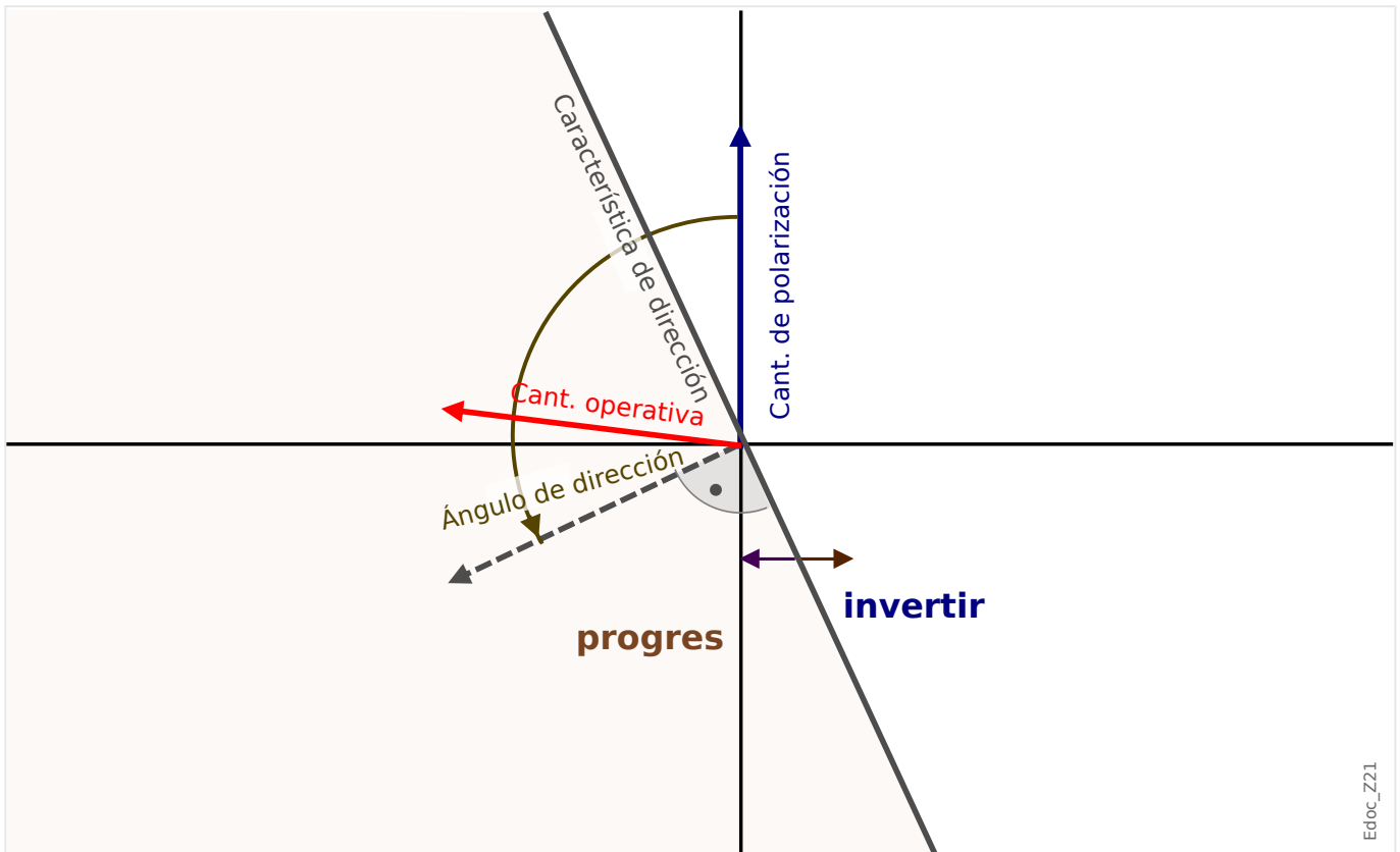
Fig. 65: Principio para determinar la dirección en todos los métodos, excepto " \cos(\phi) ", " \sin(\phi) ".
