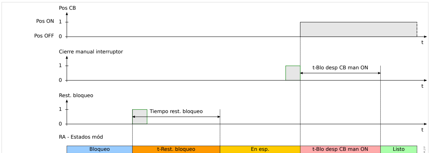
Fig. 96: Lógica de reinicio de bloqueo de AR en caso de que el reinicio de bloqueo llegue antes de que se cierre el interruptor manualmente.
