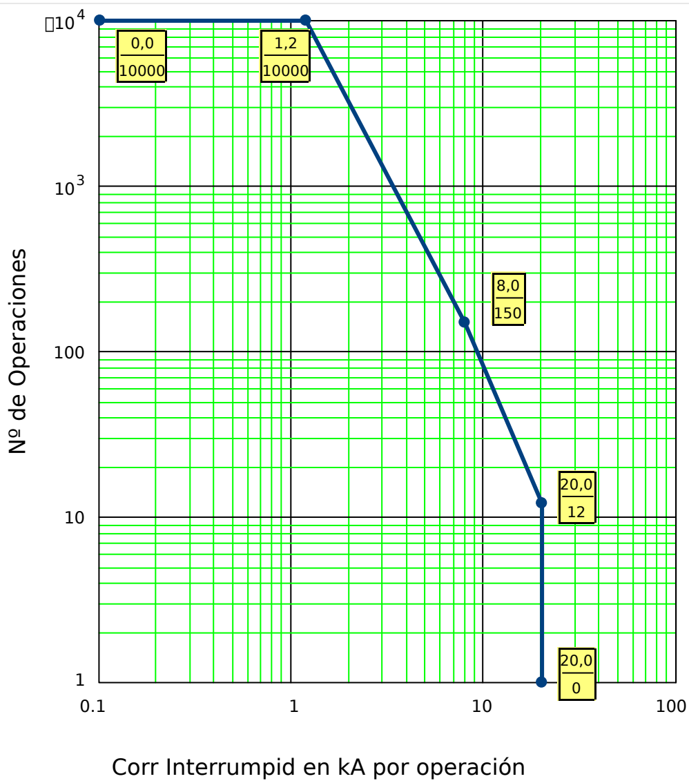
Fig. 138: Curva Mantenim Interruptor para Interrupt Circuito típico 25kV
