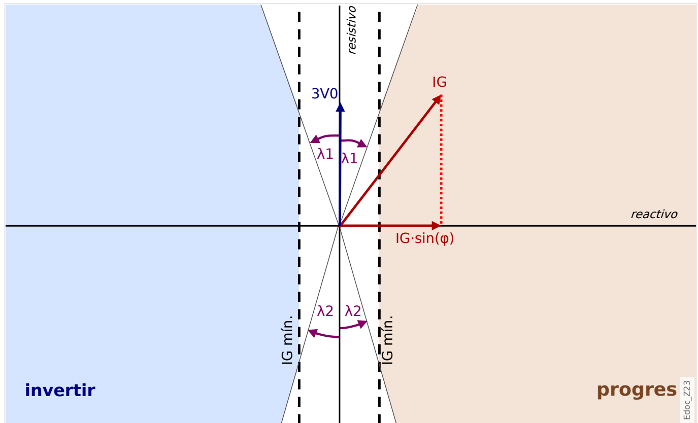
Fig. 68: Principio para determinar la dirección en el método "sin(φ)".
