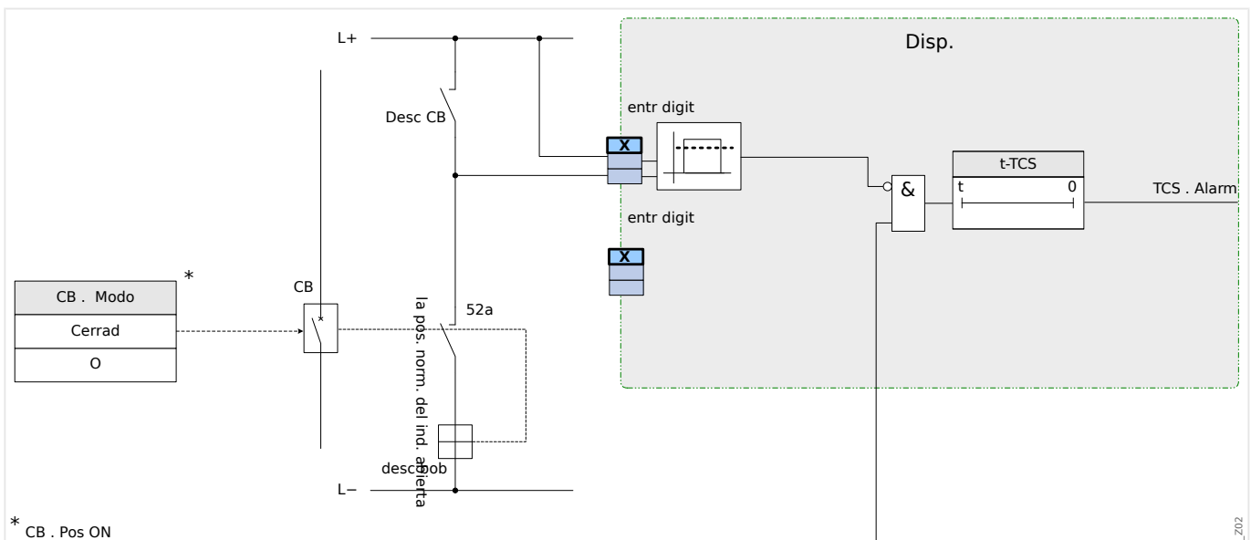
Fig. 130: Ejemplo de conexión: Supervisión del circuito de desconexión solo con un contacto auxiliar CB »Aux ON« (52a).
