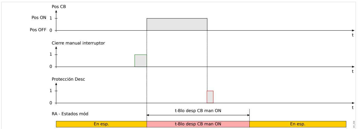
Fig. 95: Desconexión de protección mientras transcurre el tiempo de bloqueo de cierre manual.
