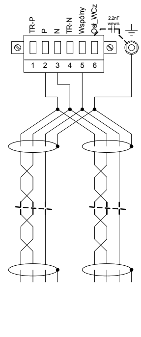
Ekranowanie po stronie urządzenia uziomione. Brak rezystorów terminujących.
