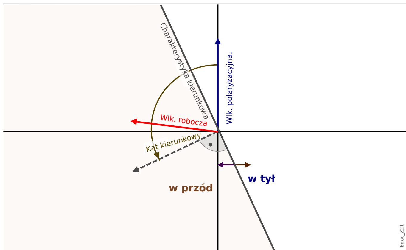
Rys. 74: Zasada określania kierunku obowiązująca dla wszystkich metod z wyjątkiem „ \cos(\phi) ”, „ \sin(\phi) ”.
