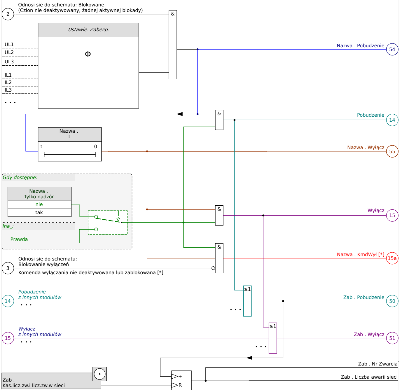
Rys. 71: Schemat ogólny działania każdego elementu zabezpieczającego HighPROTEC.
