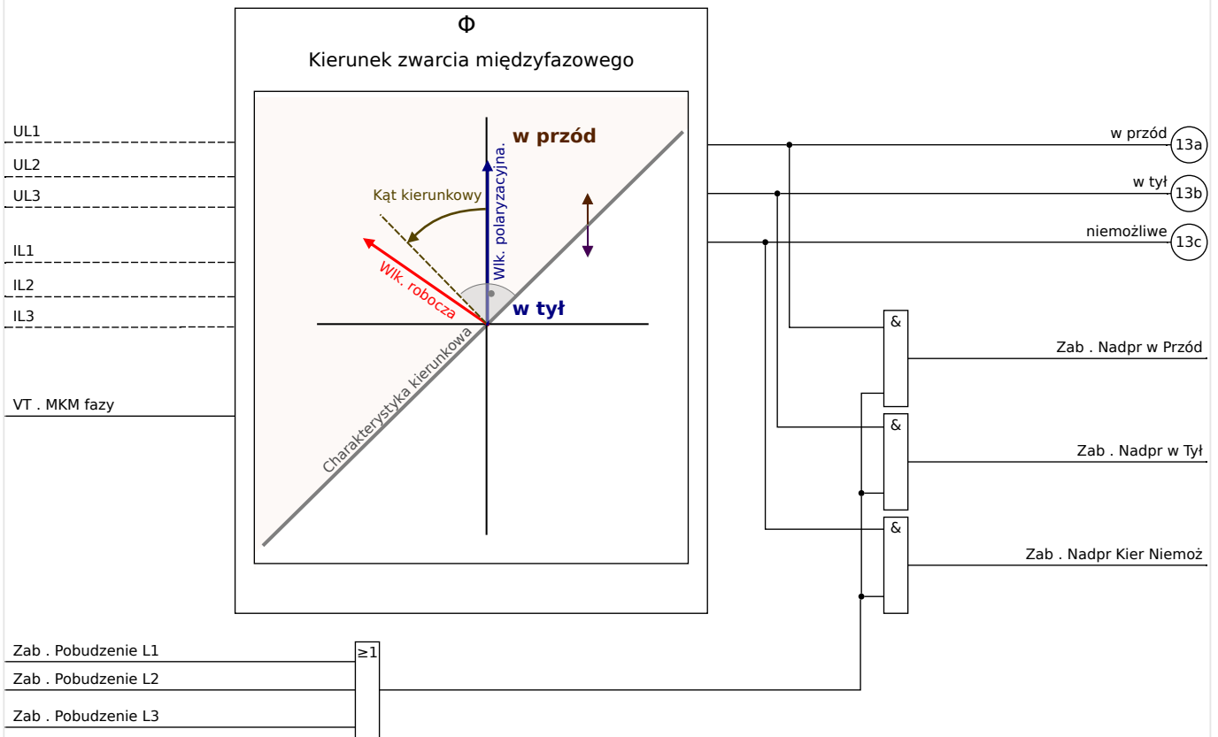
Rys. 73: Kierunek zwarcia międzyfazowego.
