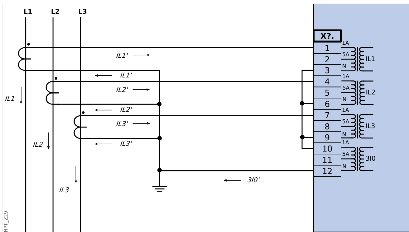
Rys. 23: Trójfazowy pomiar prądu; I_n wtórny = 1 A. Pomiar prądu doziemnego w układzie Holmgreena 3I_0 wtórny = 1 A.
