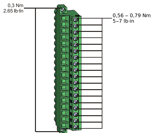
Rys. 176: Zaciski pomiaru napięcia kart pomiarowych „TU-OR5” i „TU-DI8”).
