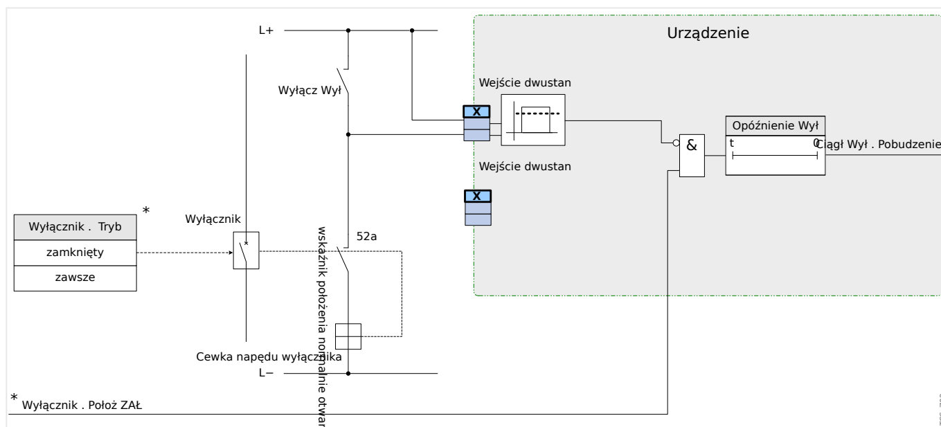
Rys. 151: Przykład okablowania: Układ kontroli ciągłości obwodów wyłącznika z tylko jednym stykiem pomocniczym wyłącznika „Położ ZAŁ” (52a).
