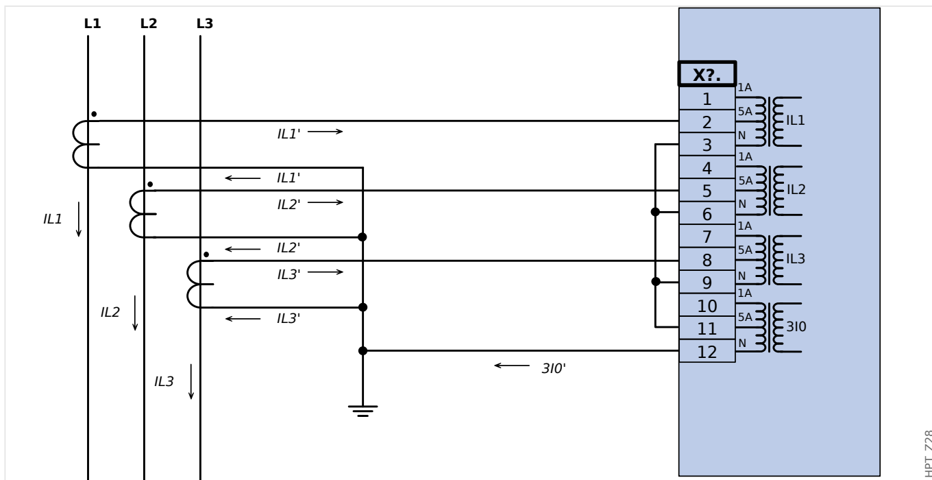
Rys. 22: Trójfazowy pomiar prądu; I_n wtórny = 5 A. Pomiar prądu doziemnego w układzie Holmgreena 3I_0 wtórny = 5 A.
