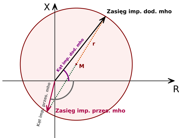
Rys. 92: Obszar roboczy (w kolorze jasnoczerwonym) typu MHO (okręgu), przy „Włączenie kierunku” = „Nieaktywny”.
