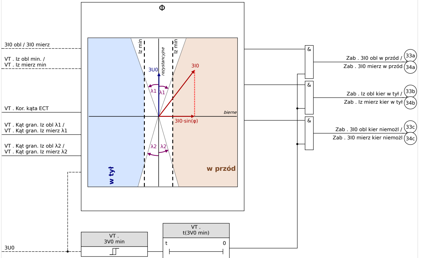
Rys. 79: Określanie kierunku metodą „sin( \phi )”.
