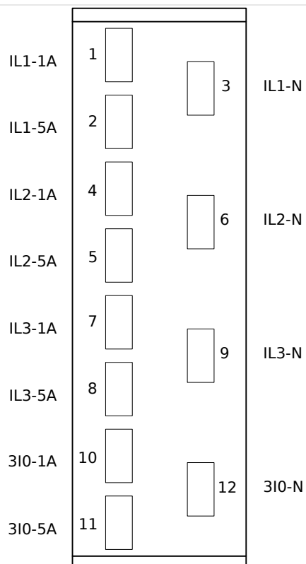
Rys. 19: TIs — przypisanie elektromechaniczne
