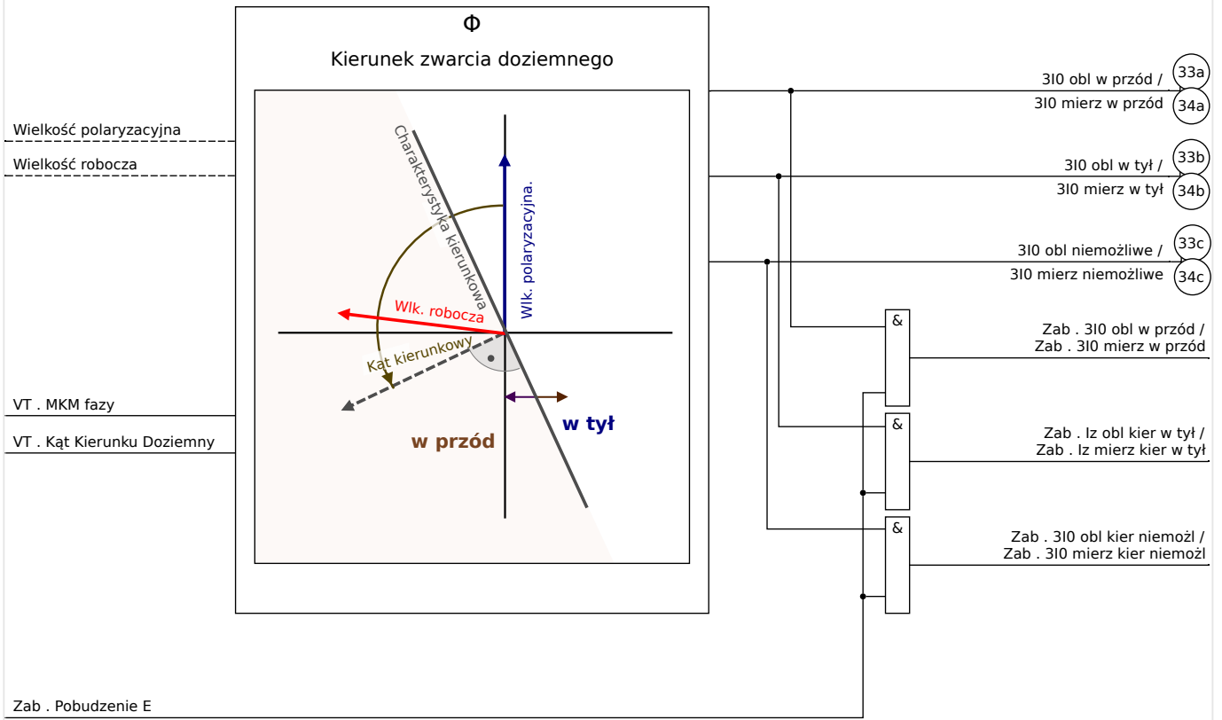
Rys. 75: Zasada określania kierunku obowiązująca dla wszystkich metod z wyjątkiem „ \cos(\phi) ”, „ \sin(\phi) ”.
