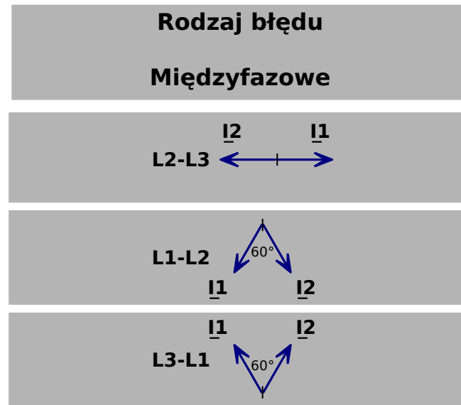
Rys. 90: Fazory (wskazy) prądu składowej zgodnej i przeciwnej przy różnych typach zwarć.
