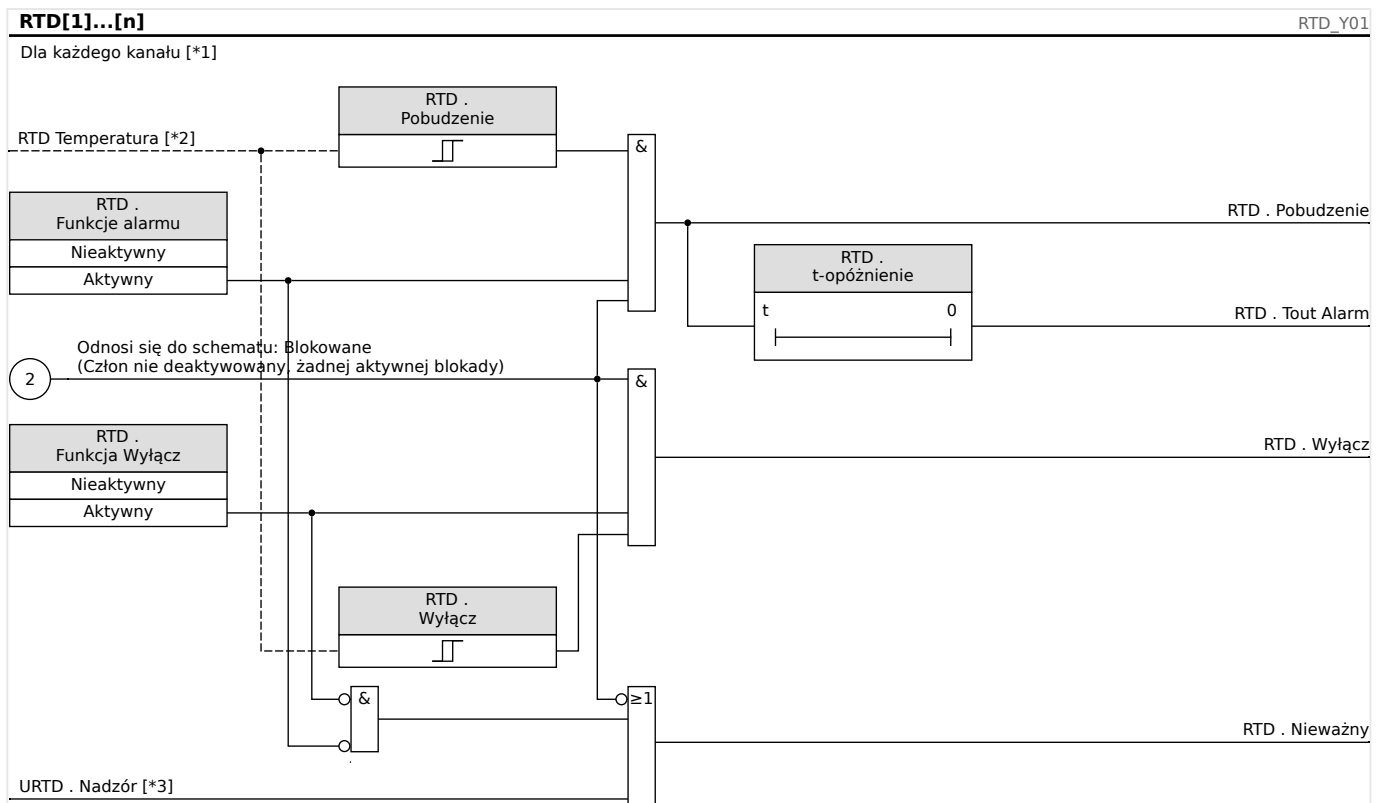
Rys. 148: Ogólna zasada działania (alarm z opóźnieniem, wyzwolenie bezzwłoczne).
