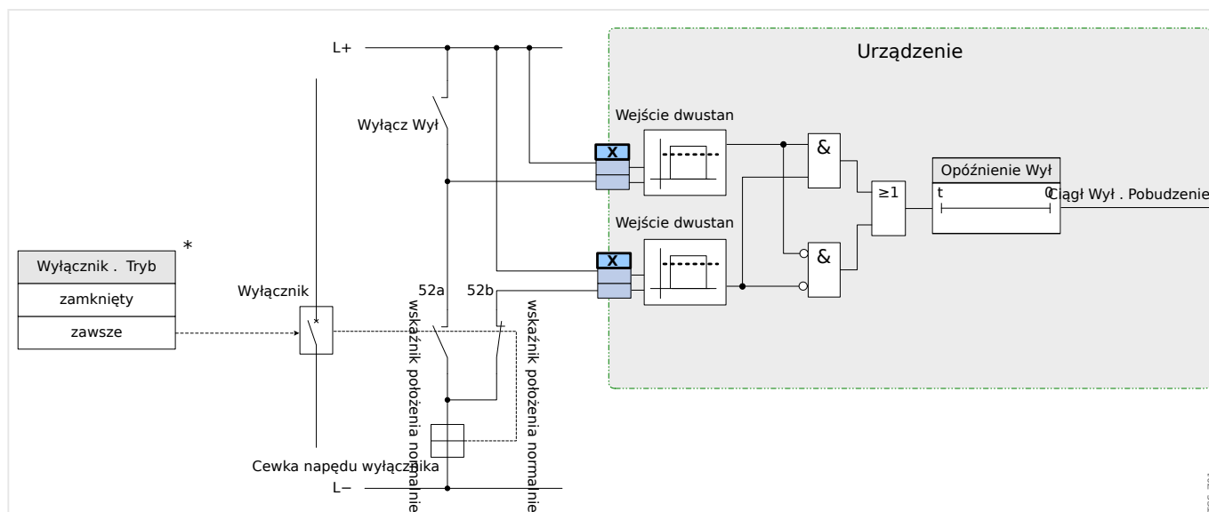
Rys. 150: Przykład okablowania: Układ kontroli ciągłości obwodów wyłącznika z dwoma stykami pomocniczymi wyłącznika „Położ ZAŁ” (52a) i „Położ WYŁ” (52b).
