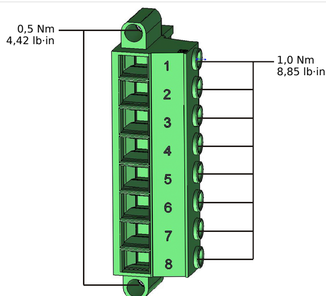
Rys. 175: Zaciski pomiaru napięcia karty pomiarowej „TU” (↳ „TU — wejścia do pomiaru napięcia”).
