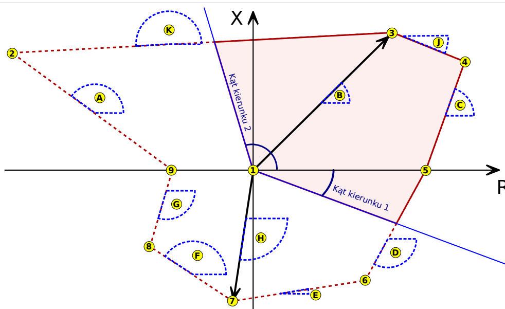
Rys. 95: Obszar roboczy (w kolorze jasnoczerwonym) typu poligonalnego, przy „Włączanie kierunku” = „Aktywny”.
