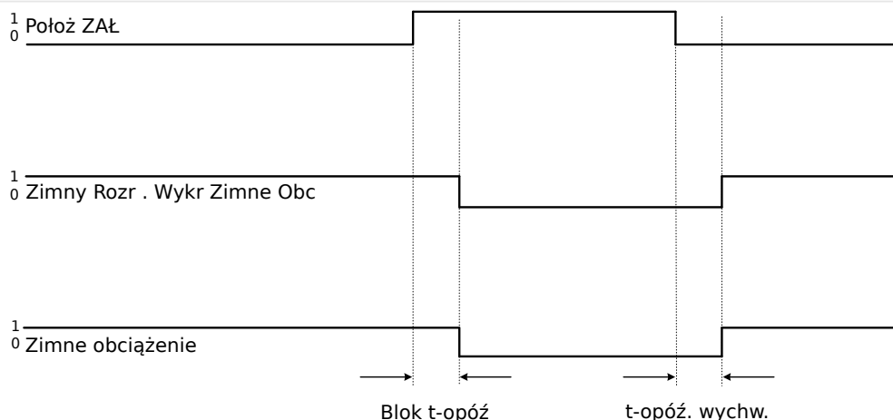
Rys. 119: Przykładowy tryb: Położenie wyłącznika.
