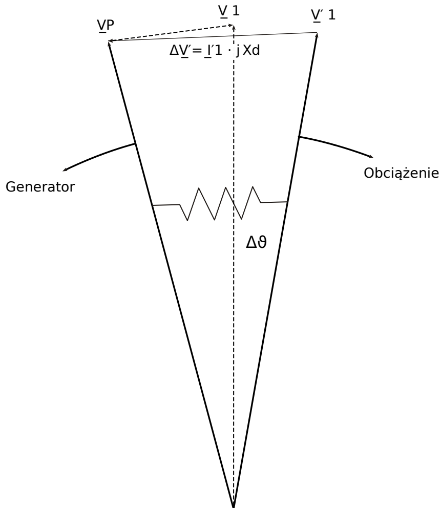
Rys. 132: Wektory napięcia przy awarii sieci.
