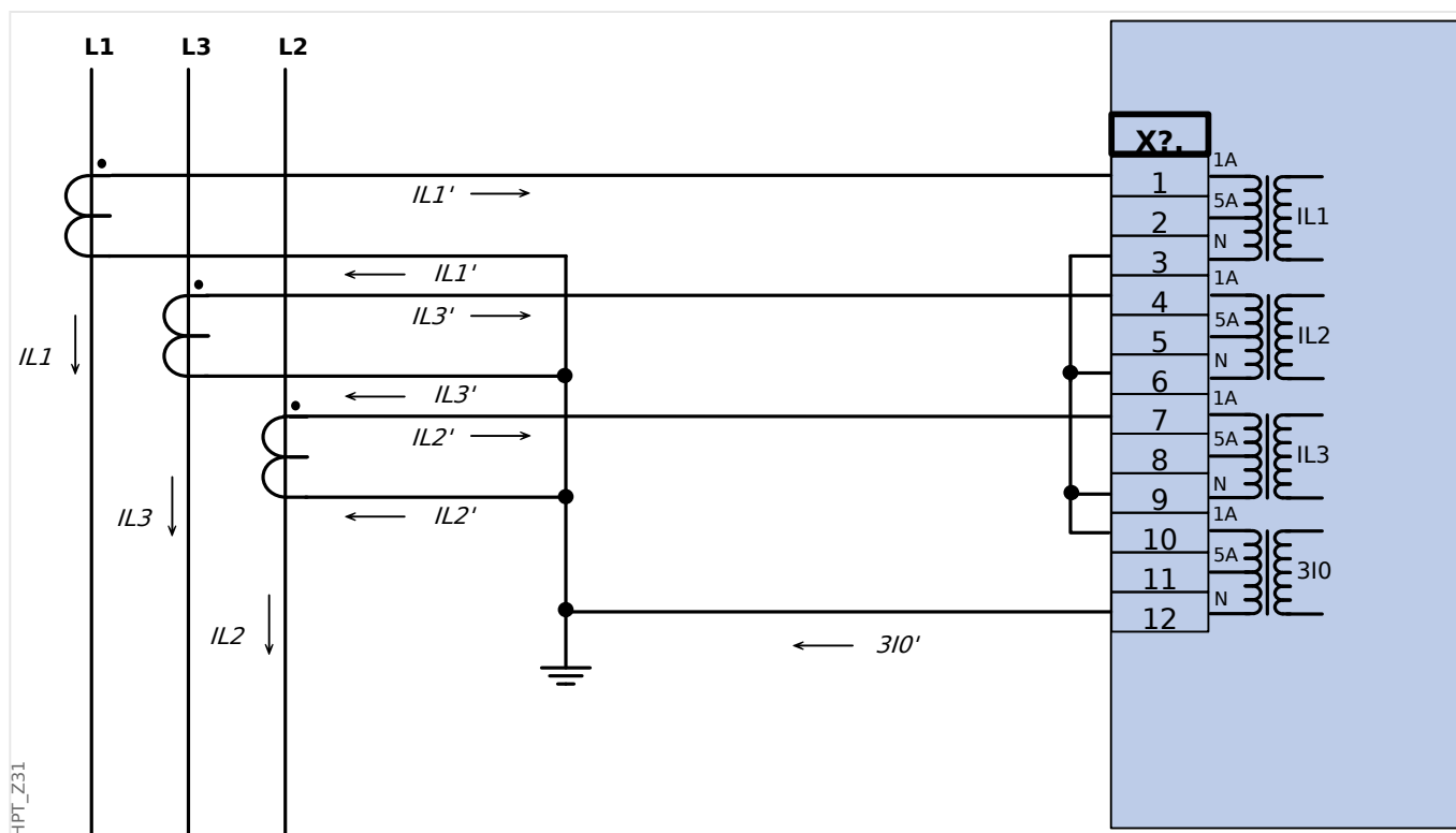
Rys. 25: Trójfazowy pomiar prądu; I_n wtórny = 1 A. Pomiar prądu doziemnego w układzie Holmgreena 3I_0 wtórny = 1 A.
