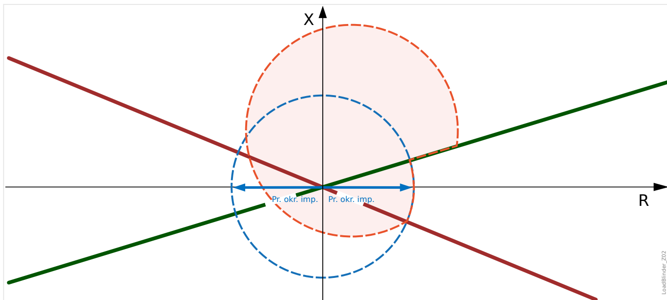
Rys. 109: Strefa wyzwania zabezpieczenia odległościowego (czerwony obszar) przy aktywnym ograniczniku obciążenia.
