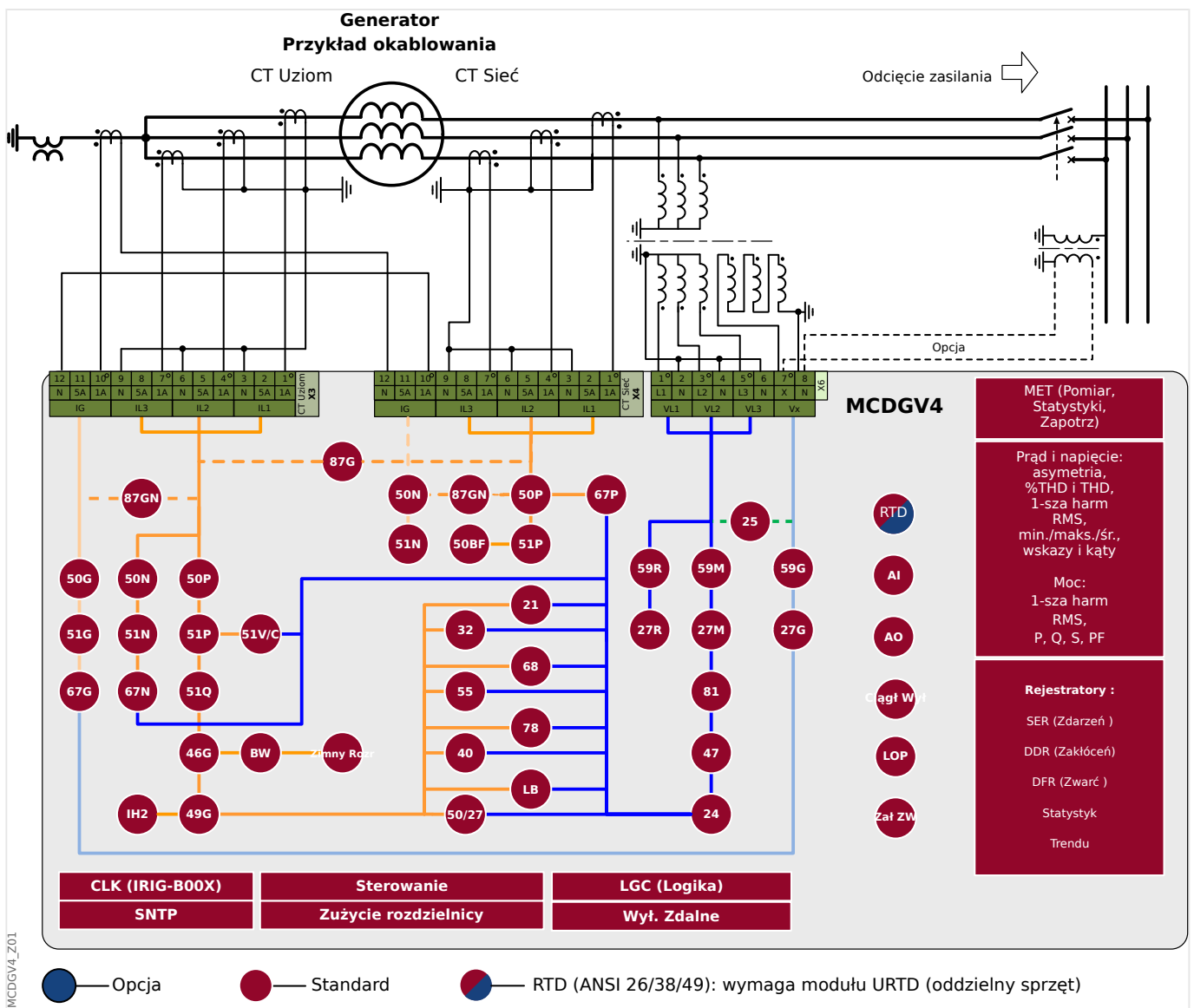
Rys. 1: Opis funkcjonalny MCDGV4
