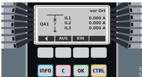
Abb. 154: Beispiel einer Steuer-Seite mit „Leistungsschalter“ in Störstellung (bzw. unplausiblem Zustand).
