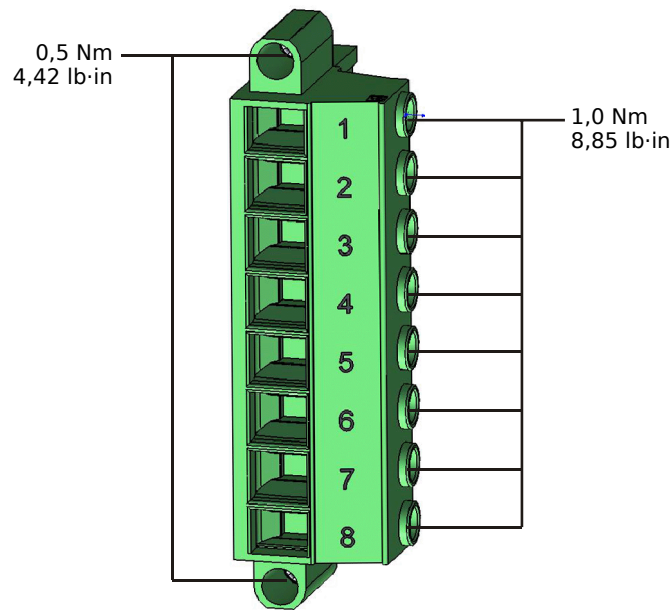
Abb. 174: Spannungsmessstecker der Spannungsmesskarte „TU“ (↳ „TU - Spannungsmesseingänge“).
