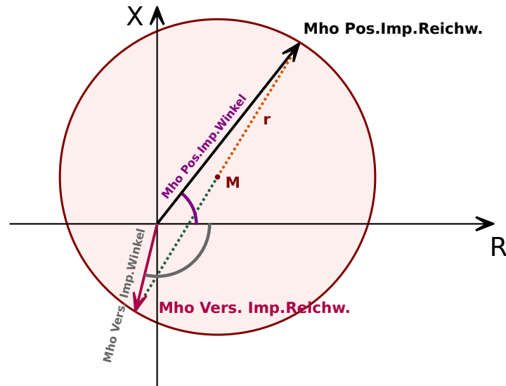
Abb. 91: Impedanzcharakteristik (hellrote Fläche) vom Typ MHO (Kreis), mit inaktiver Richtungserfassung.
