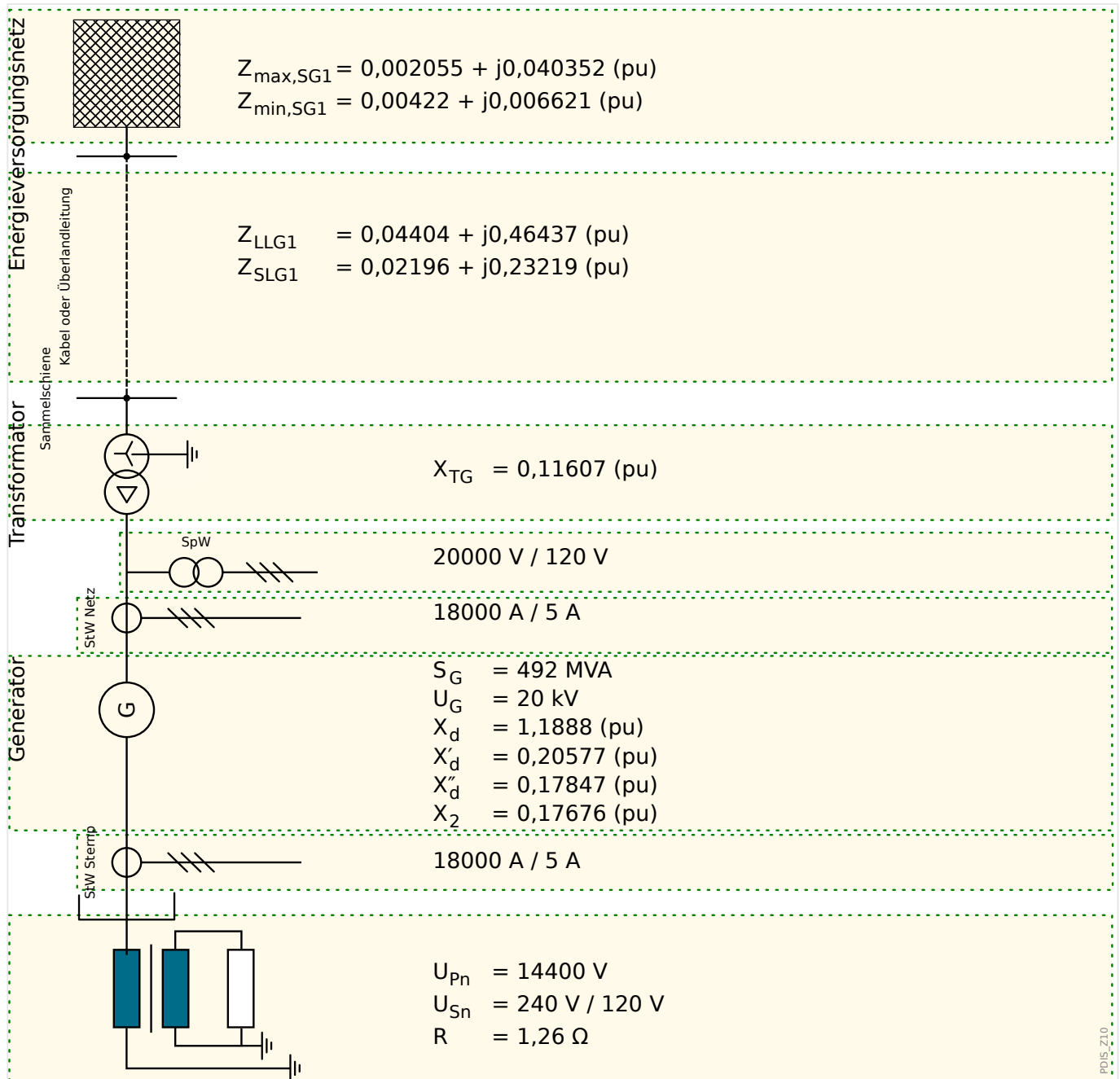
Abb. 98: Abzweigbild mit generatorbasierten Daten.
