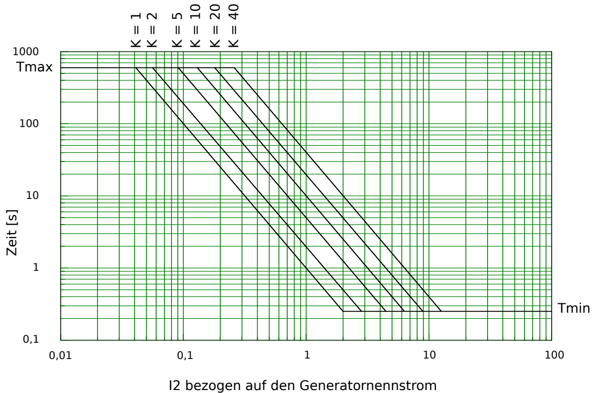
Abb. 112: Schieflastauslösekennlinien.
