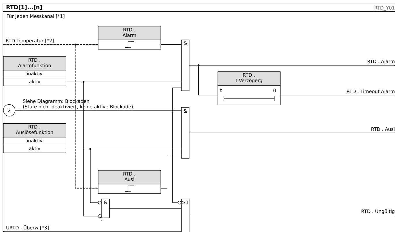
Abb. 147: Generelles RTD-Funktionsprinzip.
