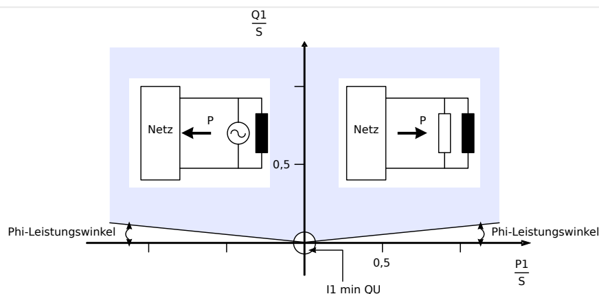
Abb. 139: Variante 1: Leistungswinkelüberwachung.
