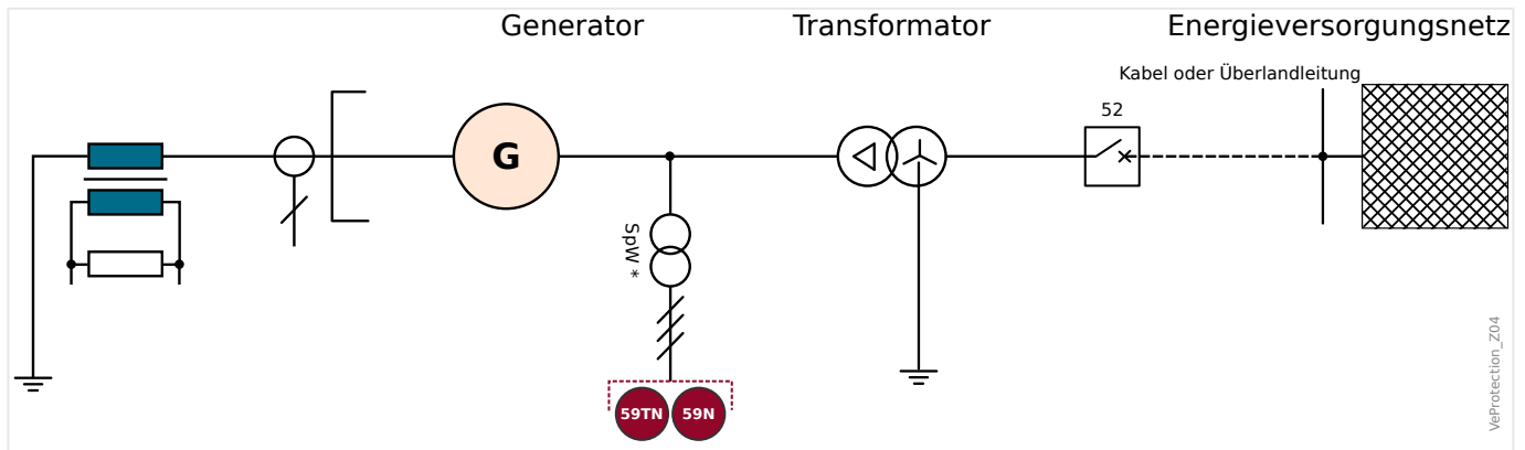
Abb. 127: 100% Stator-Erdfehler-Schutz mittels ANSI 59TN/59N-Kombination.
