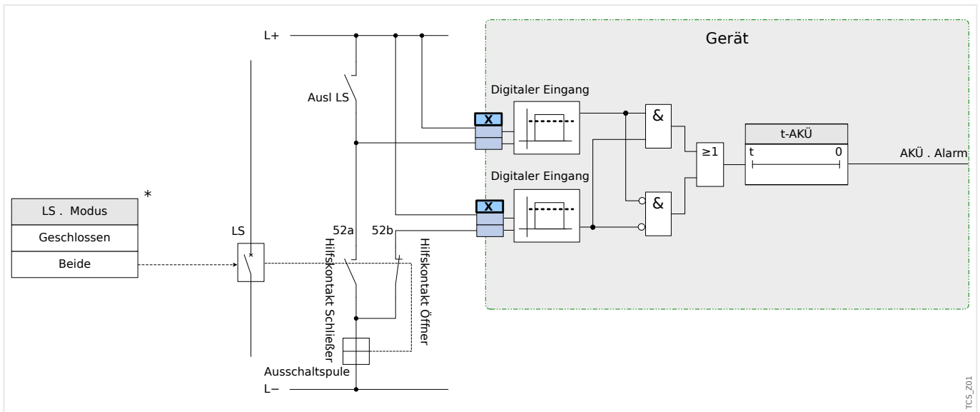
Abb. 149: Anschlussbeispiel (Empfehlung): Auslösekreisüberwachung mit zwei Hilfskontakten »Hiko EIN« (52a) und »Hiko AUS« (52b).
