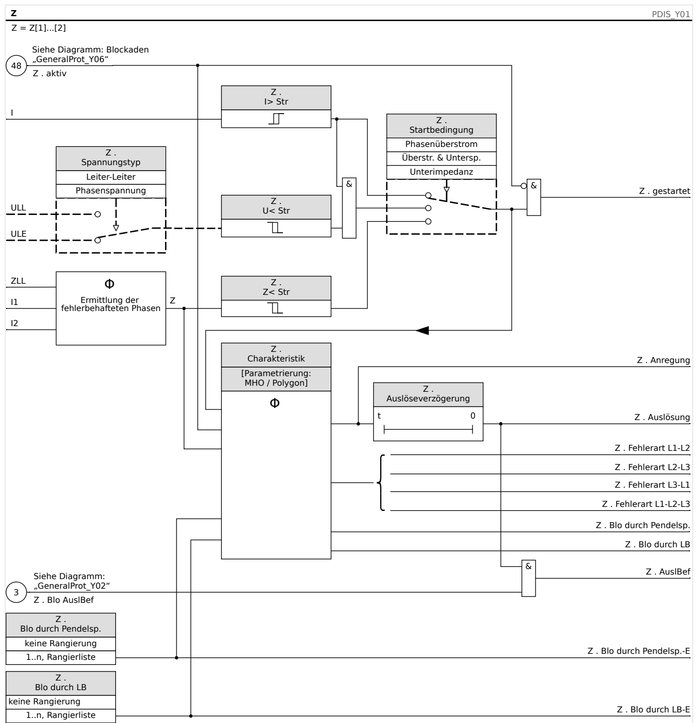
Abb. 96: Funktionalität des Phasendistanzschutzes.
