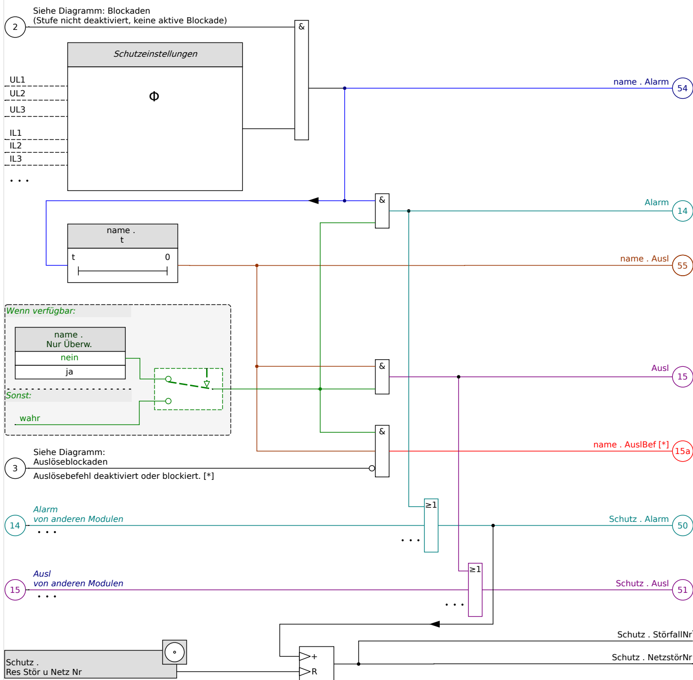
Abb. 71: Grobe Skizze der Funktionalität einer HighPROTEC-Schutzfunktion.
