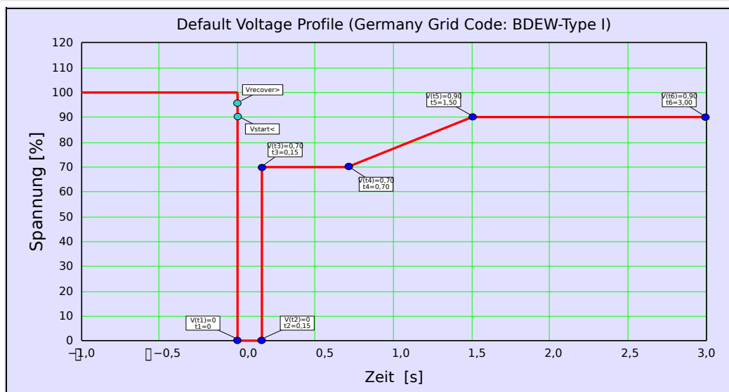
Abb. 144: LVRT-Werkseinstellung (BDEW-Typ-I).
