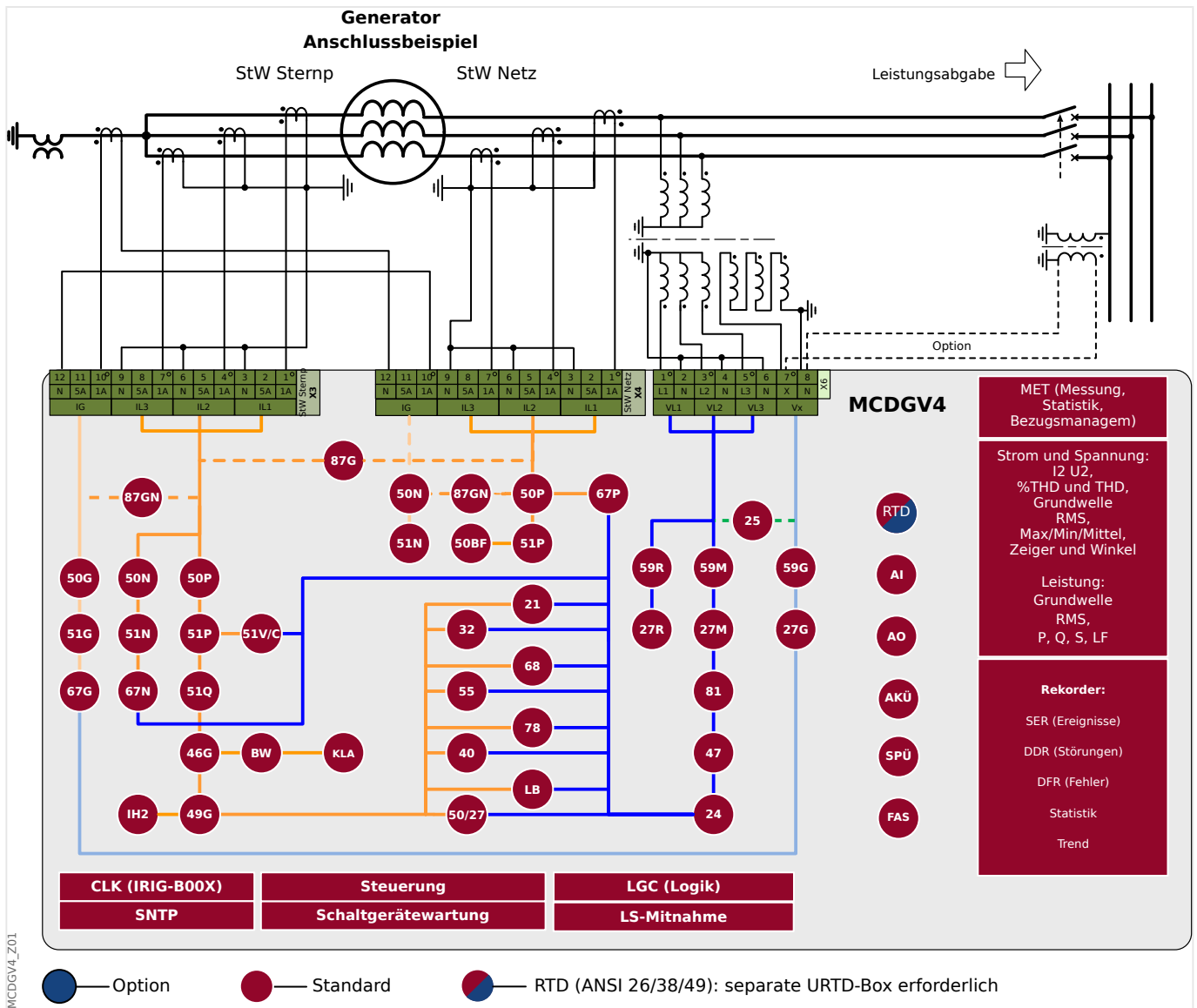
Abb. 1: Funktionsübersicht für das MCDGV4.
