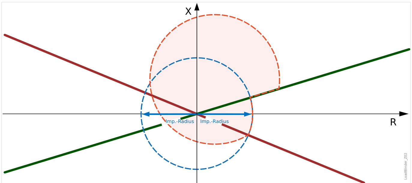
Abb. 108: Auslösebereich des Distanzschutzes (hellrote Fläche) bei aktiver Lastausblendung.
