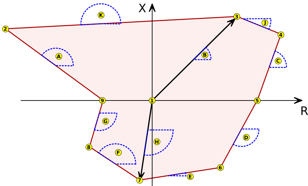
Abb. 93: Impedanzcharakteristik (hellrote Fläche) vom Typ Polygon mit inaktiver Richtungserfassung.
