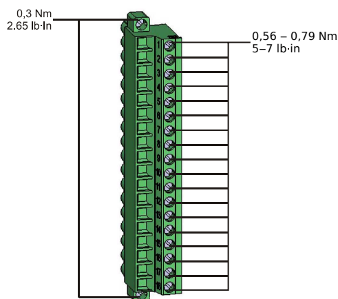
Abb. 175: Spannungsmessstecker der Spannungsmesskarten „TU-OR5“ und „TU-DI8“.
