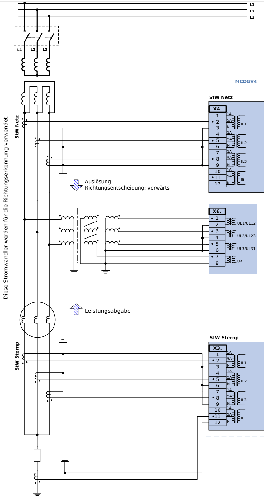
Abb. 47: Niedrohmgig geerdeter Generatorsternpunkt und Step-UP Trafo – nur Phasendifferenzialschutz.
