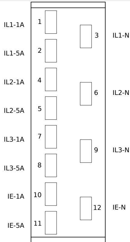
Abb. 17: TI - Elektromechanische Zuordnung
