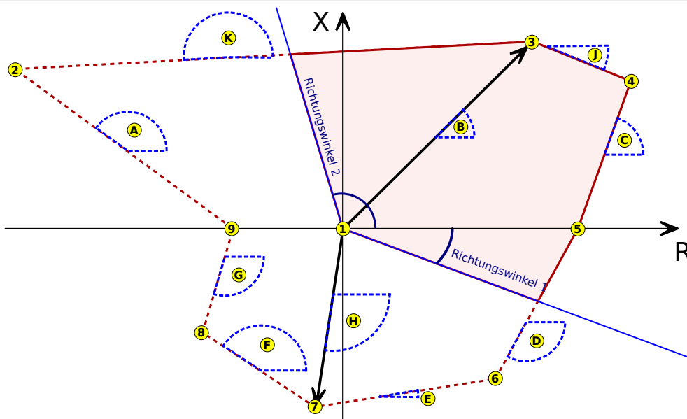
Abb. 94: Impedanzcharakteristik (hellrote Fläche) vom Typ Polygon mit aktivierter Richtungserfassung.
