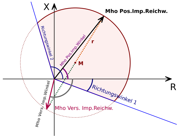
Abb. 92: Impedanzcharakteristik (hellrote Fläche) vom Typ MHO (Kreis), mit aktivierter Richtungserfassung.
