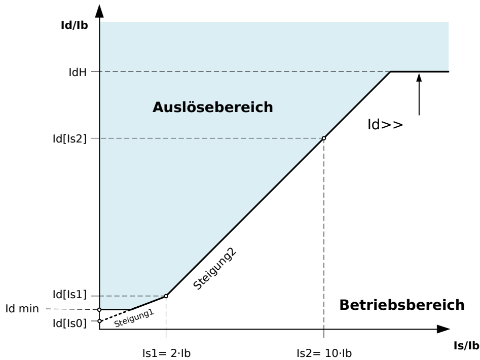
Abb. 85: Unstabilisierte Hochstromdifferenzialstufe I_{dH} .
